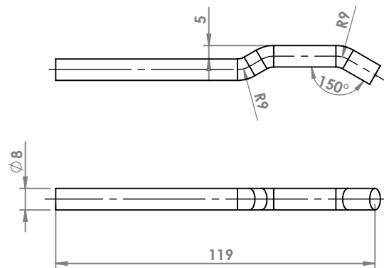
AUTO VARIE ATTACCO COD. AT 010067
