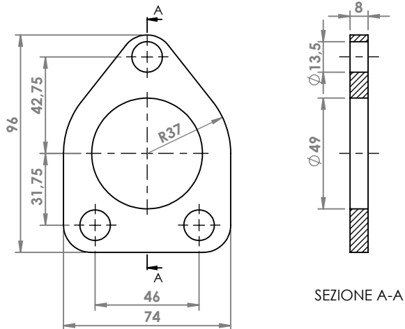
VOLVO V40 FLANGIA COD. FL 881301
