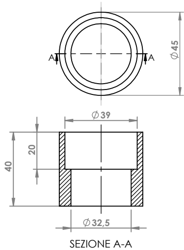
AUTO VARIE ANELLO COD. AN 715
