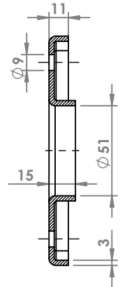
SEZIONE A-A
