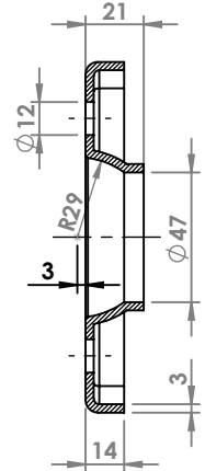
SEZIONE A-A
