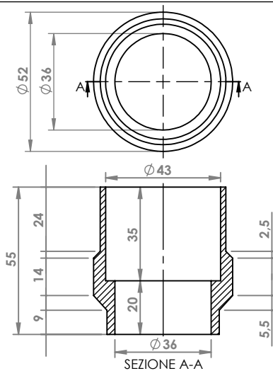
AUTO D'EPOCA ANELLO COD. AN 010051
