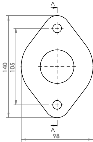
NISSAN FLANGIA COD. FL 500006
