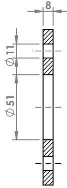
SEZIONE A-A
