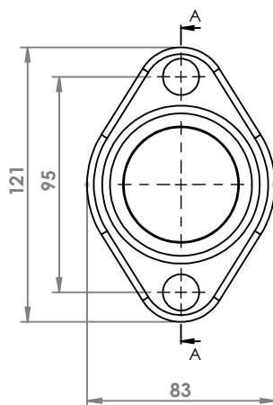
SUBARU LEGACY FLANGIA COD. FL 700102
