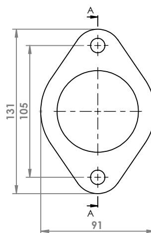
FORD FLANGIA COD. FL 260042
