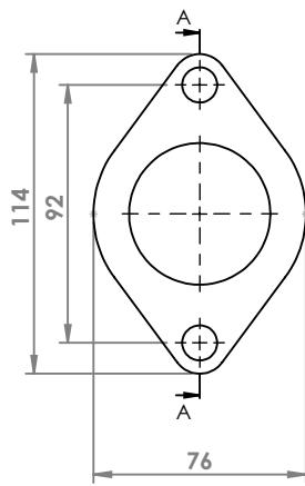
HYUNDAI FLANGIA COD. FL 300003
