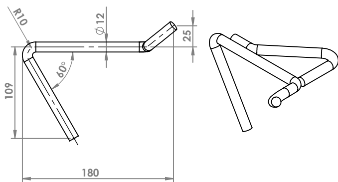
OPEL ASTRA 1.4 16V '05 ATTACCO COD. AT 520949
