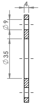
SEZIONE A-A
