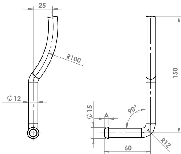
FIAT DUCATO 2.3 JTD TURBO DIESEL ATTACCO COD. AT 241513
