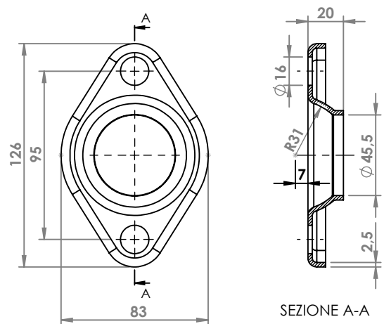
MAZDA FLANGIA COD. FL 420005
