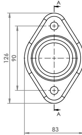
MAZDA FLANGIA COD. FL 420007
