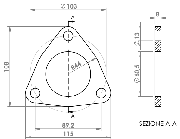
VOLVO S40 - V40 FLANGIA COD. FL 880905
