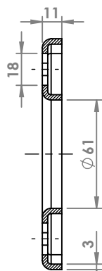
SEZIONE A-A
