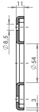
SEZIONE A-A
