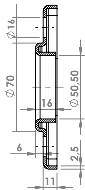
SEZIONE A-A
