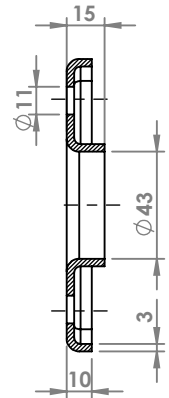
SEZIONE A-A
