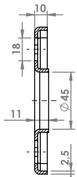
SEZIONE A-A
