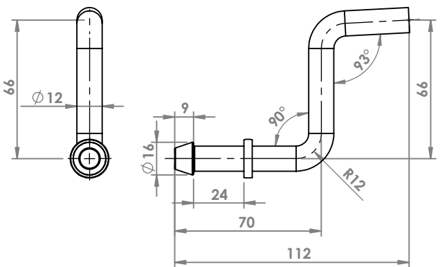
MERCEDES CLASSE A ATTACCO COD. AT 440710
