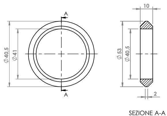
CITROEN AX 10 ANELLO \phi esterno mm 53 \phi interno mm 40,50 COD. AN 140701
