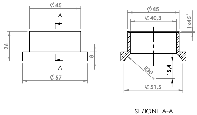
CITROEN PEUGEOT ANELLO \phi esterno mm 57 COD. AN 140001
