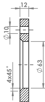
SEZIONE A-A
