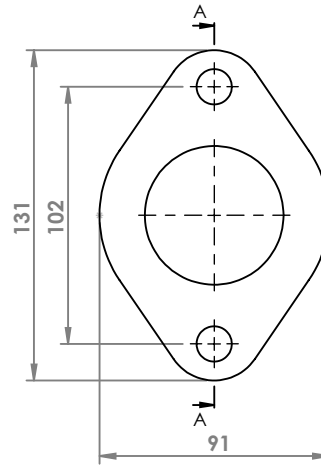
HYUNDAI FLANGIA COD. FL 300004
