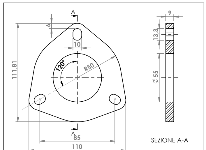
FIAT MAREA/BRAVA FLANGIA COD. FL 240032
