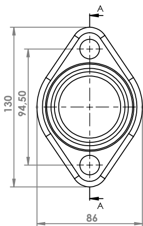
AUTO VARIE FLANGIA COD. FL 010069
