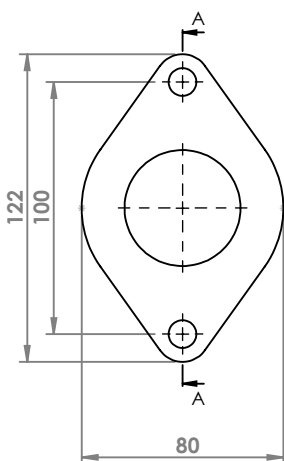
FORD FIESTA FLANGIA COD. FL 260379
