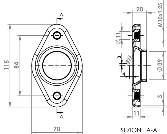
TOYOTA YARIS 1.0 16V '99 FLANGIA COD. FL 801210 / IM
