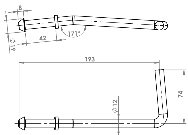
PEUGEOT 206 1.4 - 1.6 16V '05 ATTACCO COD. AT 541236
