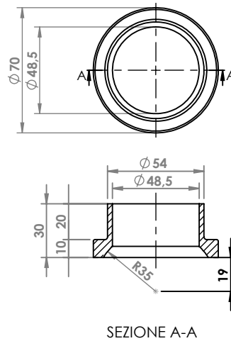
FIAT DUCATO ANELLO \varnothing esterno mm 70 \varnothing interno mm 48,5 COD. AN 241501
