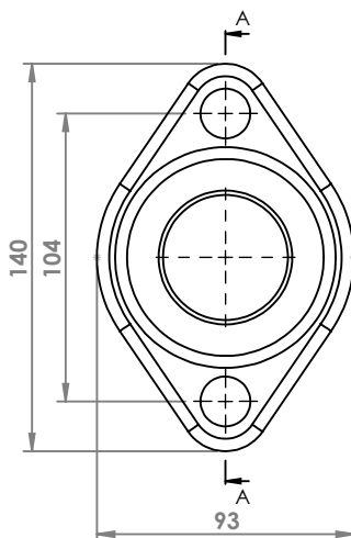
NISSAN FLANGIA COD. FL 500010
