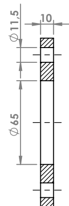
SEZIONE A-A
