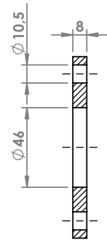
SEZIONE A-A
