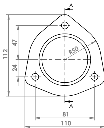
AUTO VARIE FLANGIA COD. FL 010053
