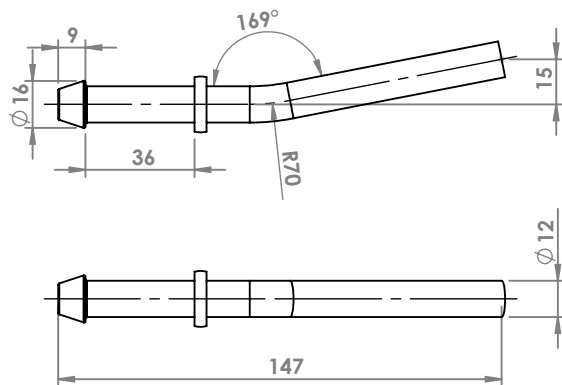
MERCEDES CLASSE A ATTACCO COD. AT 440709
