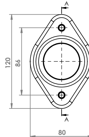
HONDA JAZZ FLANGIA COD. FL 281113
