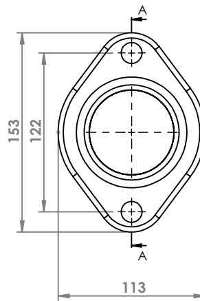
NISSAN FLANGIA COD. FL 500009
