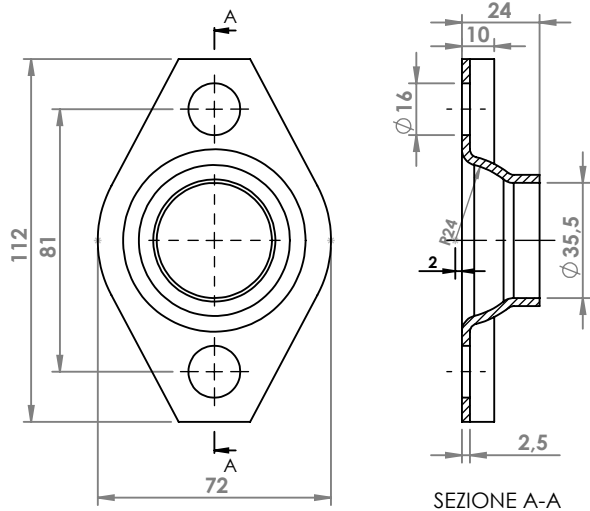
TOYOTA FLANGIA COD. FL 800016
