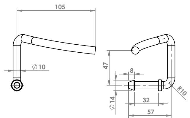
BMW SERIE 1 ATTACCO COD. AT 120902
