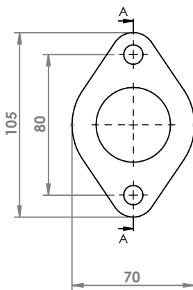
NISSAN FLANGIA COD. FL 500008
