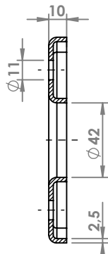
SEZIONE A-A
