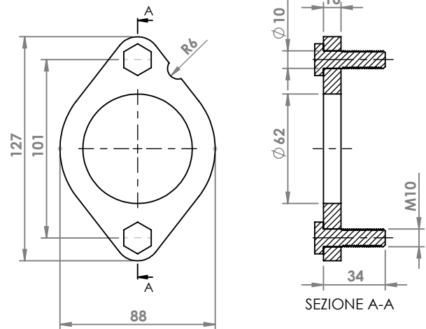
VOLVO FLANGIA COD. FL 880002
