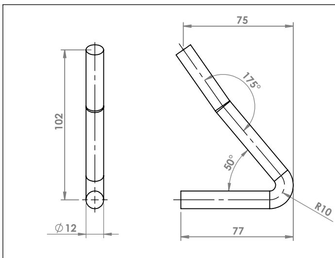
CITROEN BERLINGO ATTACCO COD. AT 141310
