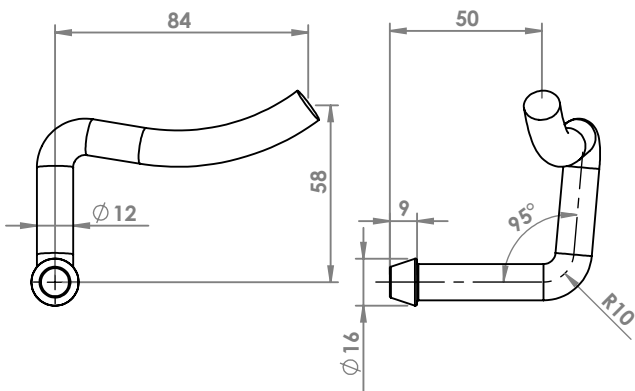
BMW SERIE 1 ATTACCO COD. AT 120908
