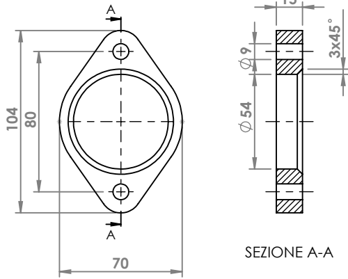
OPEL ASTRA FLANGIA COD. FL 520959
