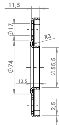
SEZIONE A-A
