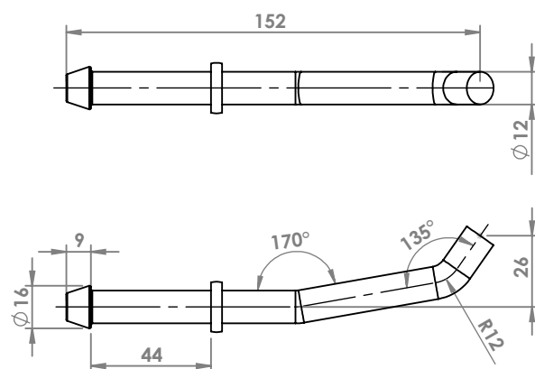
CITROEN C3 1.6 '02 ATTACCO COD. AT 141606
