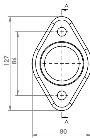
FIAT SEDICI FLANGIA COD. FL 243902
