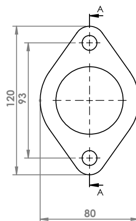
AUTO VARIE FLANGIA COD. FL 010071
