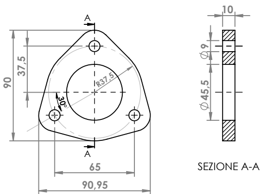
LANCIA 2000 I FLANGIA COD. FL 380002
