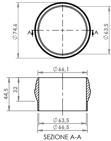
AUTO VARIE ANELLO COD. AN 010036
