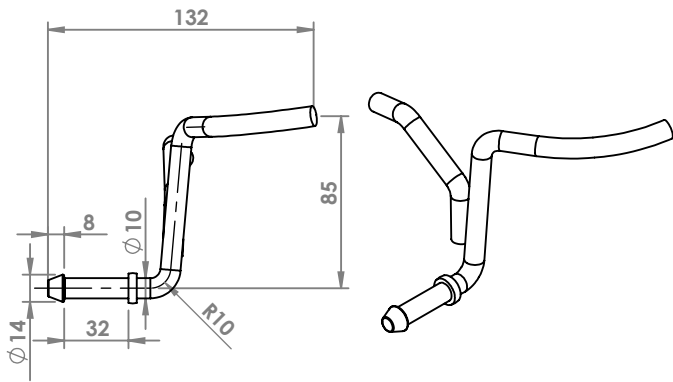
BMW SERIE 1 ATTACCO COD. AT 120903
