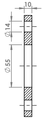
SEZIONE A-A
