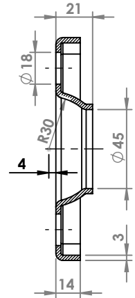
SEZIONE A-A
