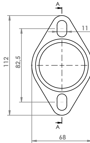
FORD FIESTA DIESEL FLANGIA COD. FL 260365
