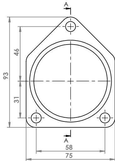
MERCEDES E250 TD FLANGIA COD. FL 441201
