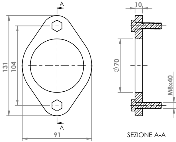
VOLVO V70 2.4 20V SW FLANGIA COD. FL 881103
