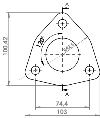
HONDA FLANGIA COD. FL 280009
