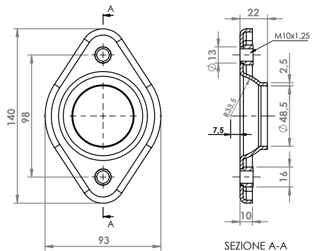
TOYOTA FLANGIA COD. FL 800021
