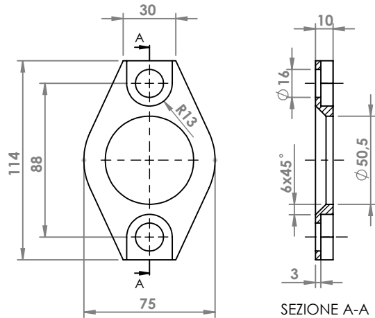
RENAULT CLIO 1.9 D FLANGIA COD. FL 601330
