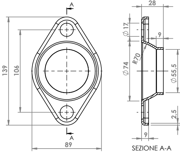
SUZUKI VITARA FLANGIA COD. FL 720118
