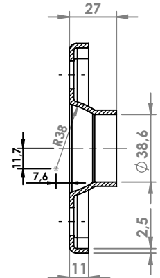
SEZIONE A-A
