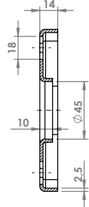
SEZIONE A-A
