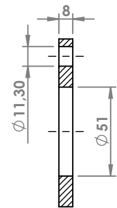
SEZIONE A-A
