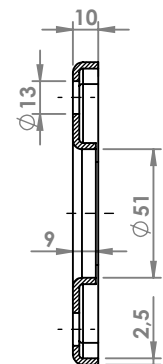
SEZIONE A-A
