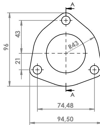
AUTO VARIE FLANGIA COD. FL 010059
