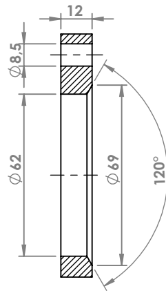
SEZIONE A-A
