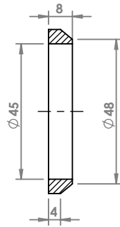
SEZIONE A-A
