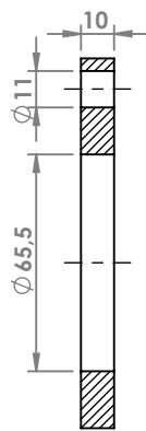
SEZIONE A-A
