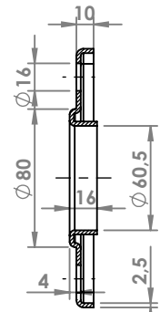
SEZIONE A-A
