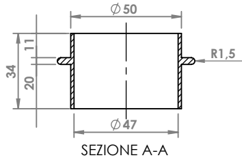
SEZIONE A-A
