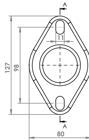
NISSAN ALMERA FLANGIA COD. FL 500708
