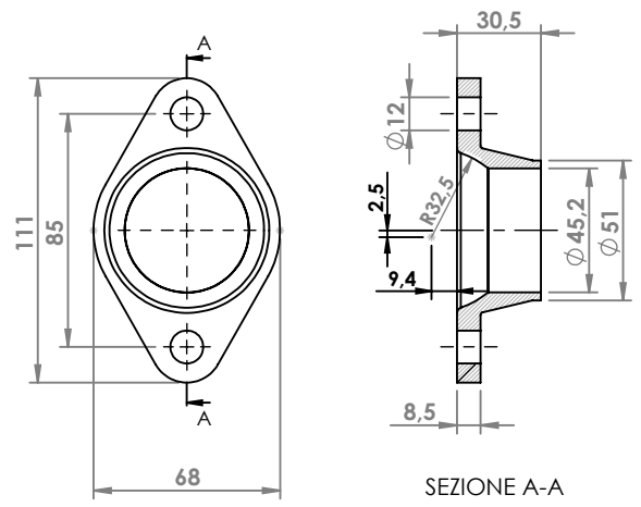
PEUGEOT FLANGIA COD. FL 540006
