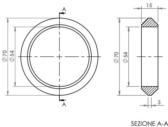
CITROEN BX GTI ANELLO \phi esterno mm 70 \phi interno mm 54 COD. AN 140305
