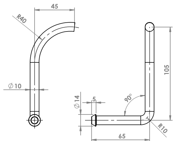
FIAT BRAVO 1.4 '07 TURBO JET ATTACCO COD. AT 242349
