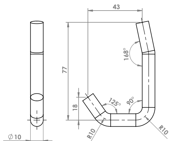
AUTO VARIE ATTACCO COD. AT 010039
