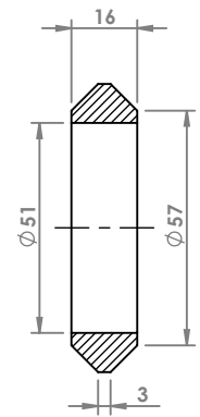
SEZIONE A-A
