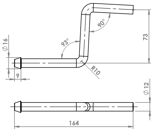
PEUGEOT 206 1.4 HDI '01 ATTACCO COD. AT 541239
