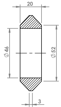
SEZIONE A-A
