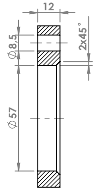
SEZIONE A-A
