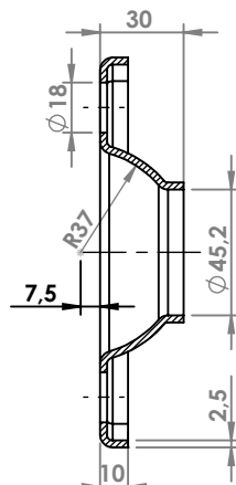
SEZIONE A-A
