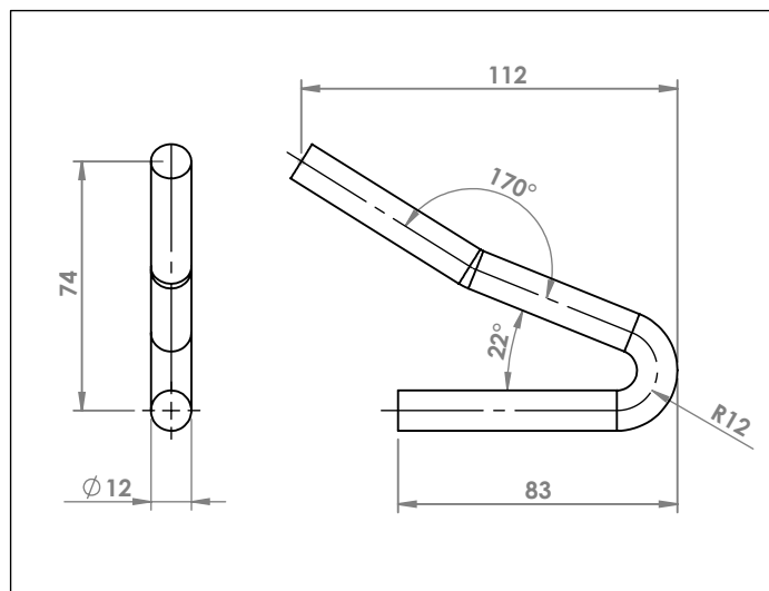
CITROEN BERLINGO ATTACCO COD. AT 141311
