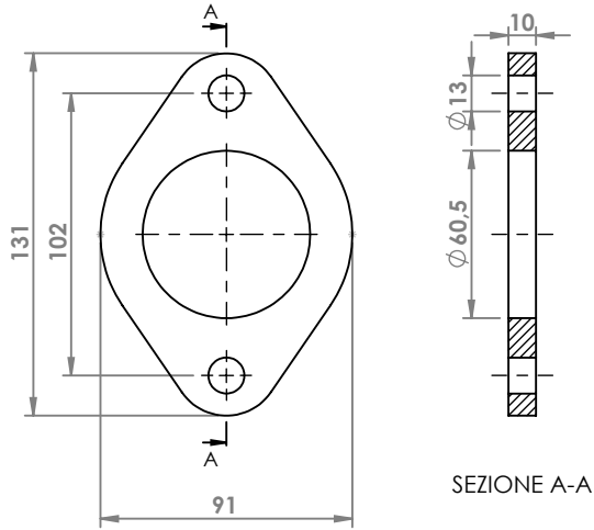
KIA SORENTO FLANGIA COD. FL 310501
