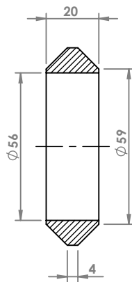
SEZIONE A-A
