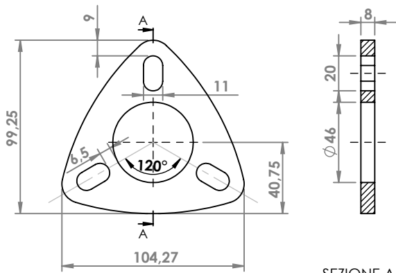
SEZIONE A-A
