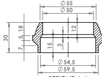
SEZIONE A-A
