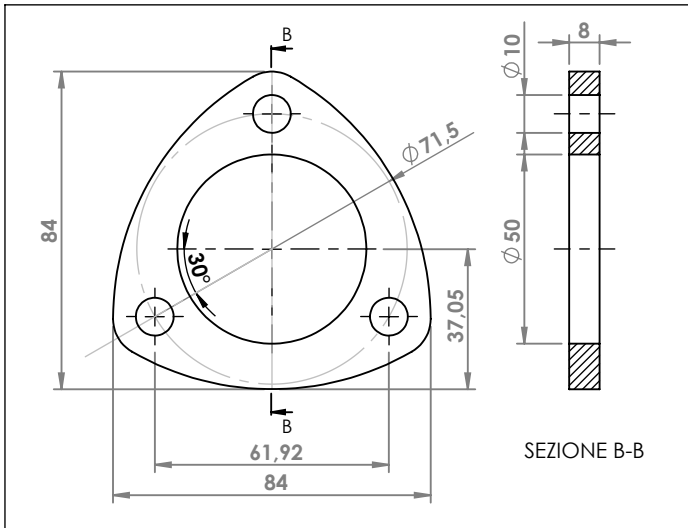
VW FLANGIA COD. FL 860041
