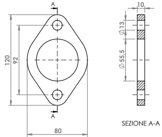
KIA SORENTO FLANGIA COD. FL 310502
