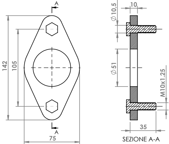
FORD MONDEO 1.6 1.8 FLANGIA COD. FL 261216/ PD
