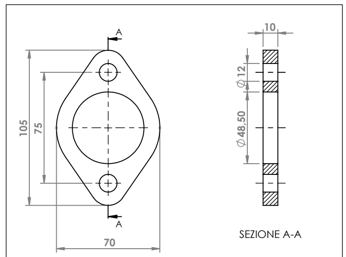
BMW FLANGIA COD. FL 120038
