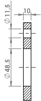
SEZIONE A-A
