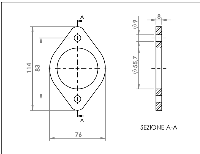
VW GOLF FLANGIA COD. FL 860141
