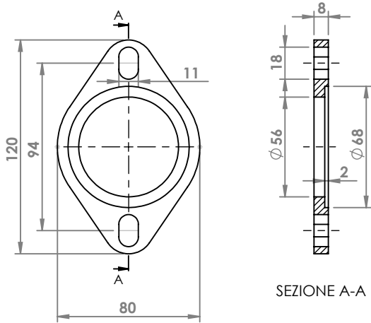
TOYOTA FLANGIA COD. FL 800023
