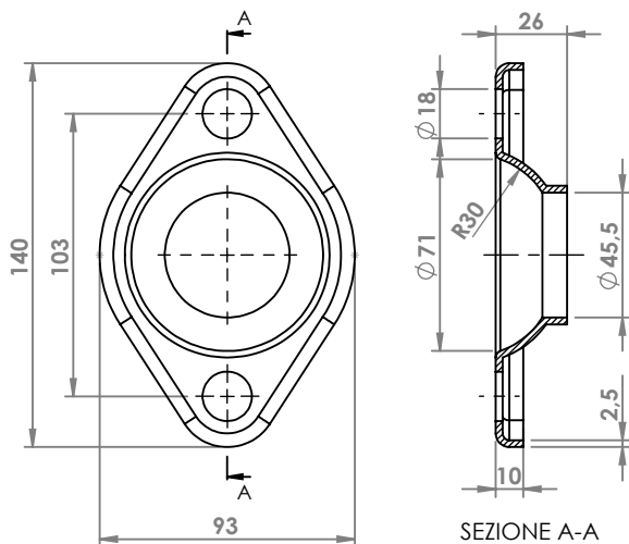
RENAULT CLIO 3 FLANGIA COD. FL 601331
