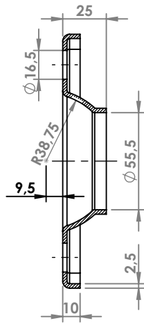
SEZIONE A-A
