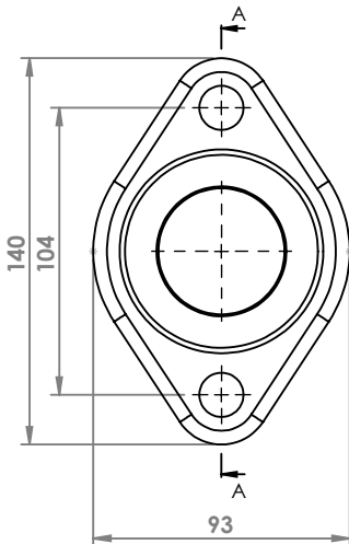
SUZUKI FLANGIA COD. FL 720003
