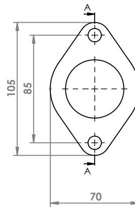
HYUNDAI GETZ FLANGIA COD. FL 300605
