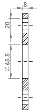
SEZIONE A-A
