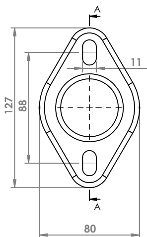
NISSAN JUKE FLANGIA COD. FL 501004
