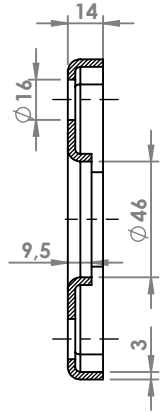
SEZIONE A-A
