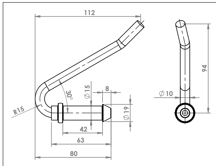
CITROEN BERLINGO ATTACCO COD. AT 141305
