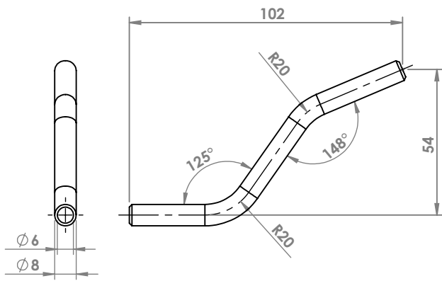
AUTO VARIE ATTACCO COD. AT 010032
