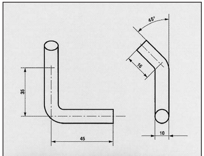
HONDA CRX 1500/88 ATTACCO per posteriore COD. AT 280507
