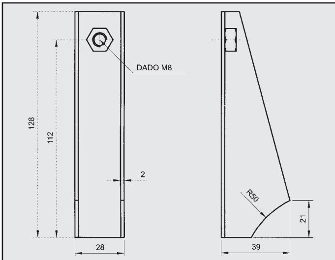
SUZUKI VITARA ATTACCO per posteriore COD. AT 720110
