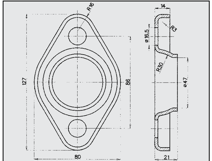
HONDA CIVIC 1.4 CAT FLANGIA COD. FL 280426
