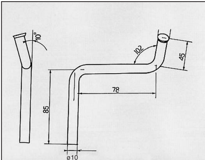
323 ATTACCO centrale COD. AT 420602
