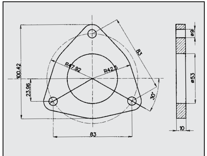
ALFA ROMEO 146 JTD FLANGIA COD. FL 021109
