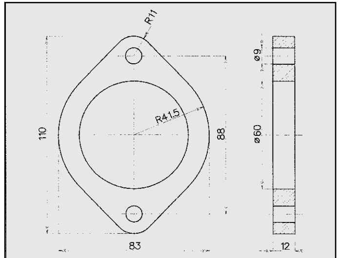
FIAT BRAVO - MAREA 2.0 KAT FLANGIA COD. FL 242323
