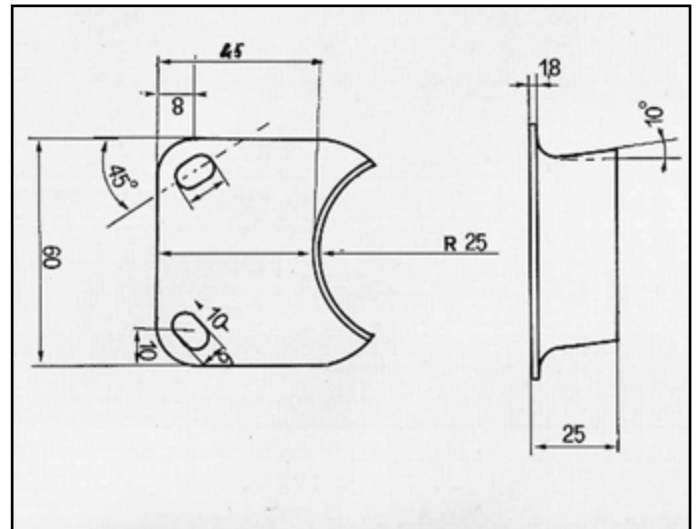
132 ATTACCO per centrale COD. R 240701
