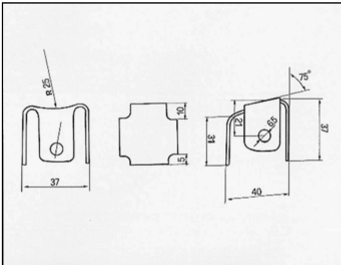
238-B B1-E ATTACCO per posteriore coda COD. AT 241301
