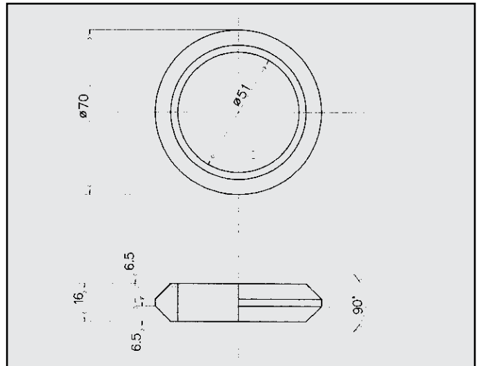
RENAULT CLIO ANELLO COD. AN 601301
