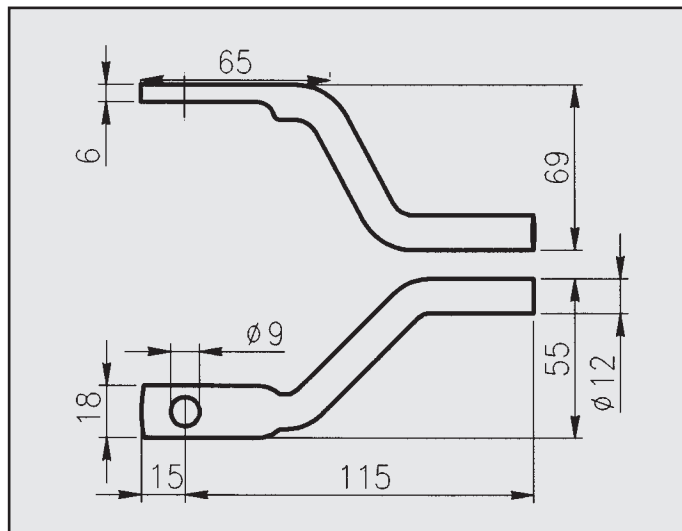
MITSUBISHI PAJERO '90 ATTACCO centrale COD. AT 460211
