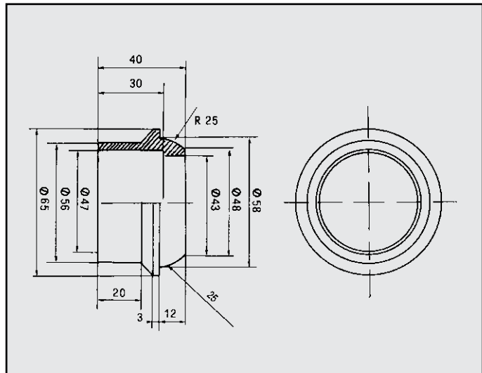
MITSUBISHI COLT 1200 - 1400 ANELLO per anteriore COD. AN 460102
