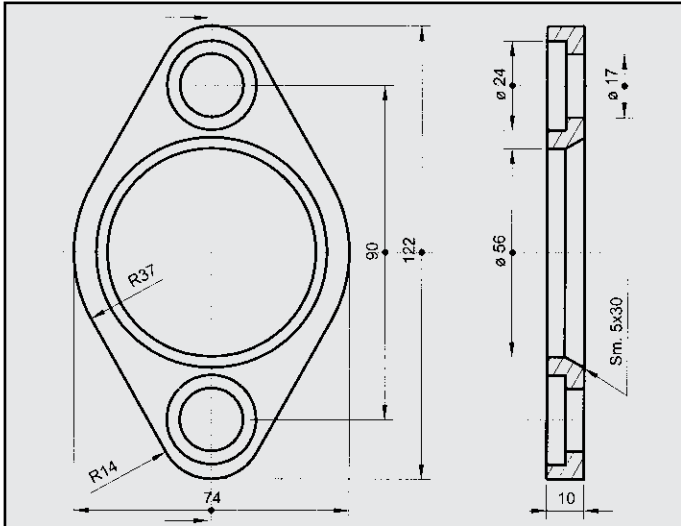
AUTOBIANCHI Y10 1.3 FLANGIA COD. FL 080220
