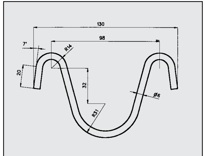
FIAT 131 DIESEL PANORAMA ATTACCO per posteriore COD. AT 240607
