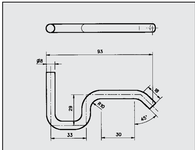
CITROEN GS 1050-1220 ATTACCO per posteriore COD. AT 140401 5490566
