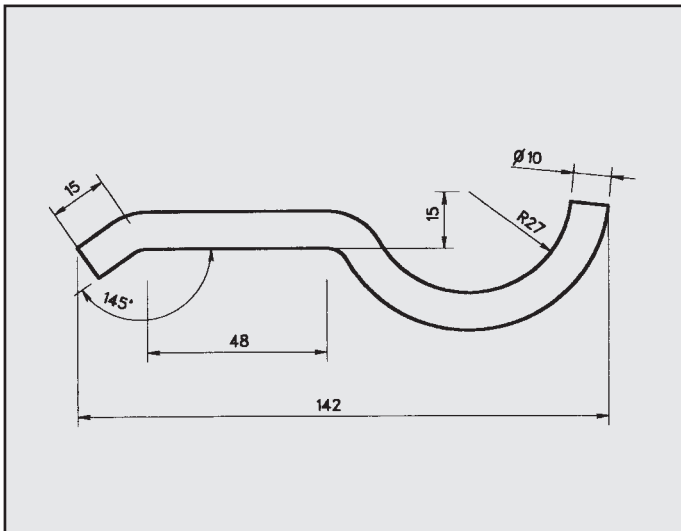
RENAULT R19 CHAMADE ATTACCO per centrale COD. AT 600904
