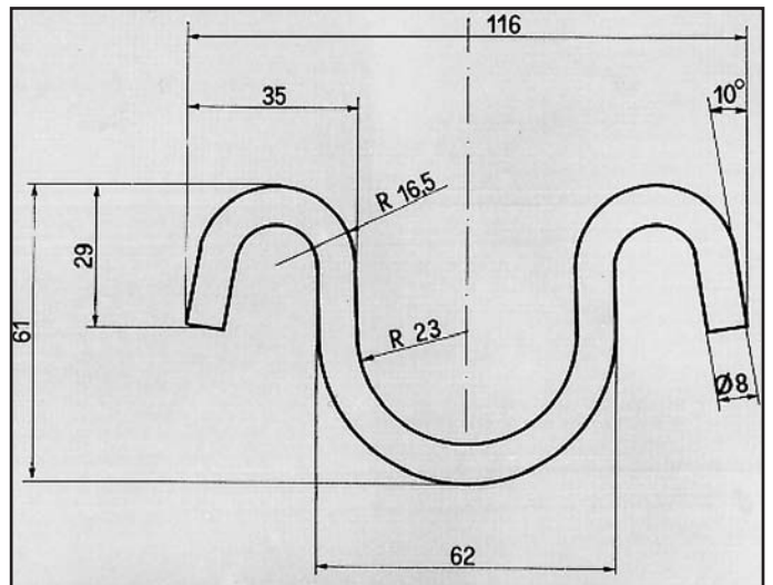
SEAT RONDA ATTACCO per posteriore COD. AT 680202
