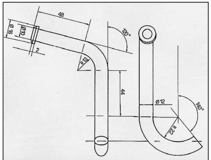
CAMRY 2 ATTACCO per centrale COD. AT 800103
