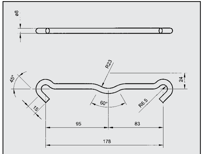
FIAT FIORINO 1.7 DIESEL ATTACCO per collettore COD. AT 241802
