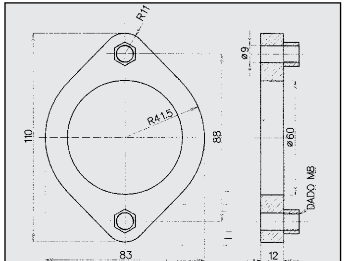
FIAT BRAVO - MAREA 2.0 KAT FLANGIA COD. FL 242324
