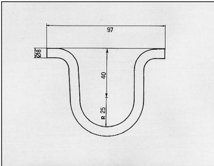
IBIZA RINFORZO per posteriore COD. R. 680101
