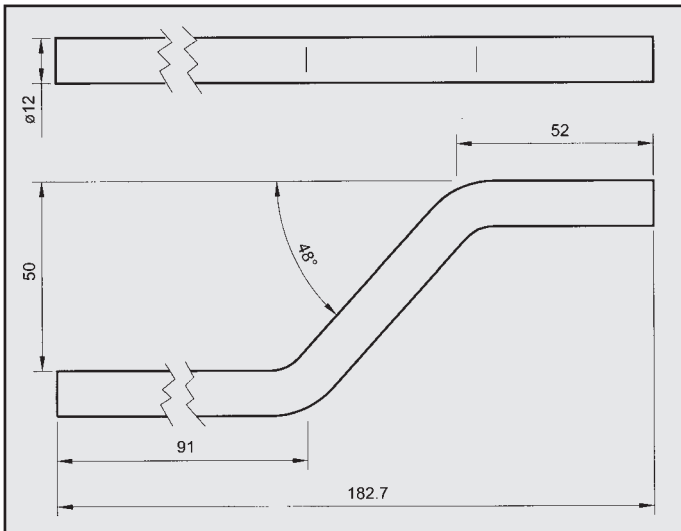
LANCIA DEDRA ATTACCO COD. AT 380812
