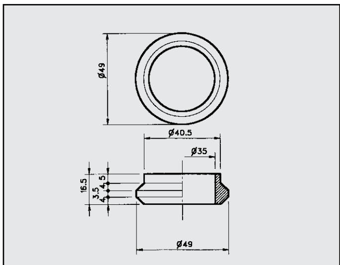
CITROEN DYANE 4 - 6 ANELLO per collettore ø esterno mm 49 ø interno mm 35 COD. AN 140802
