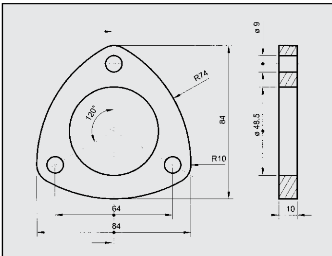
LANCIA DELTA 1.6 FLANGIA COD. FL 380336
