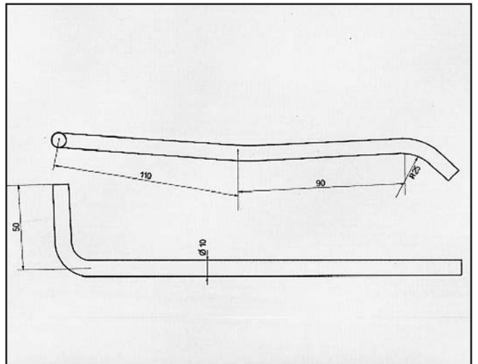
NEW CITY 1.3 RINFORZO COD. R 280803
