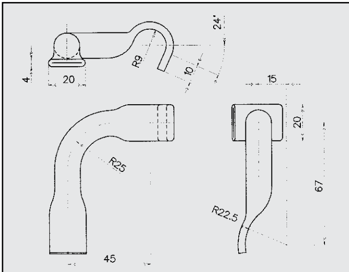
AUTOBIANCHI Y 10 ATTACCO CENTRALE COD. AT 080221
