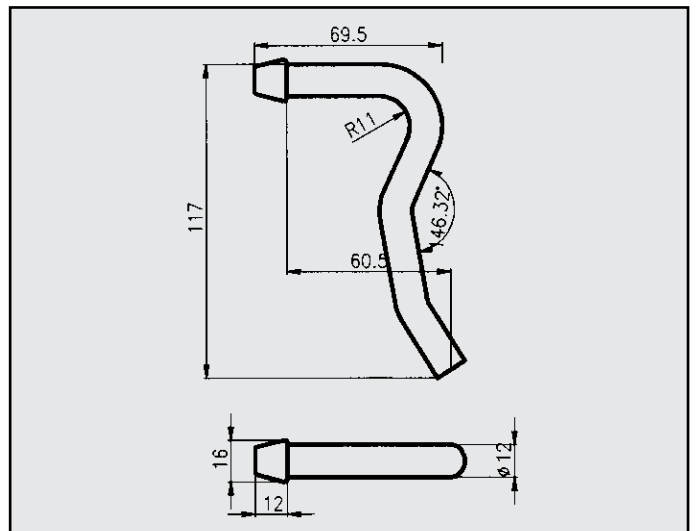
FIAT MULTIPLA ATTACCO per centrale COD. AT 242602
