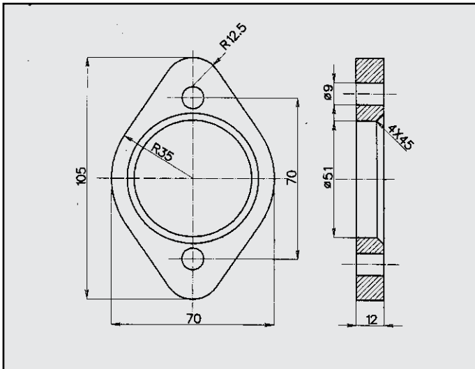
BMW 325 FLANGIA COD. FL 120504
