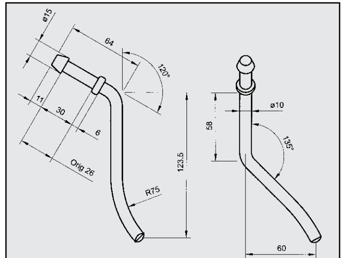
BMW 316 1.6 COMPACT ATTACCO per posteriore COD. AT 120114
