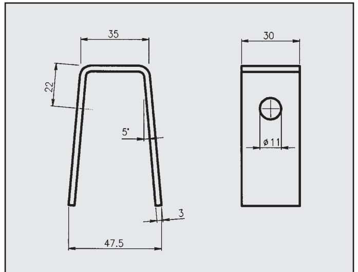
SUZUKI SJ 410 4X4 SJ 413 1.3 4X4 ATTACCO per posteriore COD. AT 720304
