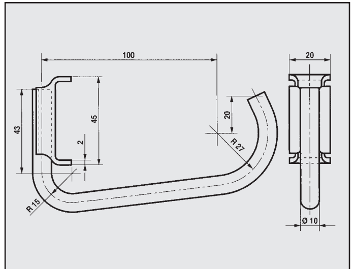
FORD ORION 1.4 ATTACCO posteriore COD. AT 260250
