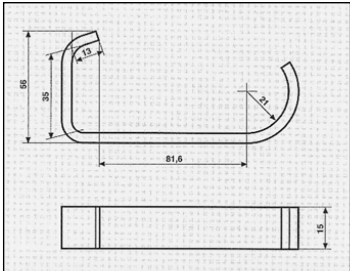
FIAT TIPO 1.4/1.6 CATALIZZATA ATTACCO posteriore COD. AT 241712 7657985
