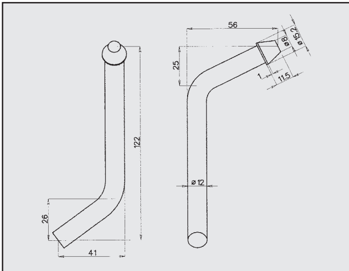
TICO ATTACCO POSTERIORE COD. AT 790001
