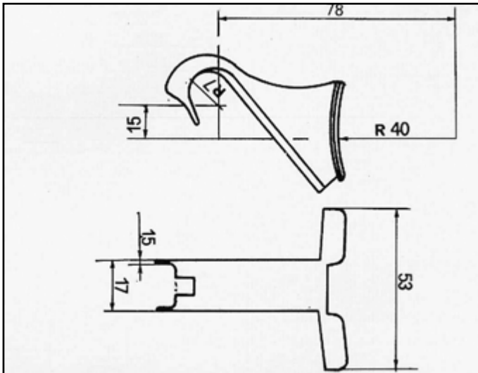
REGATA 85 ATTACCO per centrale COD. AT 241104
