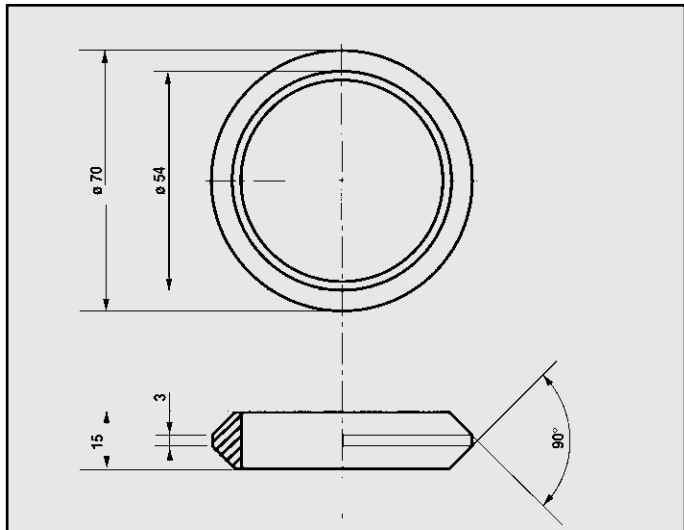
CITROEN BX GTI ANELLO \varnothing esterno mm 70 \varnothing interno mm 54 COD. AN 140305
