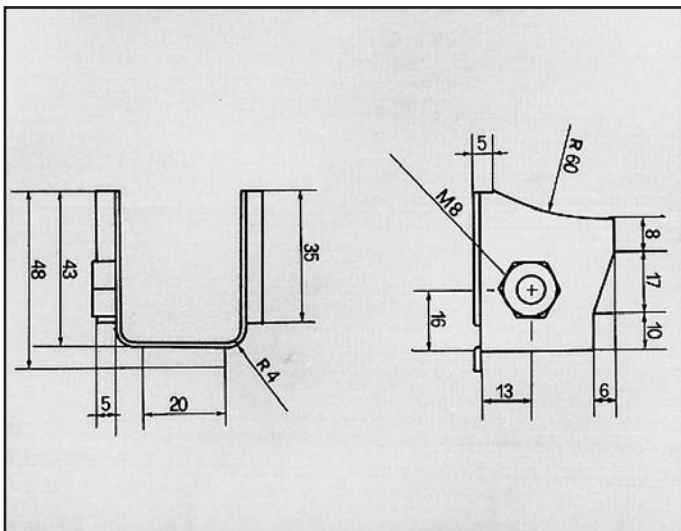
MINI 3 CILINDRI ATTACCO per posteriore COD. AT 320103
