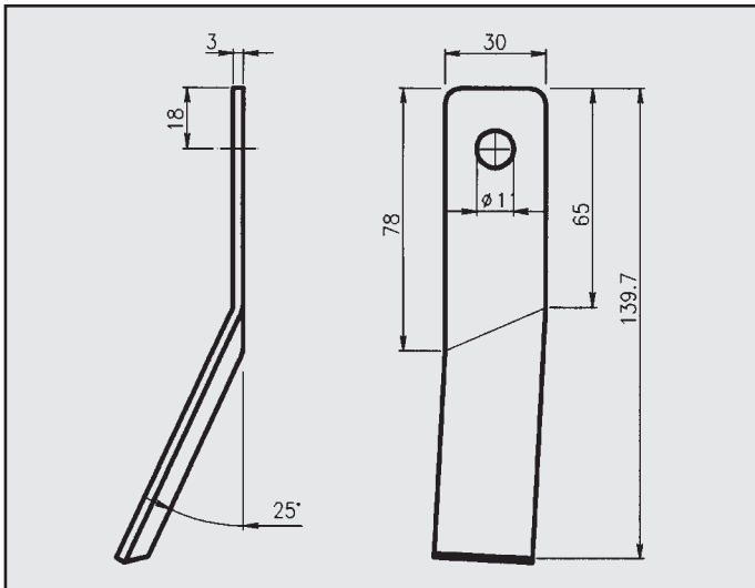
SUZUKI SJ 410 4X4 ATTACCO per posteriore COD. AT 720306
