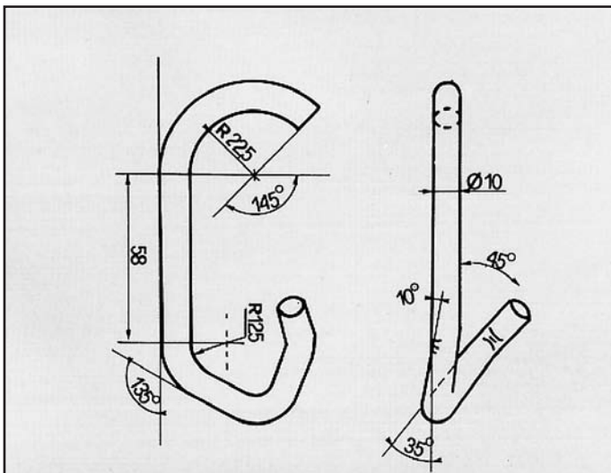
ACCORD 86 ATTACCO per posteriore COD. AT 280105
