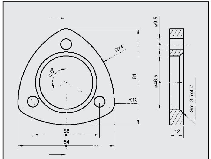
B M W FLANGIA COD. FL 120014
