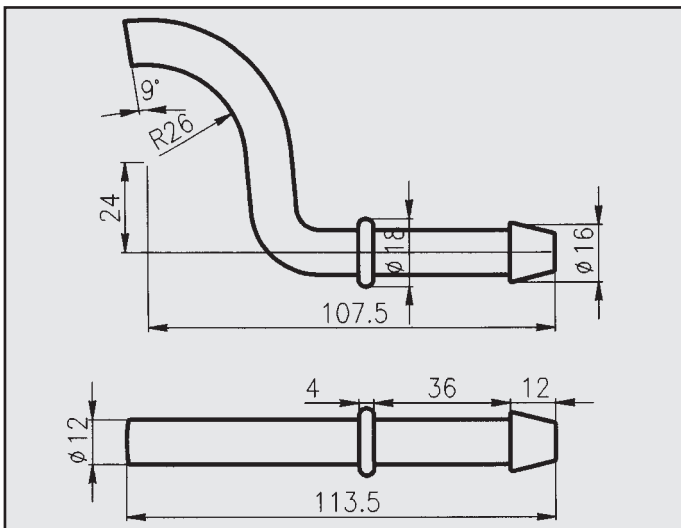
MERCEDES CLASSE A ATTACCO COD. AT 440701
