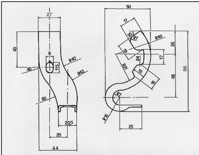
GOLF GTI 1600 ATTACCO per posteriore dx COD. AT 860109
