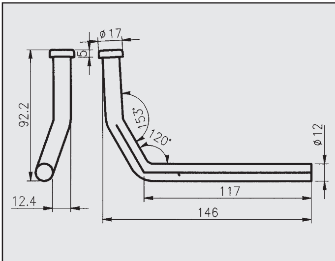
HYUNDAI LANTRA 1.5 GLI 1.6 16V 1.8 GT ATTACCO per posteriore COD. AT 300205
