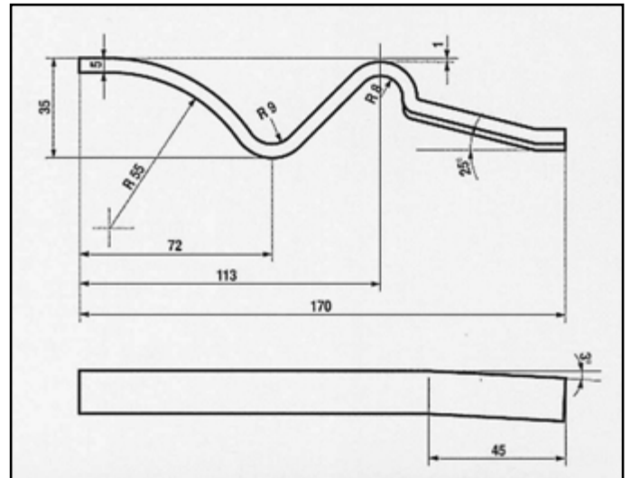
FIAT UNO 60/70 S-SX 1100/1300 09/89 ATTACCO per centrale COD. AT 240917
