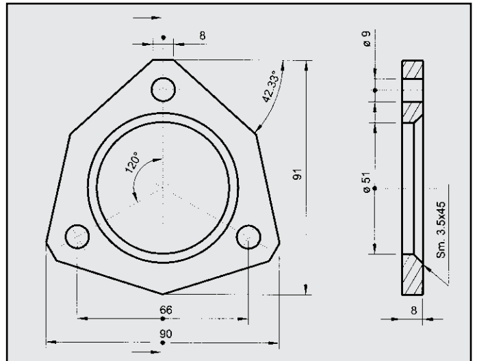
LANCIA FLANGIA COD. FL 380337
