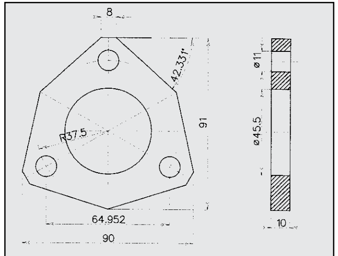
VOLKSWAGEN FLANGIA COD. FL 860029
