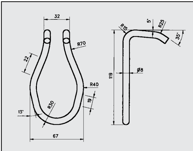
FIAT REGATA 85 ATTACCO per posteriore COD. AT 241105
