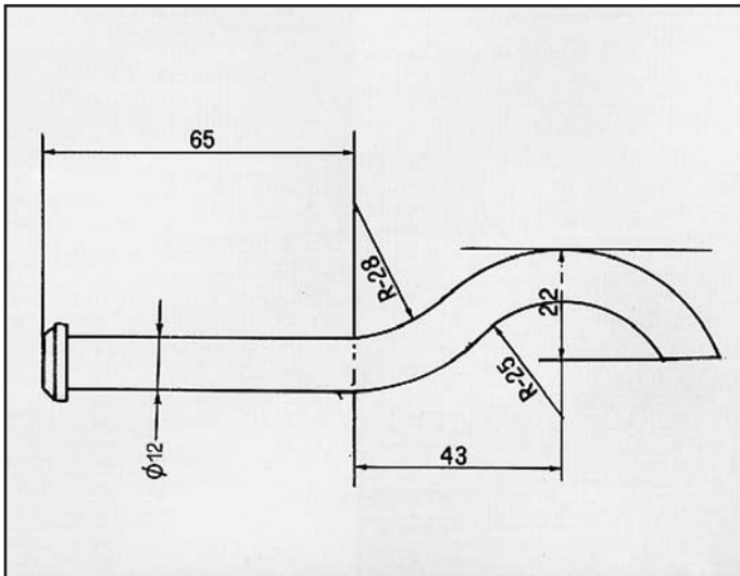
STARLET ATTACCO per centrale COD. AT 800802
