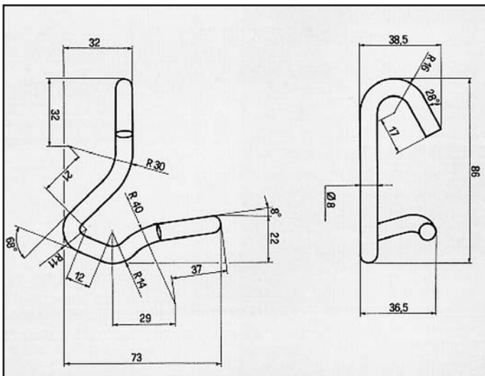
R14 ATTACCO per posteriore COD. AT 600402
