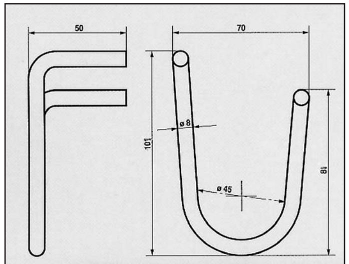
SEAT MALAGA 1400 - 1600 ATTACCO per posteriore COD. AT 680502
