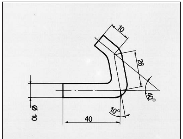
ACCORD 1800 ATTACCO per posteriore COD. AT 280108
