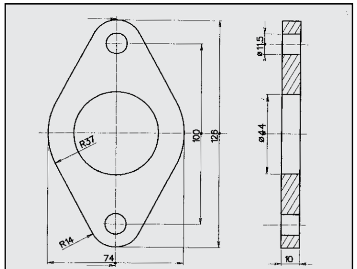
DAIHATSU FLANGIA COD. FL 180307
