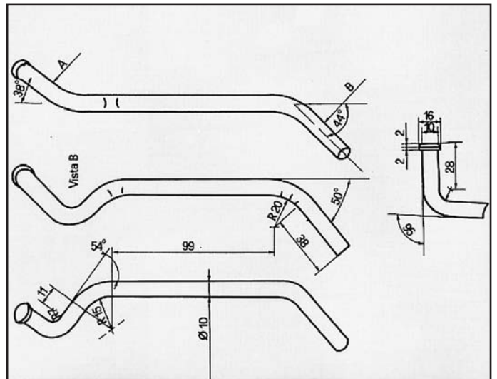
FAMILIA TURBO ATTACCO per anteriore COD. AT 420104
