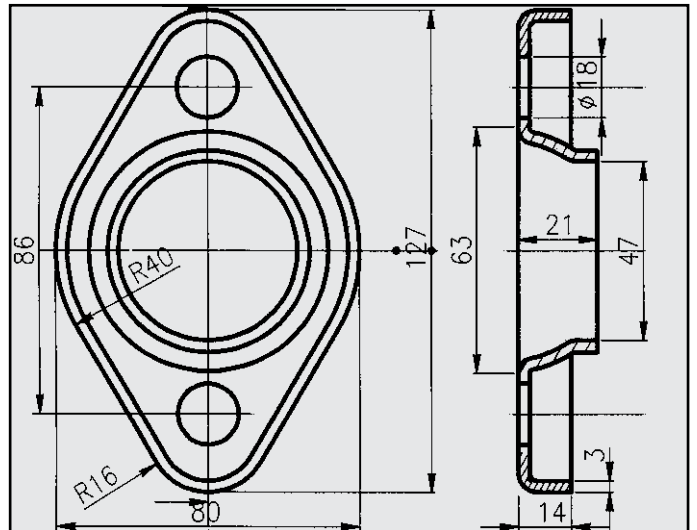
ROVER 214 SUZUKI VITARA FLANGIA COD. FL 620610
