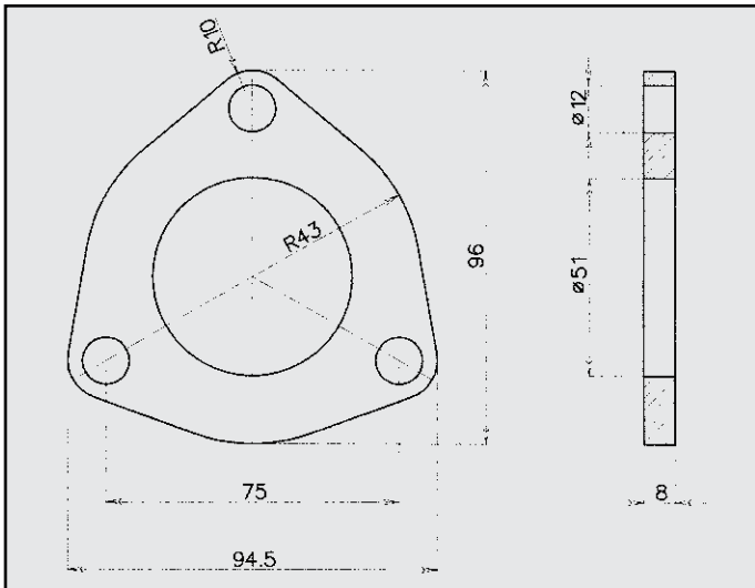
HONDA CIVIC 1.4 FLANGIA COD. FL 280429
