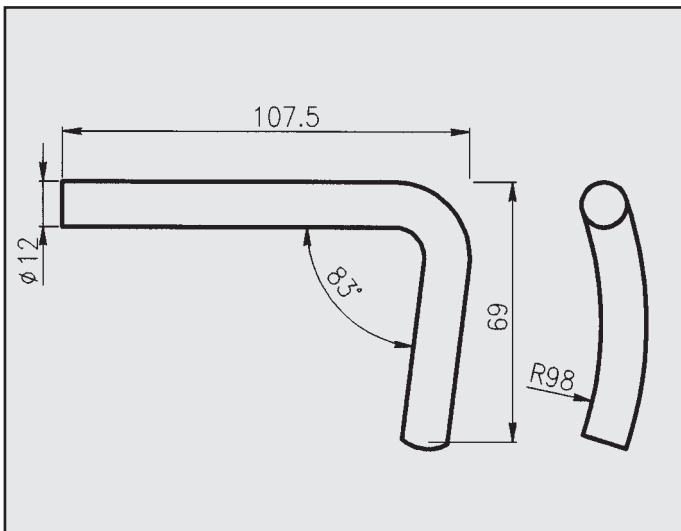
OPEL ASTRA 1.4 ATTACCO per posteriore COD. AT 520911
