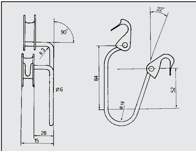
ALFA 75 TWIN SPARK ATTACCO per posteriore COD. AT 020307
