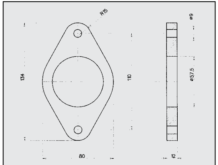
ALFA ROMEO FLANGIA COD. FL 020003
