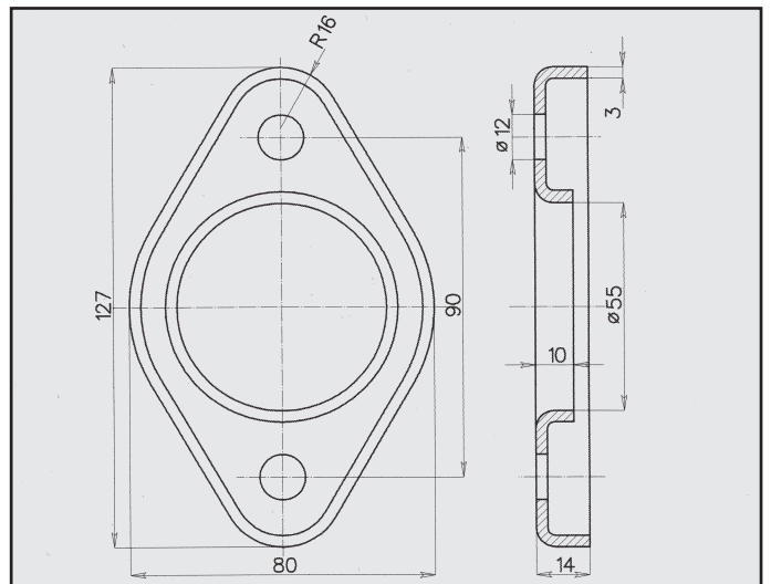
NISSAN PRIMIERA 2.0 FLANGIA CENTRALE COD. FL 500418
