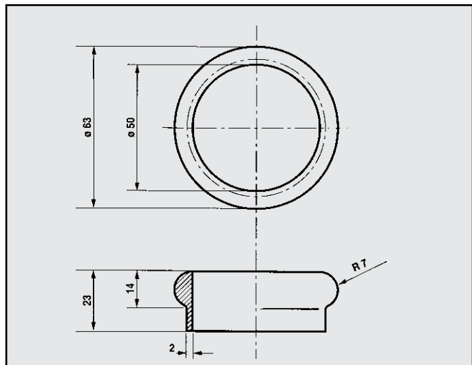
MITSUBISHI PAJERO ANELLO \varnothing esterno mm 63 \varnothing interno mm 50 COD. AN 460201
