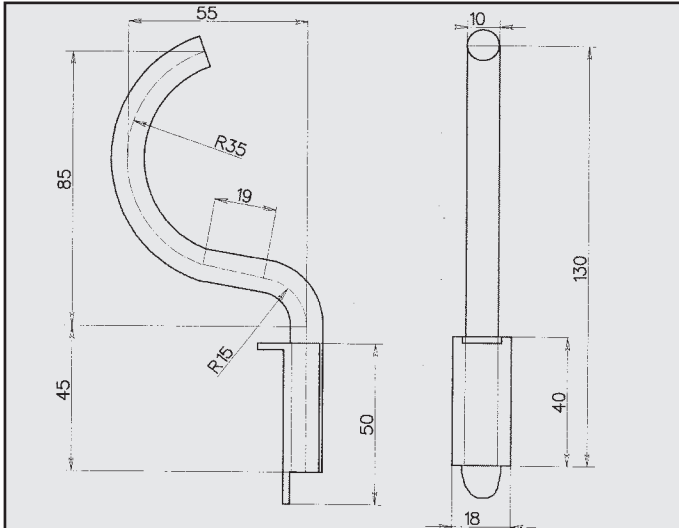
FORD ESCORT SW 1,6 16V '93 ATTACCO PER POSTERIORE COD. AT 260255
