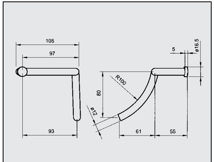
AUDI A4 1.6 ATTACCO per posteriore COD. AT 040603
