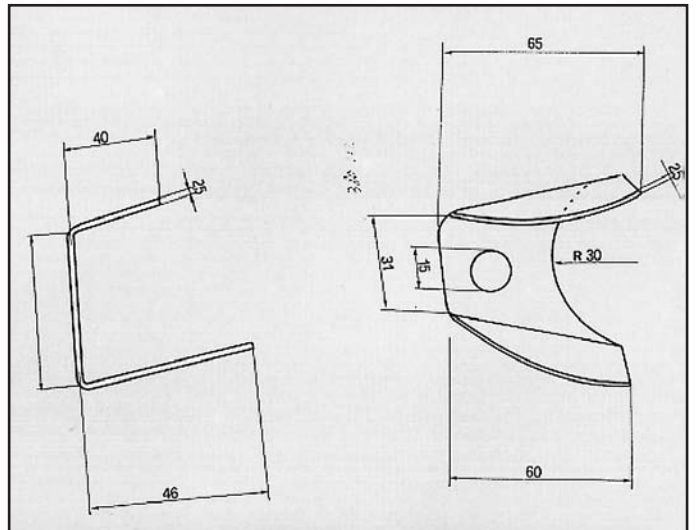
DELTA/PRISMA ATTACCO per collettore COD. AT 380312
