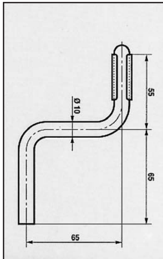
SKODA FAVORIT ATTACCO silenziatore centrale COD. AT 690102
