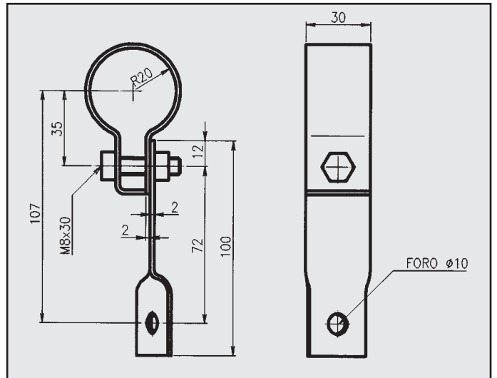
ROVER MINI 1.3 ATTACCO a fascetta per posteriore COD. AT 620502
