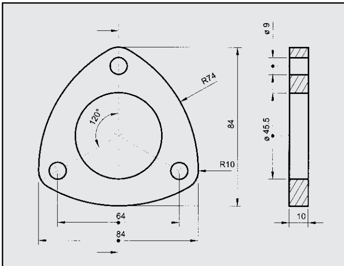
LANCIA DELTA 1.3 FLANGIA COD. FL 380335
