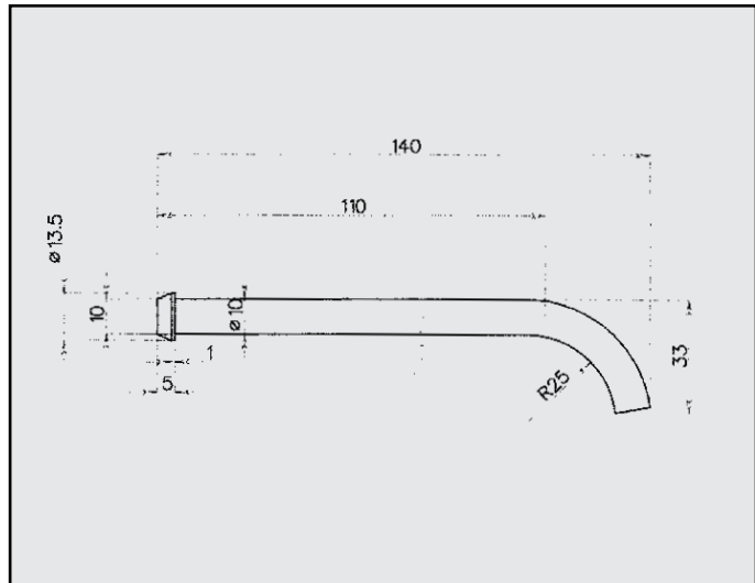
FIAT PUNTO ATTACCO COD. AT 242232
