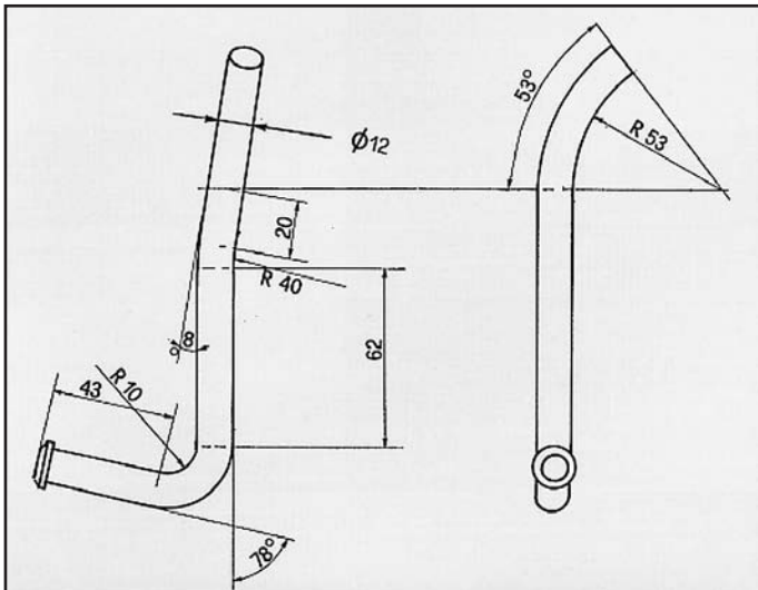
COROLLA FX ATTACCO per posteriore COD. AT 800406
