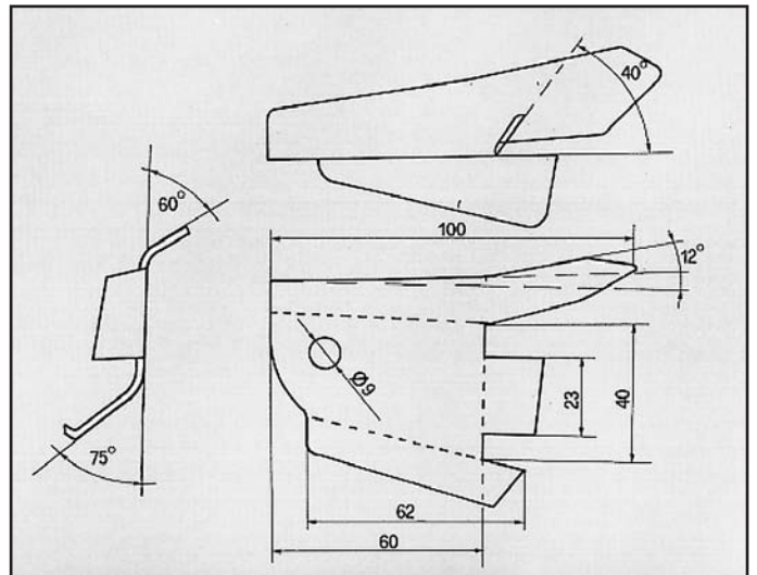
BETA/TREVI ATTACCO per centrale COD. AT 380106
