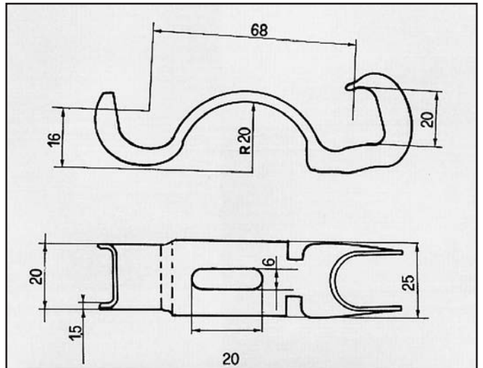
R14 ATTACCO per posteriore COD. AT 600403
