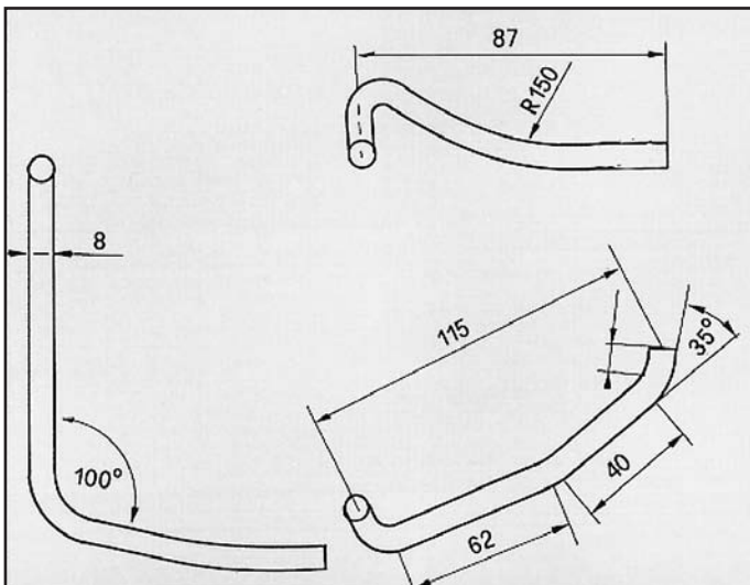
R5 EXPRESS BENZINA/DIESEL ATTACCO per posteriore COD. AT 600111
