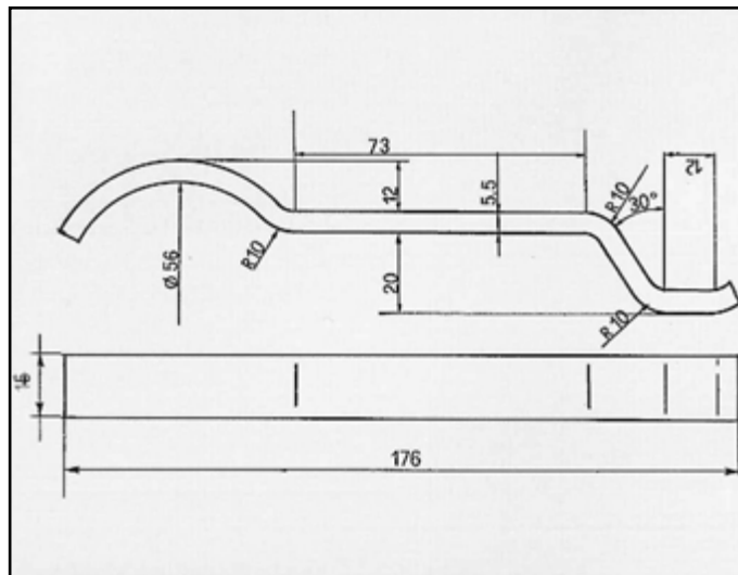
REGATA TURBO DIESEL ATTACCO per tubo collettore COD. AT 241113
