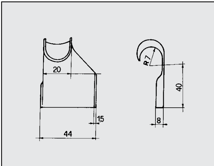
AUDI 50 ATTACCO per posteriore COD. AT 040201
