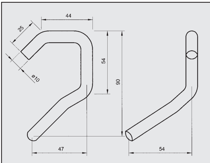
ROVER STERLING ATTACCO per posteriore COD. AT 620205
