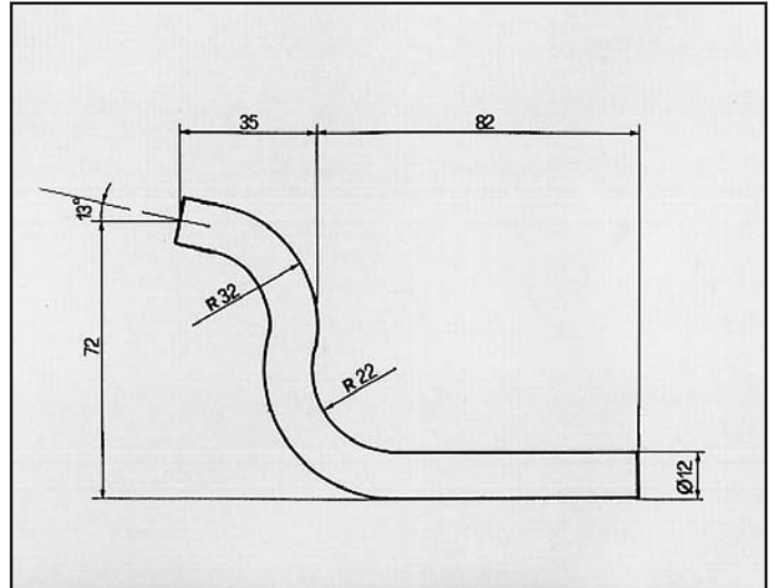
PRISMA 1300-1500 ATTACCO per posteriore COD. AT 380307
