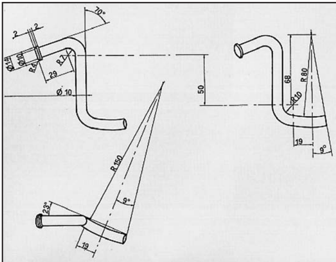
626 ATTACCO per posteriore COD. AT 420505
