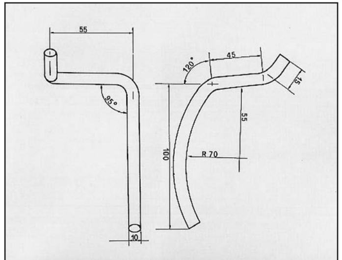
R19 ATTACCO per posteriore COD. AT 600901
