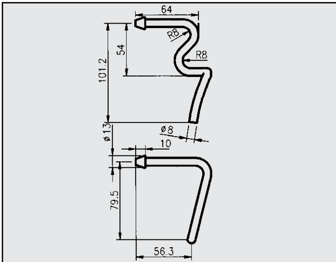
FIAT BRAVO/BRAVA 1.8 16V ATTACCO per posteriore COD. AT 242320
