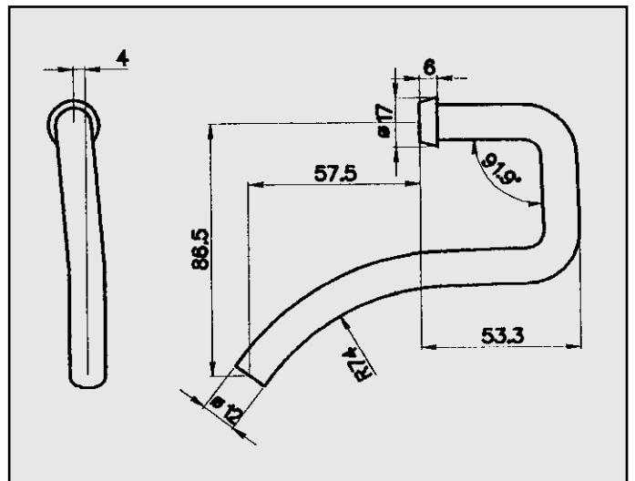
AUDI A3 TURBO-TD GOLF 1.8 '98 ATTACCO per posteriore COD. AT 040702
