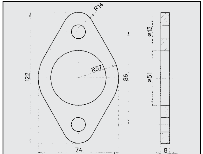
HYUNDAI LANDRA FLANGIA COD. FL 300208
