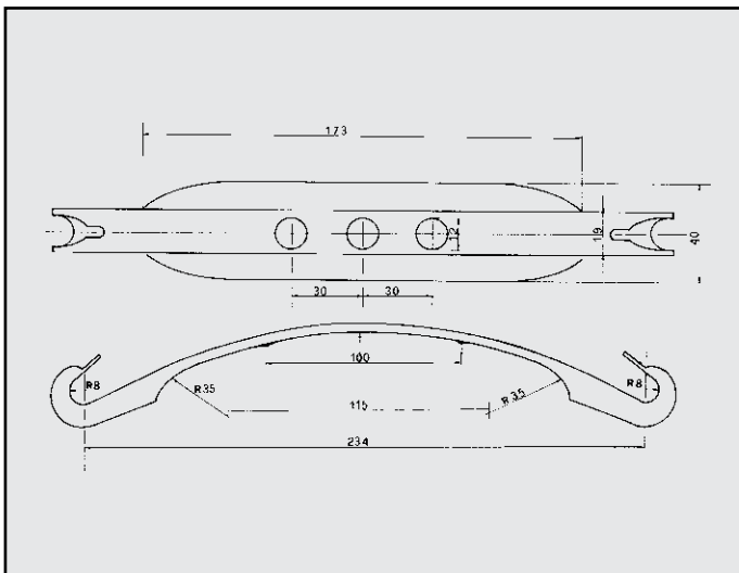
AUDI 80 1600-1800 ATTACCO per posteriore COD. AT 040303 855253609A 811253609F
