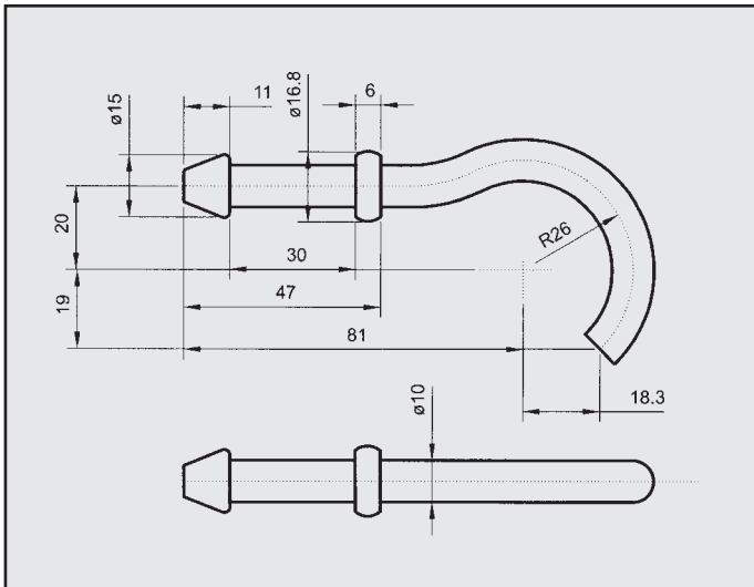
FORD FIESTA 1,2i CAT '95 ATTACCO centrale COD. AT 260336
