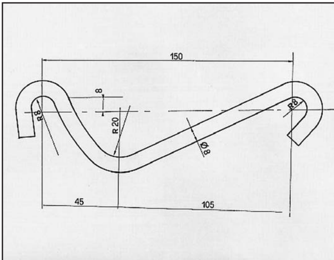
FUEGO ATTACCO per posteriore COD. AT 600702
