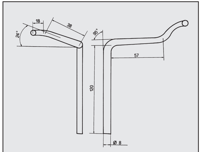
AX SPORT dal '87 ATTACCO COD. AT 140704
