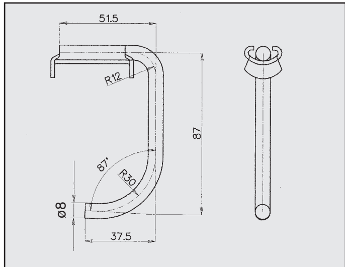
OPEL CORSA ATTACCO COD. AT 520322
