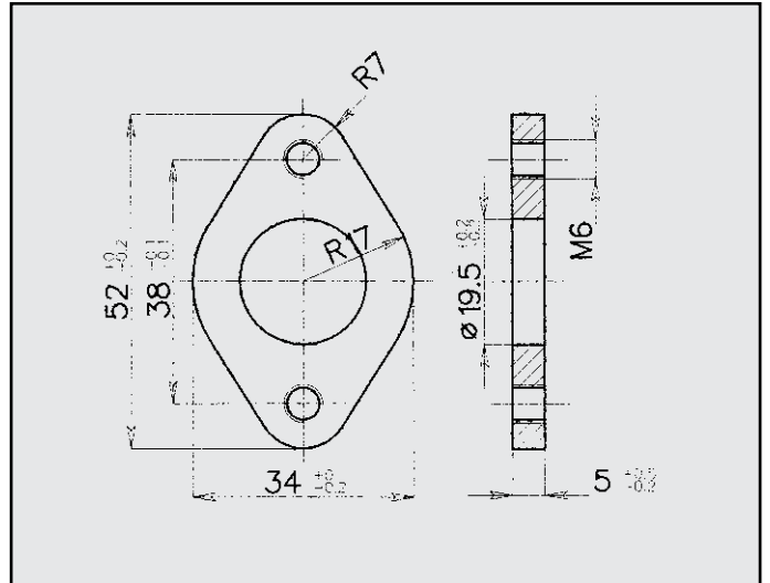
VOLKSWAGEN FLANGIA COD. FL 860023
