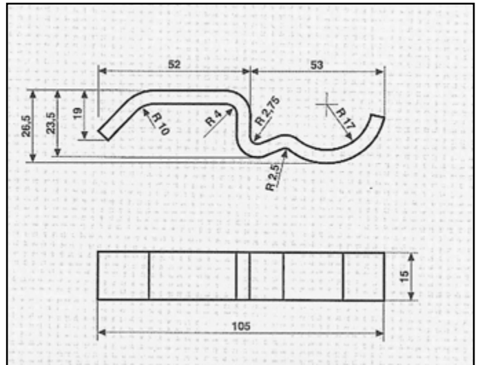
FIAT CINQUECENTO NUOVA ATTACCO centrale COD. AT 242101
