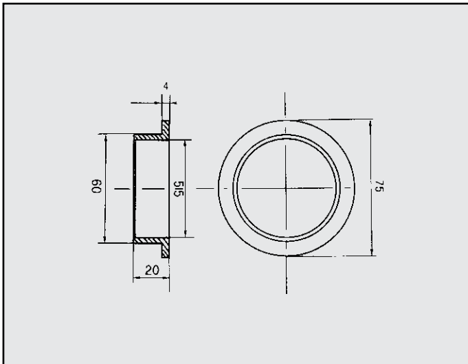
LAMBORGHINI COUNTACH 4 ANELLO per tubo centrale COD. AN 360101
