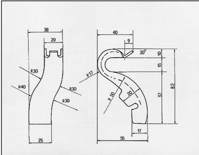
GOLF GTI 1600 ATTACCO per centrale sx COD. AT 860108
