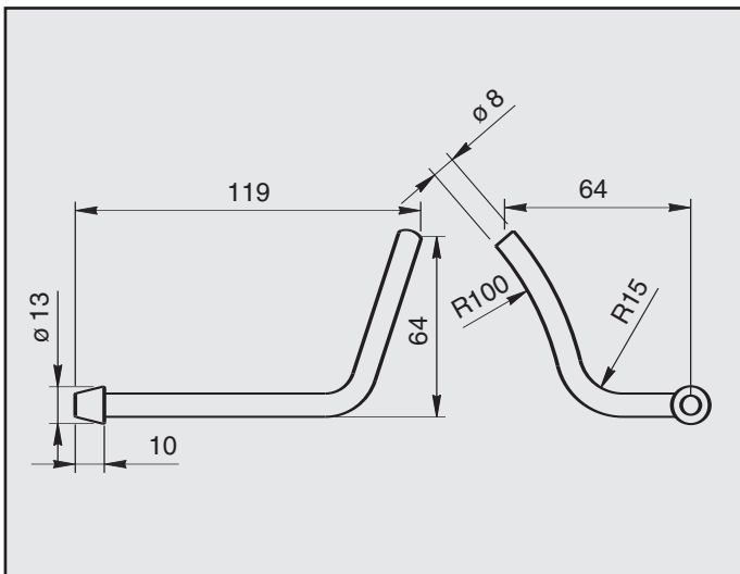
ALFA 146 / 145 ATTACCO posteriore COD. AT 021102
