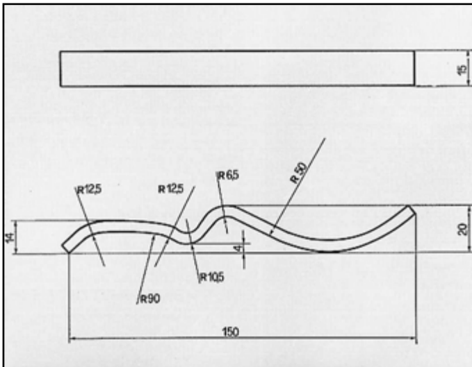
UNO TURBO IE ATTACCO per posteriore COD. AT 240907
