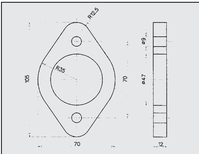
BMW 320 FLANGIA COD. FL 120407
