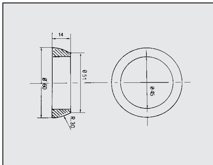
FIAT UNO DIESEL ANELLO ø esterno mm 60 ø interno mm 45 COD. AN 240901
