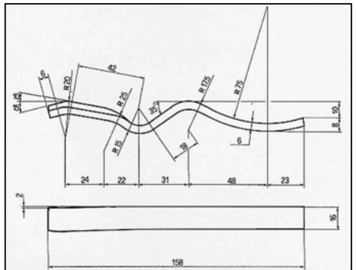
UNO TURBO DIESEL ATTACCO per posteriore COD. AT 240911
