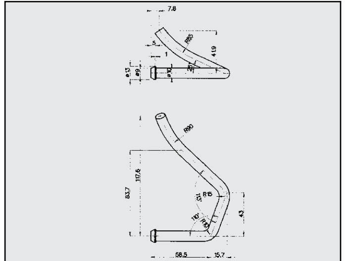
FIAT PUNTO TD ATTACCO POSTERIORE COD. AT 242240
