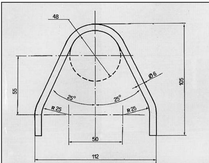
MARBELLA E TERRA RINFORZO anteriore per posteriore COD. R 680303
