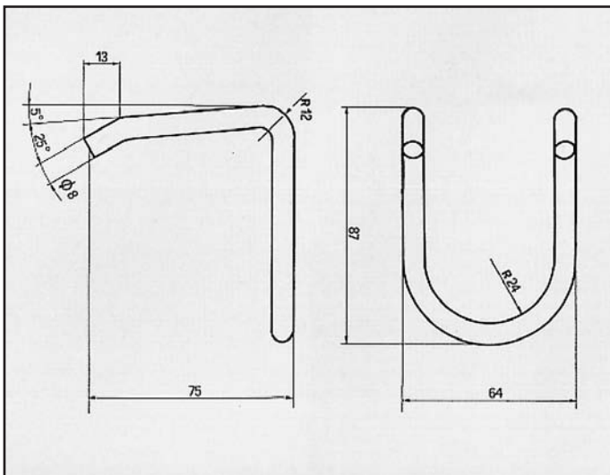
R9-R11 ATTACCO per posteriore COD. AT 600205
