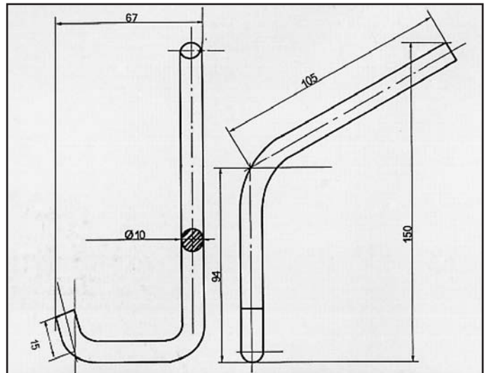
BALLADE SPORT ATTACCO per posteriore COD. AT 280304
