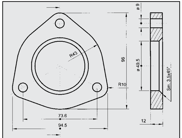
FIAT CROMA FLANGIA COD. FL 240003
