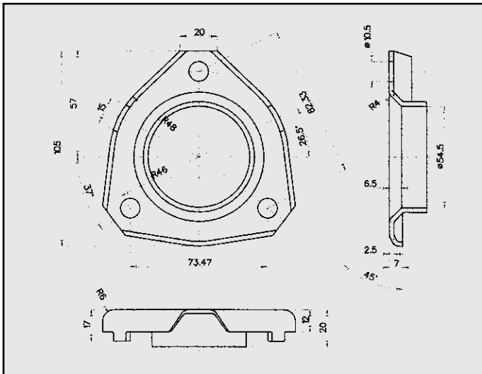
PEUGEOT 206 FLANGIA COD. FL 541208
