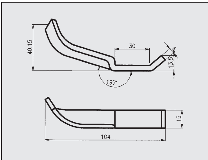
SEAT INCA ATTACCO per posteriore COD. AT 680701
