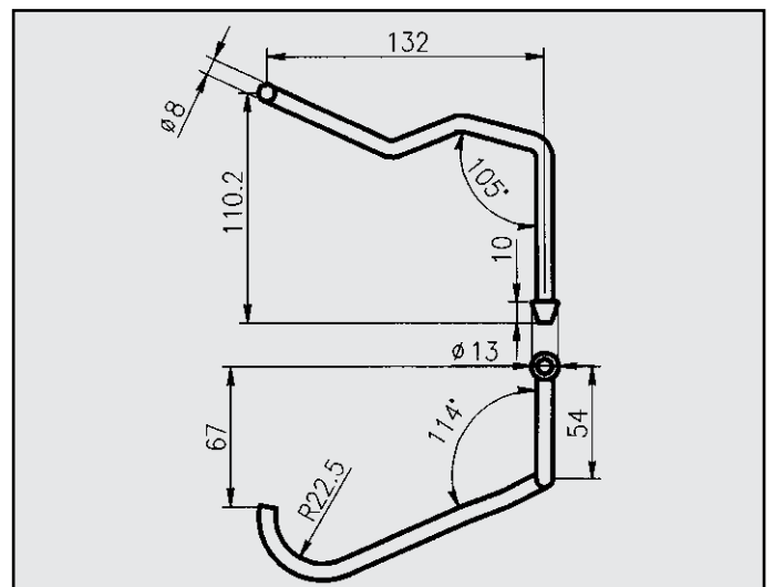
FIAT BRAVO/BRAVA 1.8 16V ATTACCO per posteriore COD. AT 242312
