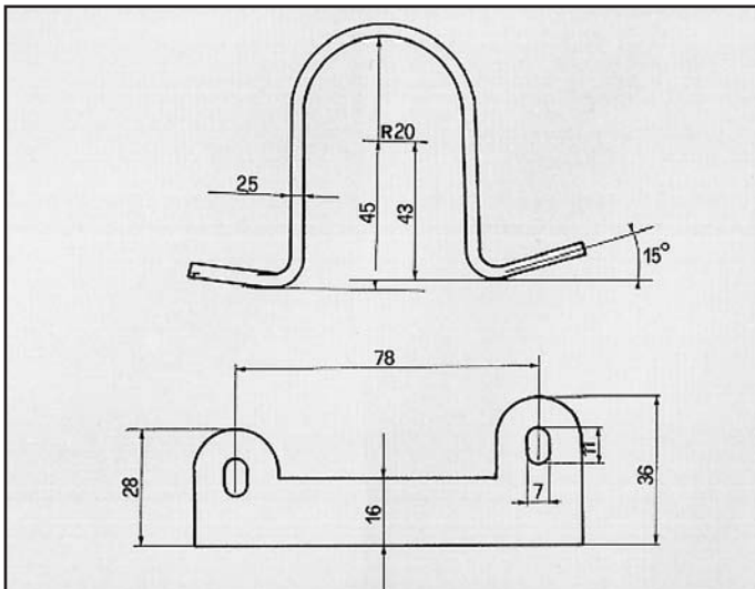
R5 ATTACCO per posteriore COD. AT 600103
