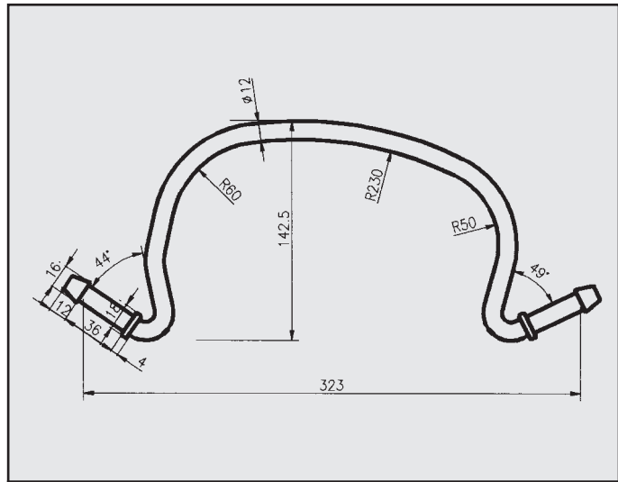
MERCEDES CLASSE A ATTACCO posteriore COD. AT 440702
