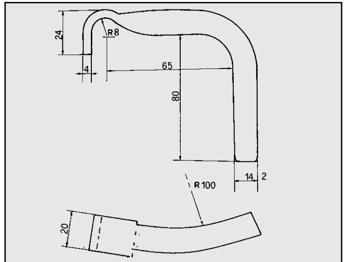
Y10 1300 GTIE ATTACCO anteriore per posteriore COD. AT 080211 7649426
