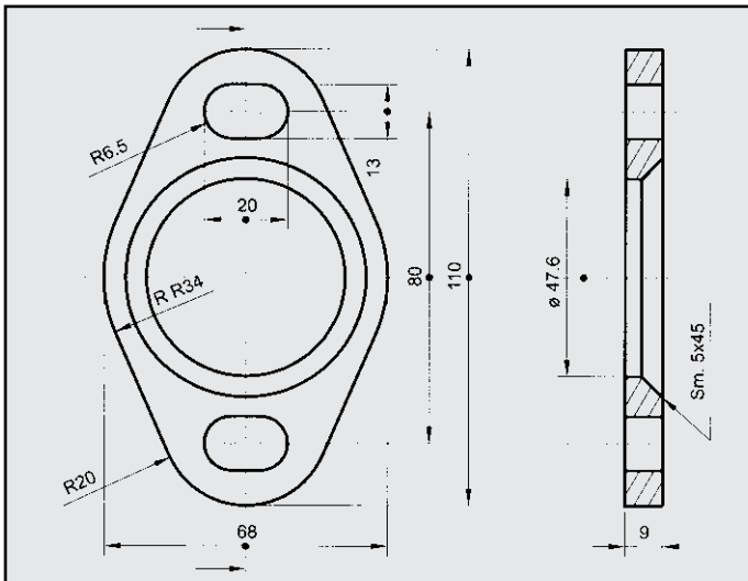
FIAT TIPO 1.1 - 1.4 FLANGIA COD. FL 241718
