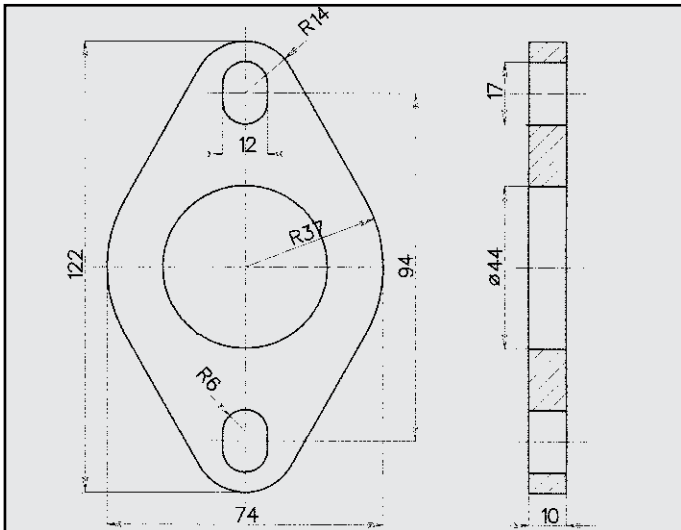
DAIHATSU FERENZA 1.6 FLANGIA COD. FL 180308
