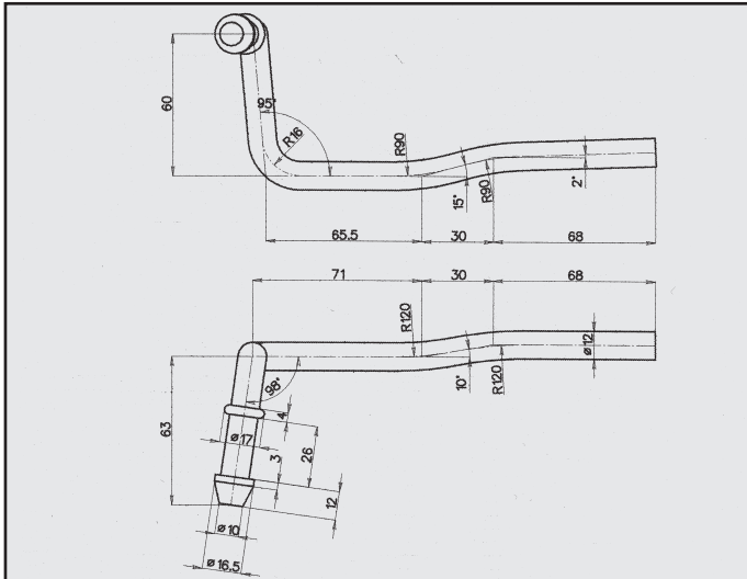
ALFA 156 ATTACCO centrale COD. AT 021207
