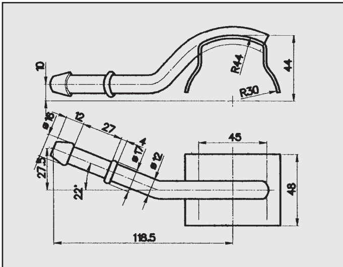
LANCIA K 2.0 ATTACCO per centrale COD. AT 380903
