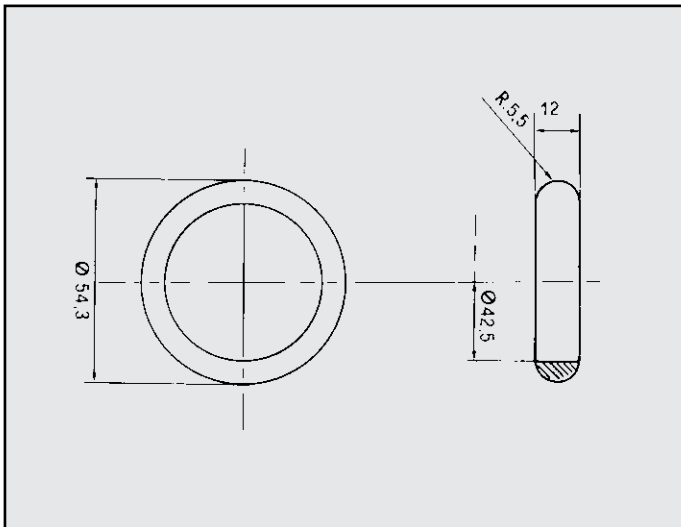
FORD FIESTA ANELLO per manicotto COD. AN 260301
