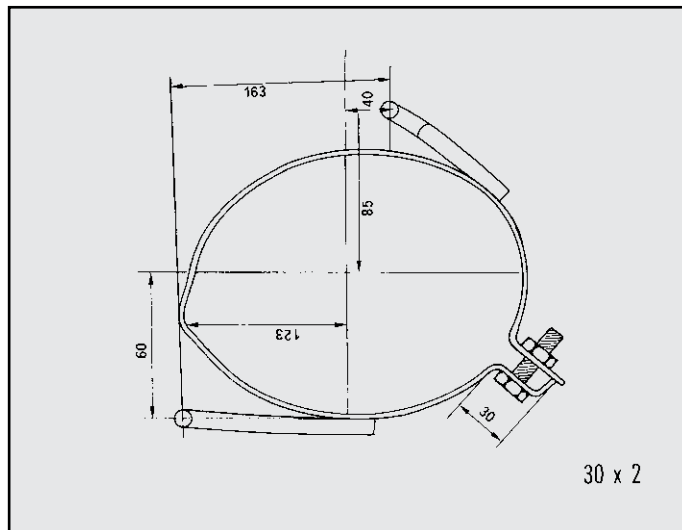
PEUGEOT 205 GTI 1600/1900 SPECIALE FASCETTA per barilotto COD. F 540305
