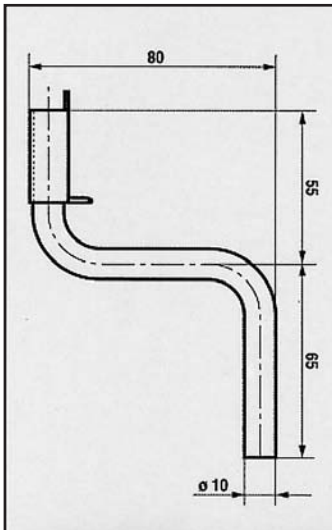
SKODA FAVORIT ATTACCO silenziatore centrale COD. AT 690101
