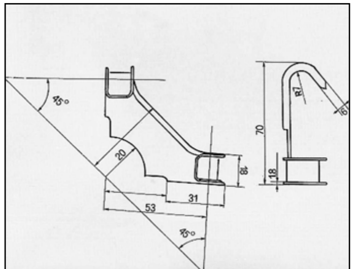
RITMO 1ª SERIE ATTACCO per posteriore COD. AT 240803
