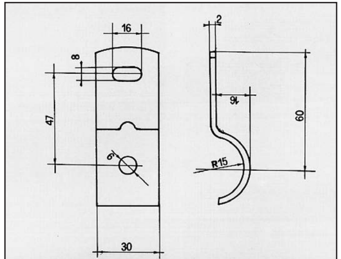
R4 R6 ATTACCO per tubo posteriore COD. AT 600802
