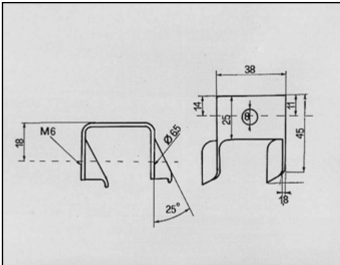
127-900 ATTACCO per posteriore COD. AT 240204
