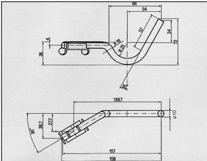
ESCORT 1600 DIESEL ATTACCO per posteriore COD. AT 260230
