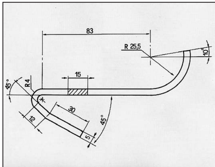
740 TURBO ATTACCO per posteriore COD. AT 880202
