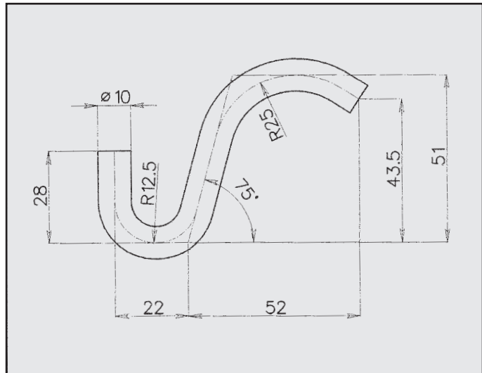
OPEL CORSA /COMBO ATTACCO CENTRALE COD. AT 520321
