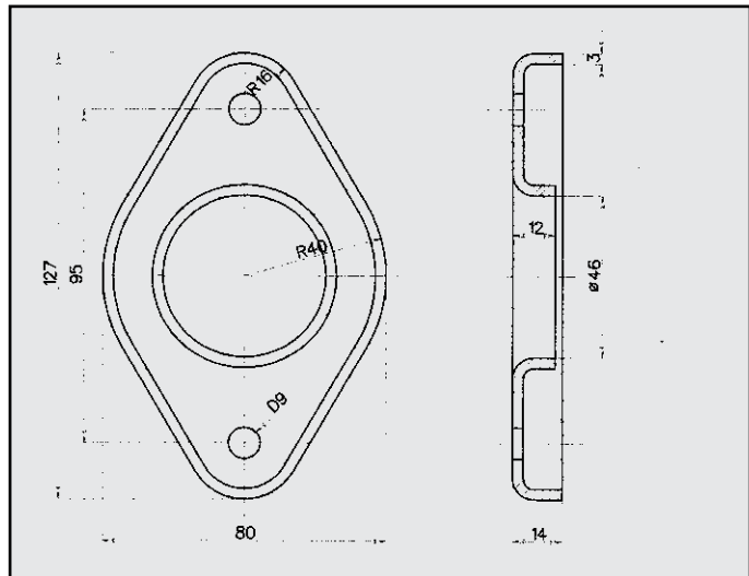
PEUGEOT 307 1.6-1.4 FLANGIA COD. FL 541301
