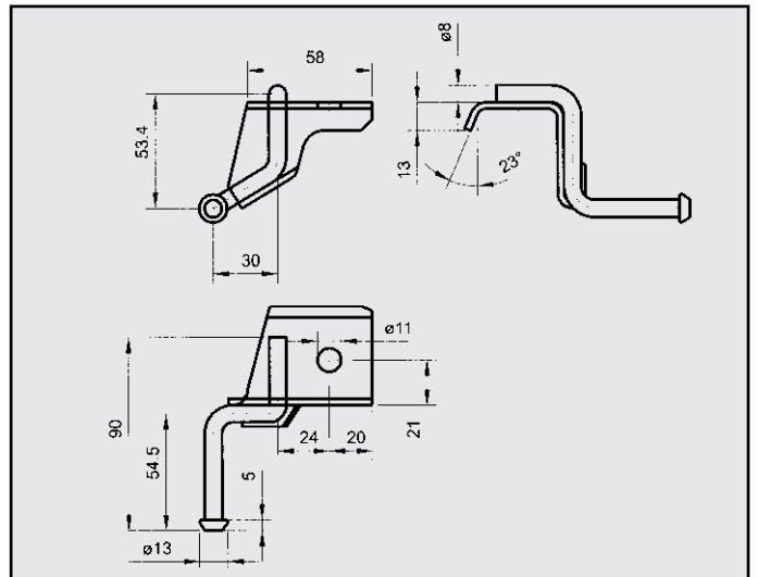
FIAT MULTIPLA NUOVO DAILY ATTACCO COD. AT 242601
