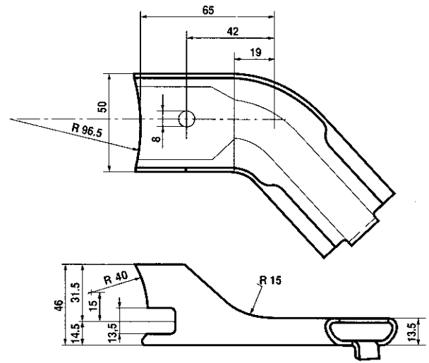
BMW 520 ATTACCO per centrale COD. AT 120207
