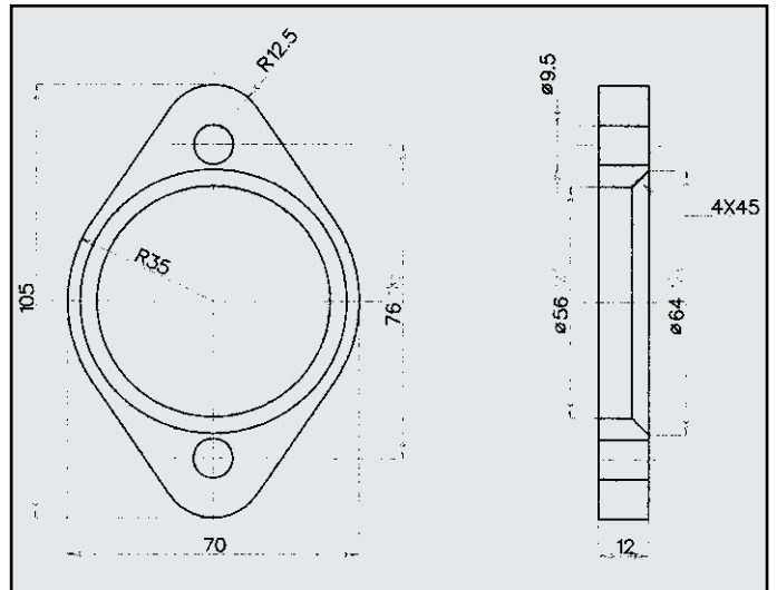
MERCEDES 190 D FLANGIA COD. FL 440303
