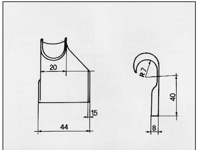
POLO 1ª SERIE ATTACCO per posteriore COD. AT 860301
