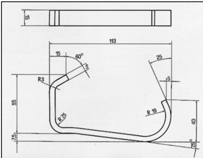
TIPO BENZINA E DIESEL ATTACCO per posteriore COD. AT 241702
