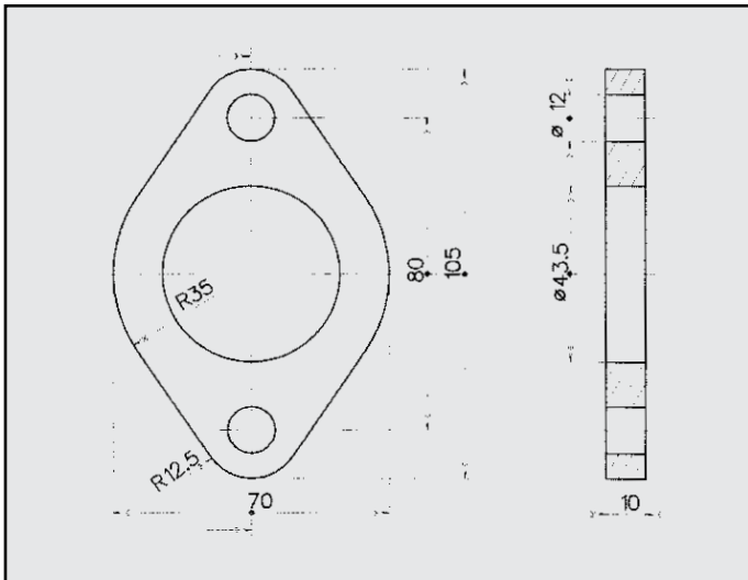
OPEL CORSA DIESEL FLANGIA COD. FL 520320
