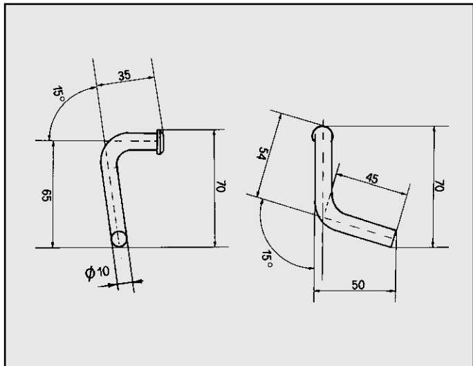
MIRA TURBO ATTACCO per posteriore COD. AT 180102
