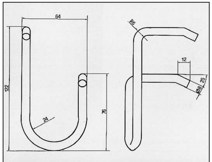
R9 ATTACCO per centrale COD. AT 600201
