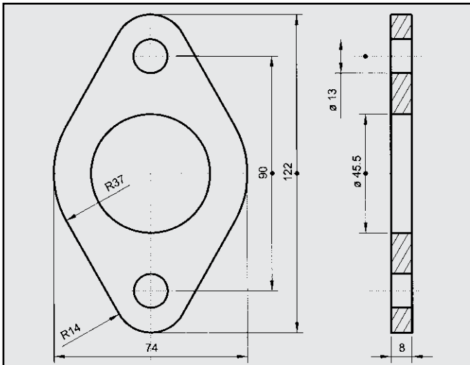
FORD FIESTA FLANGIA COD. FL 260339
