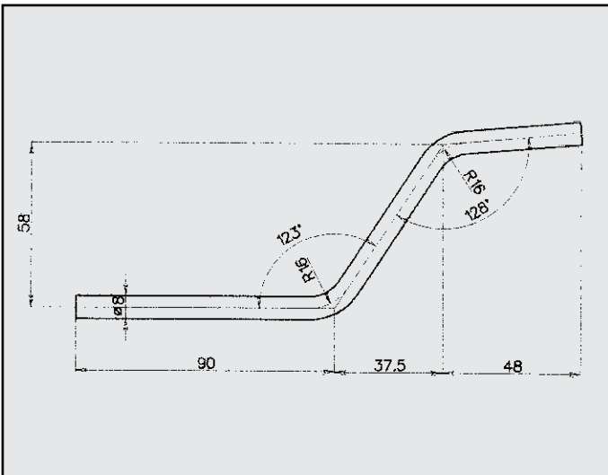
FIAT PUNTO 55 ATTACCO COD. AT 242238
