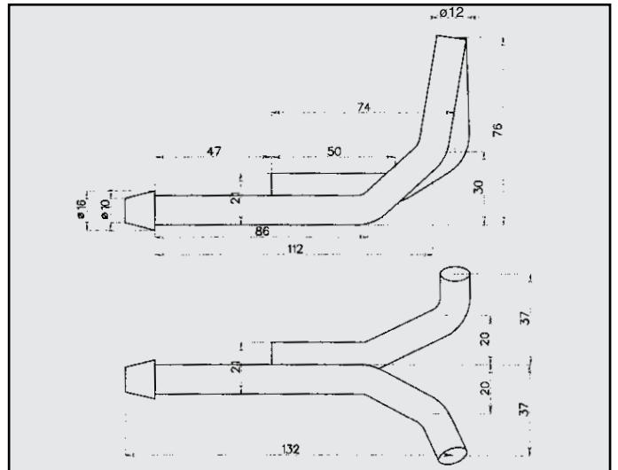
AUDI A4 CENTRALE 1.6/1.8 ATTACCO COD. AT 040608
