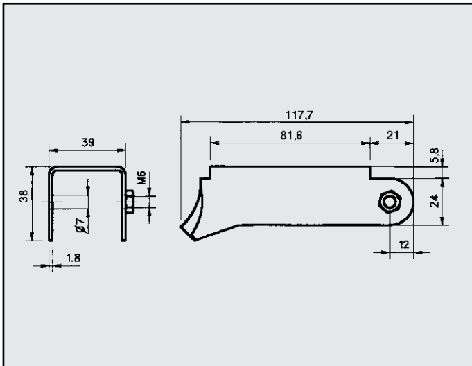
AUTOBIANCHI Y10 4x4 ATTACCO COD. AT 080208 7670005
