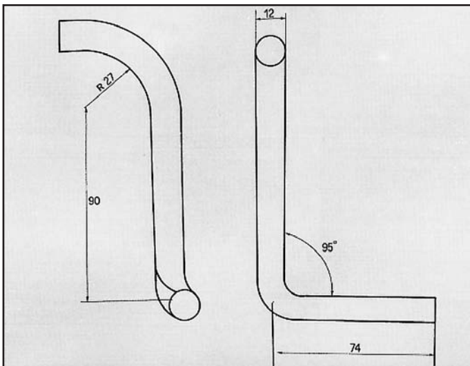
PRISMA 4WD ATTACCO per posteriore COD. AT 380326
