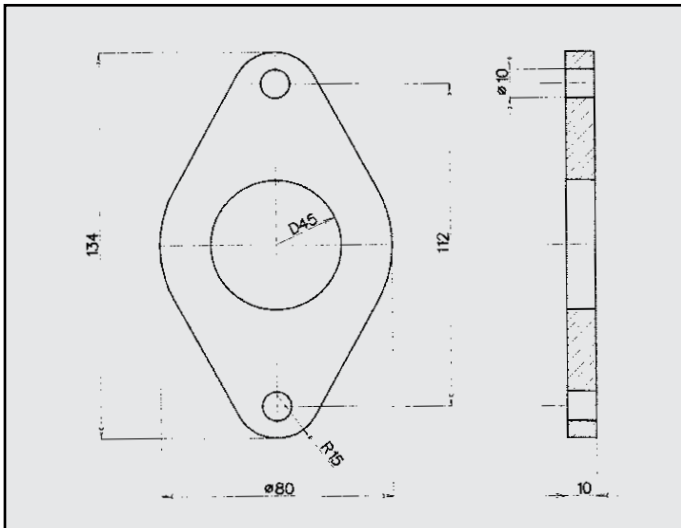
FIAT PALIO FLANGIA COD. FL 243008
