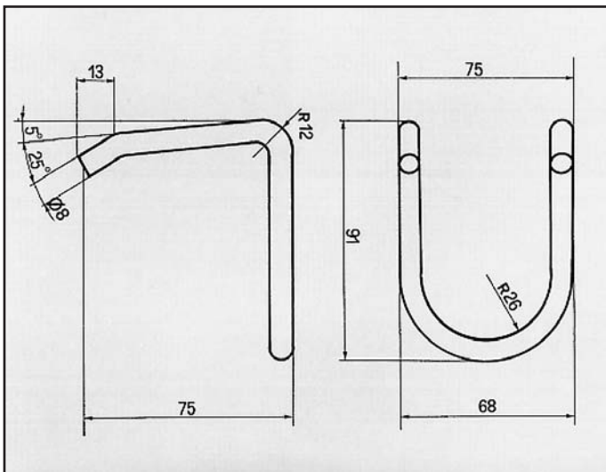
R 21 DIESEL ATTACCO per posteriore COD. AT 601002
