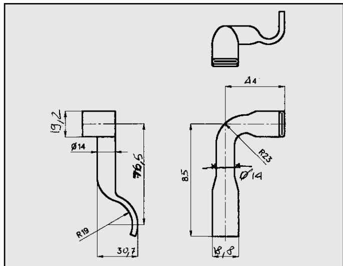
PANDA FIRE ATTACCO per posteriore COD. AT 240108
