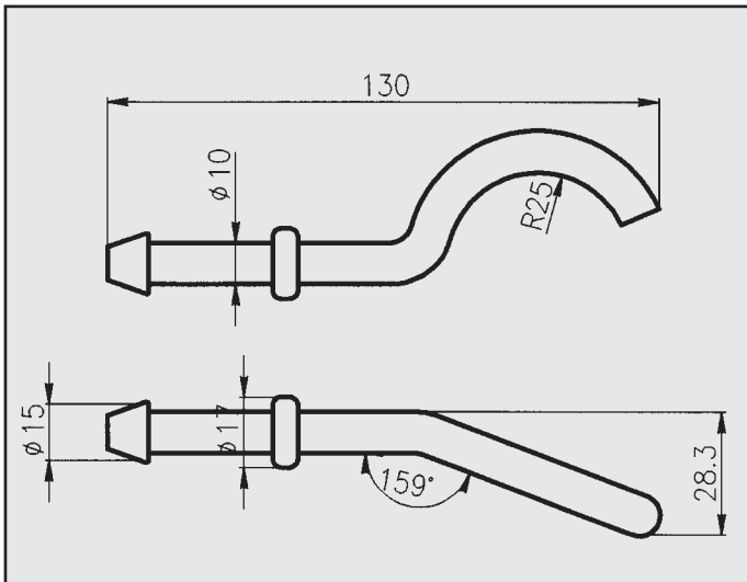
FORD ESCORT ATTACCO per posteriore COD. AT 260273
