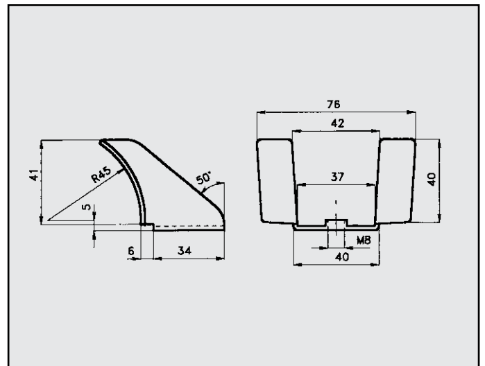
FIAT 132 ATTACCO per posteriore COD. AT 240702
