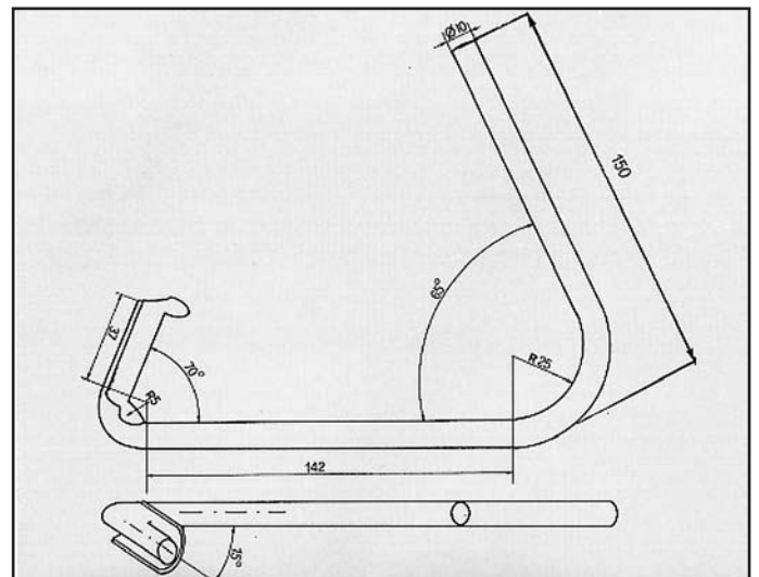
SCORPIO 2000 RATTACCO per posteriore COD. AT 260802
