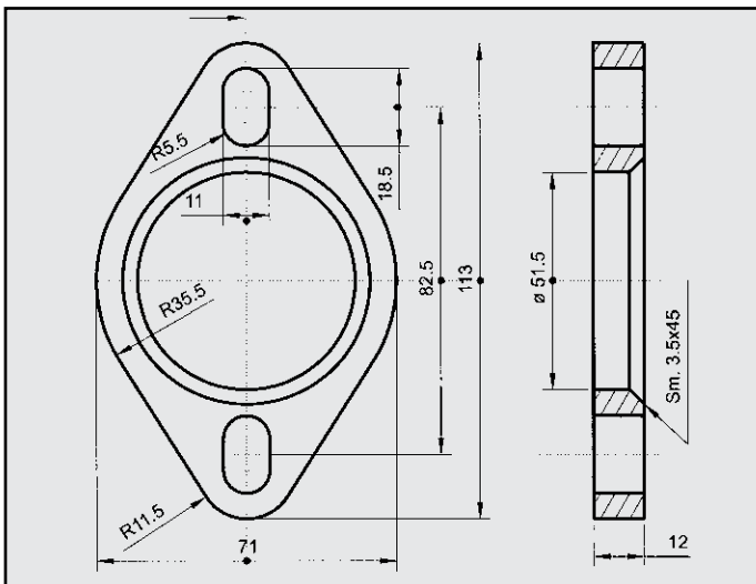
FORD FIESTA FLANGIA COD. FL 260343
