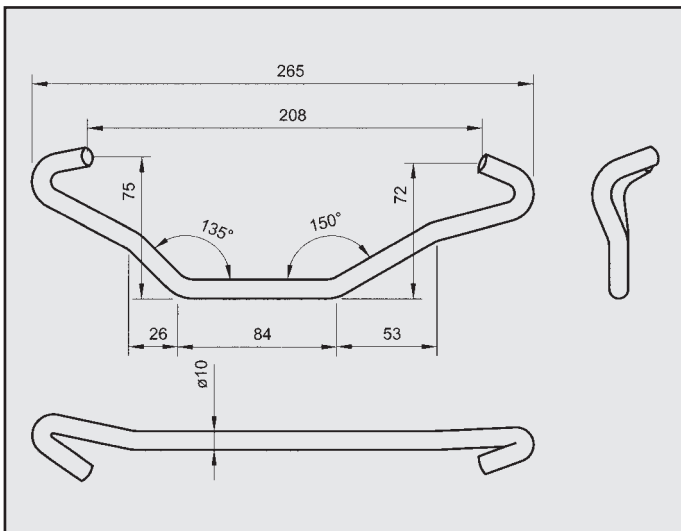
MITSUBISHI PAJERO ATTACCO per posteriore COD. AT 460203
