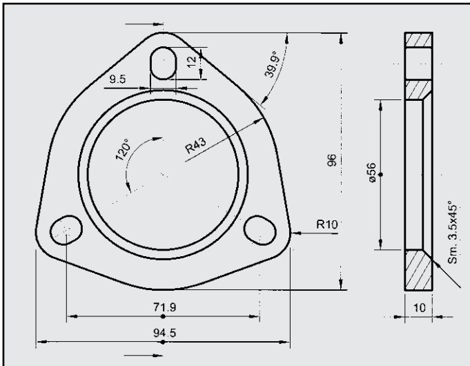
ALFA 155 TS FLANGIA COD. FL 021006
