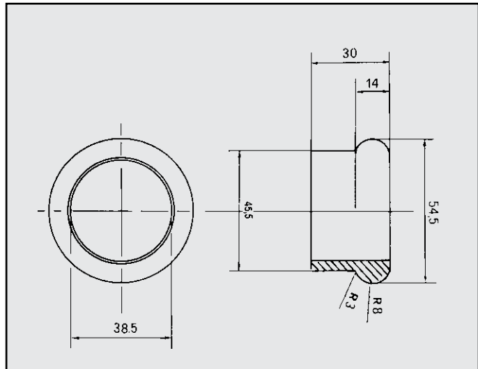
MITSUBISHI COLT ANELLO per manicotto posteriore COD. AN 460101
