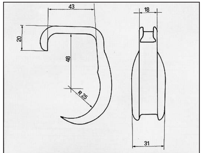
MANTA ATTACCO per posteriore COD. AT 520208
