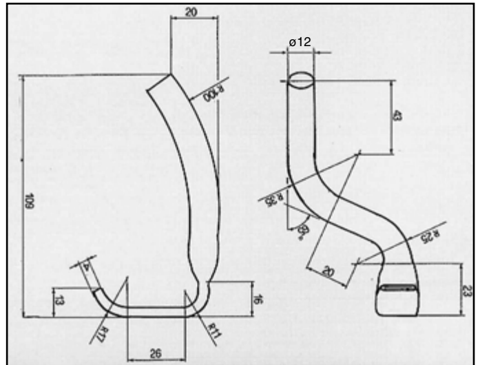
UNO DIESEL ATTACCO per posteriore COD. AT 240909
