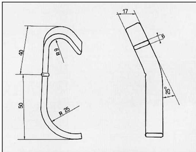
OPEL MONZA ATTACCO per posteriore COD. AT 520701
