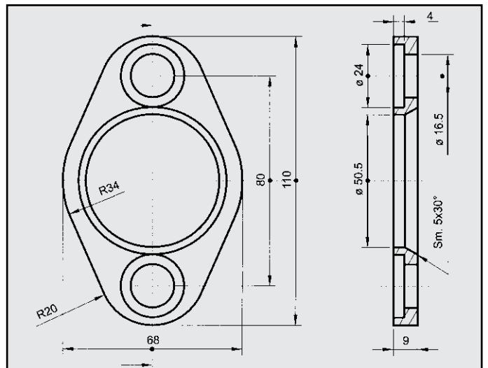
AUTOBIANCHI Y10 1.1 - 1.3 FLANGIA COD. FL 080218
