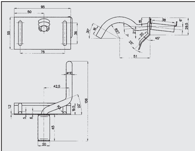
PEUGEOT 406 ATTACCO per tubo COD. AT 541104
