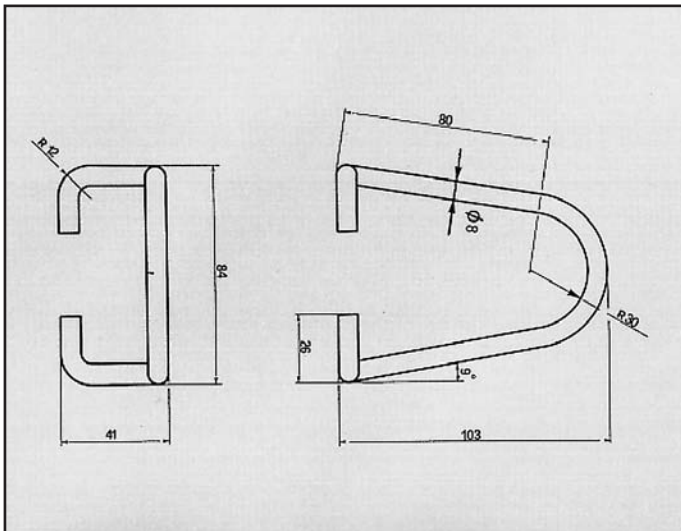
ESCORT 1100-1300 ATTACCO per centrale COD. AT 260210
