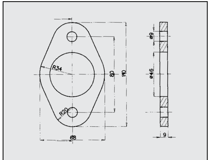
FIAT TIPO 1.4 FLANGIA COD. FL 241725
