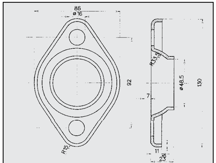
ROVER FLANGIA COD. FL 620707
