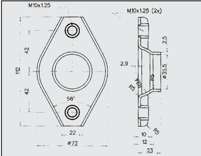
TOYOTA FLANGIA COD. FL 800006
