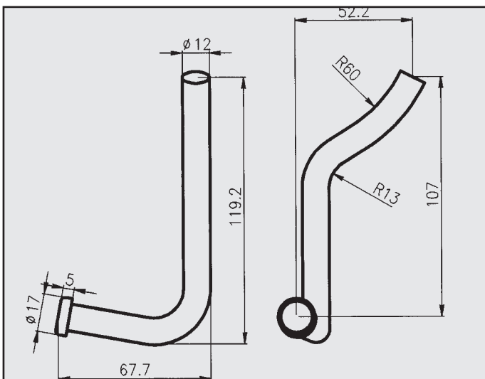
TOYOTA COROLLA FX ATTACCO per posteriore COD. AT 800418
