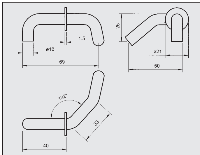
ROVER 620 Ti TURBO ATTACCO DX per posteriore COD. AT 621002
