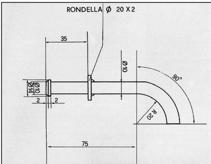
FAMILIA TURBO ATTACCO per posteriore COD. AT 420107
