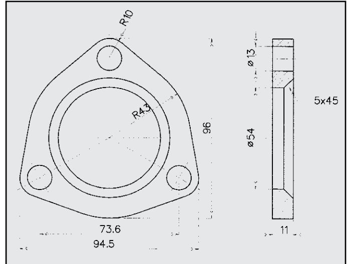
FIAT CROMA FLANGIA COD. FL 242902
