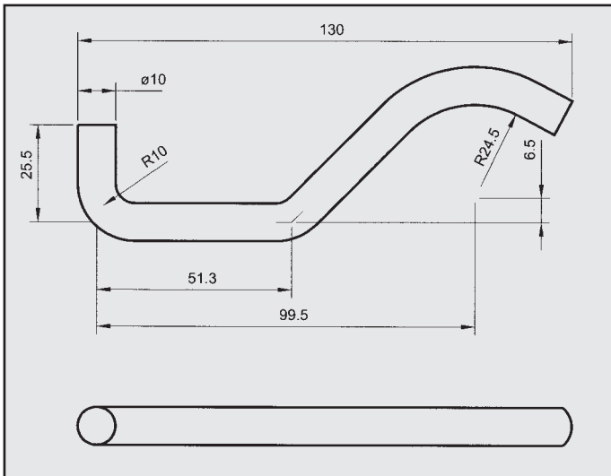
HONDA CRX 1,3 - 1,5 ATTACCO COD. AT 280509
