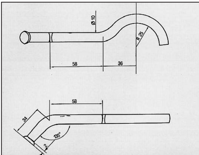
626 2000 16V ATTACCO tubo posteriore COD. AT 420519
