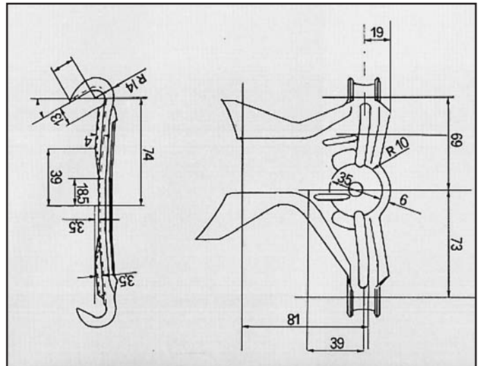
230 E / 85 ATTACCO COD. AT 440206
