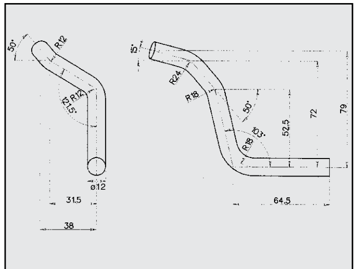
ALFA GTV ATTACCO CENTRALE COD. AT 020613
