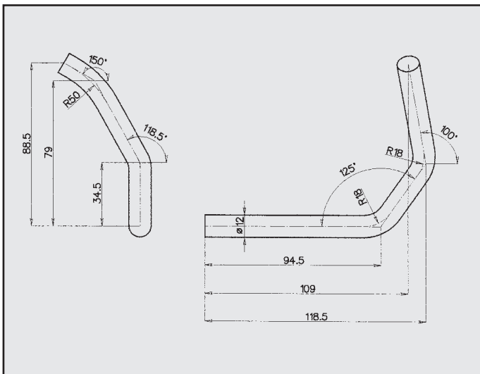
OPEL ASTRA ATTACCO per posteriore COD. AT 520932
