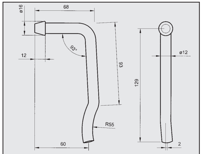
NISSAN PRIMERA 2.0 ATTACCO SX per posteriore COD. AT 500412
