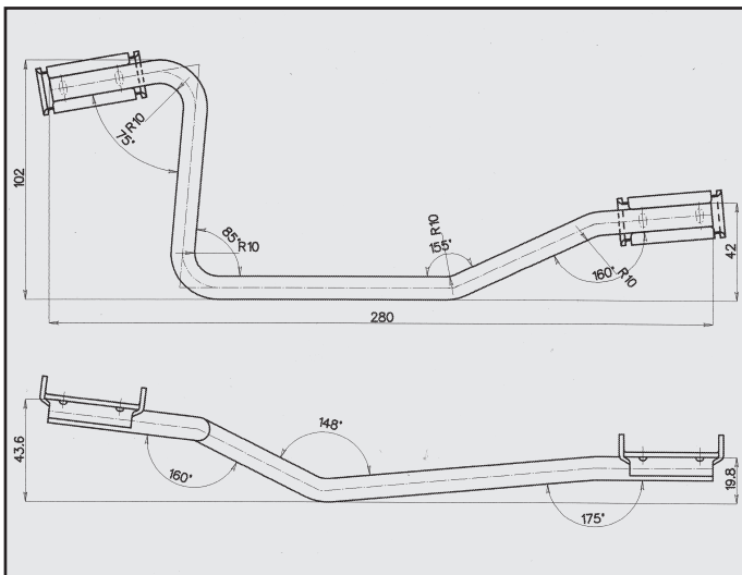
CITROEN XSARA PICASSO ATTACCO POSTERIORE COD. AT 141206
