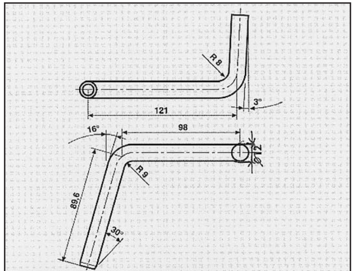
VOLKSWAGEN GOLF 92 1.400 e 1.800 CATALIZZATA ATTACO posteriore COD. AT 860117
