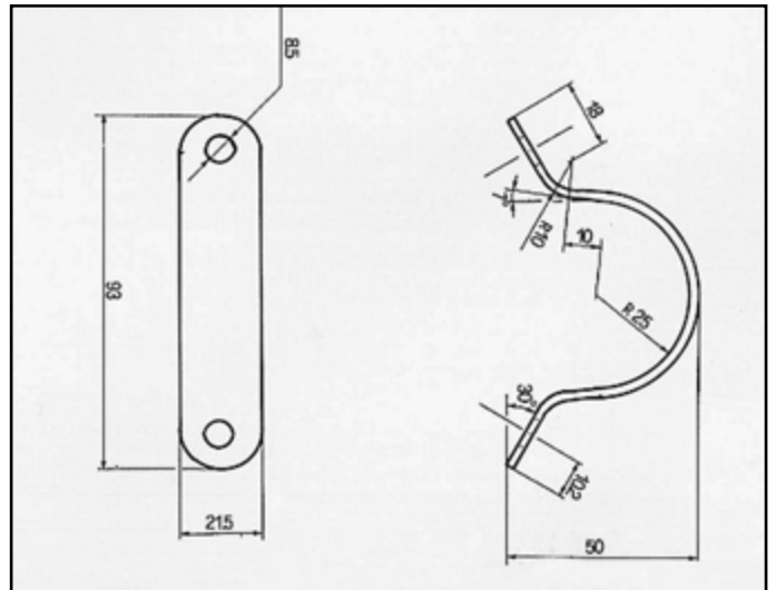
FIAT 242 BENZINA E DIESEL ATTACCO per posteriore COD. AT 241402
