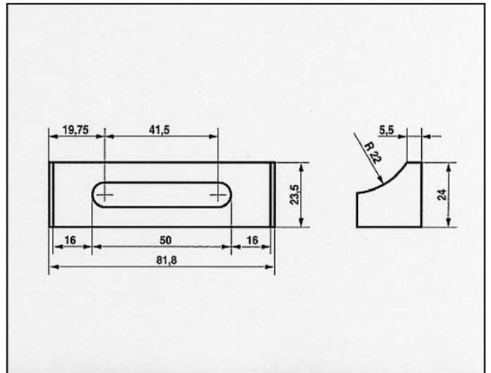
VOLVO 344-60 ATTACCO COD. AT 880601
