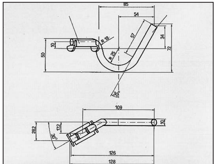
ESCORT XR3 ATTACCO per centrale COD. AT 260217
