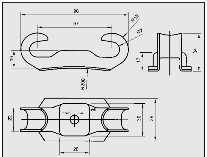
AUDI 50 80 ATTACCO per posteriore COD. AT 040205
