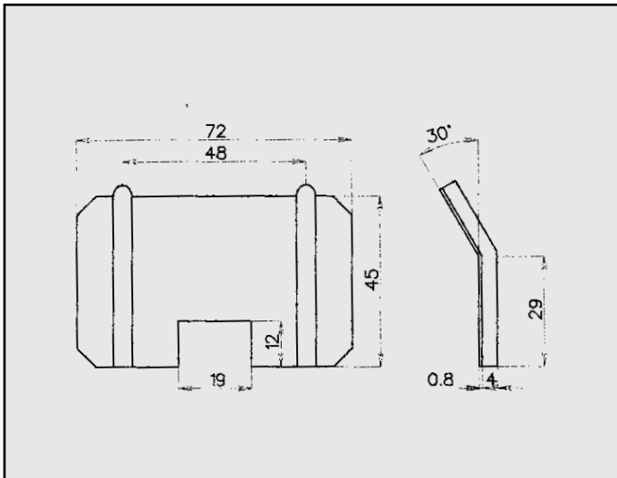
FIAT 600 PROTEZIONE CALORE COD. PC 243107
