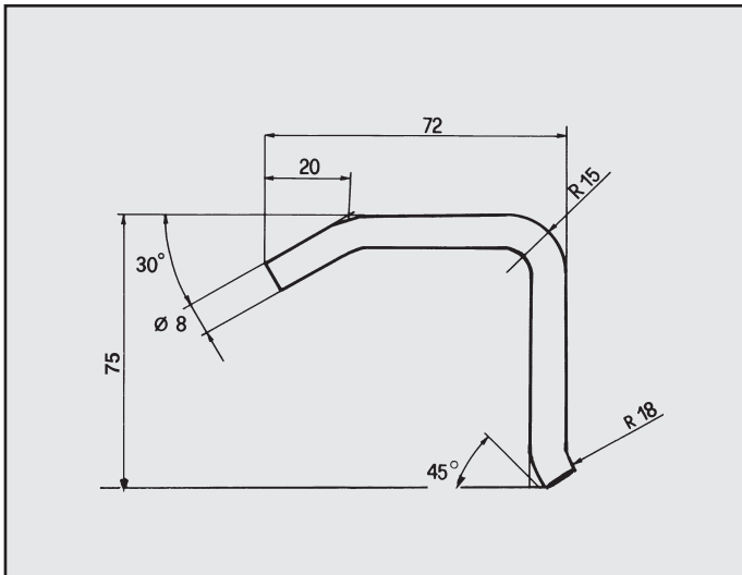
PALLAS 1300 ATTACCO per posteriore COD. AT 140501
