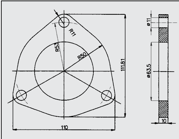
ROVER 200 FLANGIA COD. FL 621101
