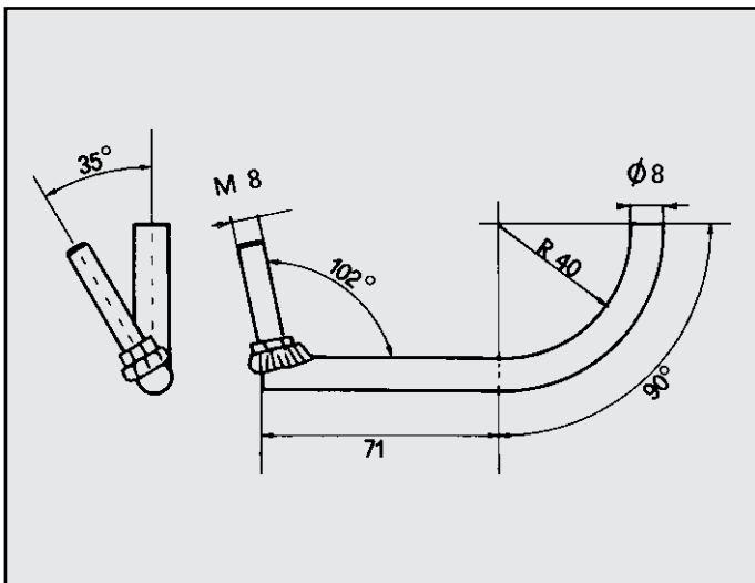
PULSAR 1600 COUPÈ ATTACCO per posteriore COD. AT 200102
