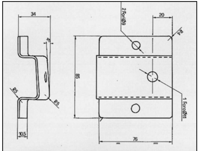
125 ATTACCO per posteriore COD. AT 240501 4241982
