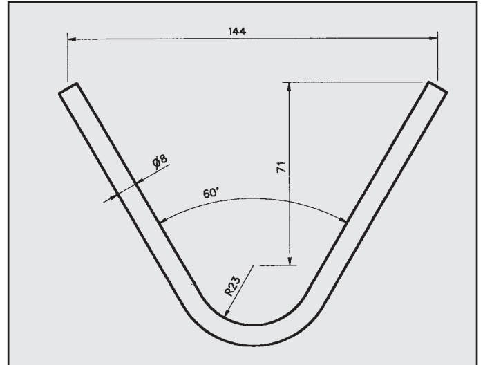
FORD SIERRA 2000 RINFORZO per posteriore COD. R 260615
