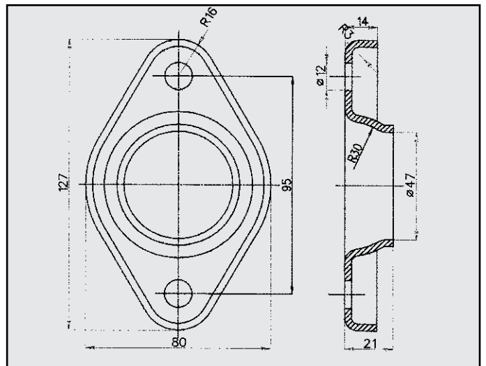
MAZDA 323 FLANGIA POSTERIORE COD. FL 420616
