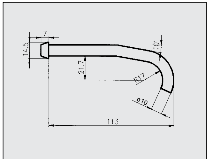
FIAT PUNTO 1.2 ATTACCO COD. AT 242226
