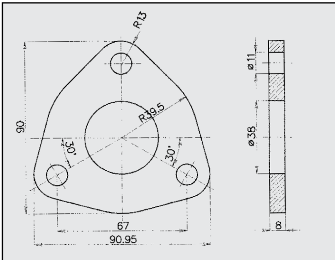
SKODA FELICITA FLANGIA COD. FL 690302
