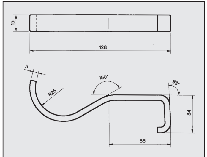
MERCEDES 380 ATTACCO per centrale COD. AT 440501
