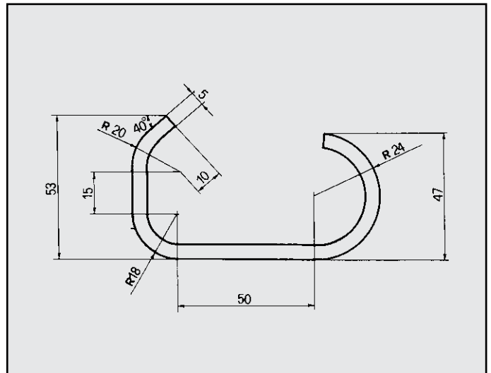
Y10 TOURING ATTACCO per posteriore COD. AT 080206
