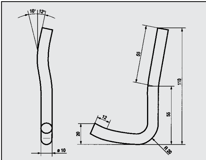
DAIHATSU CHARADE GTI-1987 ATTACCO per posteriore COD. AT 180202
