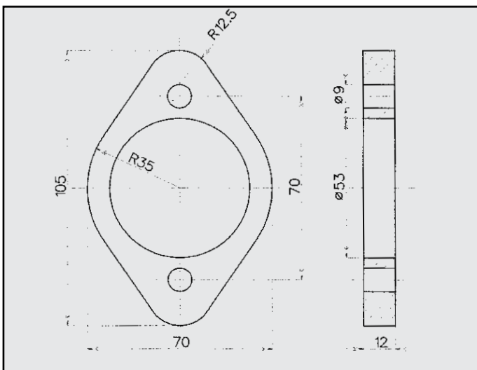
BMW 320 FLANGIA COD. FL 120408
