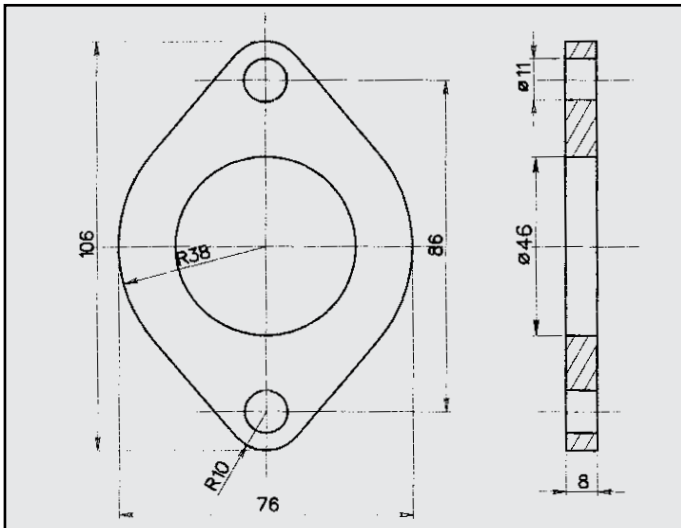
DAEWOO LANOS FLANGIA COD. FL 160202
