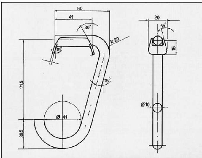
CORSA 1000-1200-1300 ATTACCO per posteriore COD. AT 520104
