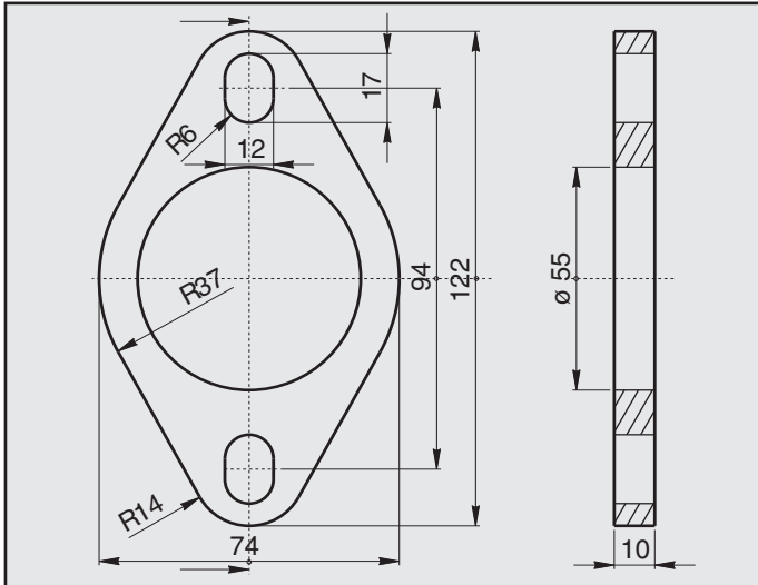
FORD ESCORT FLANGIA COD. FL 260270
