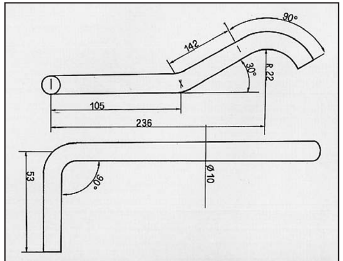
CIVIC/CRX ATTACCO per posteriore COD. AT 280412
