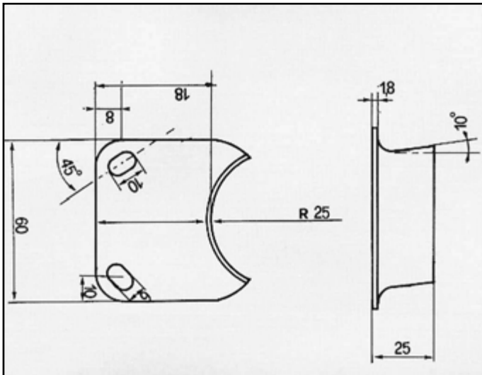
ARGENTA TURBO DIESEL ATTACCO per centrale COD. AT 241203
