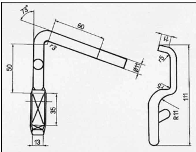
RITMO TURBO DIESEL ATTACCO per centrale COD. AT 240806
