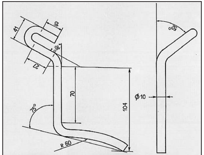
626 FWD ATTACCO per anteriore sx COD. AT 420508
