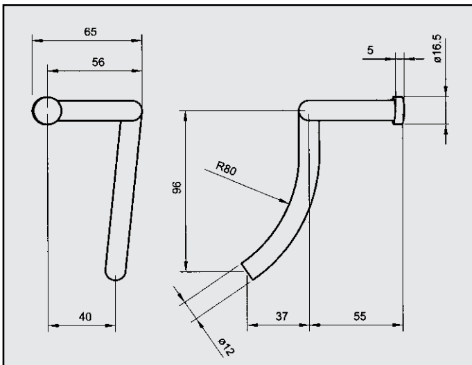
AUDI A4 1.6 1.8 ATTACCO per posteriore COD. AT 040601
