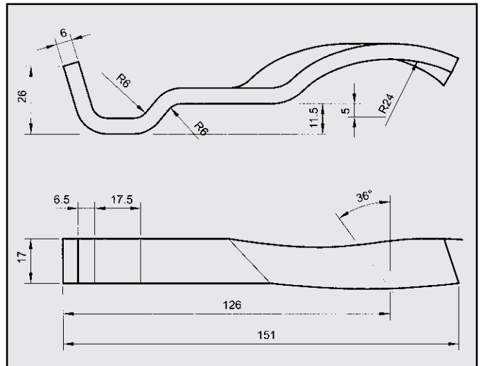
FIAT TEMPRA 1.4 ATTACCO per posteriore COD. AT 241906
