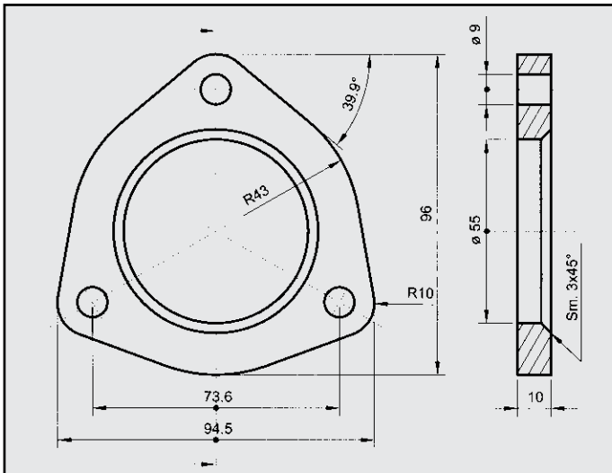
LANCIA DELTA FLANGIA COD. FL 380344
