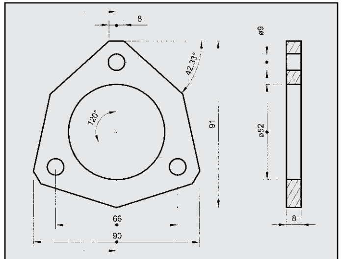
ALFA ROMEO GIULIA GT FLANGIA COD. FL 020404
