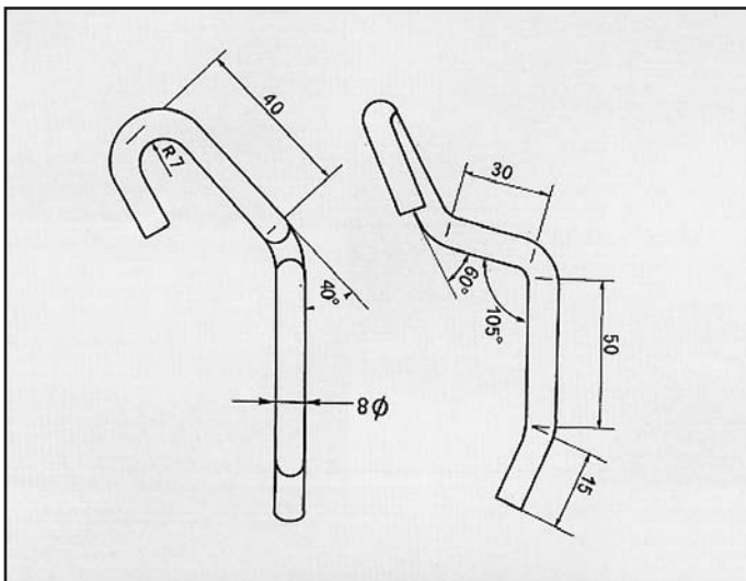
3500 V8 ATTACCO per centrale COD. AT 620101
