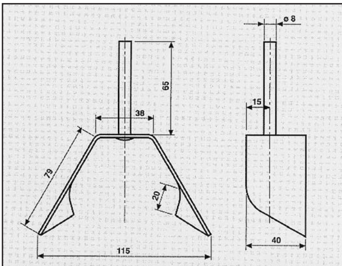
VOLVO 740 ATTACCO per posteriore COD. AT 880207 018254
