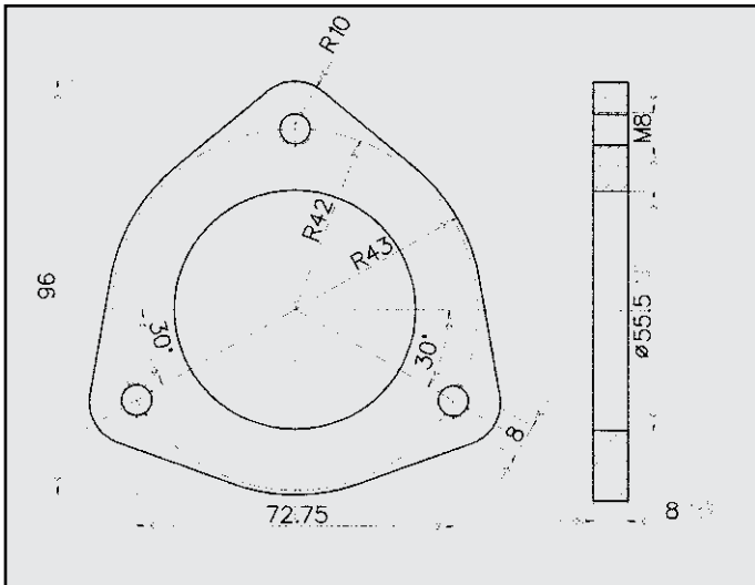
VOLKSWAGEN FLANGIA COD. FL 860026
