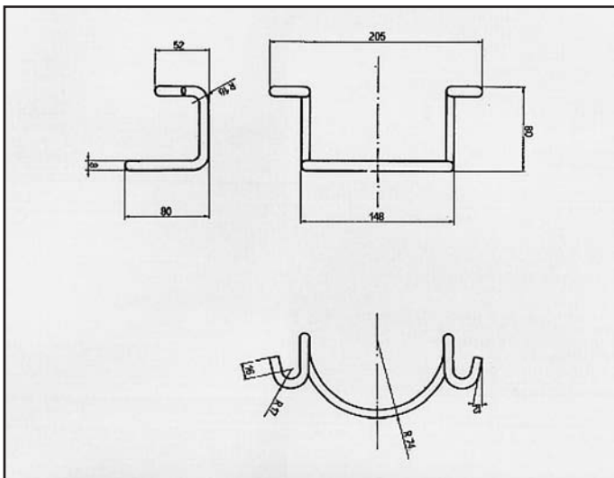
1501 ATTACCO per posteriore COD. AT 780103 0049309007
