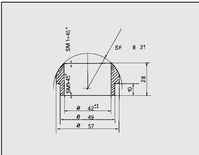
CITROEN VISA CHRONO ANELLO per posteriore \varnothing esterno mm 57 \varnothing interno mm 42 COD. AN 140101
