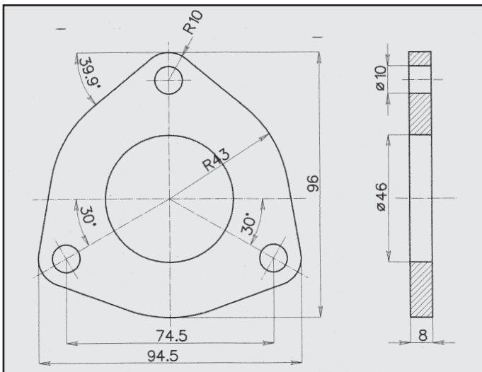
OPEL ASTRA FLANGIA COD. FL 520929
