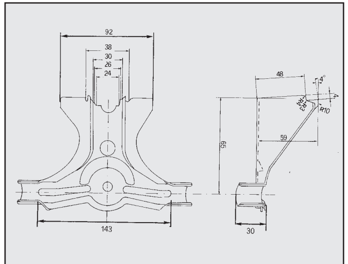
190 E ATTACCO per posteriore COD. AT 440302
