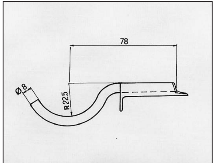
ESCORT/ORION 1600 ATTACCO per posteriore COD. AT 260223
