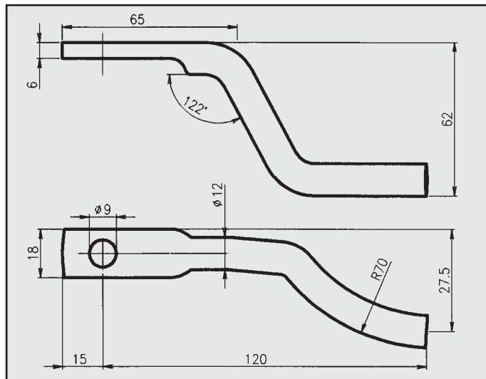
MITSUBISHI PAJERO '90 ATTACCO centrale COD. AT 460210
