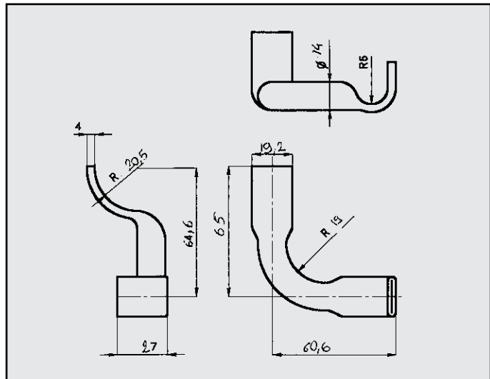
PANDA FIRE 4X4 ATTACCO per posteriore COD. AT 240107 7550388
