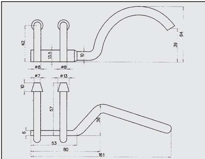
LANCIA Y 1.2i 16V ATTACCO COD. AT 381201
