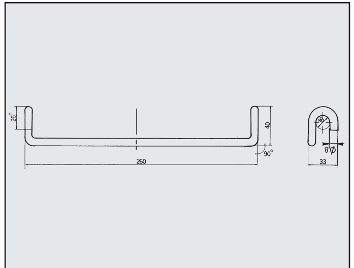
ALFA GTV 6 ATTACCO per centrale COD. AT 020601
