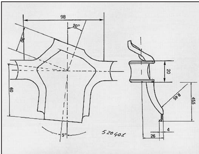
REKORD ATTACCO per centrale COD. AT 520401
