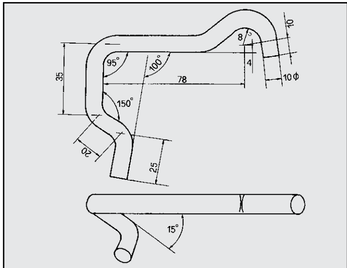
ALFA MILANO ATTACCO per posteriore dx COD. AT 020704
