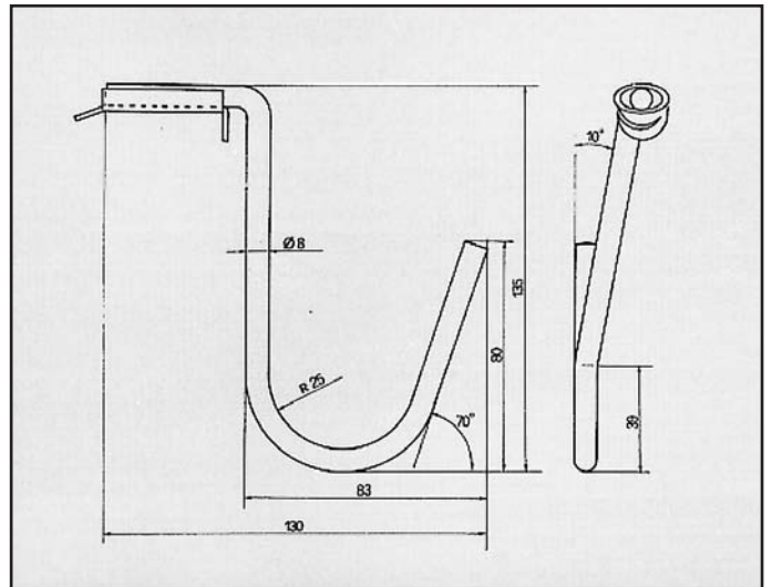
ESCORT 1600/81 ATTACCO per posteriore COD. AT 260214
