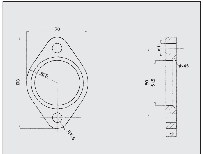
OPEL ASTRA-CENTRALE FLANGIA COD. FL 520930
