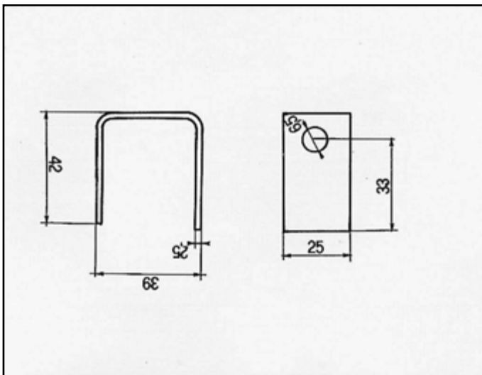
127-1050 SUPER ATTACCO per posteriore COD. AT 240206
