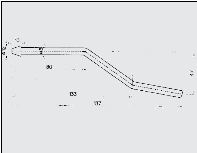
FIAT PUNTO ATTACCO COD. AT 242221
