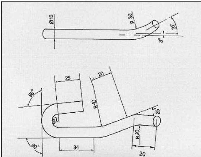
RX7 SAVANNA GTX ATTACCO per posteriore COD. AT 420402
