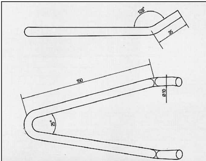
626 16V RINFORZO COD. R. 420511
