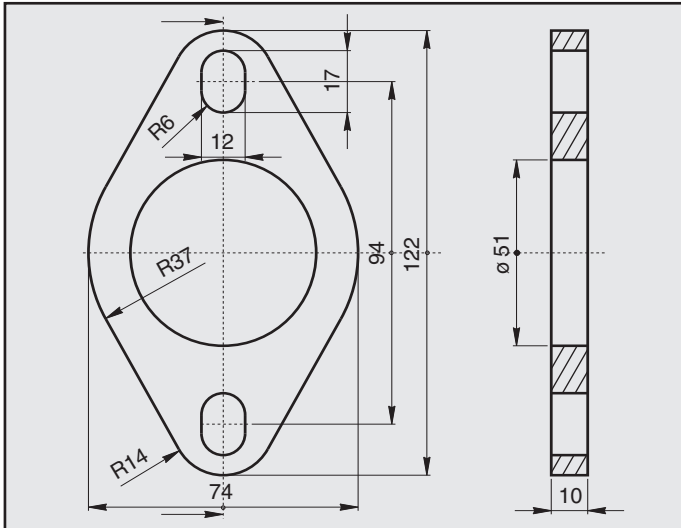
FORD ESCORT ORION FLANGIA COD. FL 260269
