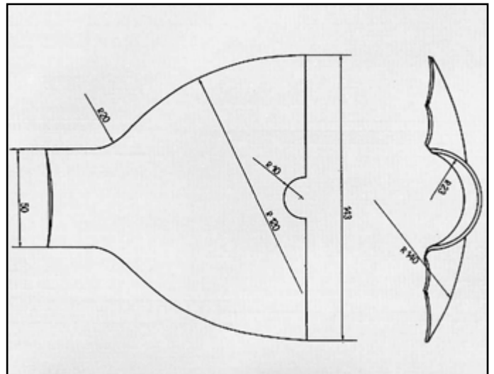
TIPO RINFORZO COD. R 241705
