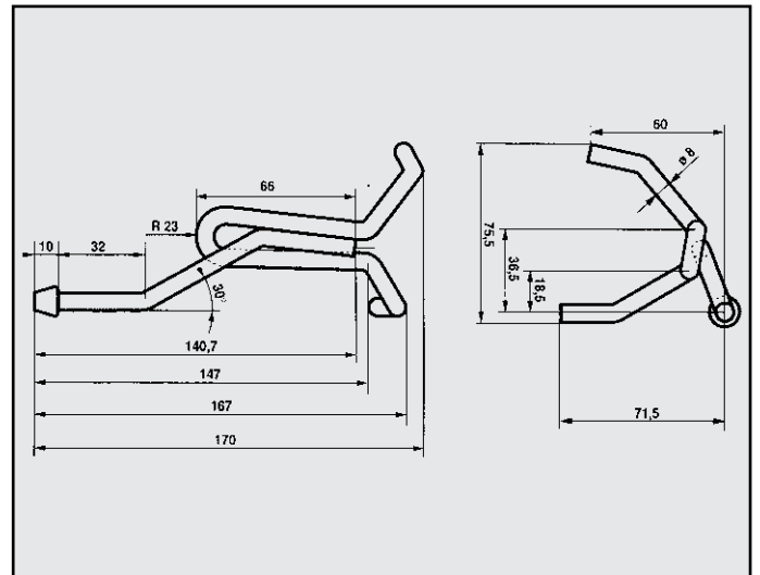
FIAT PUNTO GT ATTACCO centrale COD. AT 242204
