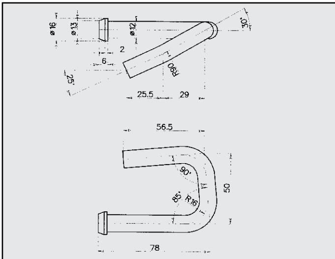
ALFA GTV ATTACCO ANTERIORE COD. AT 020609
