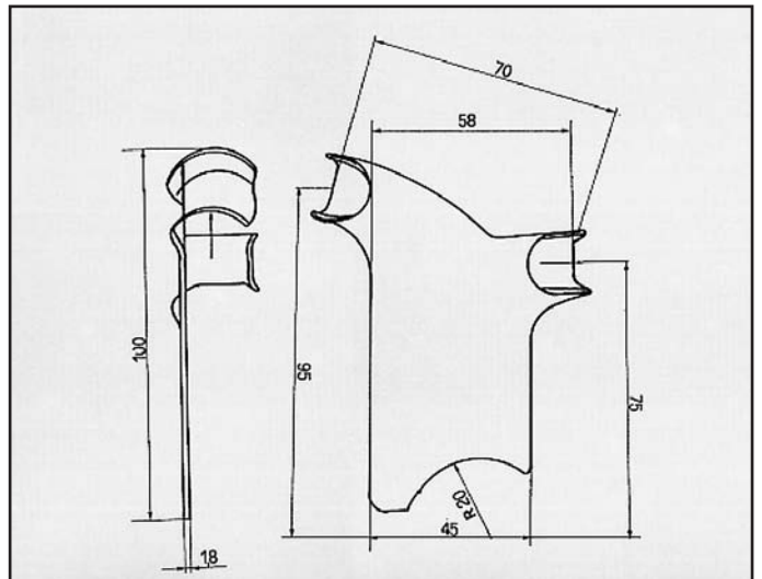
R14 ATTACCO per posteriore COD. AT 600404
