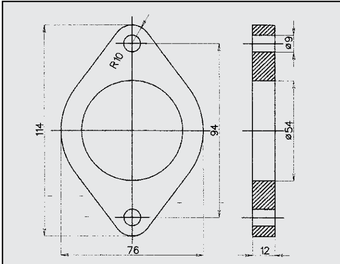
FIAT MULTIPLA FLANGIA COD. FL 242611
