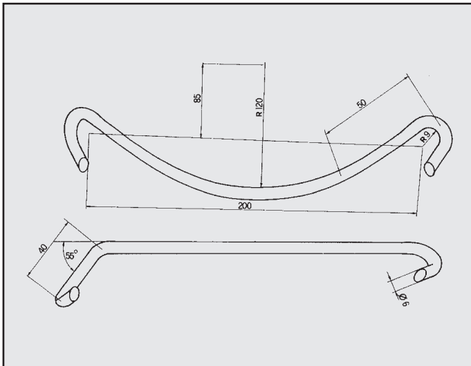
ROVER ATTACCO per posteriore COD. AT 620001
