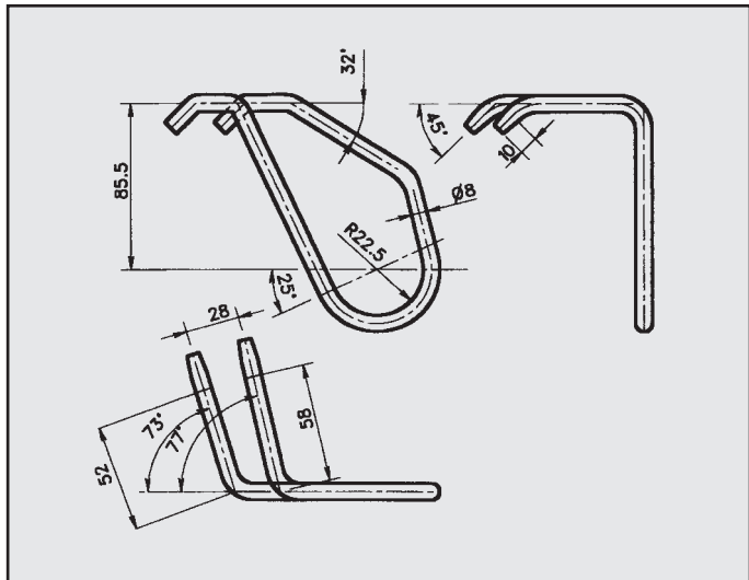
LANCIA DEDRA 1.8 I.E. ATTACCO COD. AT 380808
