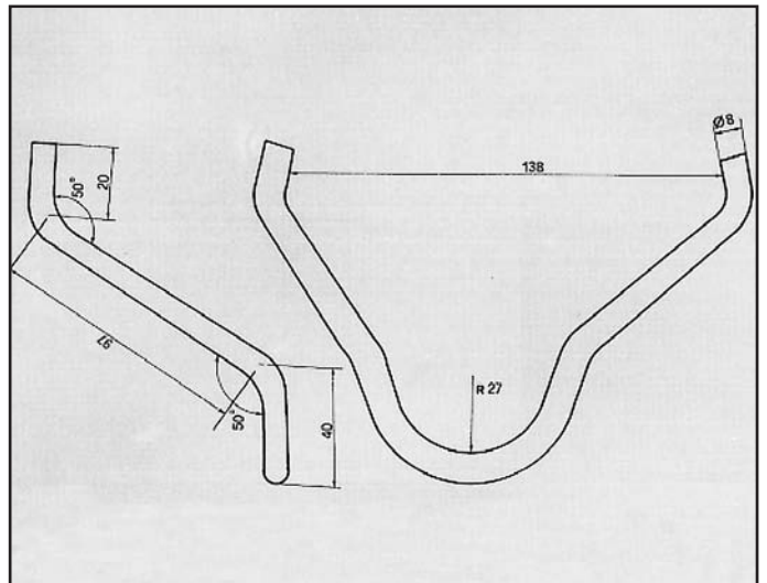
OMEGA 2000 RINFORZO COD. R 520602
