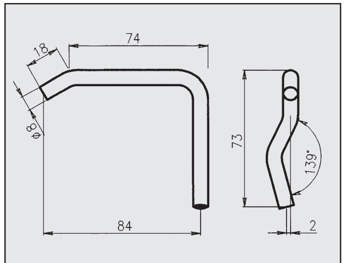
RENAULT ESPACE 2.2 ATTACCO per centrale COD. AT 601104
