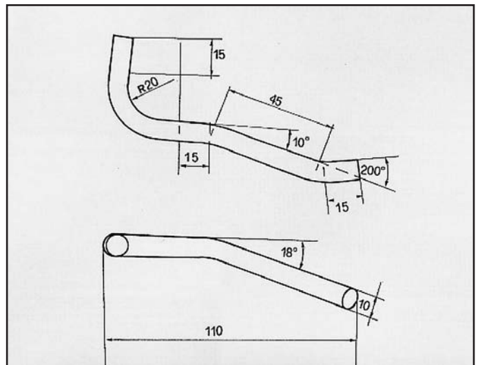
R19 ATTACCO per anteriore COD. AT 600902
