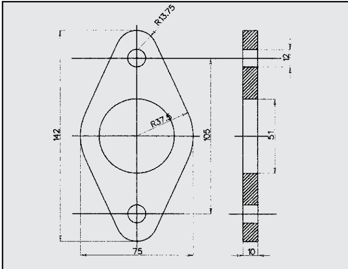
FORD MONDEO 1.6 1.8 FLANGIA COD. FL 261216
