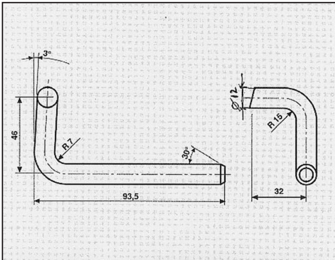
VOLKSWAGEN GOLF 1.400 e 1.800 CATALIZZATA 92 ATTACCO posteriore COD. AT 860118
