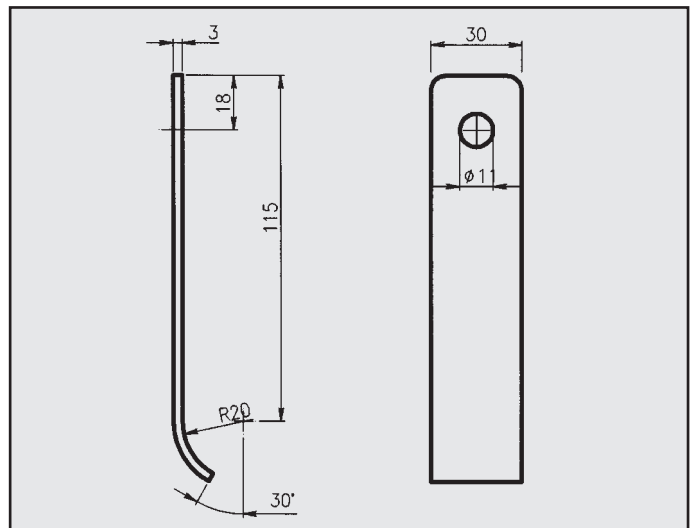
SUZUKI SJ 413 1.3 4X4 ATTACCO per posteriore COD. AT 720305
