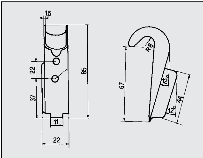
AUDI 80 GTI-GTE TURBO DIESEL ATTACCO per posteriore COD. AT 040302 055253409C-J
