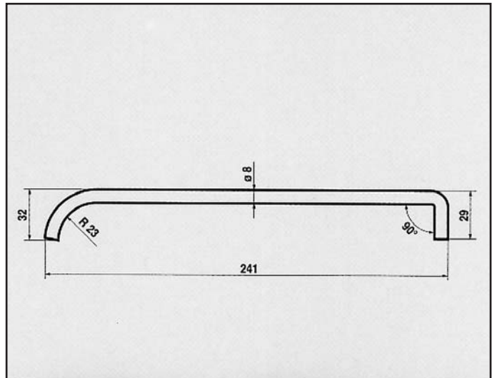
PEUGEOT RINFORZO marmitta posteriore COD. R 540701
