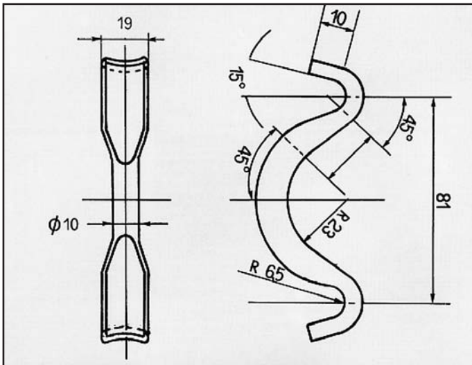
ASCONA 1.8 IE ATTACCO per centrale COD. AT 520211
