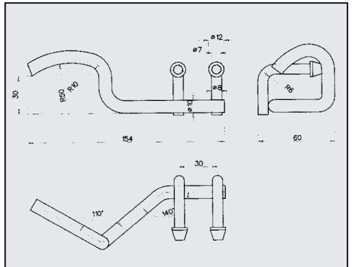
FIAT PUNTO 55 ATTACCO COD. AT 242241
