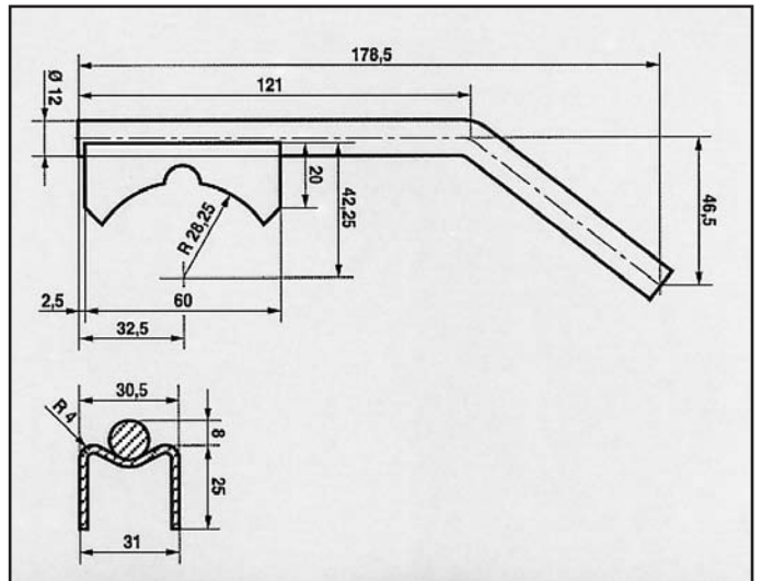
LANCIA DELTA HF ATTACCO posteriore COD. AT 380328
