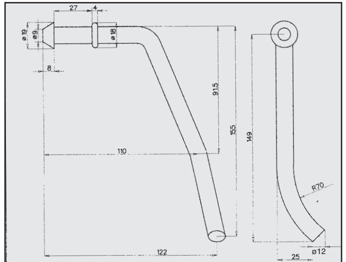
PEUGEOT 206 1.4 ATTACCO COD. AT 541203
