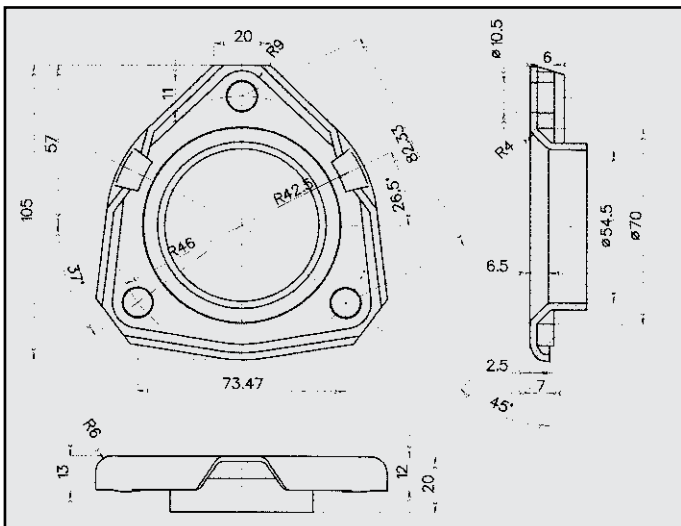
PEUGEOT 206 FLANGIA COD. FL 541211
