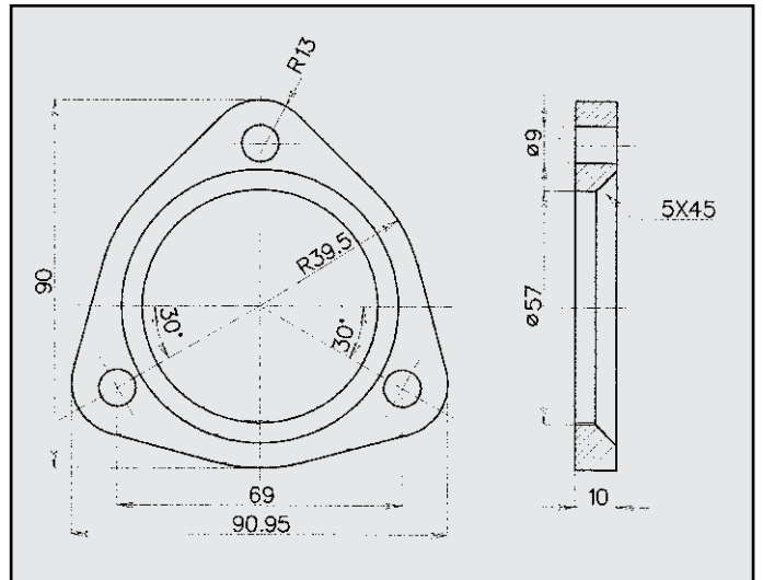
ALFA 145 FLANGIA COD. FL 021108
