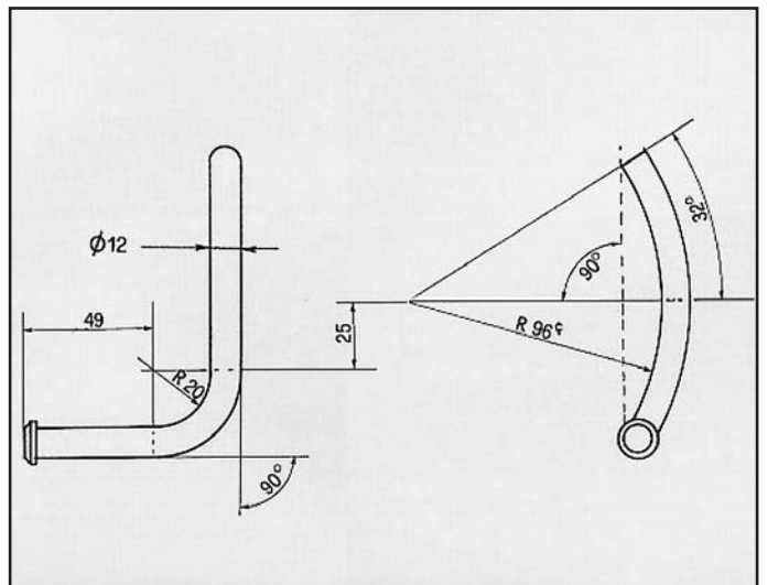
COROLLA FX ATTACCO per posteriore COD. AT 800405
