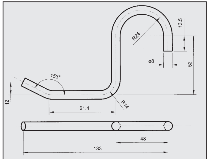
RENAULT EXPRESS 1,6 D ATTACCO posteriore COD. AT 600119
