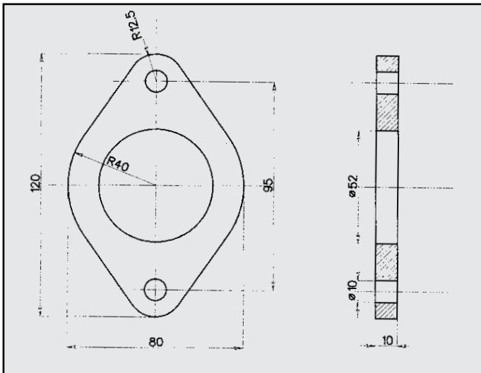
RENAULT CLIO FLANGIA COD. FL 601318
