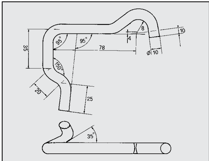
ALFA MILANO ATTACCO per posteriore sx COD. AT 020703
