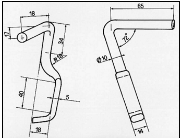
RITMO TURBO DIESEL ATTACCO per posteriore COD. AT 240808
