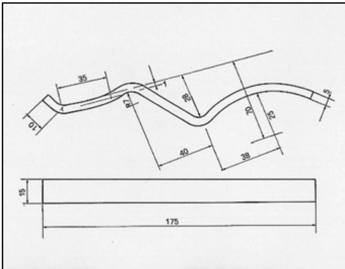
UNO 60S-60SX ATTACCO per posteriore per centrale COD. AT 240915
