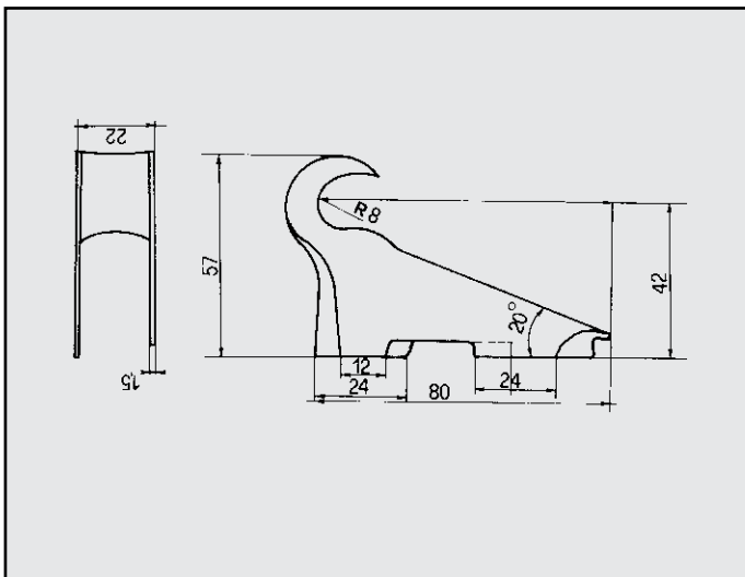
AUDI 50 ATTACCO per posteriore COD. AT 040202
