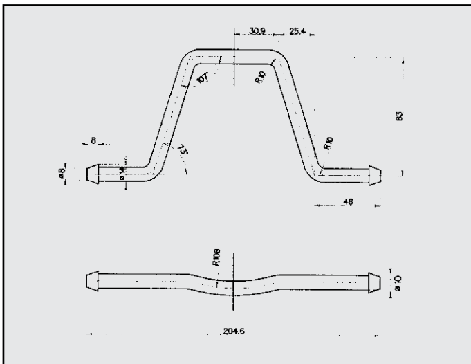
DAEWOO NUBIRA ATTACCO CENTRALE COD. AT 160309
