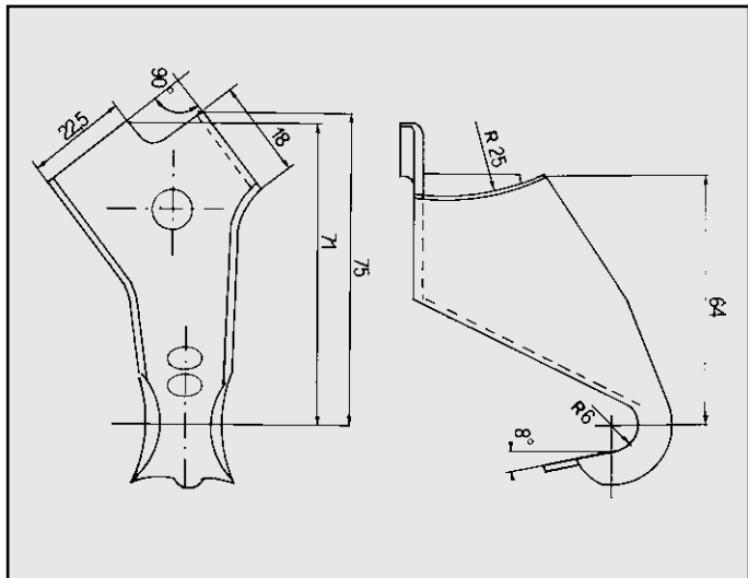
AUDIA 80 1600 D /1600/1800 ATTACCO anteriore per centrale COD. AT 040305 893253409B 811253409C
