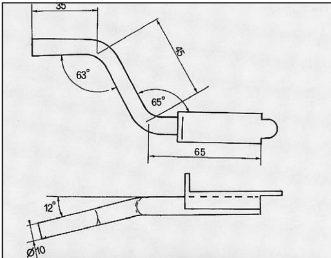
SCIROCCO 1800 ATTACCO per posteriore COD. AT 860114
