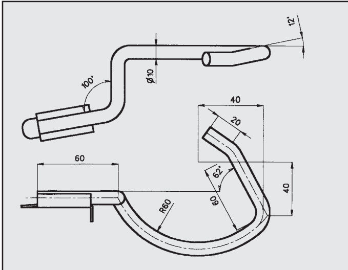
FIESTA 1400 ATTACCO per centrale COD. AT 260312
