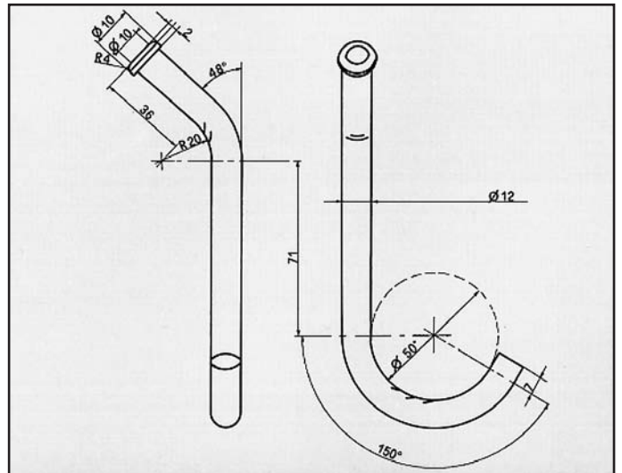
NEW CELICA ATTACCO per centrale COD. AT 800301
