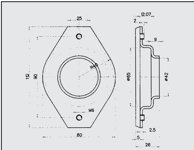
PEUGEOT 205 FLANGIA COD. FL 540319
