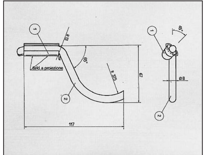
ESCORT 1100 2GL/81 ATTACCO per centrale COD. AT 260232
