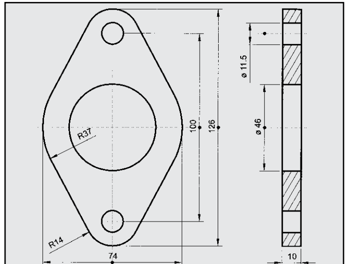
FORD FIESTA 1.2 FLANGIA COD. FL 260344
