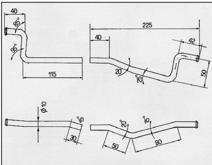
FAMILIA EGI TURBO ATTACCO per anteriore COD. AT 420102
