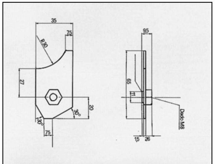
131 ATTACCO per posteriore COD. AT 240603 4409852 4333791 4333862
