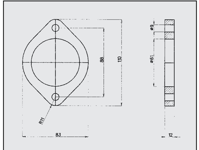
FIAT MAREA/BRAVO 2.0 FLANGIA COD. FL 242818
