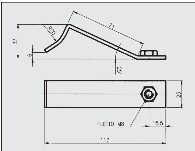
SUZUKI SJ 413 1.3 ATTACCO per posteriore COD. AT 720302
