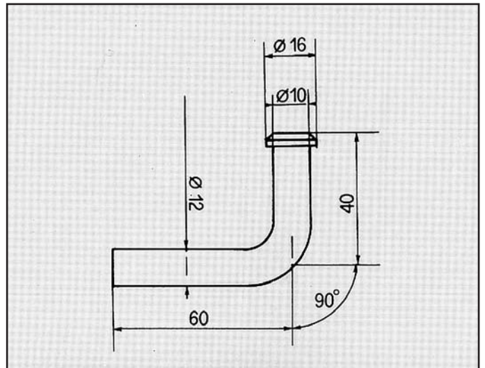
COROLLA 4ALC ATTACCO per posteriore COD. AT 800411
