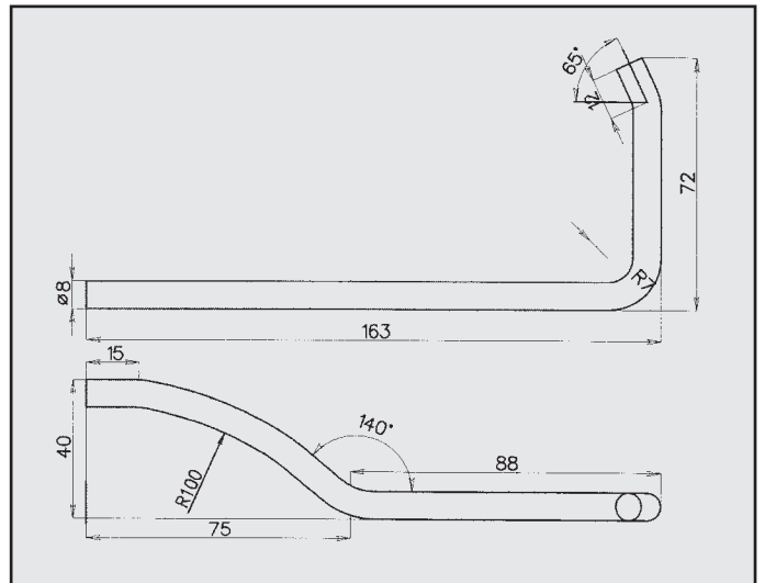
PEUGEOT 205 GTI ATTACCO COD. AT 540307
