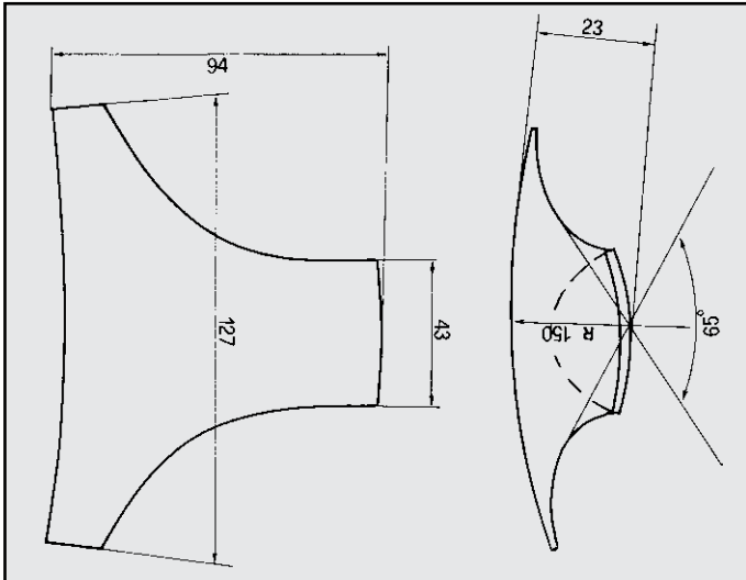
ALFASUD RINFORZO per posteriore COD. R 020101
