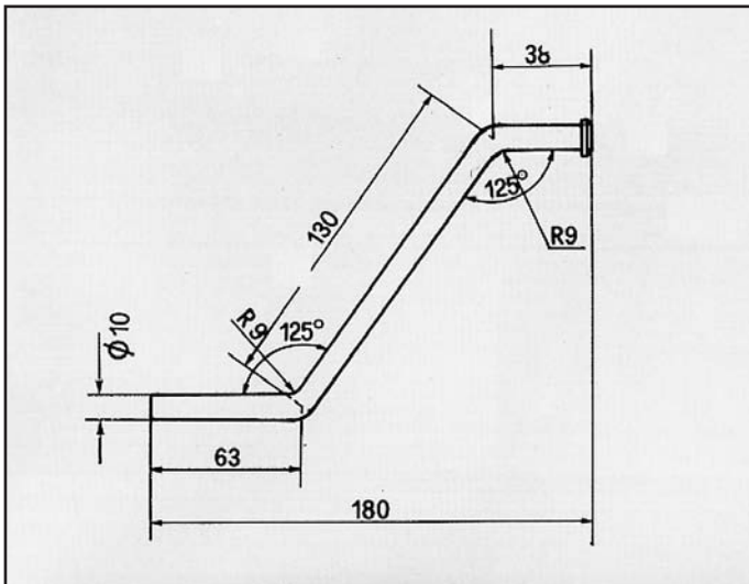
FAMILIA EGI ATTACCO per centrale COD. AT 420101
