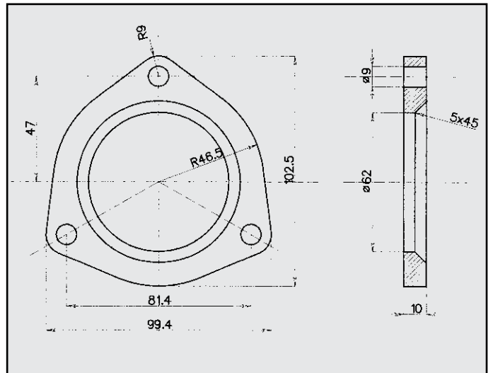
AUDI A6 2.5 TDI FLANGIA COD. FL 040803
