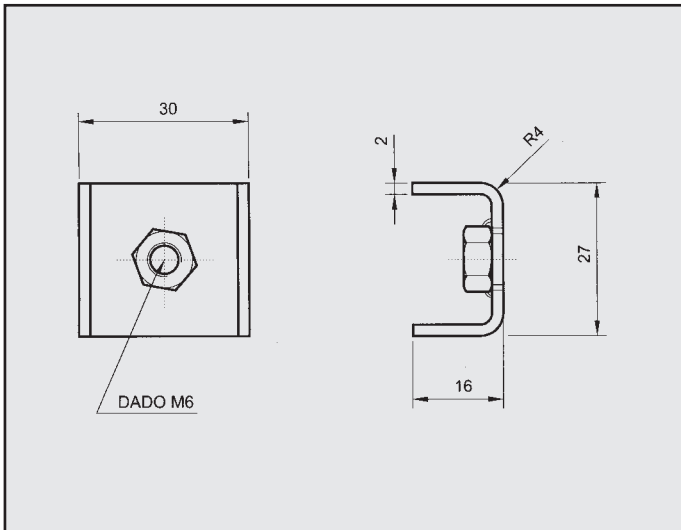
LANCIA DEDRA ATTACCO COD. AT 380811
