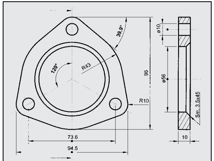
ALFA 164 FLANGIA COD. FL 020906
