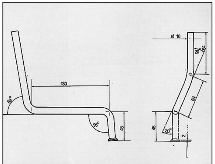
626 2000 16V ATTACCO anteriore sx per anteriore COD. AT 420516
