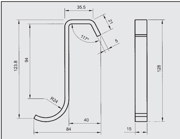
MERCEDES 280 S SE ATTACCO COD. AT 440401
