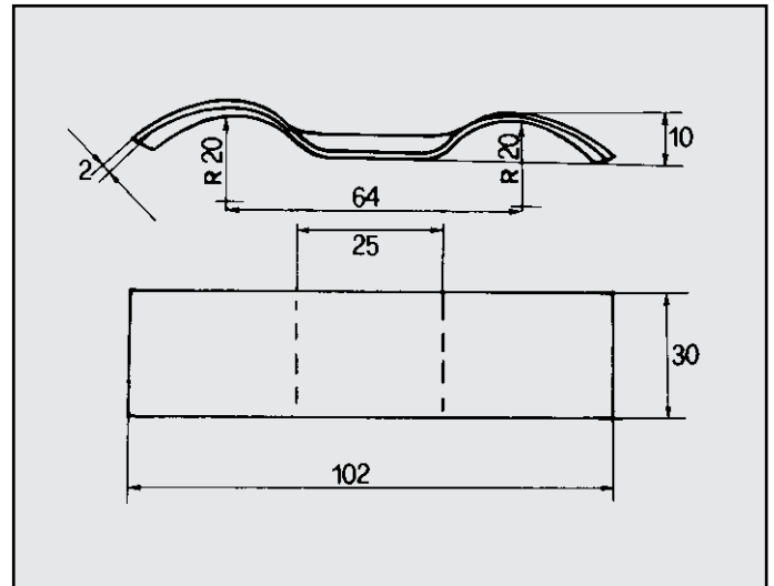
A 112 ABARTH PIASTRINA su code COD. R 080104
