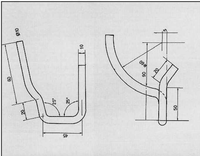
R19 ATTACCO per posteriore COD. AT 600903
