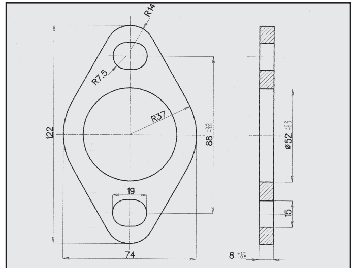
OPEL VECTRA FLANGIA COD. FL 520833
