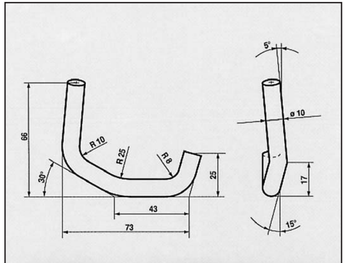
HONDA CIVIC SI/1986-87 ATTACCO per posteriore COD. AT 280417
