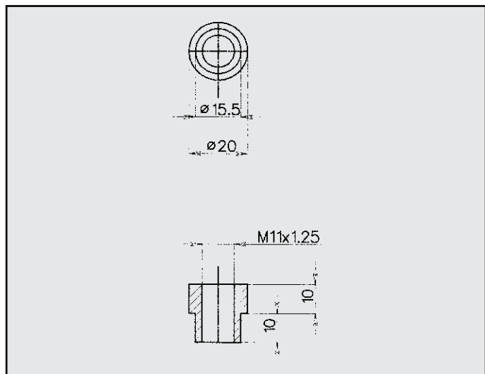
FIAT PUNTO DADO COD. DA 242235
