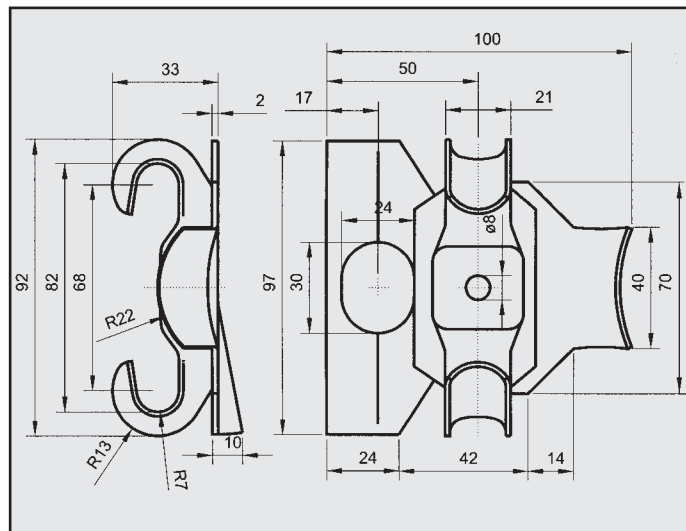
VW GOLF 1.1 1.3 1.6 1.8 ATTACCO RINFORZO per posteriore COD. AT 860106
