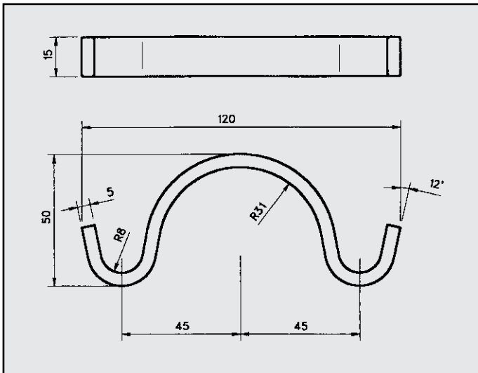
FIAT DUCATO TURBO ATTACCO per posteriore COD. AT 241504
