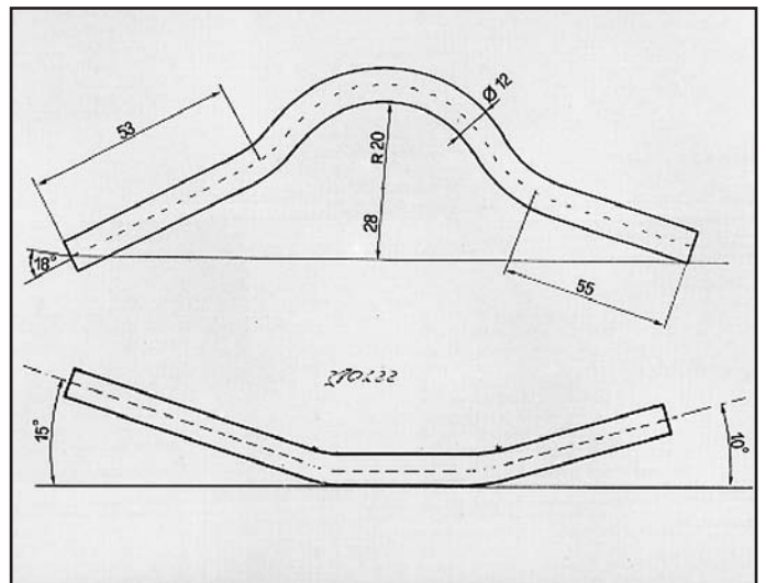
DELTA 1300-1500 ATTACCO per posteriore COD. AT 380322
