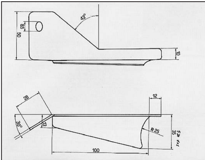
304 ATTACCO per posteriore COD. AT 540101 1724-41
