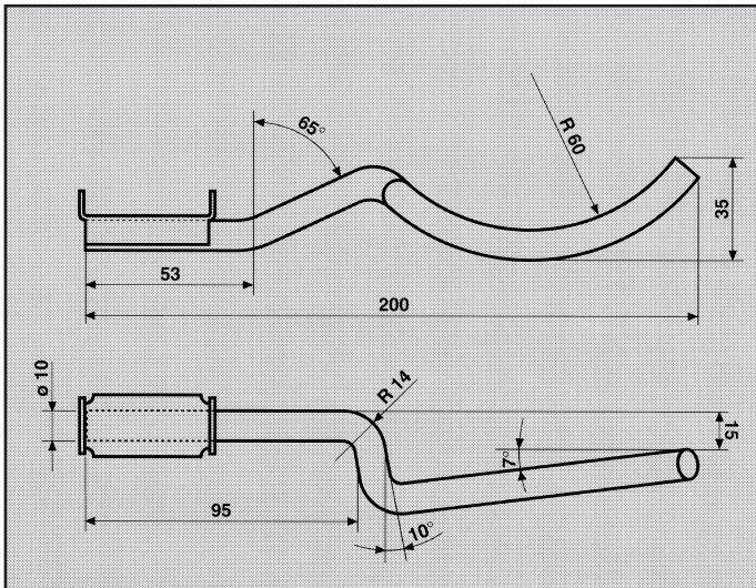
CITROEN ZX 1.4 REFLEX 03/91 1.6 CATALIZZATA ATTACCO posteriore COD. AT 140901 96041796 96041798
