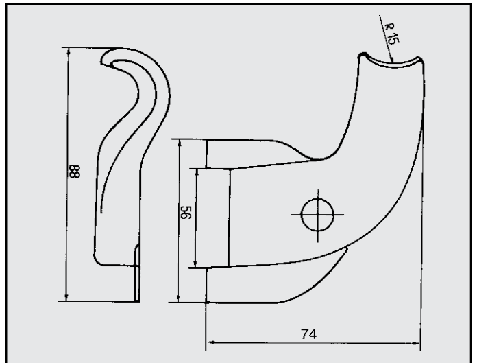
AUDI 50 STAFFA per centrale COD. AT 040204
