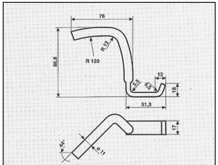
FIAT CINQUECENTO NUOVA ATTACCO posteriore COD. AT 242103
