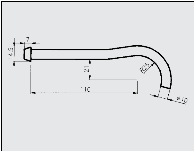
FIAT PUNTO 1.2 ATTACCO COD. AT 242227
