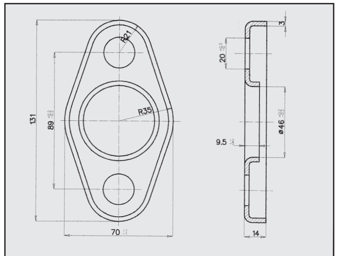
OPEL CORSA 1.6 GSI FLANGIA COD. FL 520319
