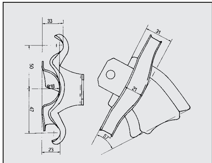
ALFASUD 1ª serie - 2ª serie / ALFA 33 ATTACCO posteriore per coda COD. AT 020106
