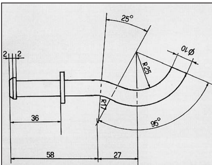
NEW FAMILIA GT TURBO ATTACCO per posteriore COD. AT 420201
