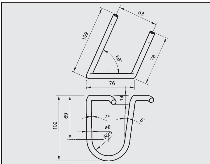
RENAULT R21 1.4 1.7 ATTACCO per posteriore COD. AT 601009
