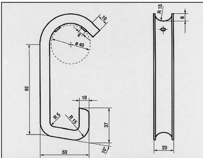
OPEL OMEGA ATTACCO per posteriore COD. AT 520605
