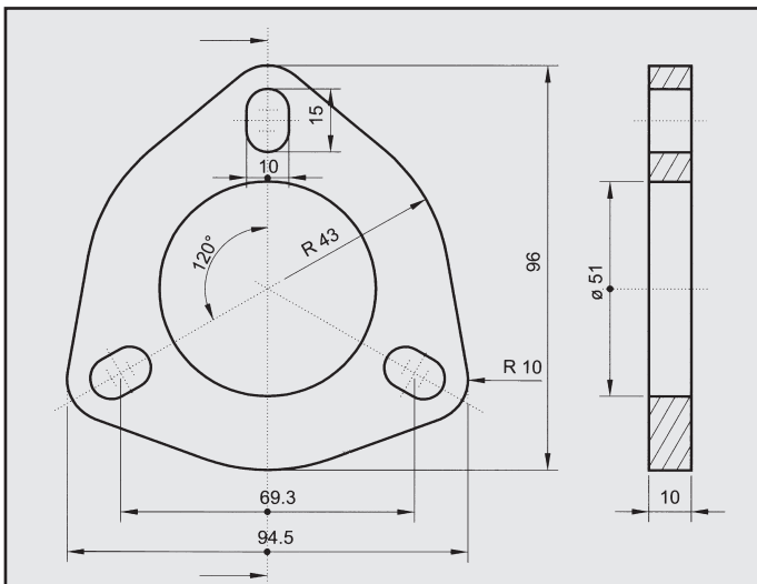
OPEL FLANGIA COD. FL 520014
