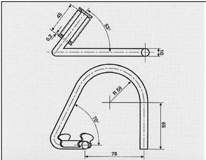
FORD FIESTA ATTACCO posteriore COD. AT 260323
