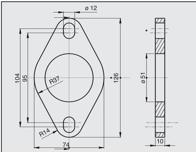
OPEL ASTRA 1.4 1.6 1.8 2.0 FLANGIA COD. FL 520919
