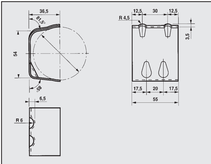
LANCIA THEMA 2.0 16V TURBO CAT RINFORZO COD. R 380710
