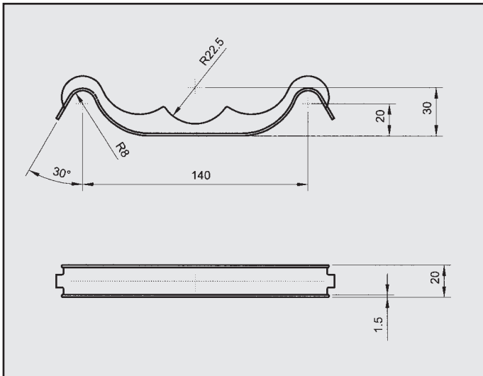
OPEL CORSA D TD ATTACCO COD. AT 520314
