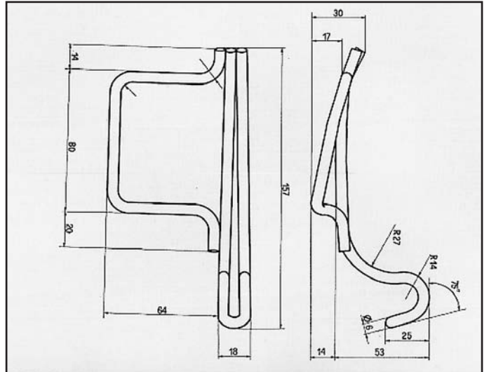
GOLF GTI 1800/84 ATTACCO per posteriore COD. AT 860111
