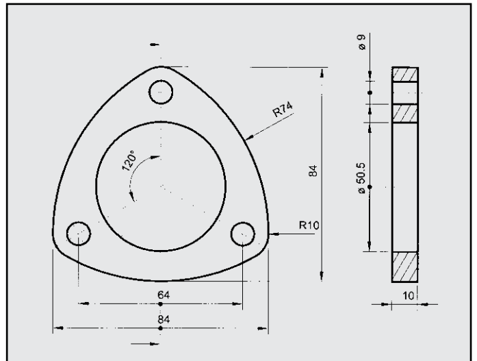
LANCIA DELTA HF TURBO FLANGIA COD. FL 380339
