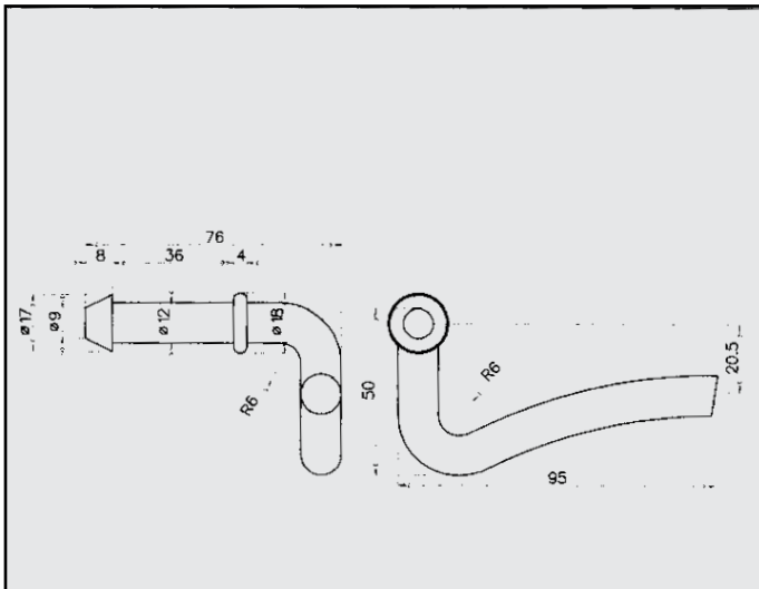
FIAT SCUDO 1.6 ATTACCO POSTERIORE COD. AT 243201
