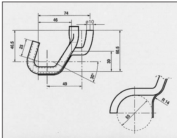
OPEL OMEGA 1991 ATTACCO per posteriore COD. AT 520607
