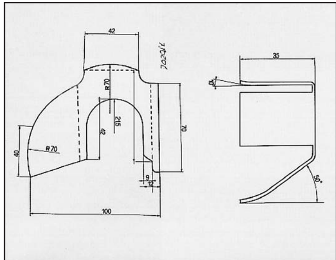
HORIZON RINFORZO per posteriore COD. R 780201 0059114807 0059129407
