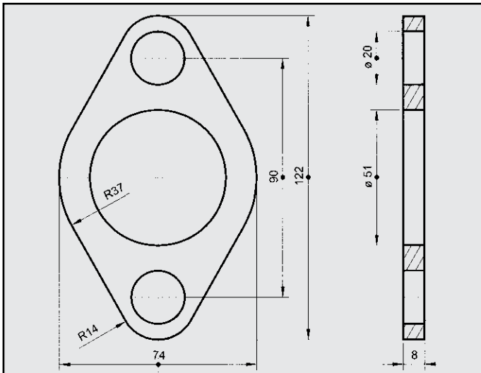
CITROEN AX 1.4 FLANGIA COD. FL 140711
