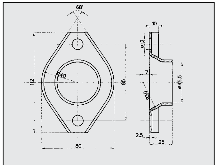
CITROEN FLANGIA COD. FL 140003
