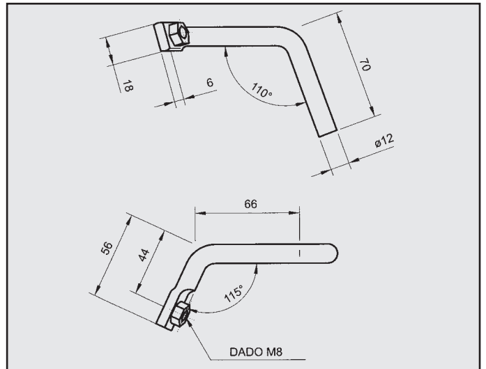
MITSUBISHI SPACE WAGON 2.0 ATTACCO per posteriore COD. AT 460305
