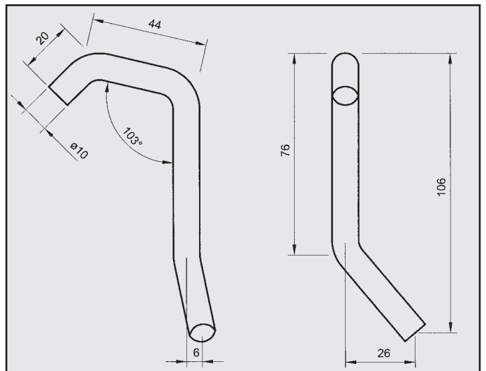
HONDA LEGEND 2.7i V6 24V ATTACCO per posteriore COD. AT 280909
