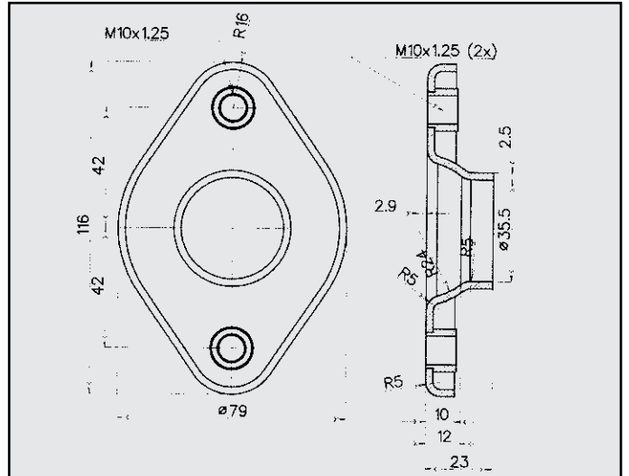
TOYOTA FLANGIA COD. FL 800010
