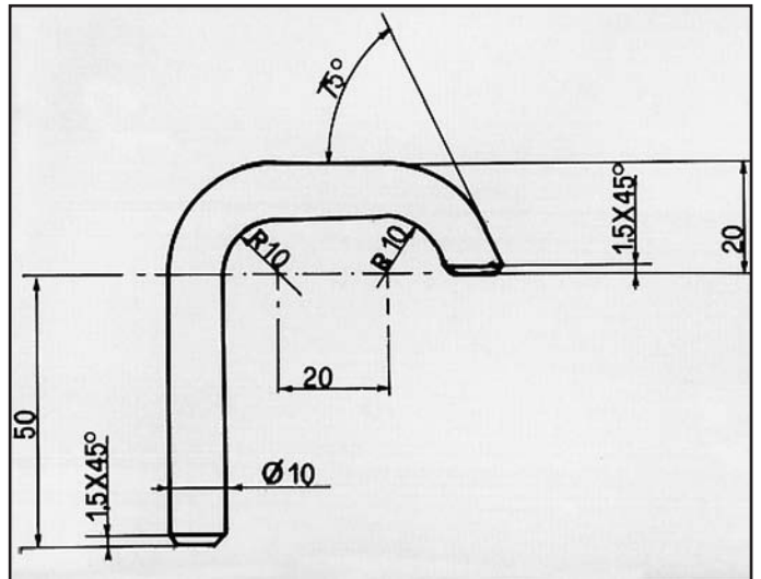
PRELUDE 1800 ATTACCO per posteriore COD. AT 280602
