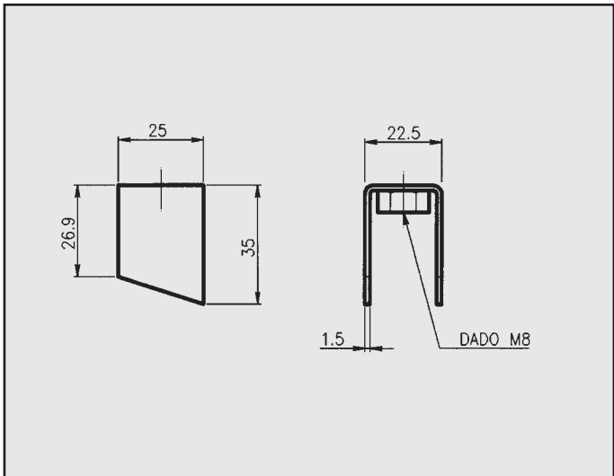
NISSAN BLUE BIRD 1.8 ATTACCO per centrale COD. AT 500504
