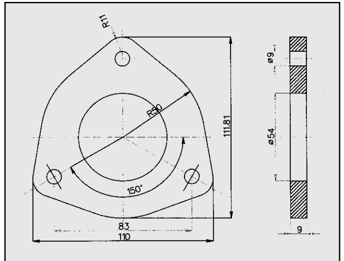
FIAT BRAVO FLANGIA COD. FL 242330
