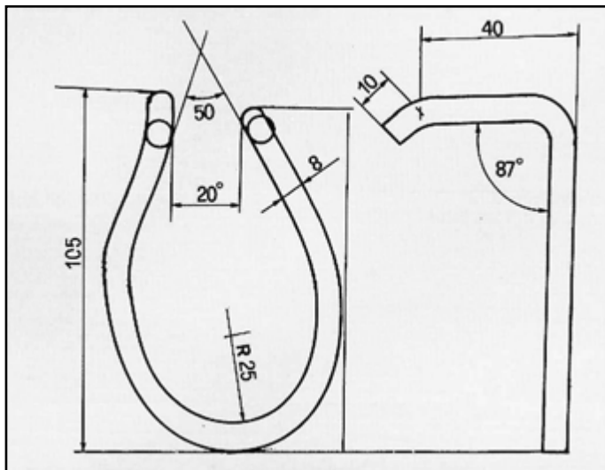
REGATA TURBO DIESEL ATTACCO per posteriore COD. AT 241110
