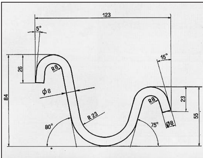
IBIZA ATTACCO per posteriore COD. AT 680103
