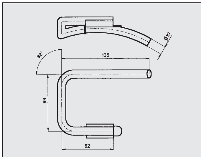
OPEL VECTRA 1400 - 1600 ATTACCO per posteriore COD. AT 520801
