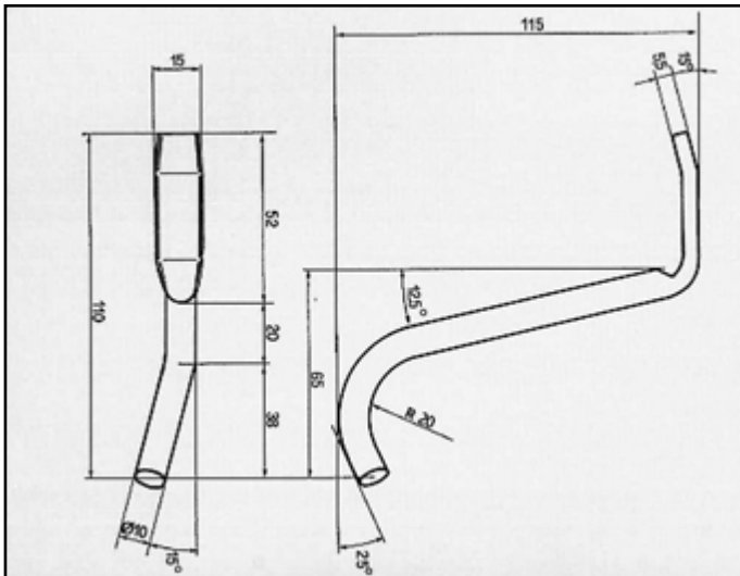
DUNA 60 ATTACCO per posteriore COD. AT 241001
