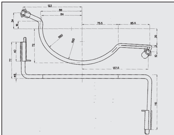
PEUGEOT 306 1.8 i CABRIO ATTACCO COD. R 540902
