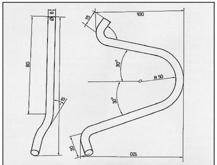
SUPRA 3.0 i TURBO RINFORZO COD. R 801002
