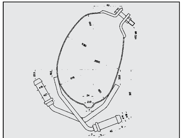
CITROEN BERLINGO FASCETTA POSTERIORE COD. F 141303
