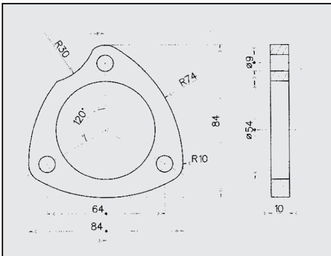
FIAT TIPO 1.9 TD FLANGIA COD. FL 241723
