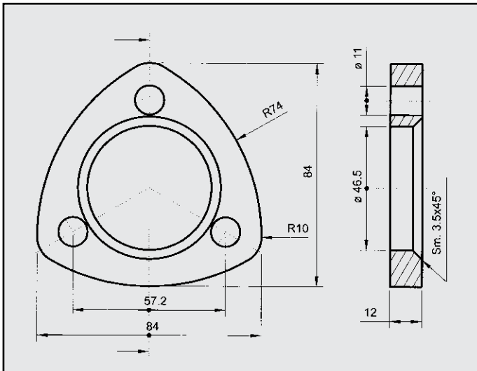
BMW FLANGIA COD. FL 120015
