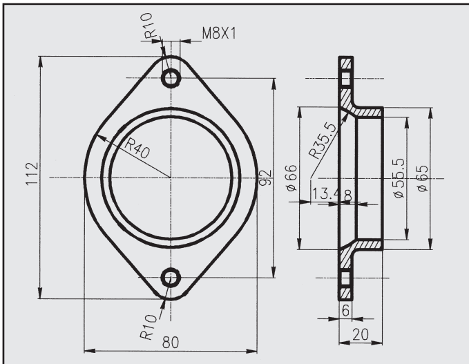
OPEL VECTRA FLANGIA COD. FL 520828
