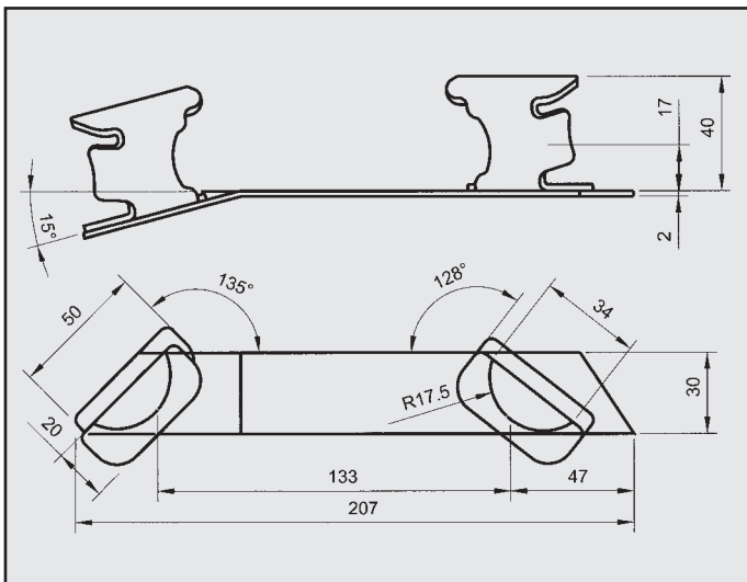
VOLVO 240 244 ATTACCO per centrale COD. AT 880501
