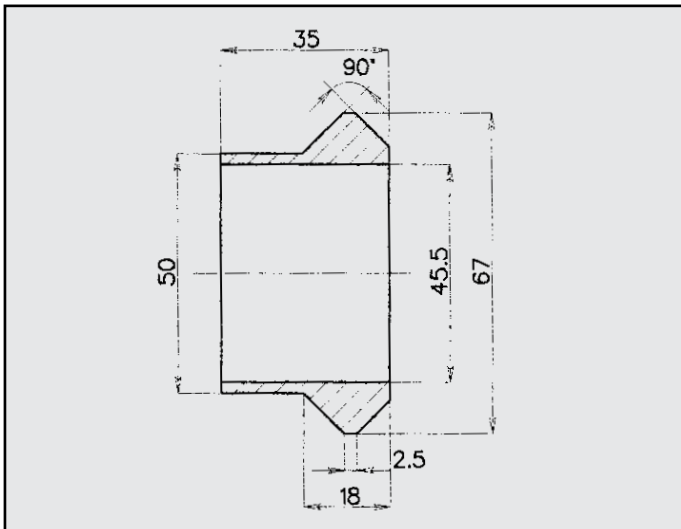
PEUGEOT 406 ANELLO COD. AN 541102
