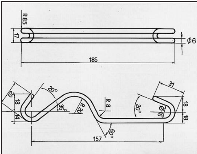
FUEGO ATTACCO per posteriore COD. AT 600701
