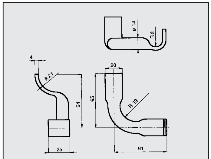
Y10 4x4 ATTACCO per tubo centrale COD. AT 080213
