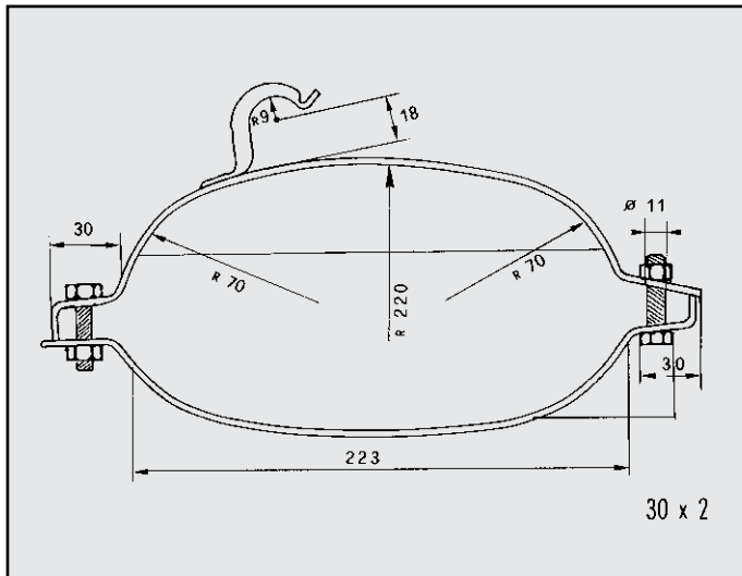
BOSI FASCETTA COD. F 100003
