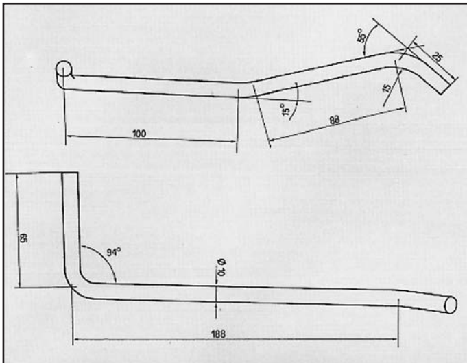
CIVIC 1.6/CRX RINFORZO COD. R. 280414
