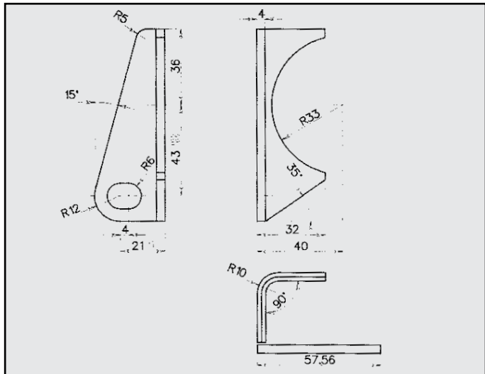
CITROEN AX 1.4 ATTACCO COD. AT 140717
