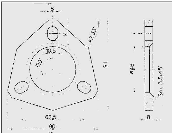
AUDI 80 DIESEL FLANGIA COD. FL 040312
