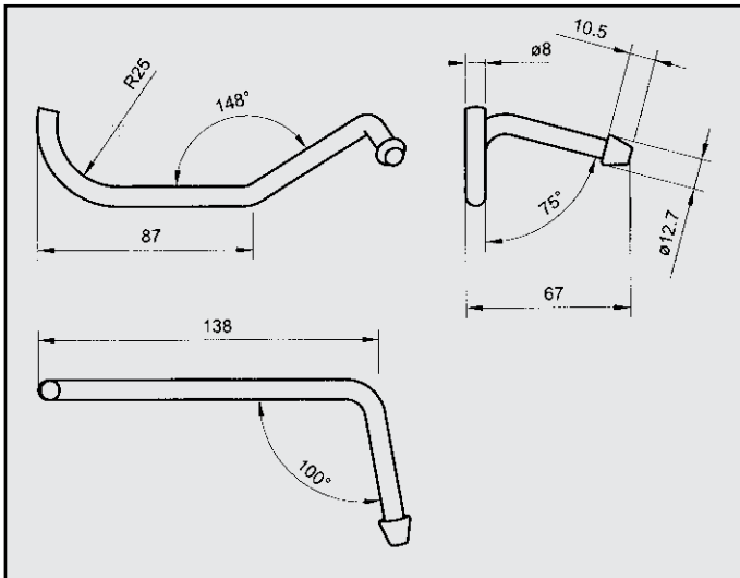
FIAT BRAVO BRAVA ATTACCO centrale posteriore COD. AT 242306
