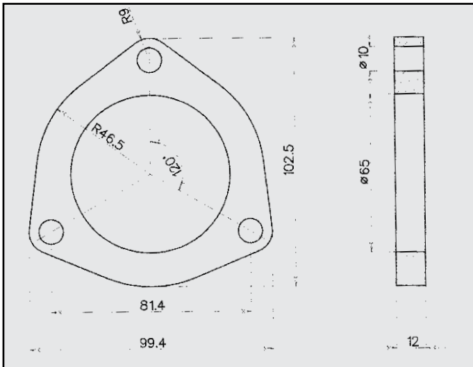
VOLKSWAGEN FLANGIA COD. FL 860017
