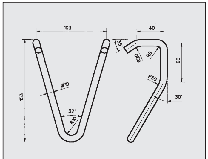
HONDA ACCORD ATTACCO per posteriore COD. AT 280102
