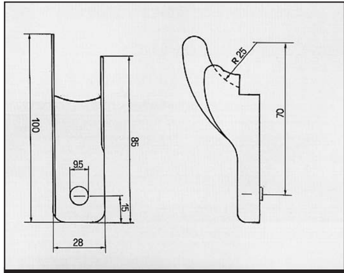
104 ATTACCO per posteriore COD. AT 540201 1724-66
