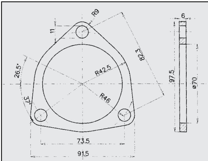
PEUGEOT 206 FLANGIA COD. FL 541209
