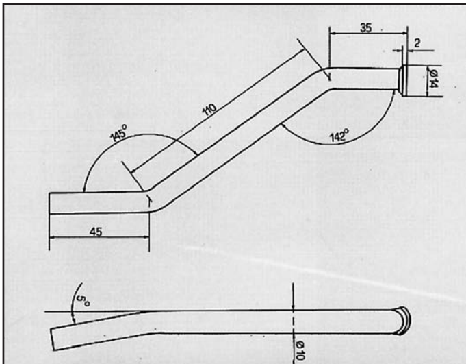
626 2000 16V ATTACCO anteriore sx per posteriore COD. AT 420518
