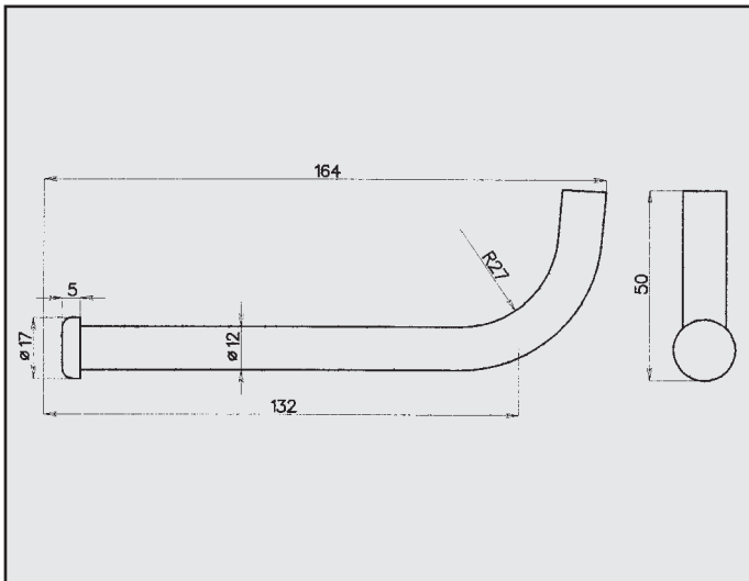
MERCEDES 380 SE ATTACCO COD. AT 440505
