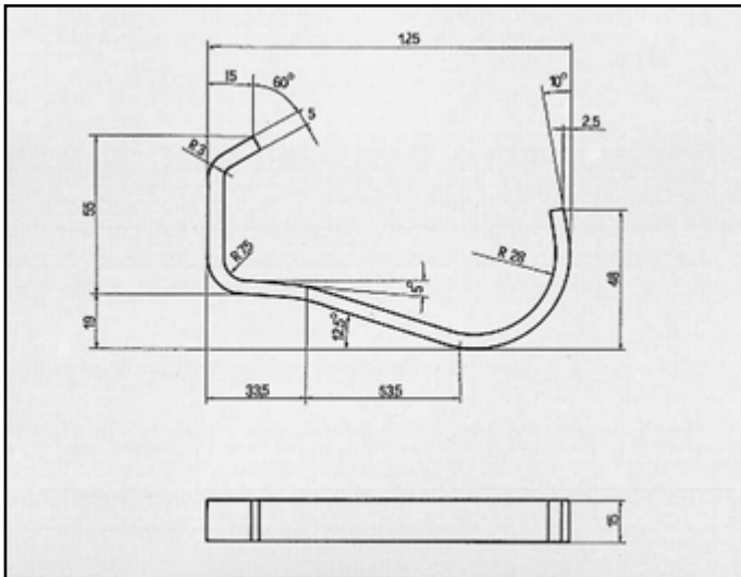
TIPO TURBO DIESEL ATTACCO per posteriore COD. AT 241708 7610385
