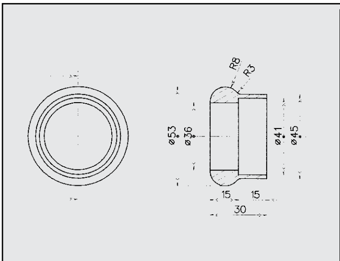
RENAULT TW TWINGO ANELLO COD. AN 601205
