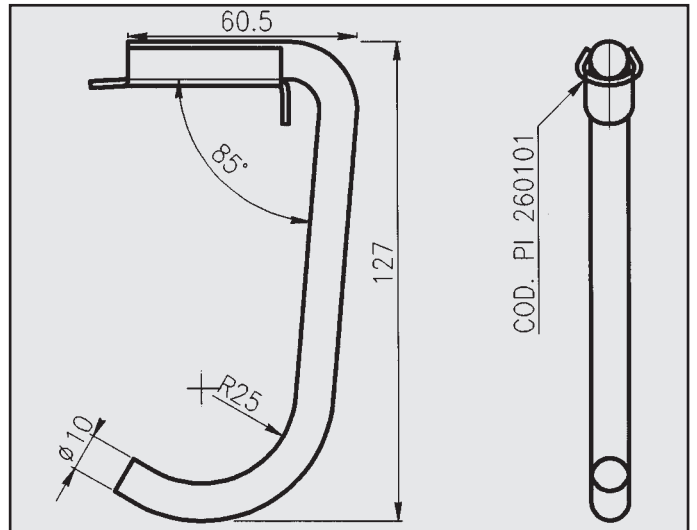
FORD FIESTA 1.6 '92 1.6 GT 16V '94 ATTACCO per posteriore COD. AT 260347
