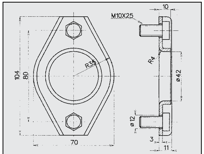
DAEWOO MATIZ - TICO FLANGIA CENTRALE COD. FL 160107
