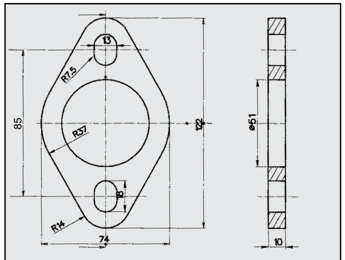
KIA FLANGIA COD. FL 310103
