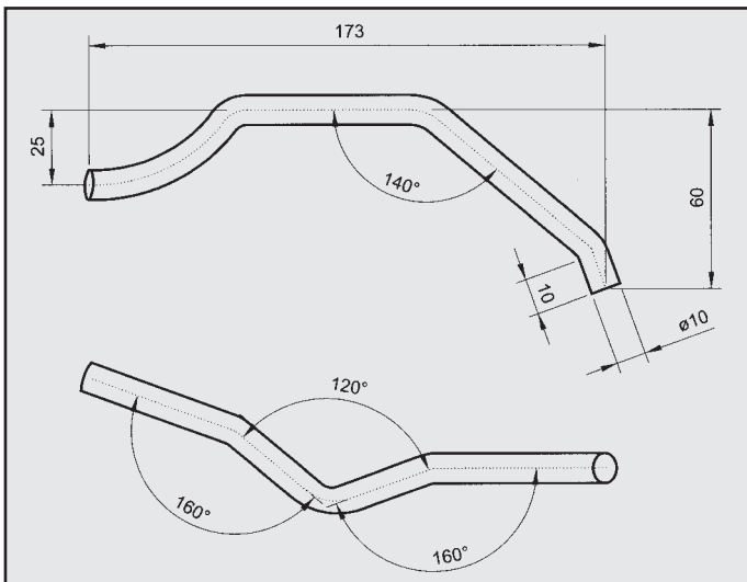
NISSAN MICRA ATTACCO per posteriore COD. AT 500206
