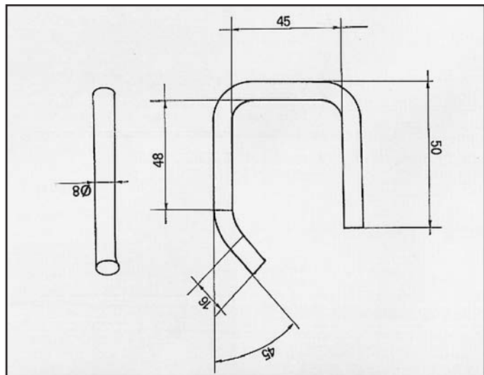
HORIZON ATTACCO per posteriore COD. AT 780203 0059114807 0059129407
