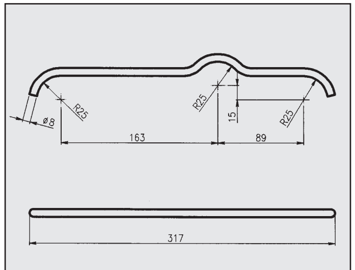
RENAULT 19 1.4 RINFORZO COD. R 600911
