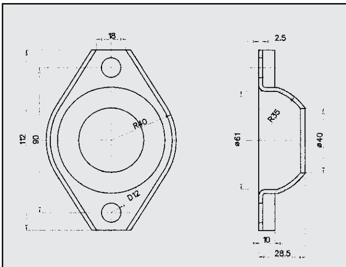
PEUGEOT 205 FLANGIA COD. FL 540320
