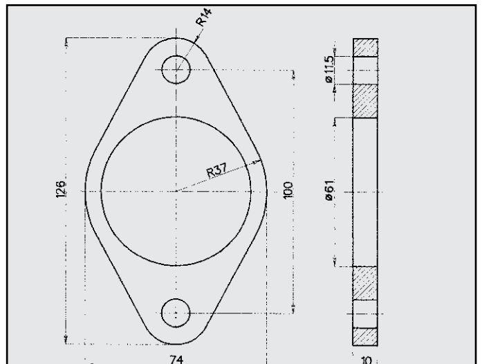
FORD FIESTA 1.2 S 16V FLANGIA COD. FL 260356
