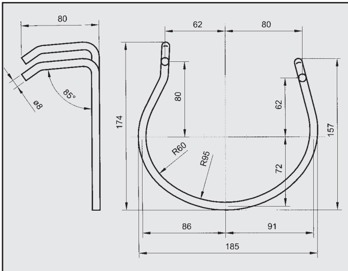
PEUGEOT 405 ATTACCO Tondino 8 (Sostituisce FASCETTA COD. F 540702) COD. AT 540703
