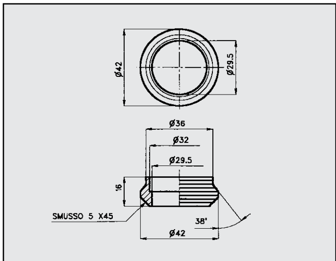
CITROEN DYANE 4 - 6 ANELLO ø esterno mm 42 ø interno mm 29,5 COD. AN 140801
