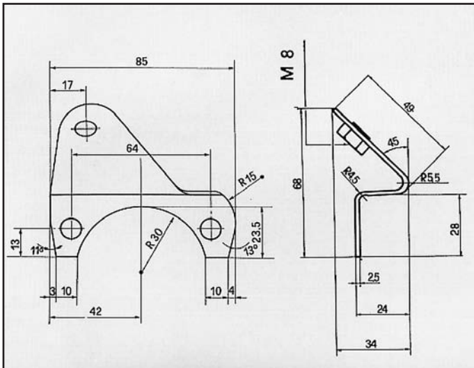
DELTA/PRISMA 1ª SERIE ATTACCO per posteriore COD. AT 380305
