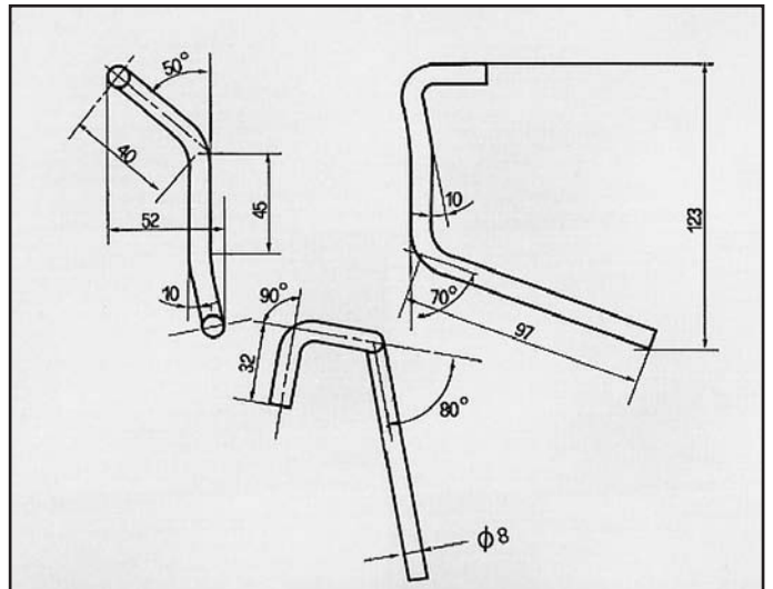
COROLLA 2ª SERIE ATTACCO per posteriore COD. AT 800403
