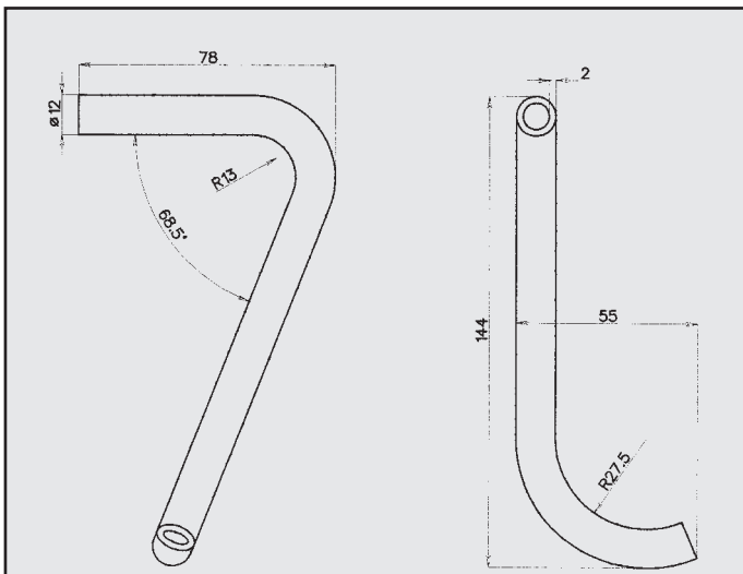
MERCEDES CLASSE C ATTACCO COD. AT 441002
