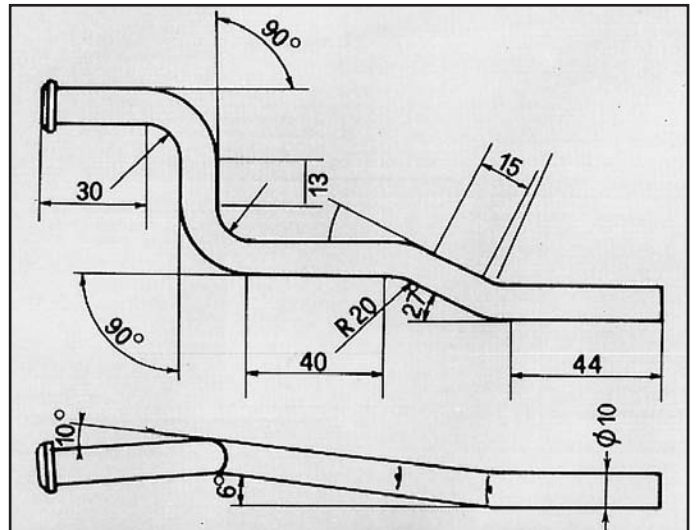
GLC 1500 ATTACCO per centrale COD. AT 420301
