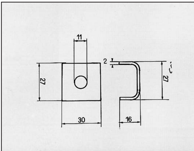
200 BENZINA E DIESEL DISTANZIALE tubo marmitta COD. AT 440205
