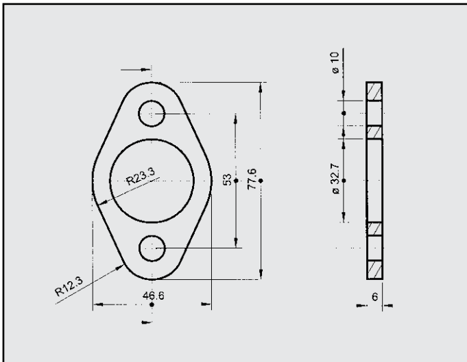
FIAT 126 FLANGIA COD. FL 240006
