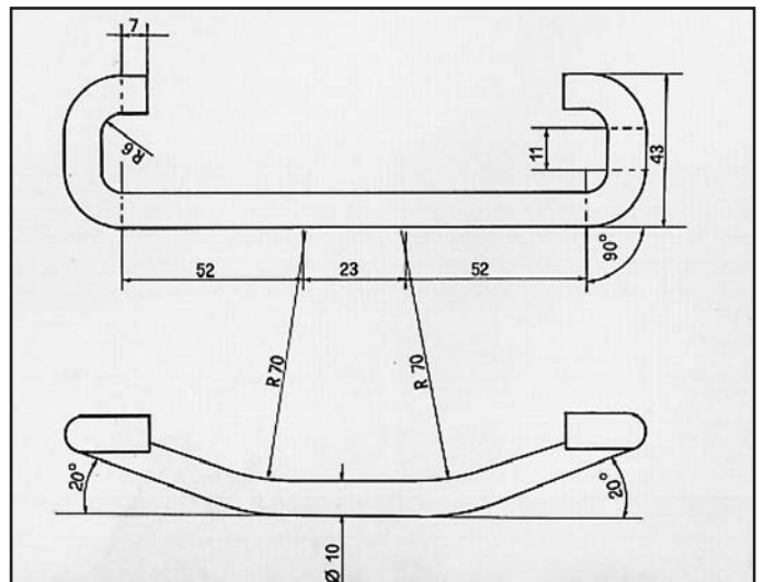
BALLADE SPORT CRX ATTACCO per centrale COD. AT 280305
