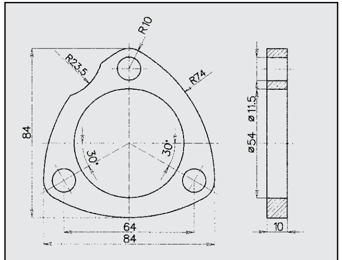
FIAT UNO GT 1.4 FLANGIA COD. FL 240010
