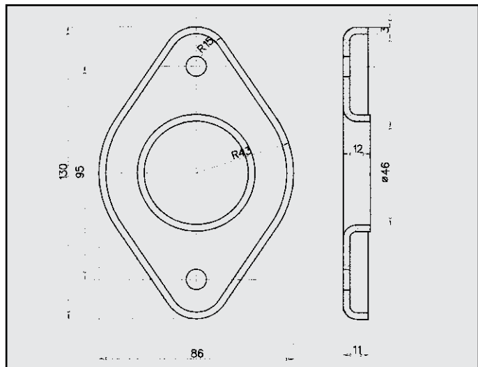
PEUGEOT 307 1.6-1.4 FLANGIA COD. FL 541302
