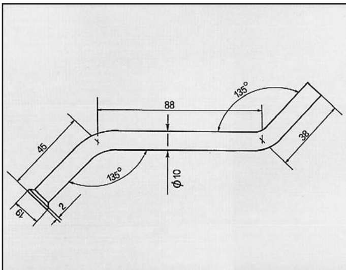
626 2000 16V ATTACCO sx per posteriore COD. AT 420513
