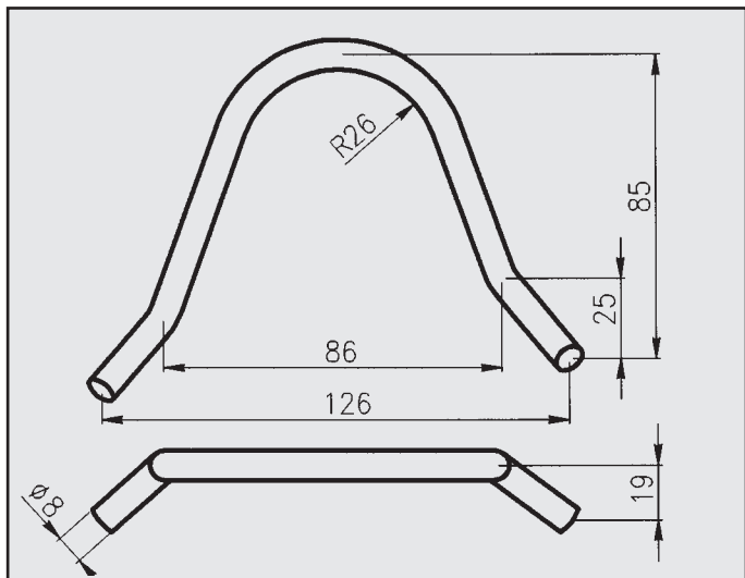
LANCIA DELTA RINFORZO COD. R 380342
