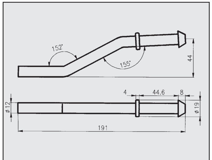
OPEL ASTRA ATTACCO per posteriore COD. AT 520921
