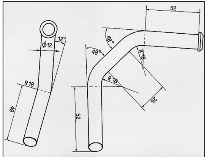
NEW MARK II ATTACCO per posteriore COD. AT 800601
