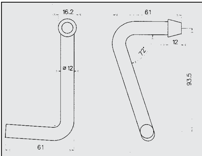
AUDI A4 1.6 1.8 ATTACCO COD. AT 040607
