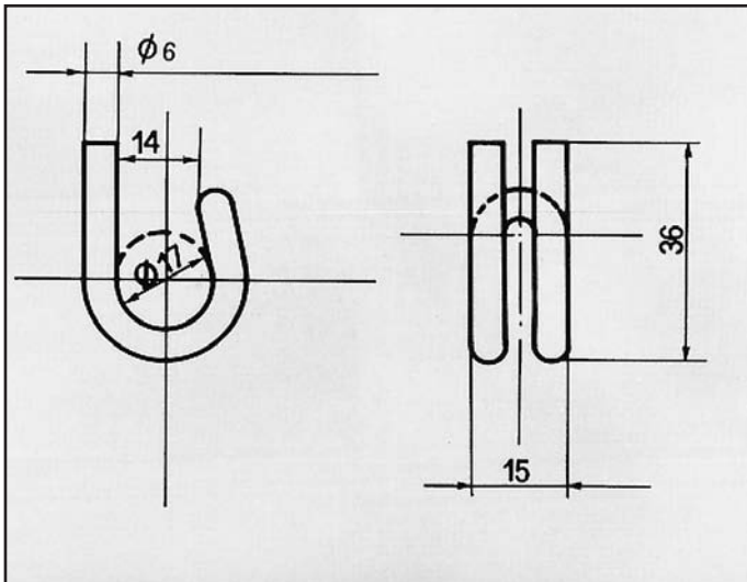
R20-R30 ATTACCO per posteriore COD. AT 600601
