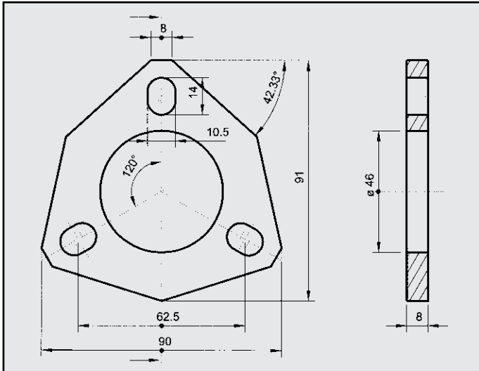
LANCIA DELTA PRISMA FLANGIA COD. FL 380341
