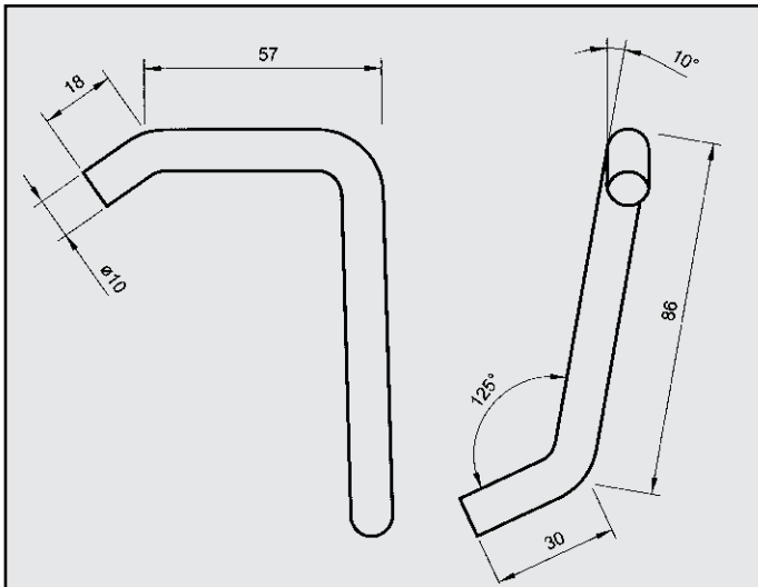
DAIHATSU FEROZA ATTACCO per posteriore COD. AT 180306
