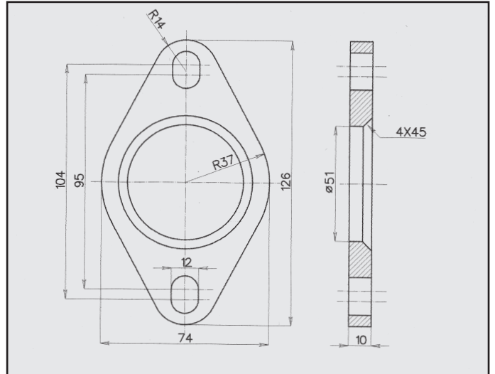
FORD ESCORT FLANGIA COD. FL 260278
