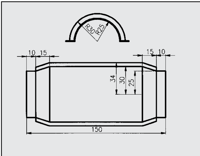
FIAT BRAVO 1.8 PROTEZIONE CALORE COD. PC 242314
