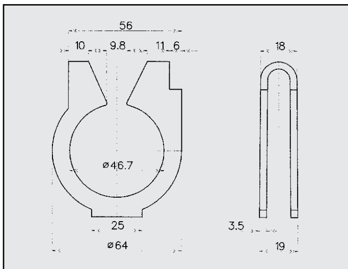
FIAT PUNTO 60 / PANDA NUOVA FASCETTA COD. F 242206
