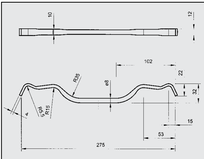
FIAT TIPO 1.4 1.6 ATTACCO per centrale COD. AT 241719
