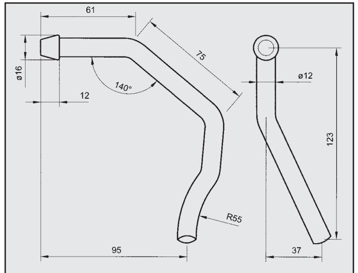
NISSAN PRIMERA 2.0 ATTACCO DX per posteriore COD. AT 500411
