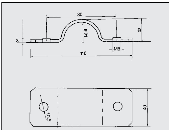
FIAT 127 FASCETTA per collettore COD. F 240202
