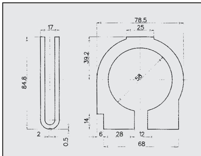
FIAT MAREA 1.6 FASCETTA COD. F 242817
