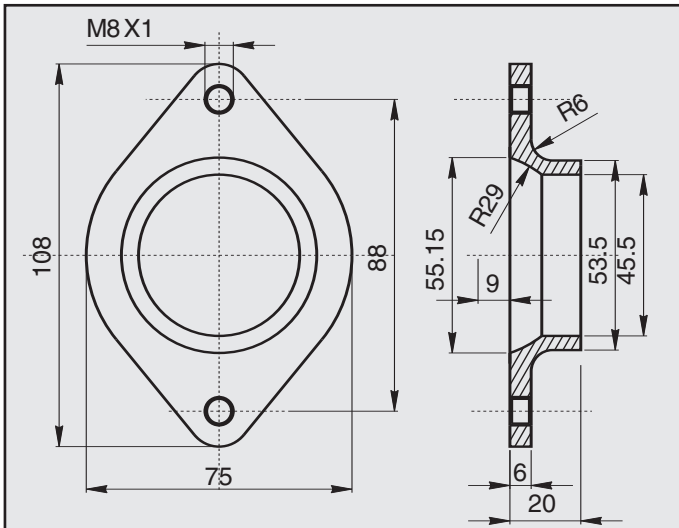
OPEL VECTRA - ASTRA 1.4 1.6 1.8 2.0 FLANGIA COD. FL 520827
