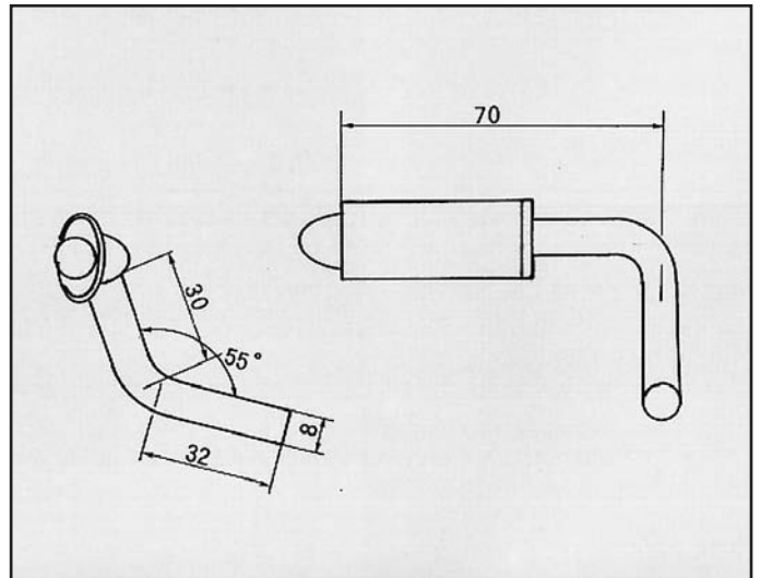
343/345 ATTACCO anteriore per posteriore COD. AT 880103
