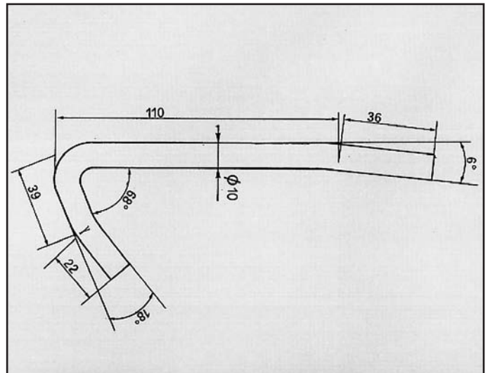
ACTY ATTACCO per posteriore COD. AT 280204
