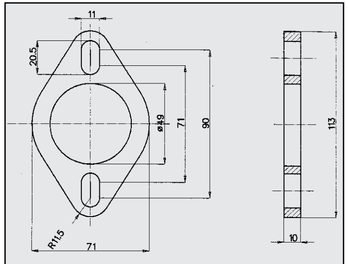
ROVER FLANGIA COD. FL 620004
