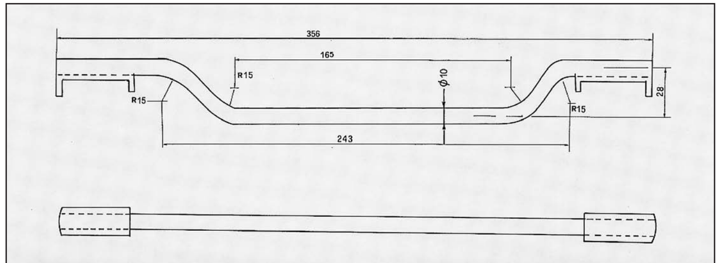
SCIROCCO 1800 ATTACCO per posteriore COD. AT 860115
