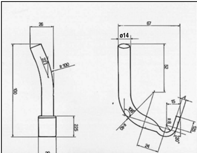
PANDA DIESEL ATTACCO centrale per marmitta posteriore COD. AT 240109
