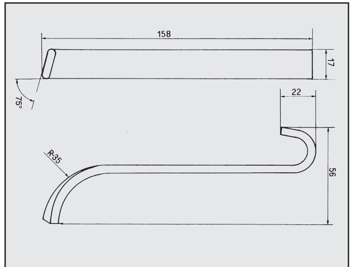
ALFA GTV 6 ATTACCO per centrale COD. AT 020602
