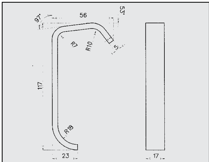
FIAT TIPO ATTACCO COD. AT 241714
