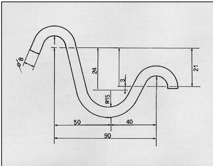
TERRA ATTACCO per posteriore COD. AT 680402
