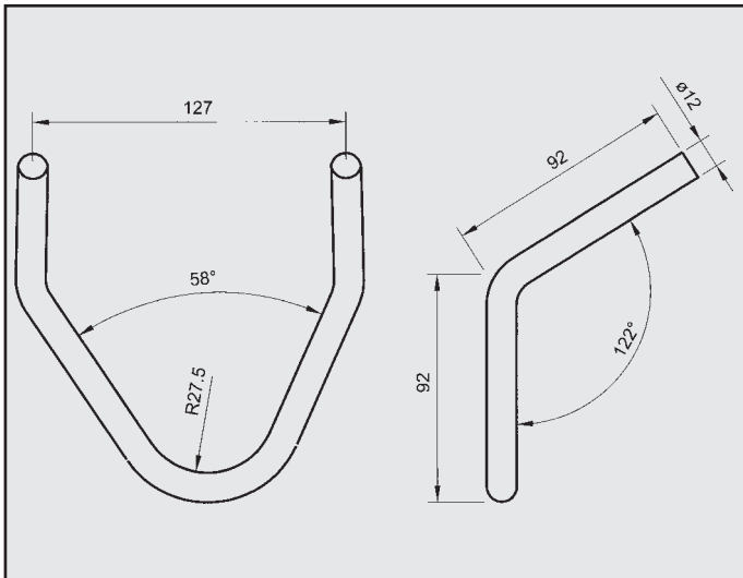
OPEL OMEGA 2.0 I.E. 16V ATTACCO per posteriore COD. AT 520611
