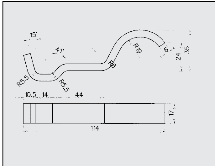
FIAT TIPO 1.1 ATTACCO per posteriore COD. AT 241720
