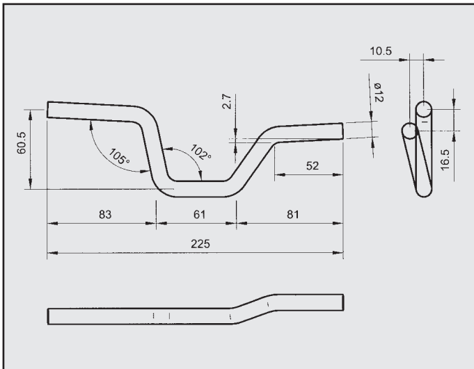
OPEL OMEGA 2.0 ATTACCO per centrale COD. AT 520612
