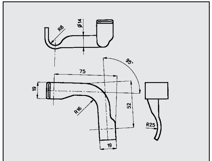
Y10 TURBO ATTACCO per tubo centrale COD. AT 080212 7538229
