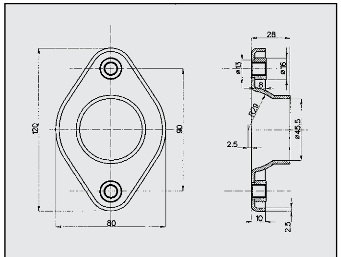
TOYOTA FLANGIA COD. FL 800004
