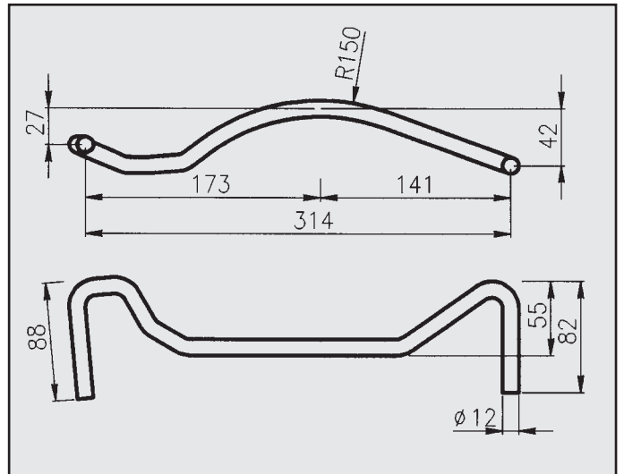
OPEL ASTRA 1.4 ATTACCO per posteriore COD. AT 520912
