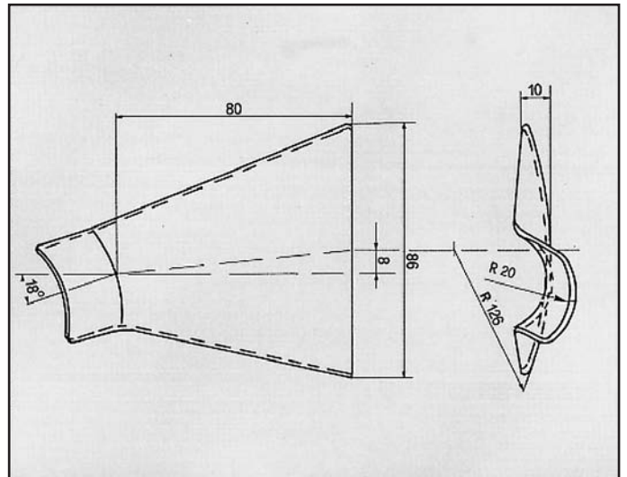
MINI 2 CILINDRI RINFORZO COD. R 320104
