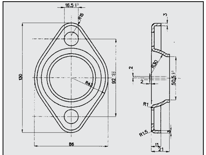
HONDA CIVIC FLANGIA COD. FL 280428
