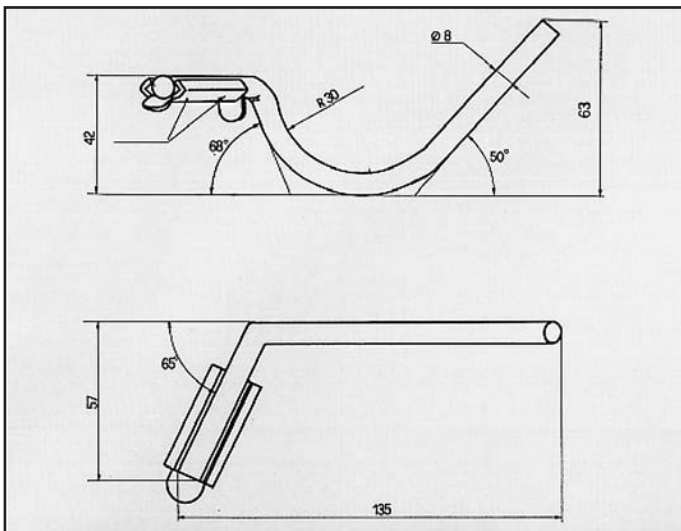
ESCORT 1600/ORION 1600 ATTACCO per centrale COD. AT 260222
