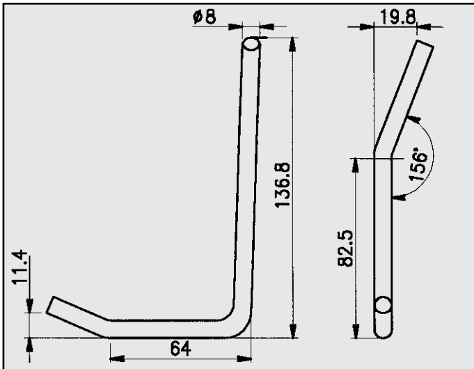
FIAT TIPO ATTACCO per posteriore COD. AT 241724
