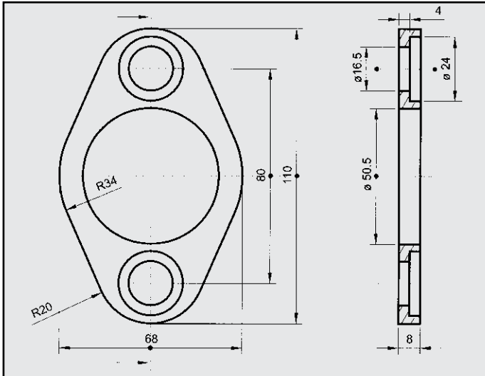
AUTOBIANCHI Y10 1.1 I.E. FLANGIA COD. FL 080219
