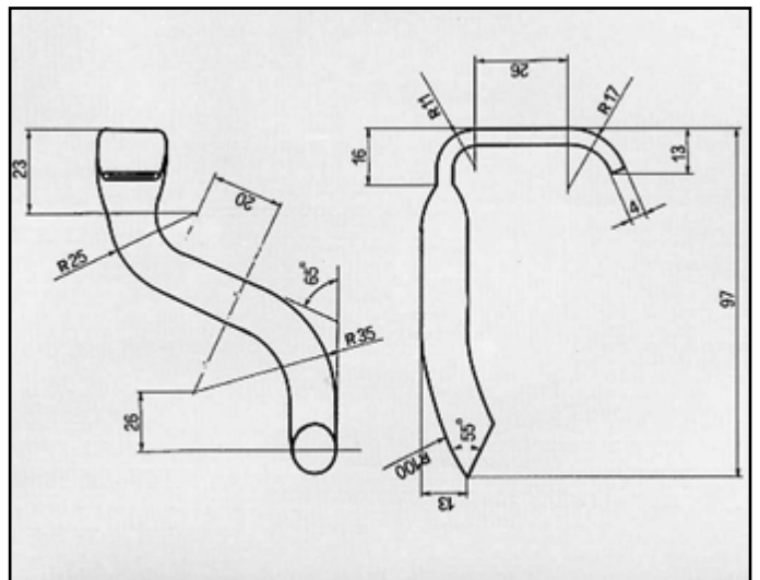
UNO SX ATTACCO per posteriore COD. AT 240905
