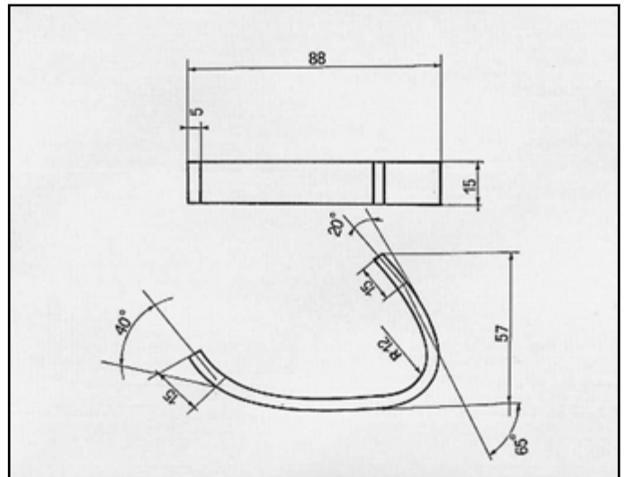
RITMO 1ª SERIE ATTACCO per posteriore COD. AT 240802
