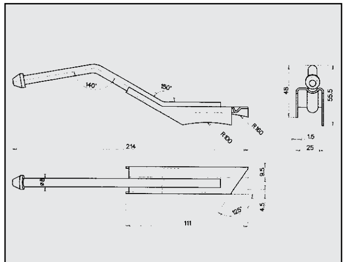
FIAT PUNTO ATTACCO COD. AT 242242
