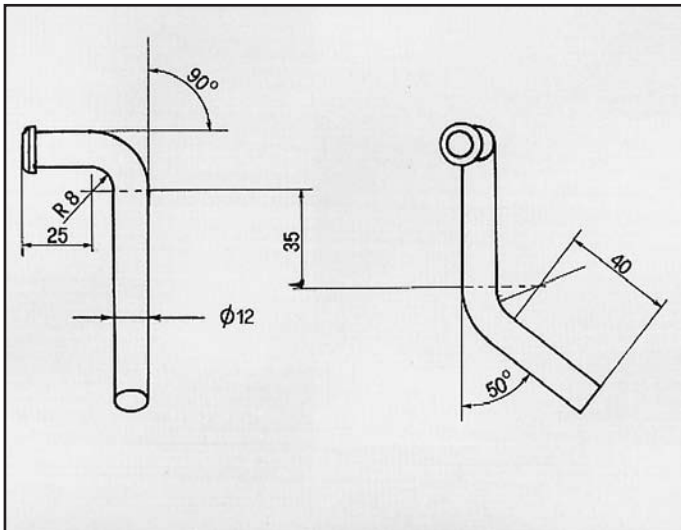
CELICA ATTACCO per posteriore COD. AT 800201
