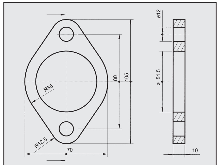
OPEL ASTRA FLANGIA COD. FL 520904
