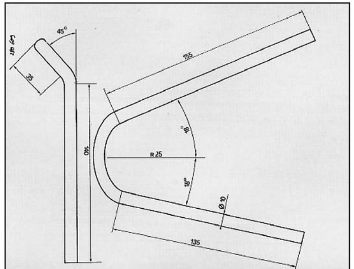
PRELUDE 4WS RINFORZO per posteriore COD. R 280609
