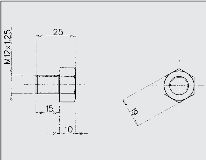
FIAT PUNTO 1.2 / FIORINO 1.4 - 1.6 VITE COD. VI 242236
