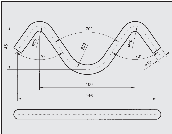
OPEL CALIBRA 2.0 i 16V ATTACCO per posteriore COD. AT 521003
