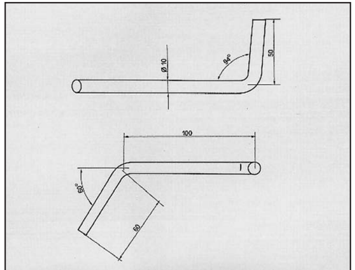
PRELUDE 4WS RINFORZO per posteriore COD. R 280608
