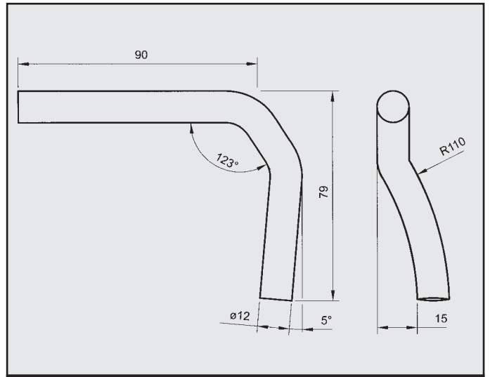
OPEL ASTRA ATTACCO per posteriore COD. AT 520906
