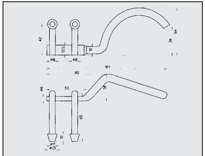
FIAT PUNTO 1.2 ATTACCO COD. AT 242225
