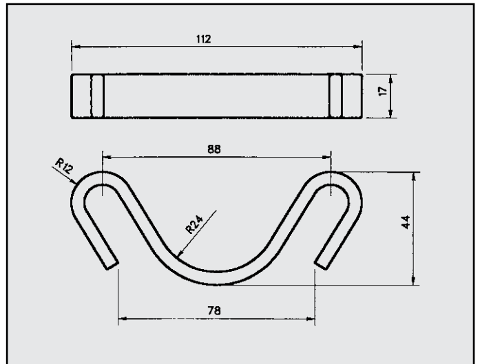
FIAT DUCATO ATTACCO per centrale COD. AT 241501
