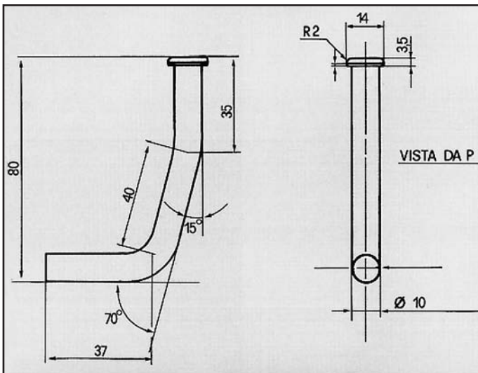
COROLLA 2ª SERIE ATTACCO anteriore per posteriore COD. AT 800402
