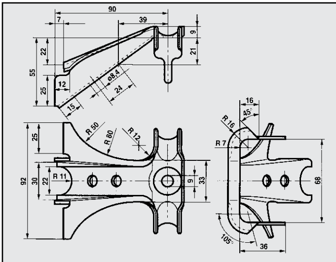
AUDI 100/2000 E 10/91 - 2500 10/91 ATTACCO posteriore COD. AT 040104 4 AO 253609E 4 AO 253609H
