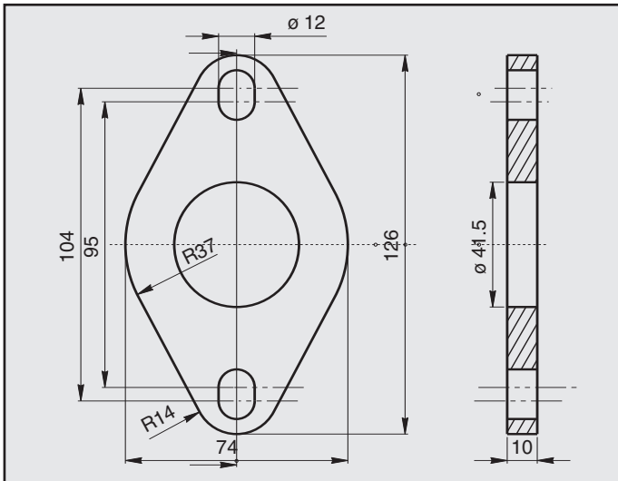
NISSAN MICRA FLANGIA COD. FL 500210
