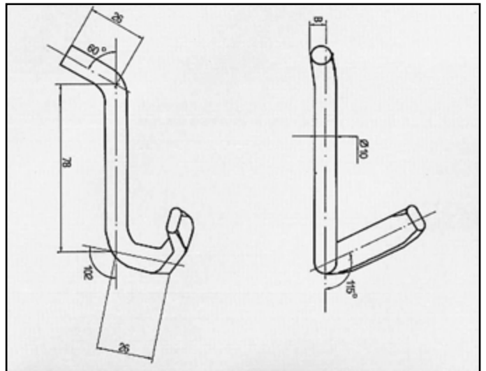
UNO 60 ATTACCO per posteriore COD. AT 240904
