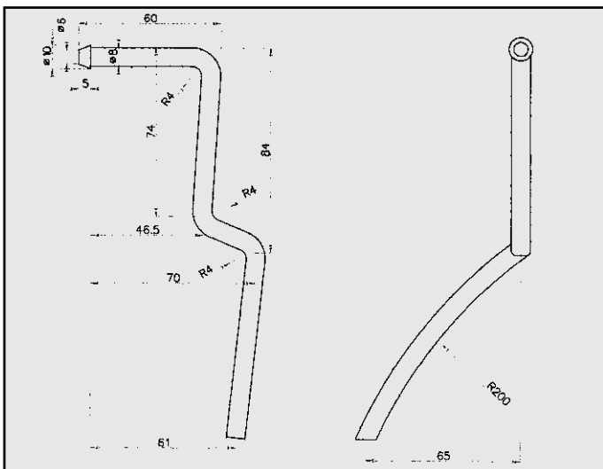
FIAT PUNTO 1.2 ATTACCO COD. AT 242230
