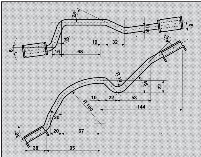
CITROEN ZX 1.4 REFLEX 03/91 1.6 CATALIZZATA ATTACCO posteriore COD. AT 140902 96041796 96041798
