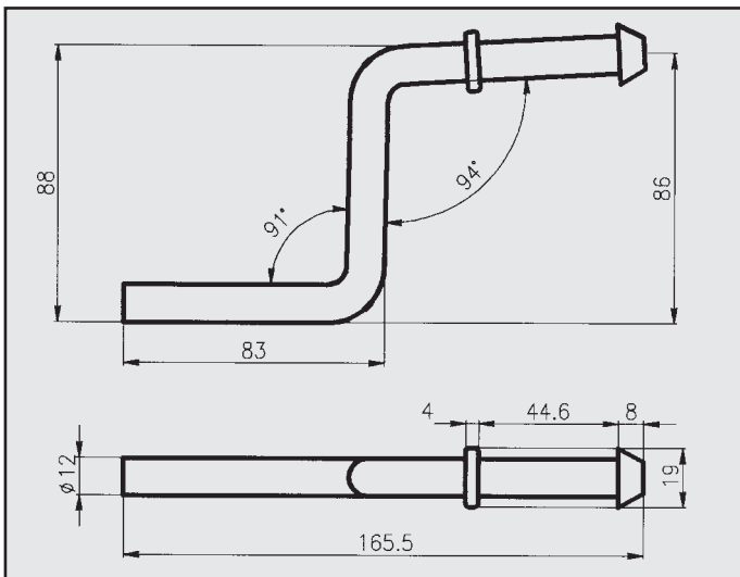
OPEL ASTRA ATTACCO per posteriore COD. AT 520924
