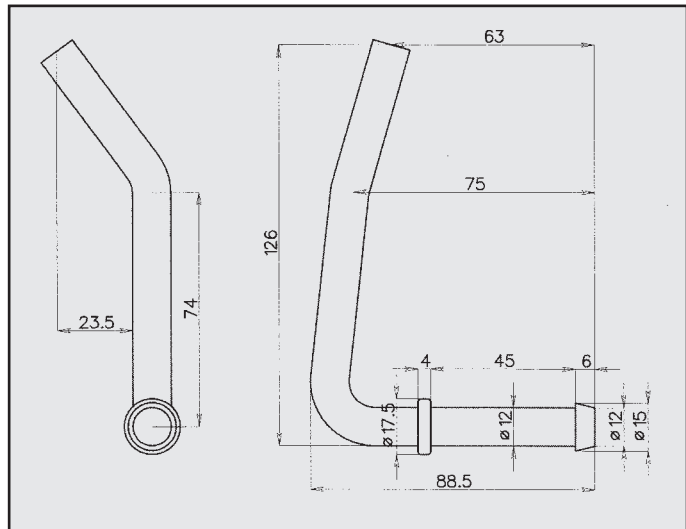
LANCIA LYBRA ATTACCO COD. AT 381102
