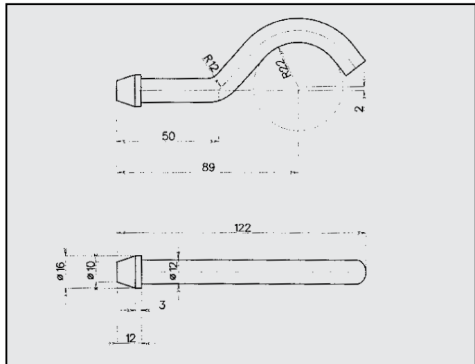
DAEWOO NUBIRA 1.6 ATTACCO POSTERIORE COD. AT 160305
