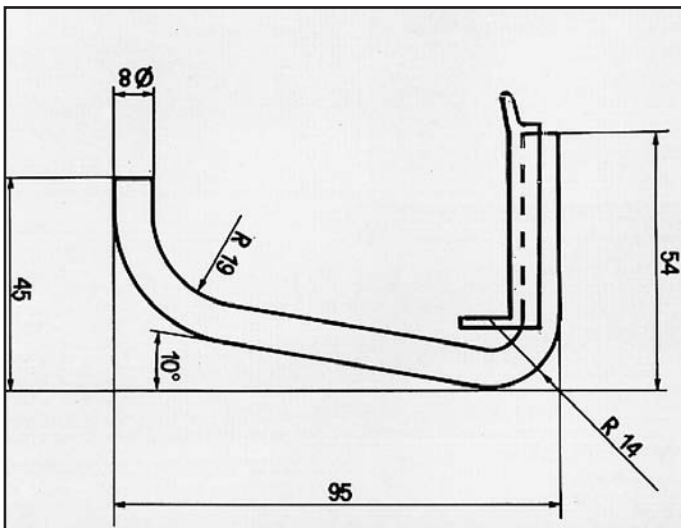
CORSA ATTACCO per posteriore COD. AT 520301
