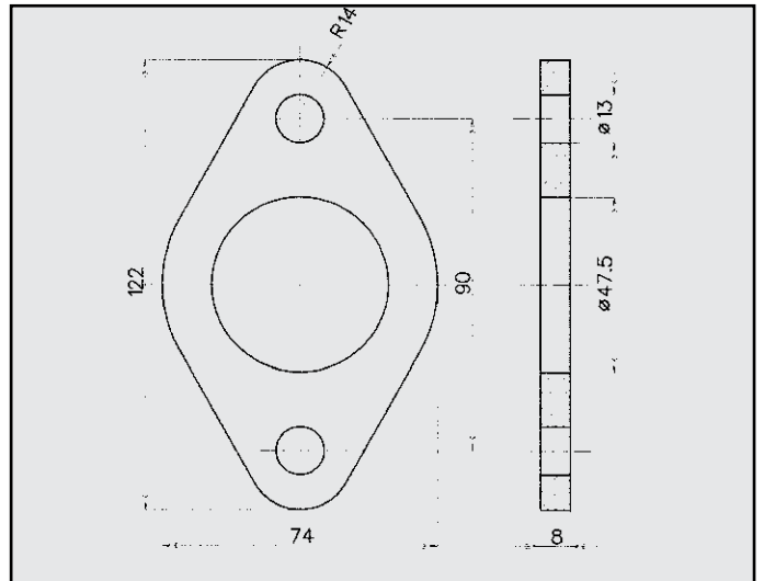
SUBARU 1.3-1.6 FLANGIA COD. FL 700001
