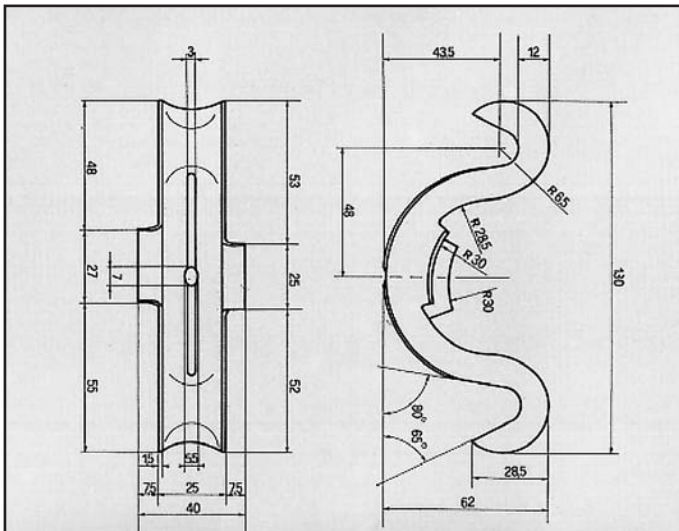
ASCONA 1300 ATTACCO per centrale COD. AT 520202
