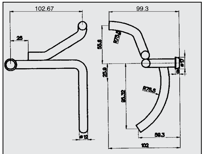
AUDI A4 ATTACCO COD. AT 040604
