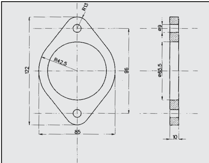
RENAULT PEUGEOT FLANGIA COD. FL 600002
