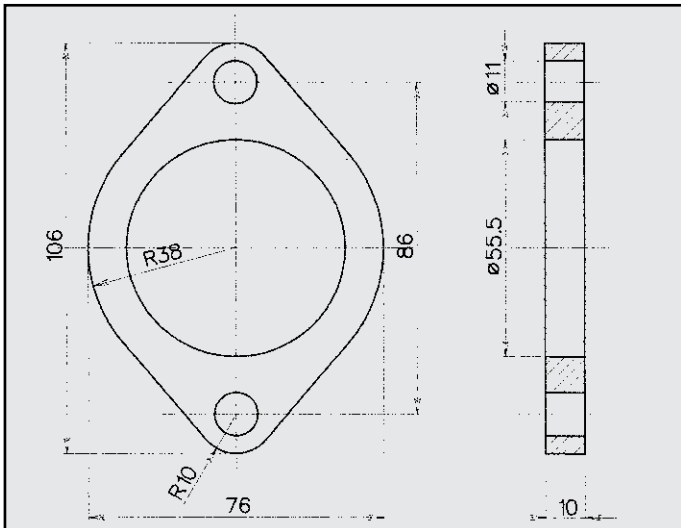
OPEL FRONTERA FLANGIA COD. FL 521402
