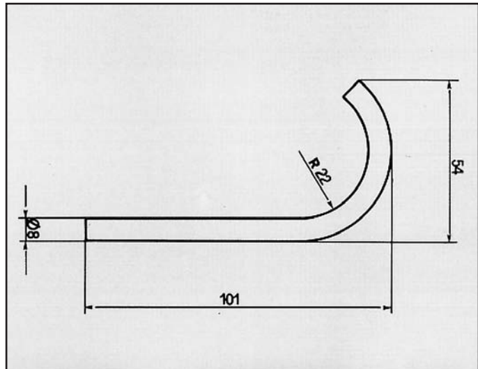
ESCORT 1100/1300/82 RINFORZO per centrale COD. R 260202 6104207 6128785
