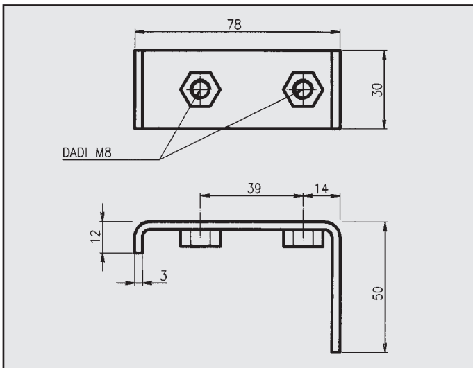
SUZUKI SJ 413 1.3 4X4 ATTACCO per centrale COD. AT 720308
