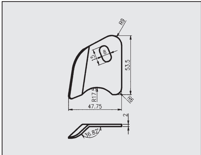
LIGIER ATTACCO collettore COD. AT 390004
