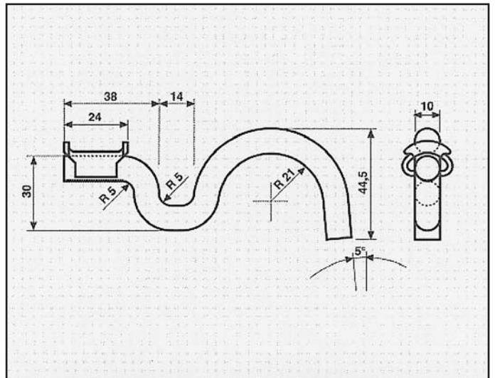
PEUGEOT 450 ATTACCO centrale COD. AT 540702
