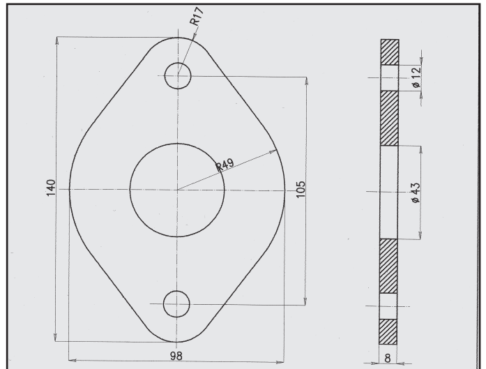
NISSAN PRIMIERA 1.6 16V FLANGIA COD. FL 500417
