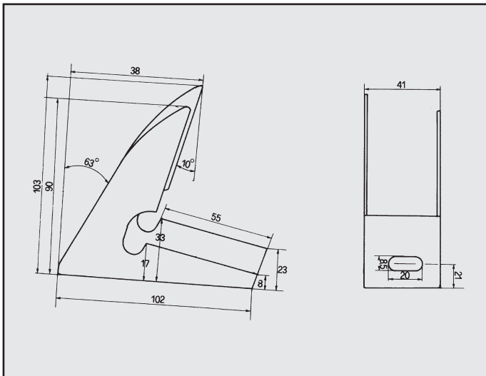
GIULIA ATTACCO per centrale COD. AT 020402
