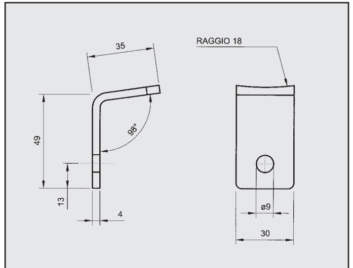
SUZUKI VITARA 1.6 ATTACCO per centrale COD. AT 720112
