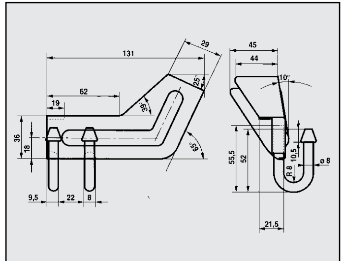
FIAT PUNTO 60/GT ATTACCO posteriore COD. AT 242203
