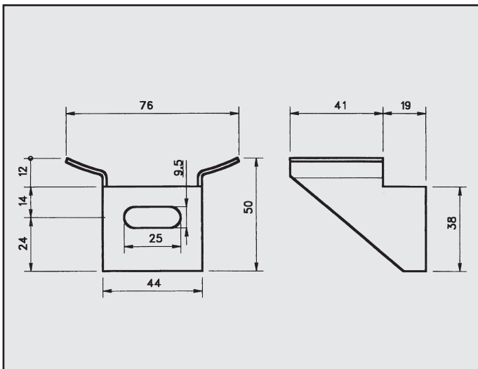
GIULIA 1300-1600 ATTACCO per posteriore COD. AT 020403
