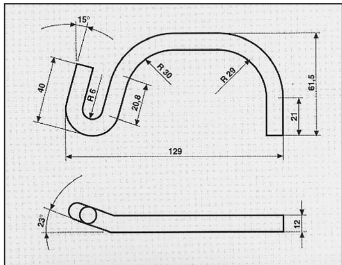
LANCIA THEMA 2000 TURBO I.E. CAT. ATTACCO centrale COD. AT 380709
