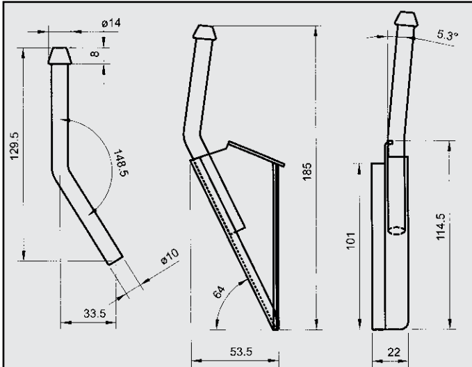
FIAT BRAVO 1.4 ATTACCO per centrale COD. AT 242301
