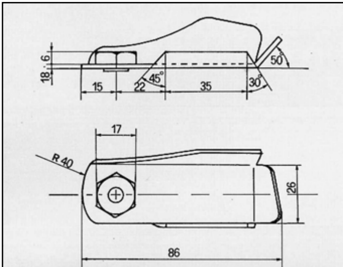
131 ATTACCO per posteriore COD. AT 240604
