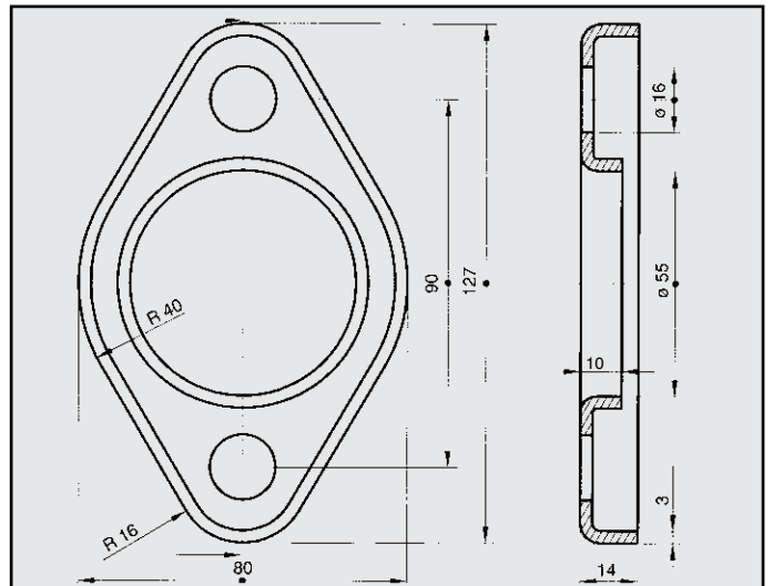
FORD ESCORT FLANGIA COD. FL 260266
