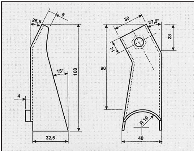
SUZUKI VITARA ATTACCO collettore marmitta COD. AT 720102
