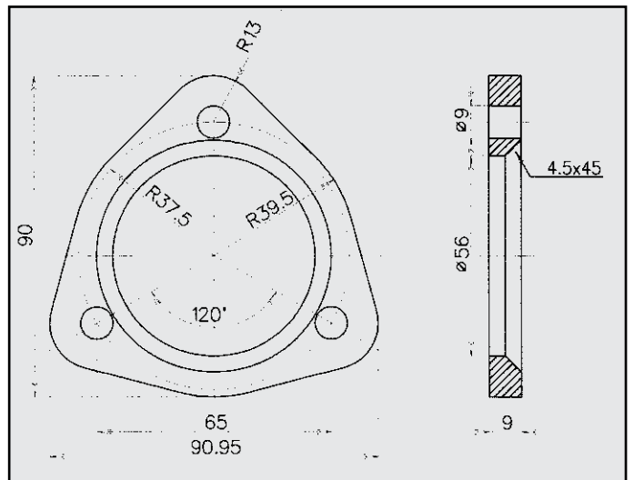
ALFA ROMEO GIULIA DUETTO FLANGIA COD. FL 020405
