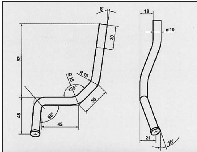
MAZDA 323 / 1986-87 ATTACCO per posteriore COD. AT 420605 E 5254100 B/C/F
