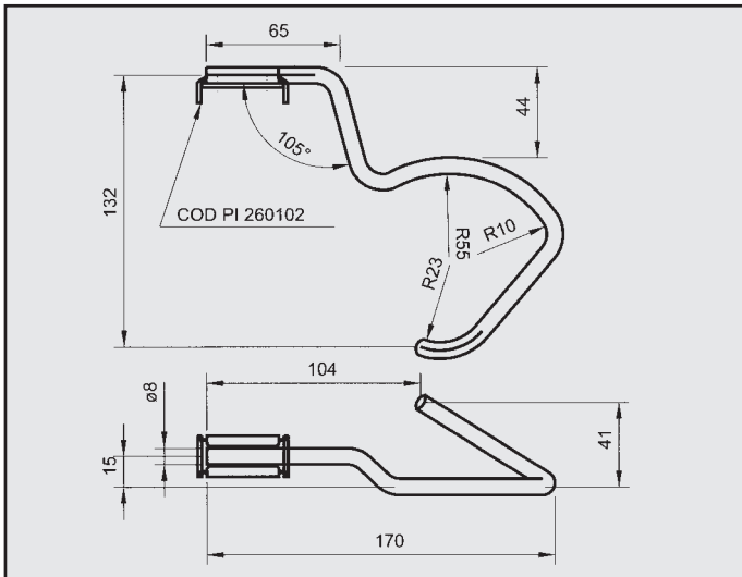
FORD COURIER ATTACCO per centrale COD. AT 261301
