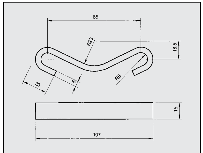
FIAT UNO CS DUNA 60 ATTACCO COD. AT 240921
