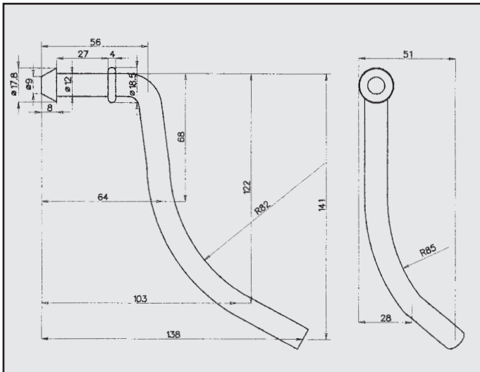
LANCIA KAPPA 2.0 ATTACCO COD. AT 380908
