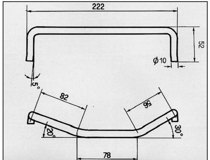
ACCORD 1600 ATTACCO per posteriore COD. AT 280106
