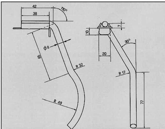
ASCONA 1800 ATTACCO per posteriore COD. AT 520203
