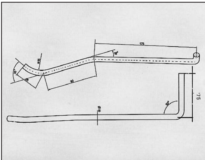
CIVIC RINFORZO COD. R. 280416
