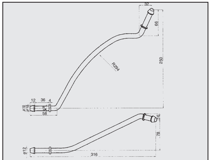
LANCIA K 2.0 20V ATTACCO COD. AT 380911
