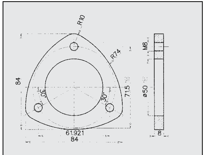
VOLKSWAGEN FLANGIA COD. FL 860025
