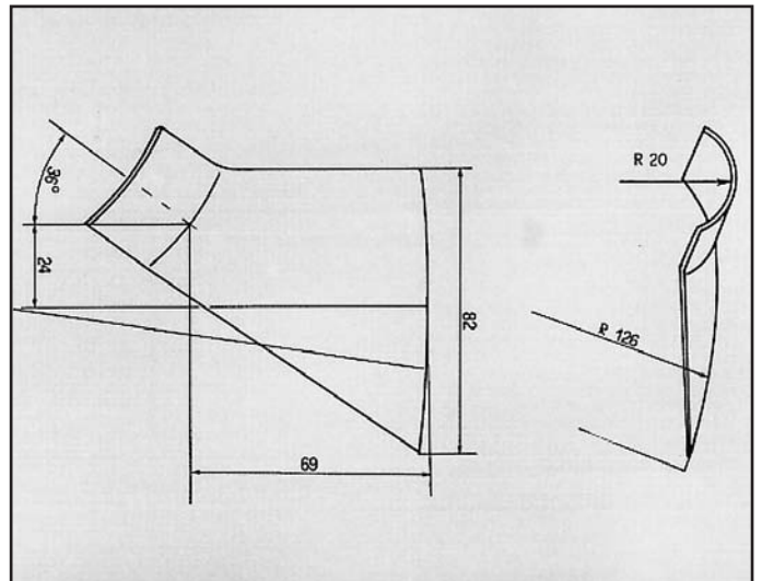
MINI 3 CILINDRI RINFORZO COD. R 320105
