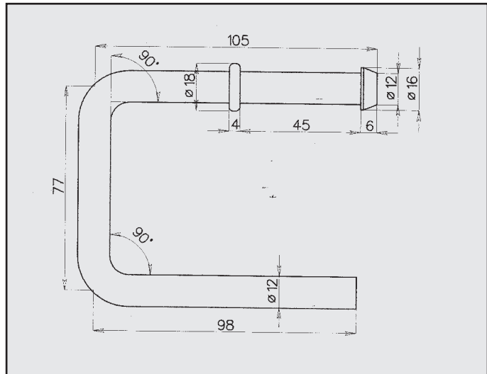
LANCIA LYBRA ATTACCO COD. AT 381101
