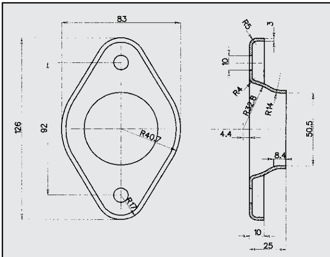
BMW FLANGIA COD. FL 120018
