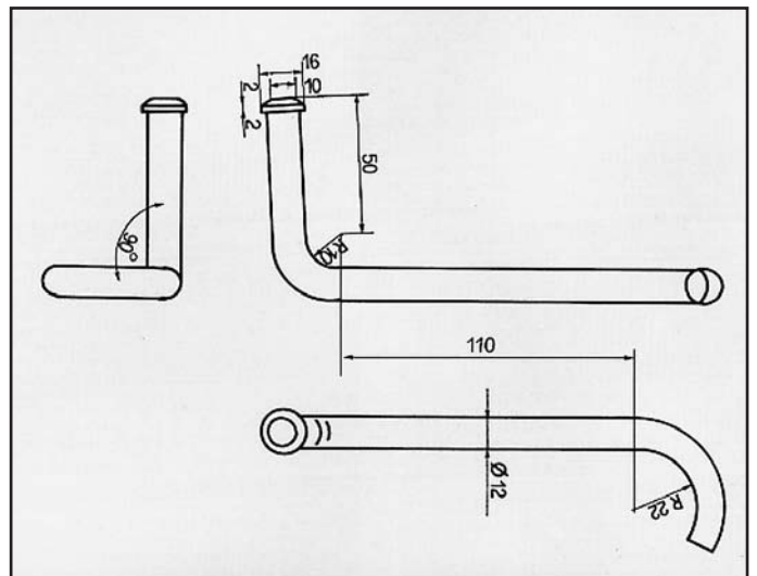
STARLET ATTACCO per centrale COD. AT 800801
