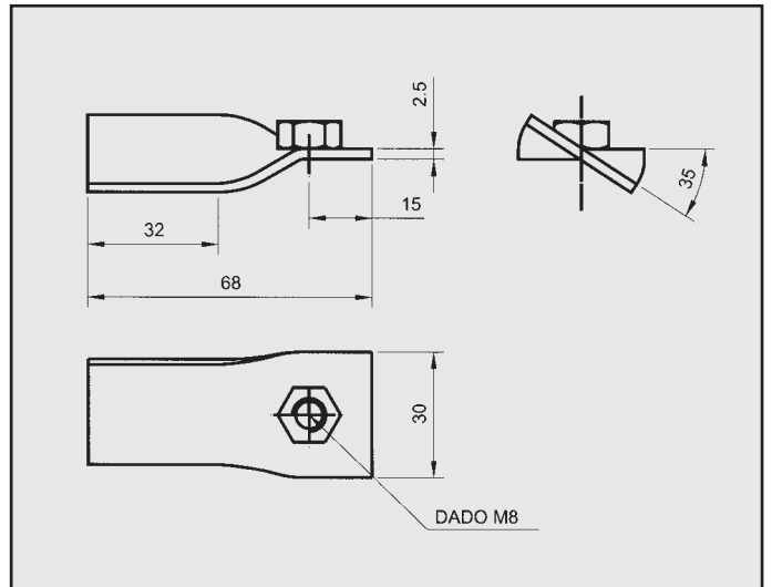
SUZUKI MARUTI ALTO 800 ATTACCO per posteriore COD. AT 720401
