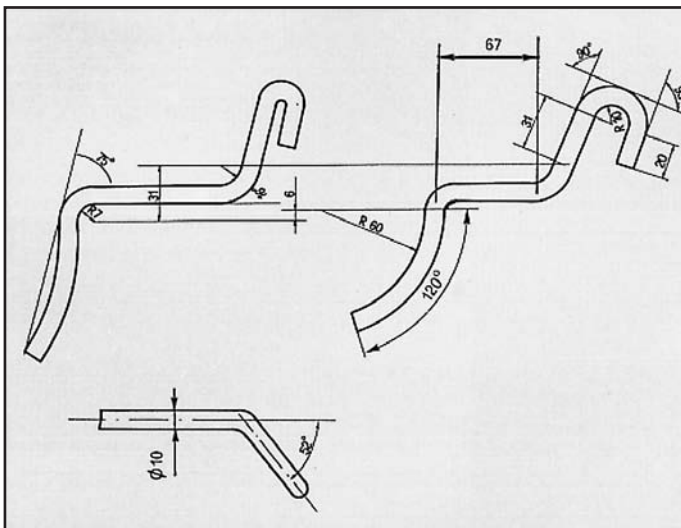
626 ATTACCO per silenziatore COD. AT 420507
