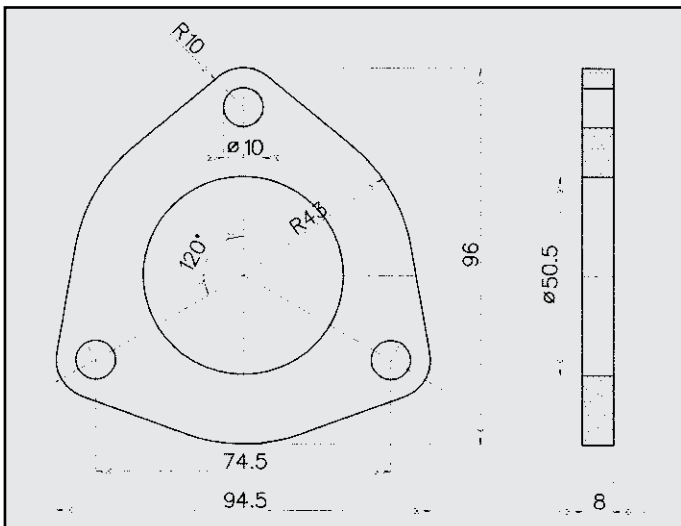
CENTRALE OMEGA FLANGIA COD. FL 520618
