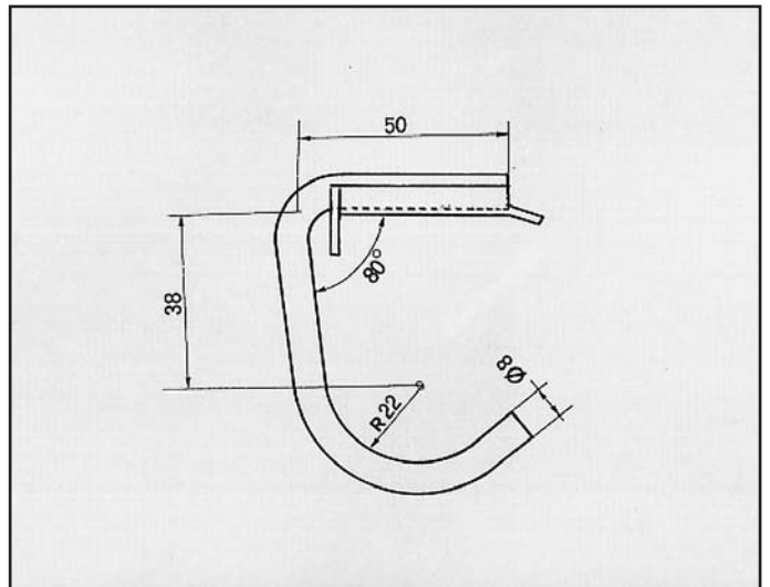
KADETT ATTACCO per posteriore COD. AT 520106
