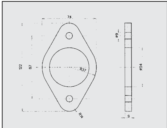
CLIO 1.2/1.4 FLANGIA CENTRALE COD. FL 601312
