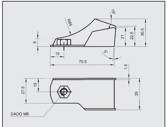
MITSUBISHI PAJERO 2.5 TD ATTACCO per posteriore COD. AT 460204
