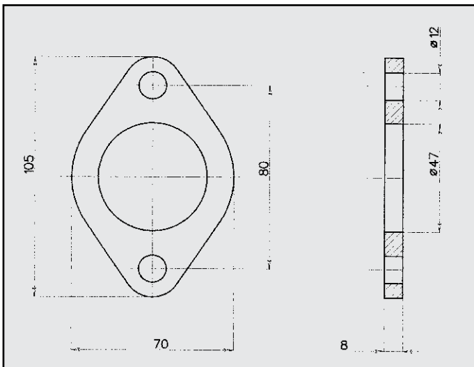
DAIHATSU CUORE 0.8 FLANGIA COD. FL 180401
