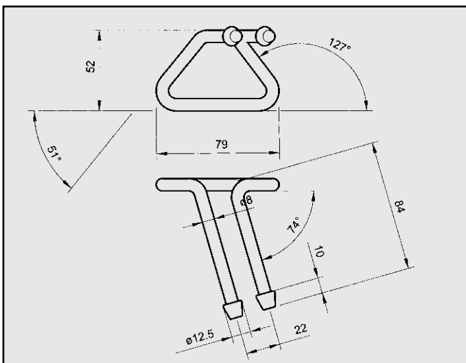
FIAT BRAVO 2.0 ATTACCO per posteriore COD. AT 242308
