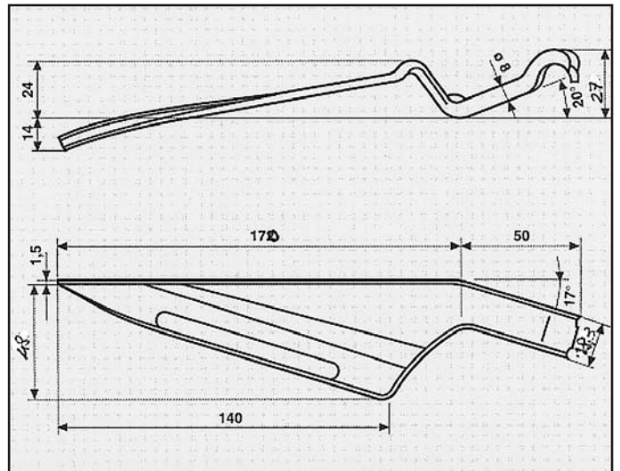
LANCIA DEDRA 1.8/2.0 i.e. T e TD ATTACCO centrale COD. AT 380803
