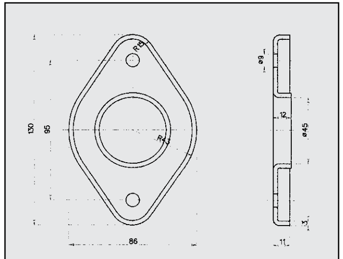
PEUGEOT 206 FLANGIA COD. FL 541206
