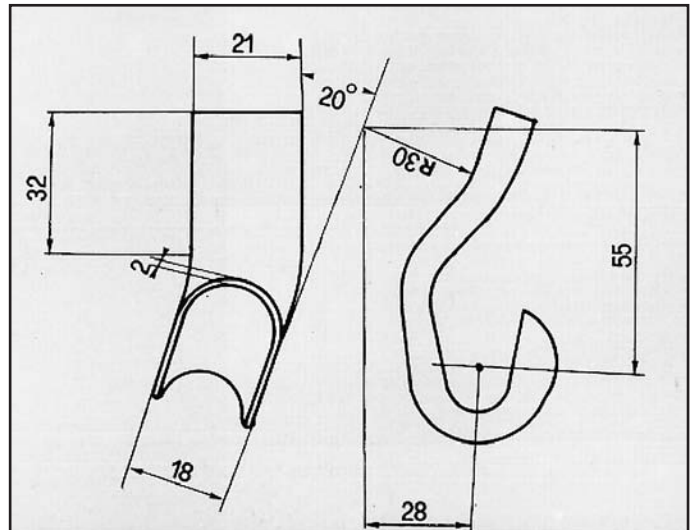
THEMA 2000 IE ATTACCO per centrale COD. AT 380701
