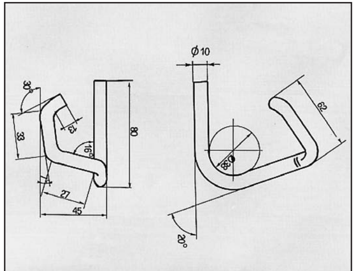
CIVIC ATTACCO per posteriore COD. AT 280404
