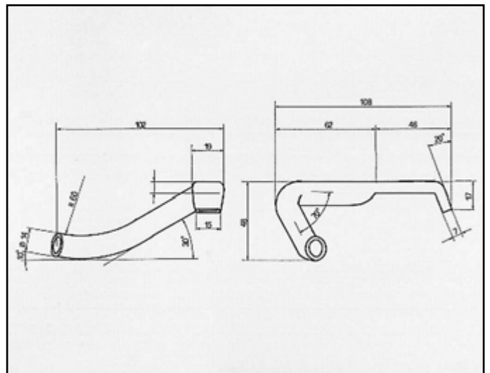
REGATA 2ª SERIE DIESEL 1700/85 SUPER ATTACCO per centrale COD. AT 241109
