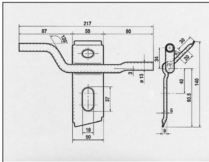
OPEL OMEGA 2000 E Berl. e Caravan/1987 ATTACCO per centrale COD. AT 520608
