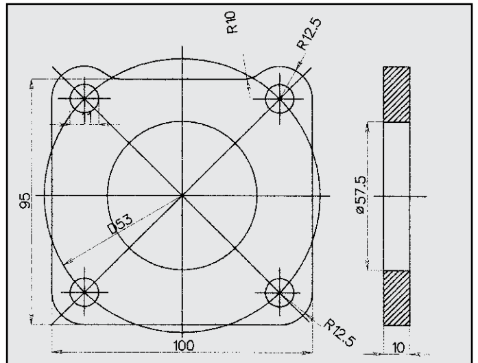
VOLKSWAGEN FLANGIA COD. FL 860030
