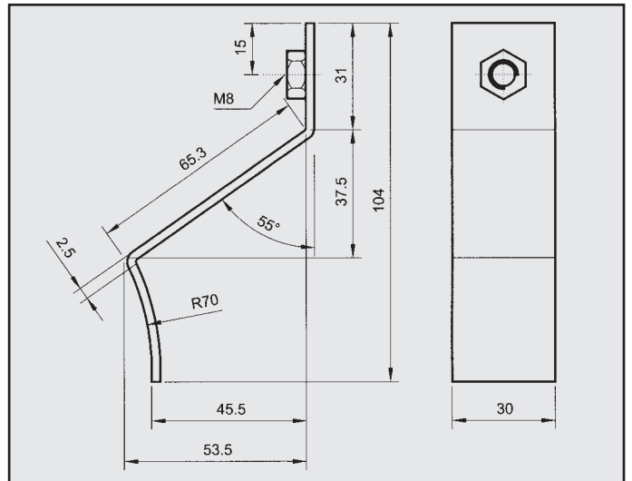
NISSAN MICRA ATTACCO per posteriore COD. AT 500207
