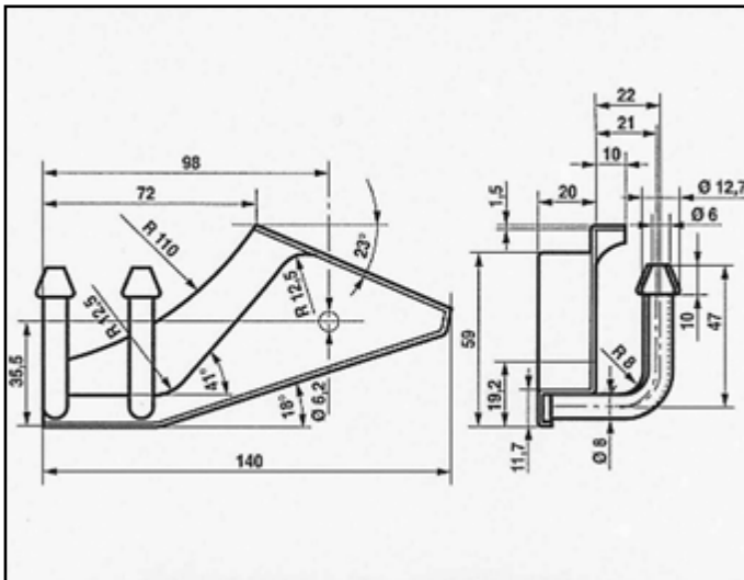
FIAT PUNTO 55 ATTACCO posteriore COD. AT 242201
