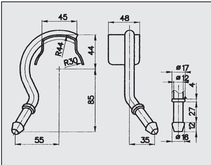
LANCIA K 2.0 ATTACCO per centrale COD. AT 380904
