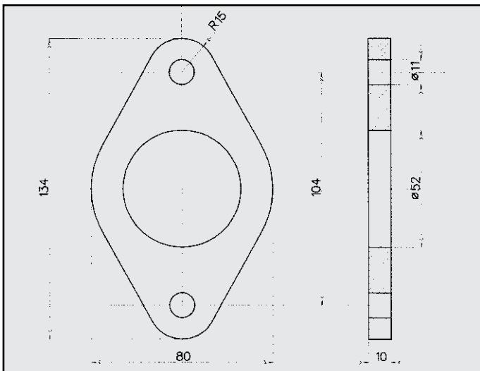
FIAT PUNTO FLANGIA COD. FL 242234
