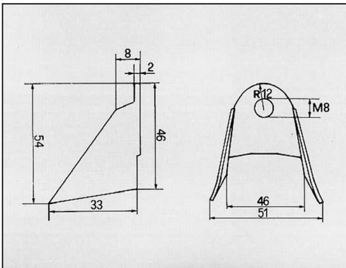
DELTA/PRISMA/PRISMA T.D. ATTACCO per collettore COD. AT 380311
