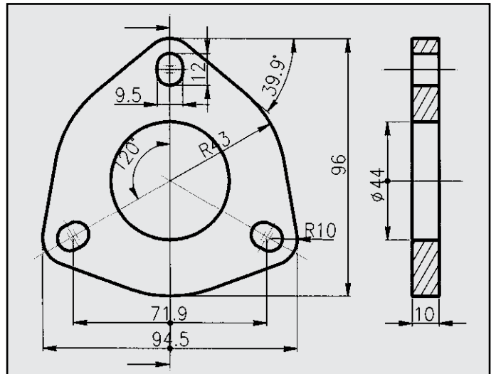
SKODA FAVORITE Catalizzata FLANGIA COD. FL 690104
