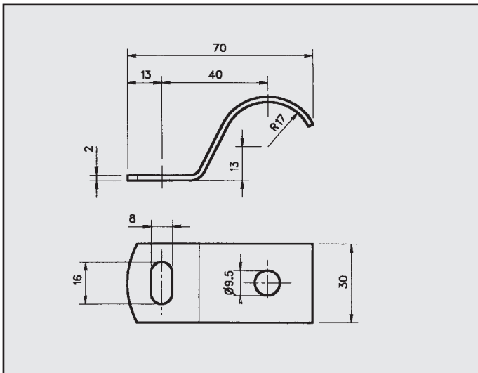
RENAULT R5 ATTACCO per tubo centrale COD. AT 600110
