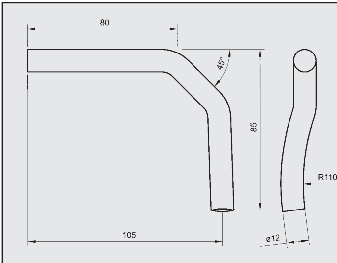
OPEL ASTRA 1.4 1.6 16V ATTACCO per posteriore COD. AT 520910
