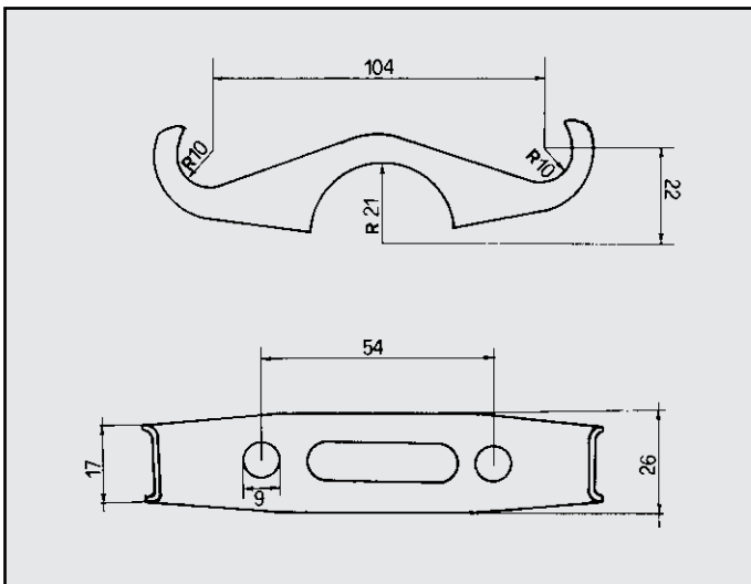
ALFASUD ATTACCO per centrale COD. AT 020103
