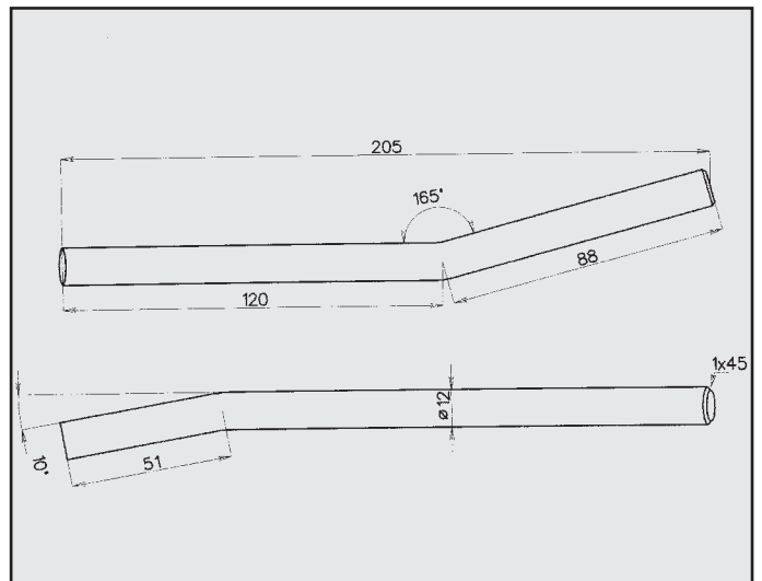
OPEL ZAFIRA ATTACCO per posteriore COD. AT 521302
