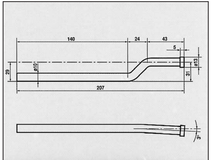
MAZDA MIATA MX5 ATTACCO per posteriore COD. AT 420801
