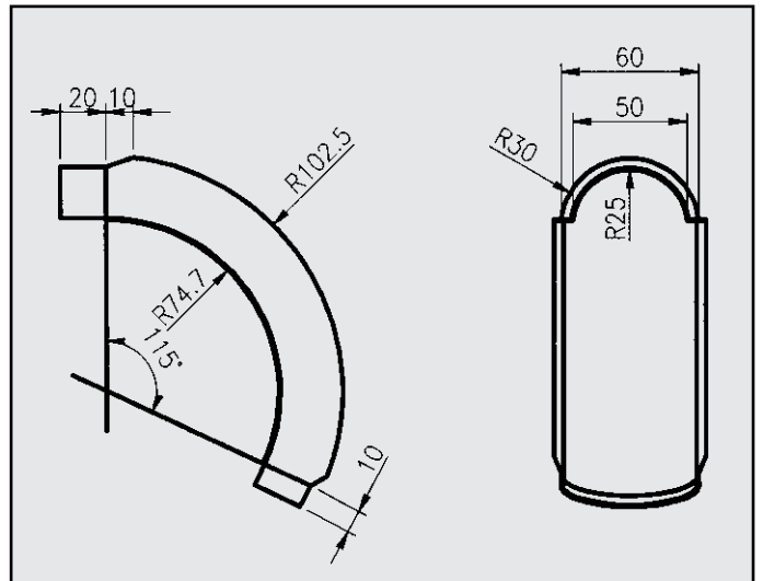
FIAT MAREA PROTEZIONE CALORE COD. PC 242806
