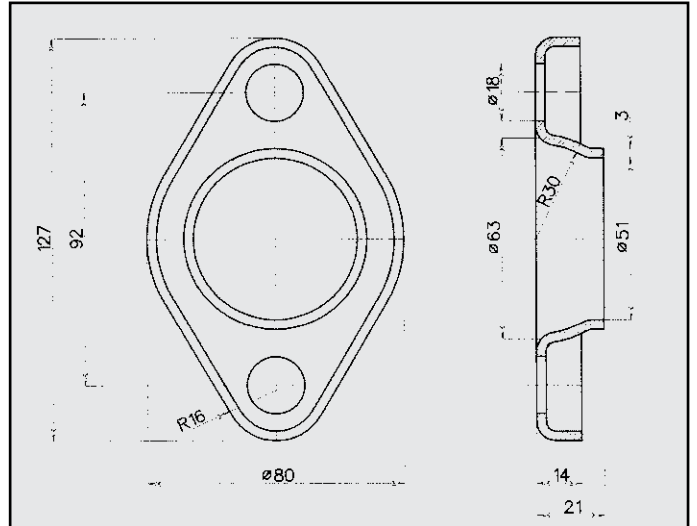
HONDA CIVIC 1.6 FLANGIA COD. FL 280427
