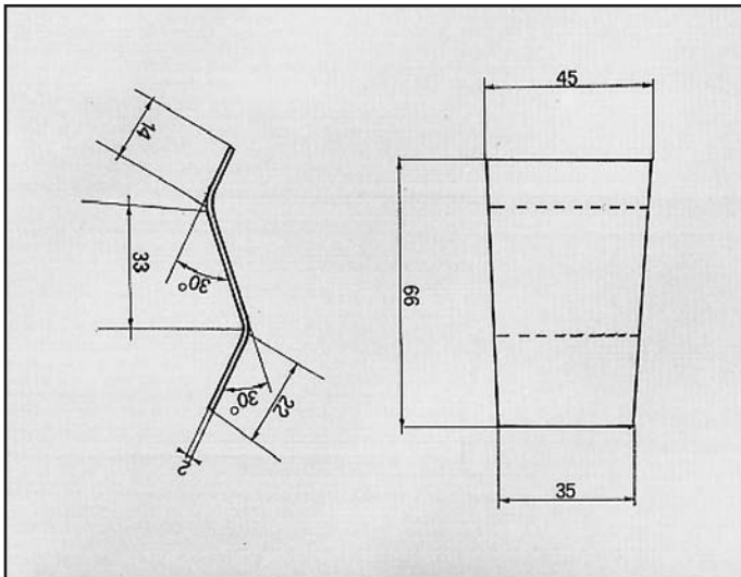
MINI DE TOMMASO RINFORZO per posteriore COD. R 320101
