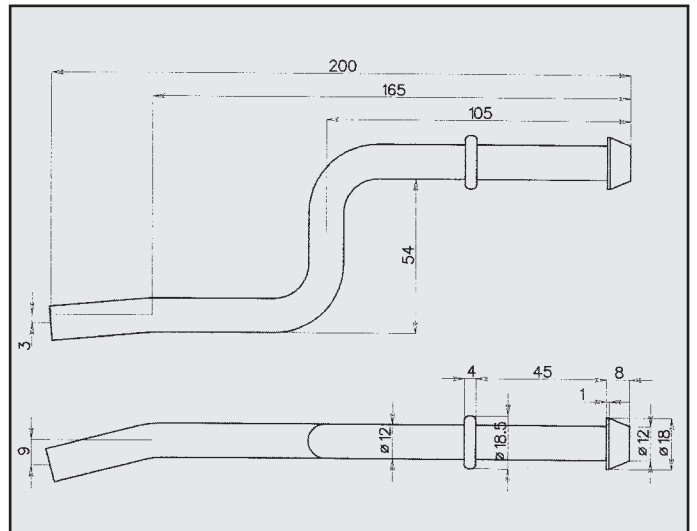
OPEL ZAFIRA ATTACCO per posteriore COD. AT 521301
