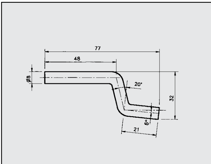
METRO 1000 ATTACCO per posteriore COD. AT 060103
