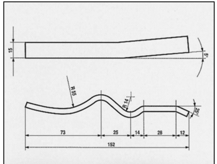
FIAT UNO TURBO I.E. 09/1989 RINFORZO centrale COD. R 240918
