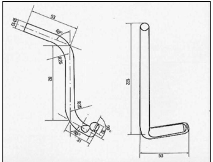
UNO 55 ATTACCO per posteriore COD. AT 240903
