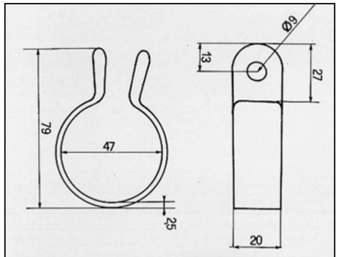
TIPO FASCETTA per rinforzo COD. R 241706
