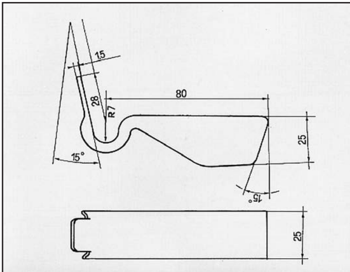
SAMARA ATTACCO marmitta speciale 2 tubi COD. AT 360101
