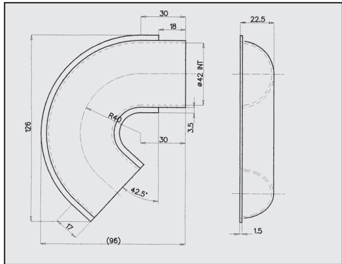
CITROEN AX/PEUGEOT 106 PROTEZIONE COD. PC 140713
