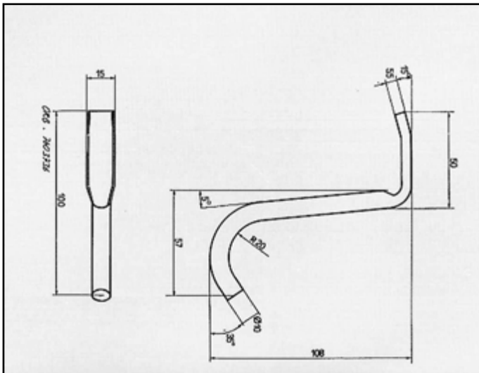
DUNA 70 ATTACCO per posteriore COD. AT 241002
