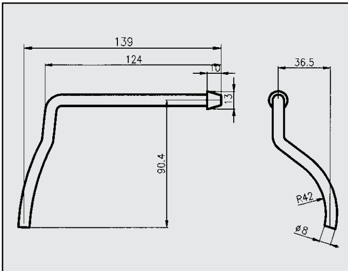
FIAT MAREA ATTACCO COD. AT 242809
