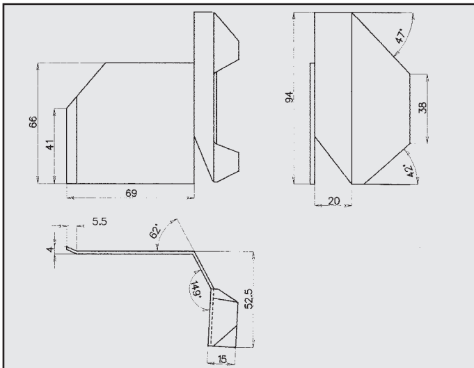
PEUGEOT 405 PROTEZIONE CALORE COD. PC 540704
