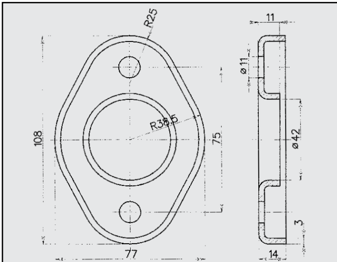
SUZUKI SJ 410 1.0 FLANGIA POSTERIORE COD. FL 720309
