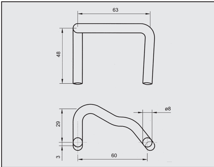
CITROEN AXEL 1.1R 1.2TRS ATTACCO per centrale COD. AT 140708
