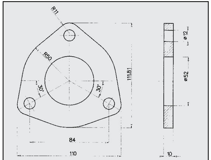
DAEWOO NUBIRA FLANGIA COD. FL 160310
