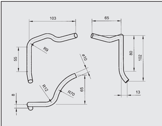
NISSAN MICRA ATTACCO per posteriore COD. AT 500205
