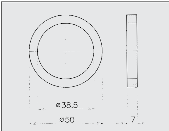
PEUGEOT ANELLO COD. AN 540004
