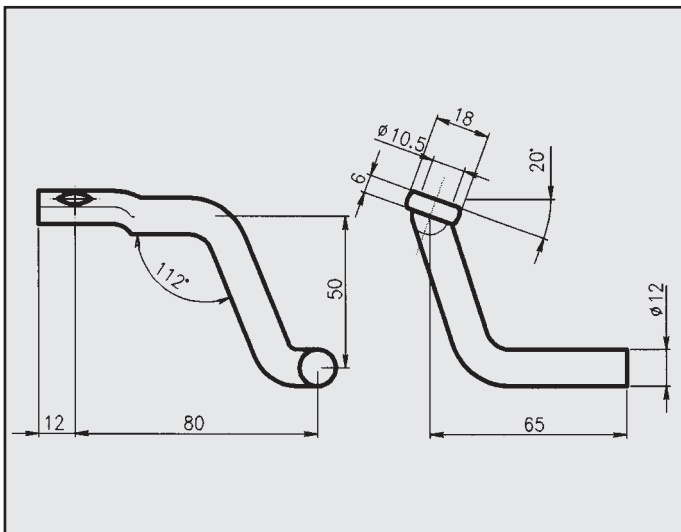
MITSUBISHI PAJERO 2.5 '86 ATTACCO per posteriore COD. AT 460207
