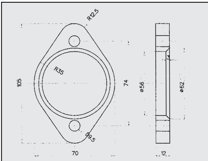
BMW 318 I FLANGIA COD. FL 120604
