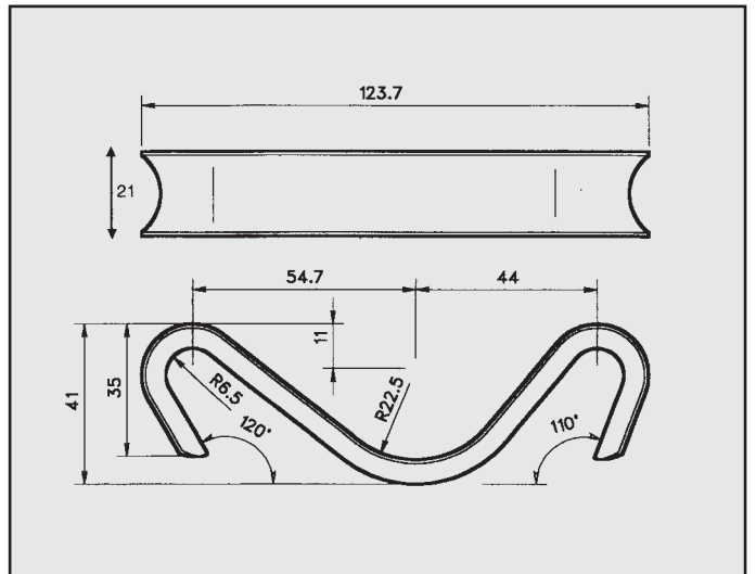
LANCIA DELTA/PRISMA 1300/86 ATTACCO per anteriore COD. AT 380313
