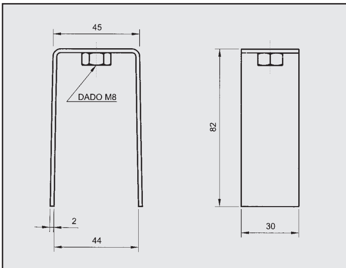
SUZUKI VITARA ATTACCO per posteriore COD. AT 720111
