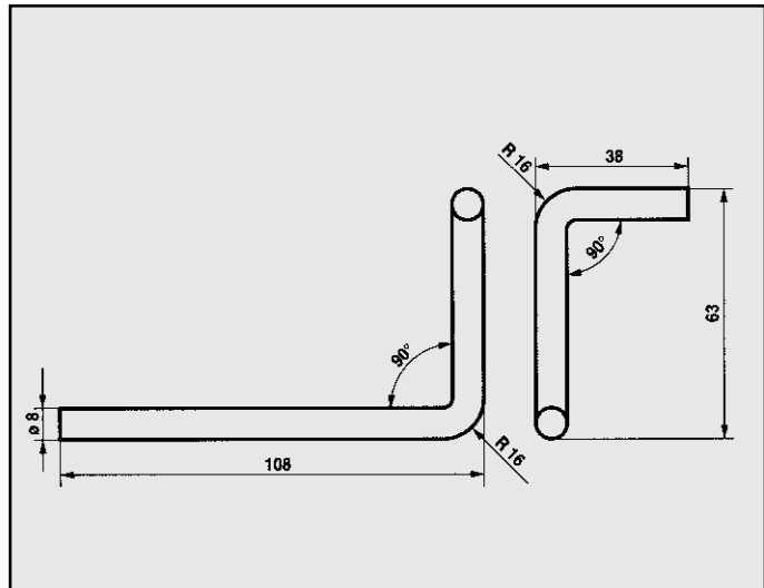
CITROEN BX GTI ATTACCO per posteriore COD. AT 140304 95634351
