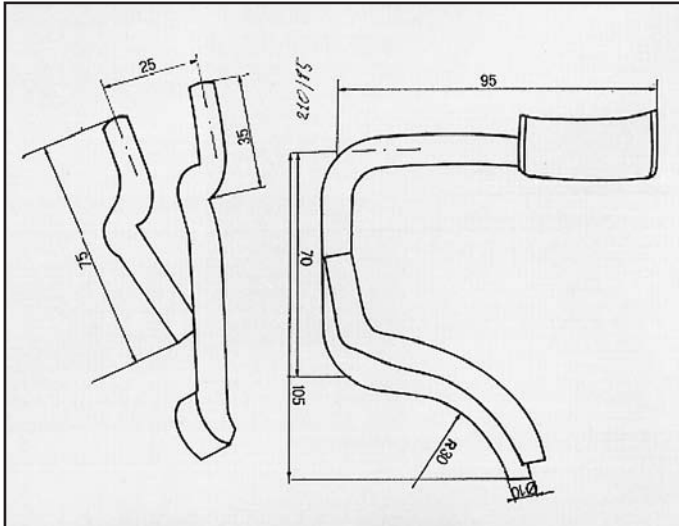
SIERRA 1800/2000 ATTACCO per centrale COD. AT 260613
