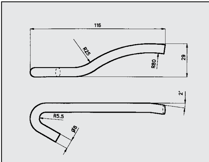
ALFA MILANO ATTACCO per posteriore SX COD. AT 020701/SX
