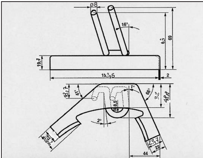
LANCIA DELTA 1.4 R 93 ATTACCO posteriore COD. AT 380331 7742193
