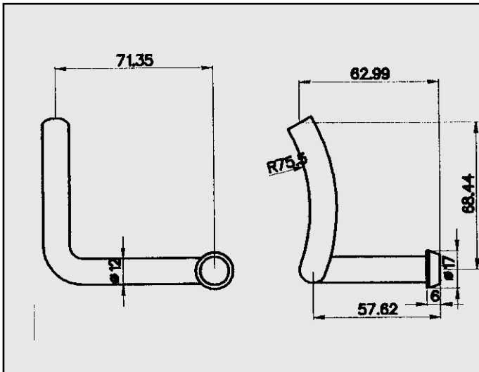
AUDI A4 ATTACCO COD. AT 040605
