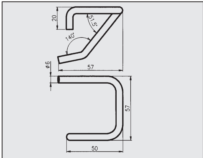
LIGIER ATTACCO anteriore COD. AT 390005
