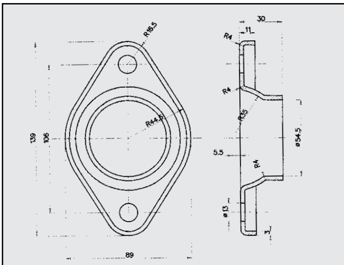
SUZUKI SANTANA ANIBAL FLANGIA COD. FL 720502
