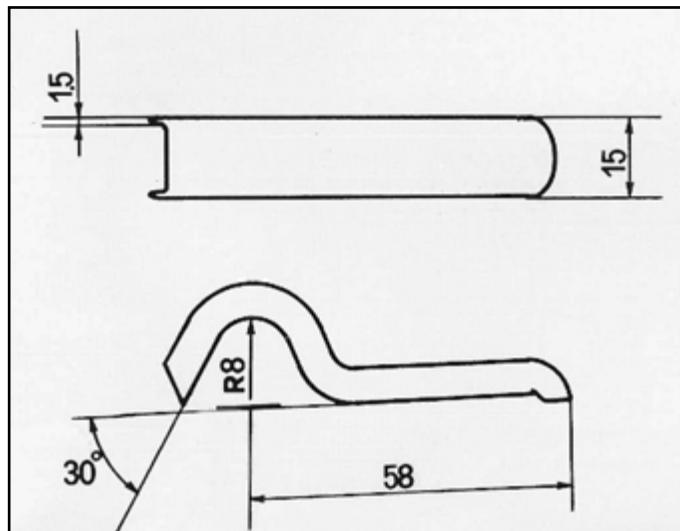
ARGENTA ATTACCO per posteriore COD. AT 241202
