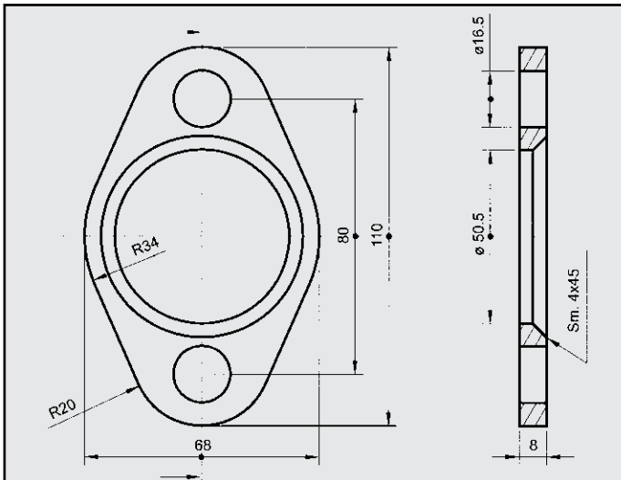
AUTOBIANCHI Y10 1.1 I.E. FLANGIA COD. FL 080221
