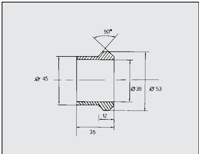
CITROEN AX 10 ANELLO ø esterno mm 53 ø interno mm 39 lunghezza mm 35 COD. AN 140702
