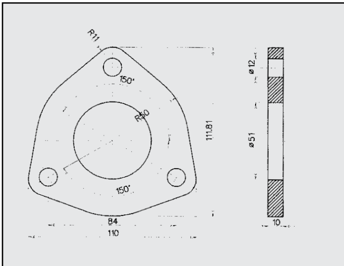
DAEWOO LANOS FLANGIA COD. FL 160203
