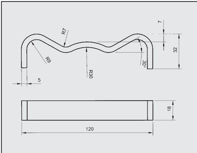
SAAB 900 I 2.0 16V ATTACCO posteriore COD. AT 640204
