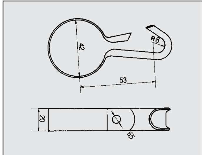
ALFASUD ATTACCO per posteriore COD. AT 020104
