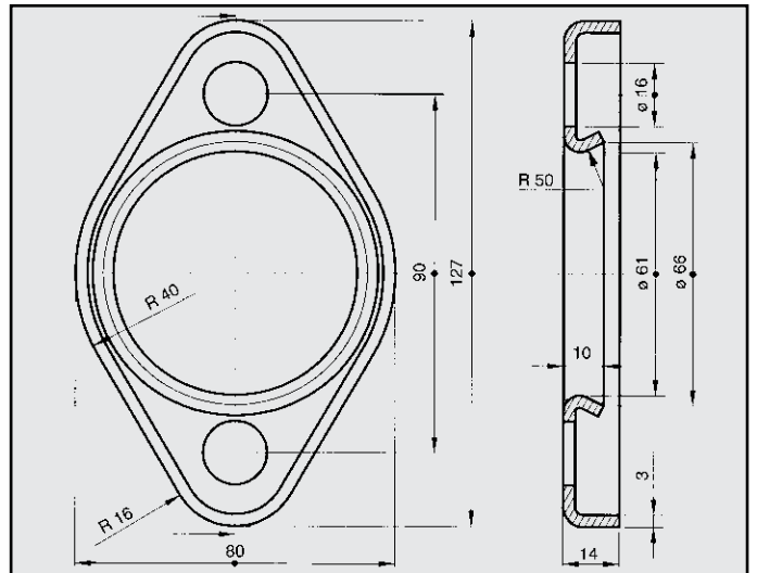
FORD ESCORT FLANGIA COD. FL 260265
