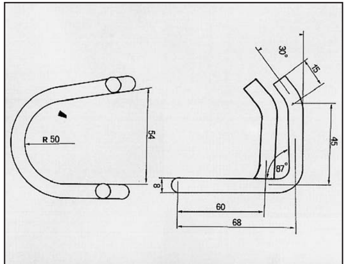
SUPER 5 ATTACCO per centrale COD. AT 600106
