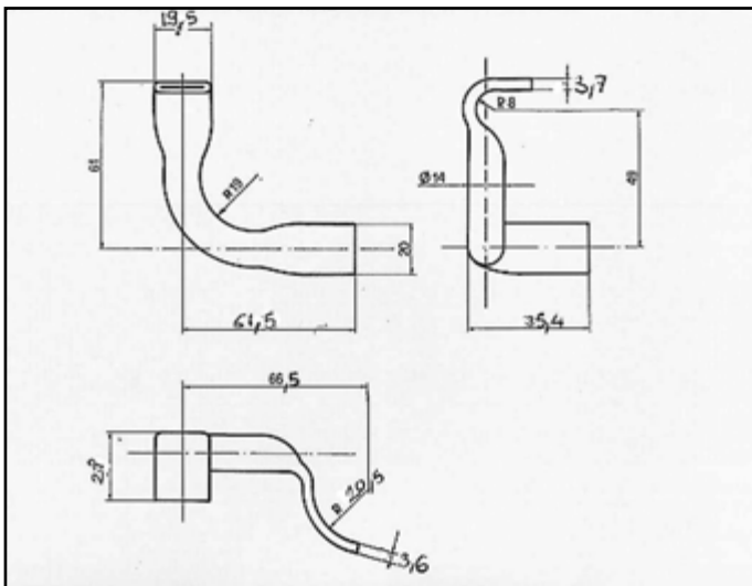
PANDA 750 YOUNG ATTACCO per posteriore COD. AT 240111
