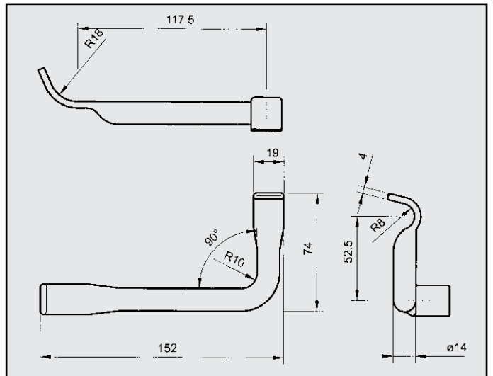
FIAT PANDA SELECTA ATTACCO per posteriore COD. AT 240113
