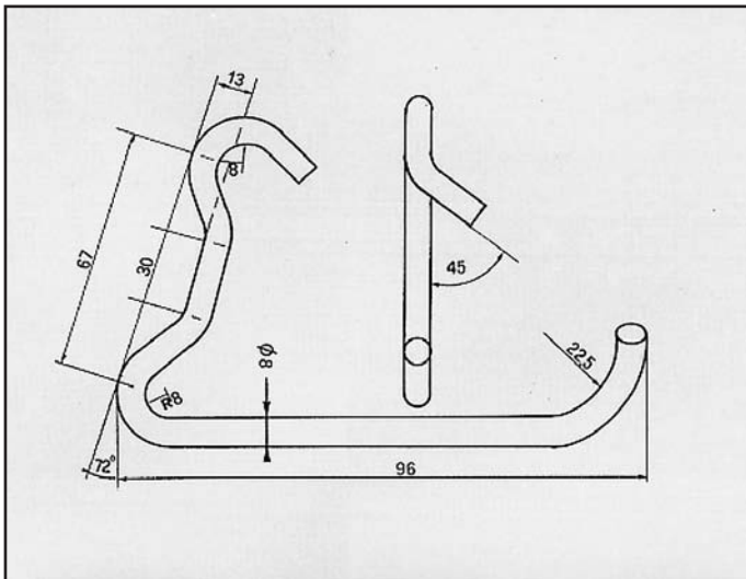
343/345 2000 ATTACCO per posteriore COD. AT 880102
