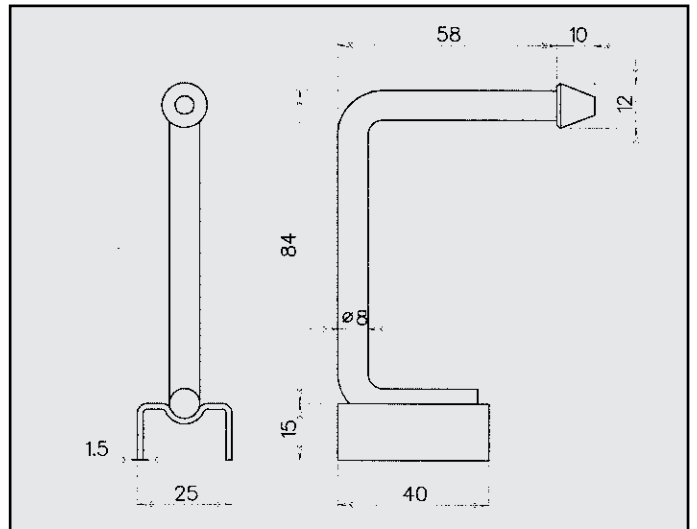
FIAT PUNTO ATTACCO COD. AT 242219
