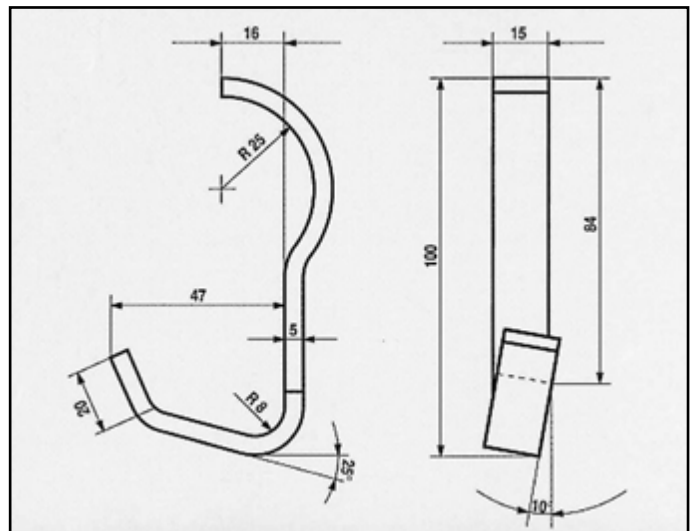
FIAT TEMPRA 1400/1600 B. e 1900 DIESEL ATTACCO per posteriore COD. AT 241901
