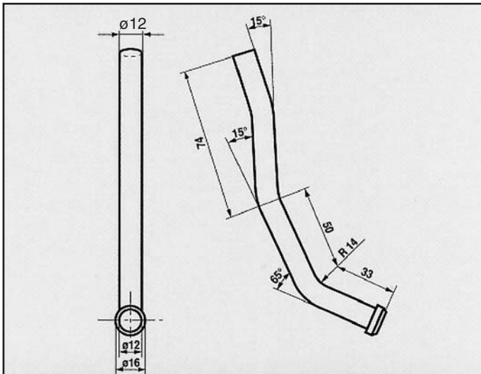
TOYOTA CRESSIDA 1984/86 ATTACCO per posteriore COD. AT 801101
