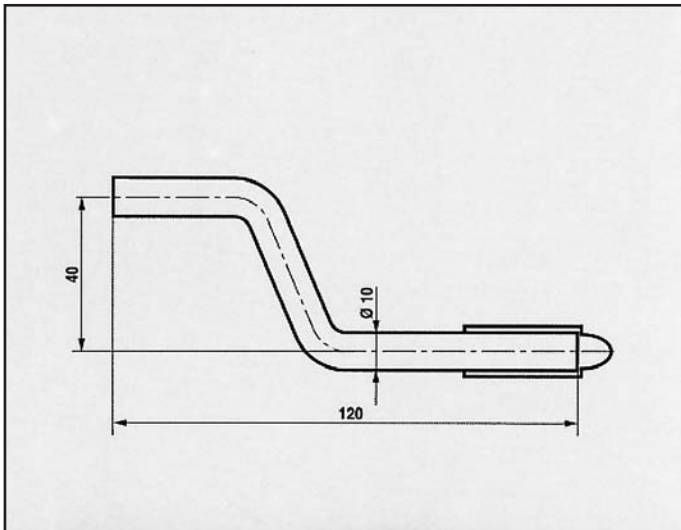
OPEL CORSA 1.6 GSI ATTACCO COD. AT 520305
