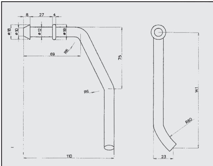
PEUGEOT 206 1.4 ATTACCO COD. AT 541204
