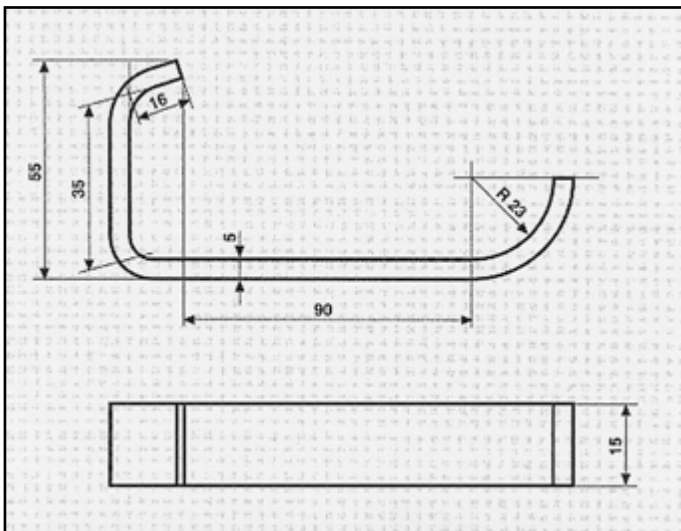
FIAT TIPO 1600 CATALIZZATA ATTACCO posteriore COD. AT 241711 7657985
