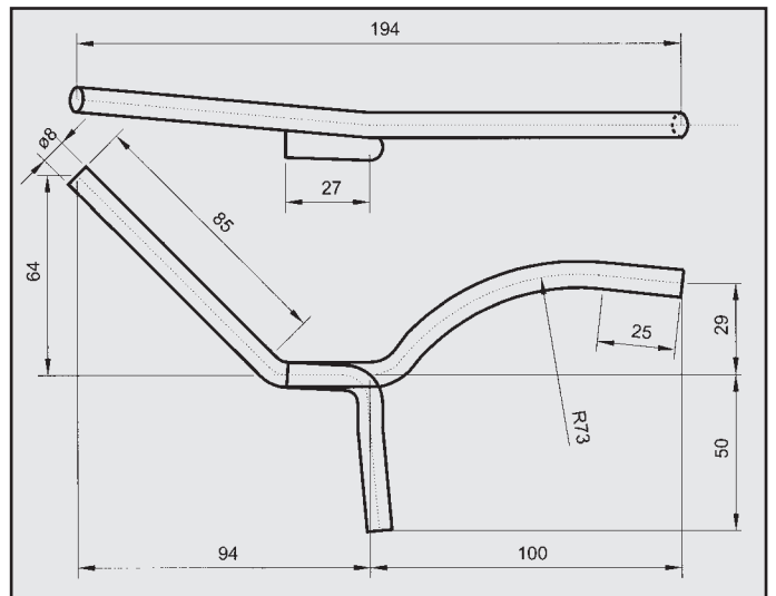
RENAULT LAGUNA 1,8 - 2,0i CAT ATTACCO centrale COD. AT 601401
