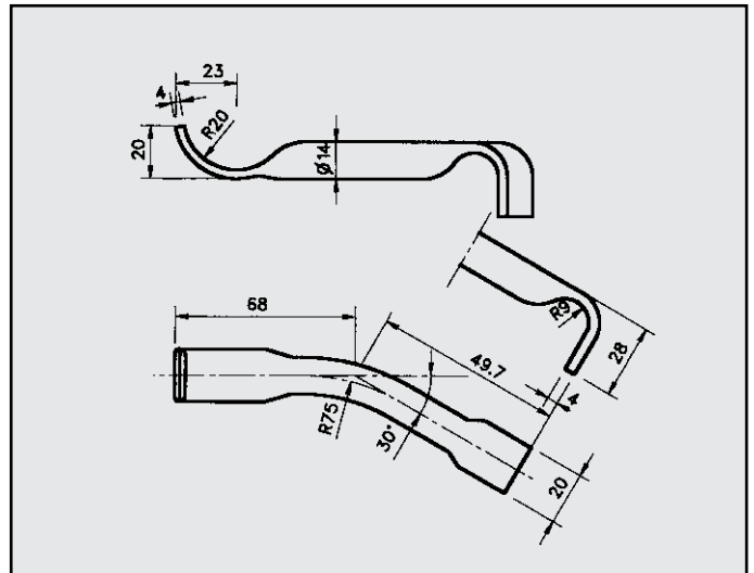
AUTOBIANCHI Y10 TOURING ATTACCO per centrale COD. AT 080205
