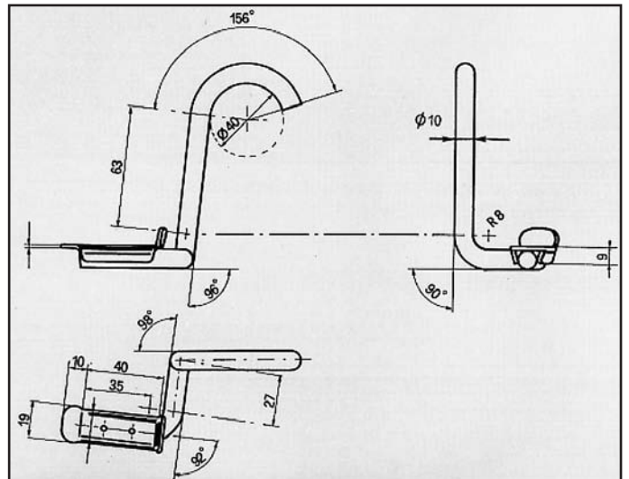
ESCORT 2ª SERIE ATTACCO per centrale COD. AT 260215
