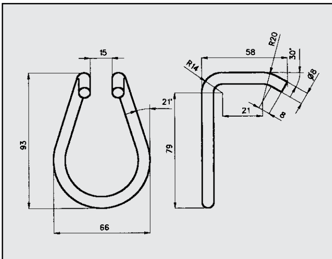
DUNA 60 - 70 ATTACCO per posteriore COD. AT 241003
