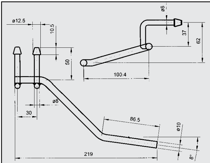
FIAT PUNTO GT ATTACCO COD. AT 242216
