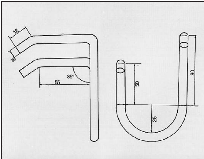
R21 NEVADA ATTACCO per posteriore COD. AT 601001
