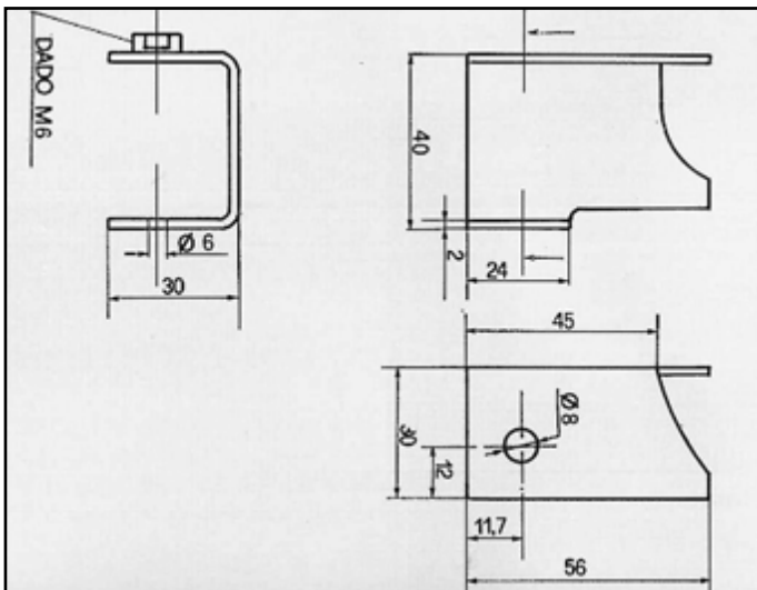
PANDA 30 / 4x4 / 45 ATTACCO per posteriore COD. AT 240105 5888166 4449004 7550388 5973760
