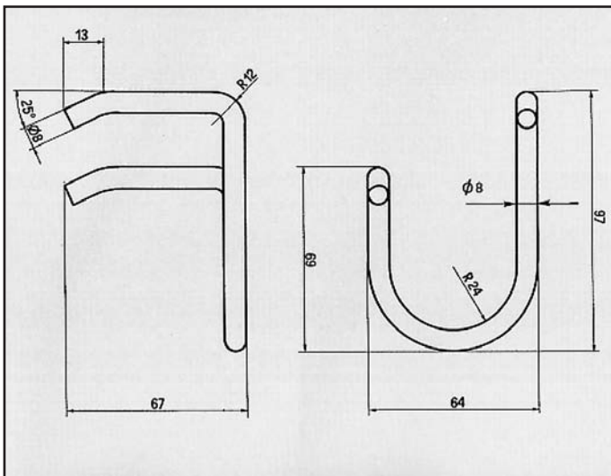
SUPER 5 ATTACCO per posteriore COD. AT 600104
