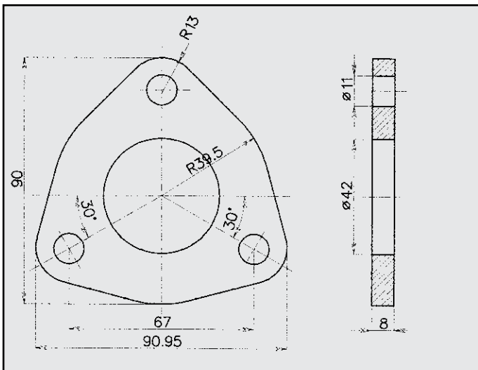
SKODA FELICITA FLANGIA COD. FL 690303
