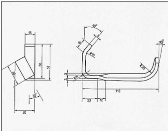
UNO 45 ATTACCO per posteriore COD. AT 240902
