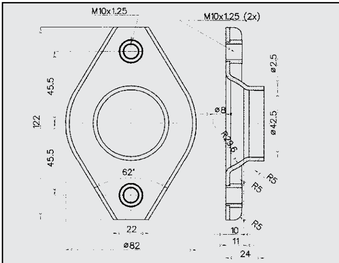
TOYOTA FLANGIA COD. FL 800007
