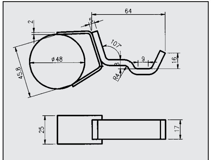
FIAT MAREA 1.8 16V ATTACCO COD. AT 242804
