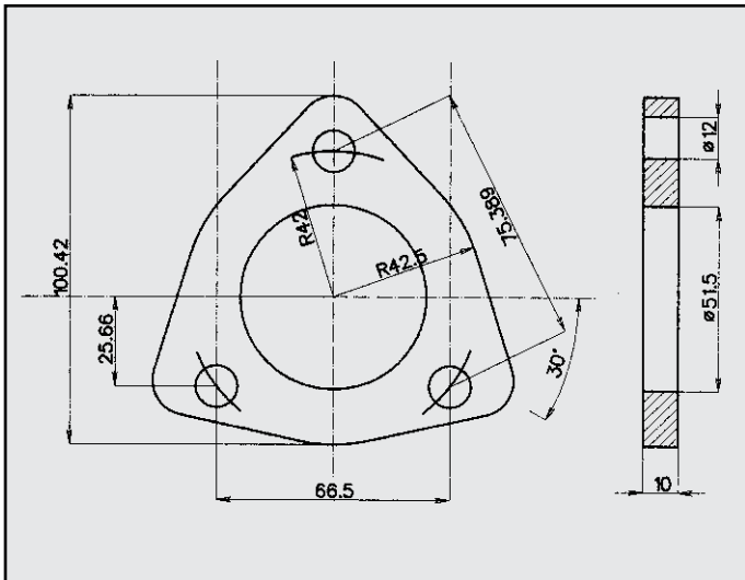
ROVER 825 FLANGIA COD. FL 620007
