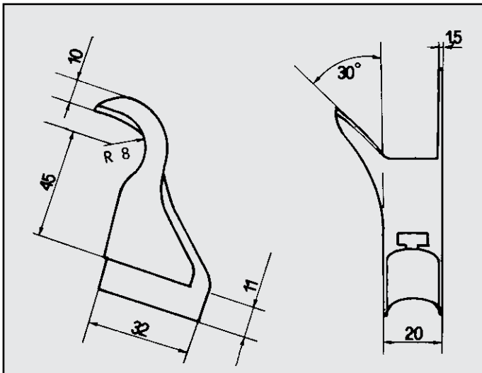
AUDI 50/80 ATTACCO per centrale COD. AT 040401
