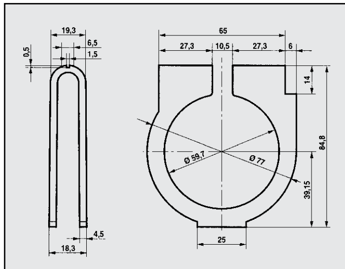
FIAT PUNTO GT FASCETTA COD. F 242207
