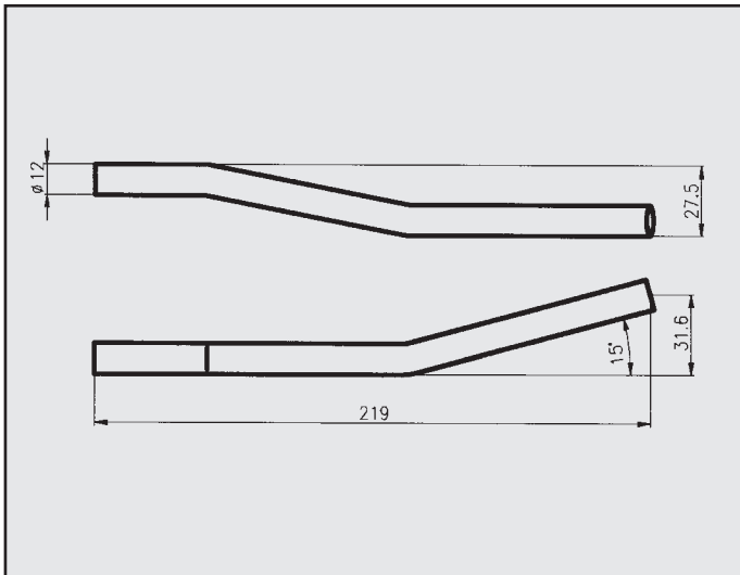
OPEL ASTRA ATTACCO per posteriore COD. AT 520922
