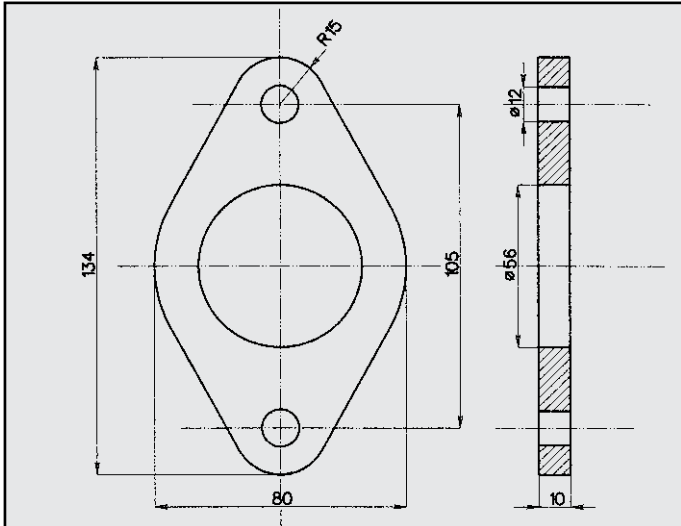
FORD MONDEO FLANGIA COD. FL 261217
