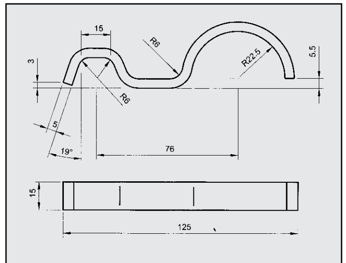
FIAT BRAVO BRAVA 1.4 ATTACCO per posteriore COD. AT 242310
