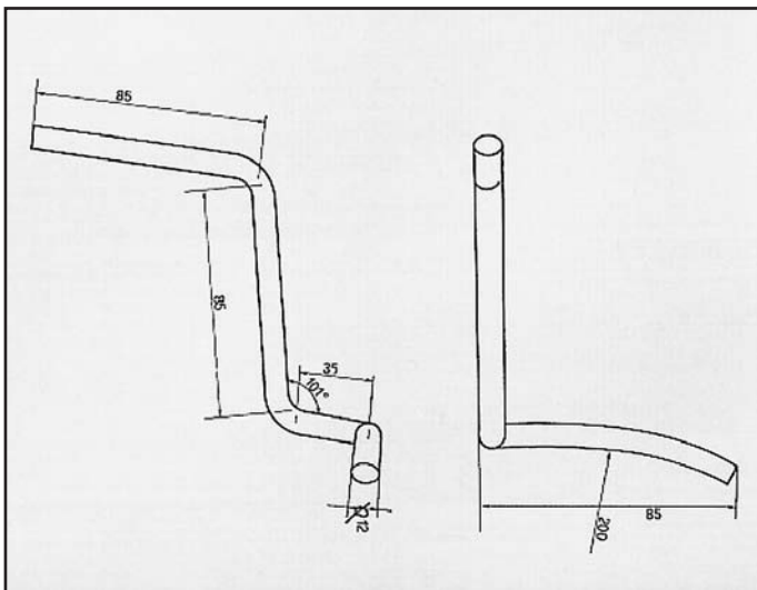
PASSAT 1600-1800 ATTACCO per anteriore COD. AT 860203
