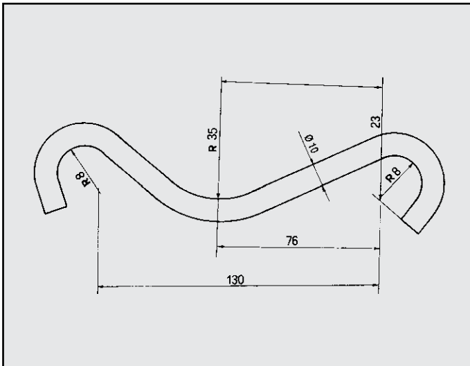
ALFA 33 ATTACCO per posteriore COD. AT 020107
