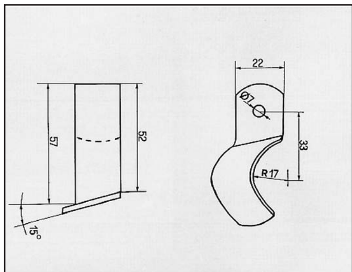
R5 ATTACCO per tubo centrale COD. AT 600101
