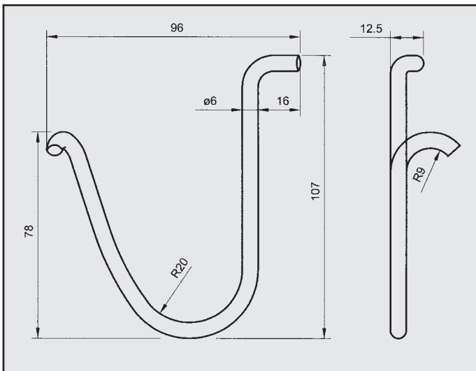
OPEL ASTRA RINFORZO COD. R 520903
