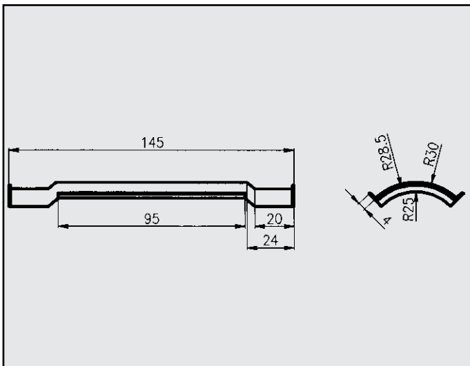
FIAT BRAVO PROTEZIONE CALORE COD. PC 242315
