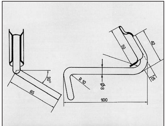
CORSA SPORT ATTACCO per posteriore COD. AT 520302
