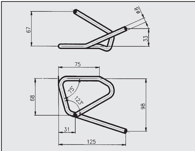
RENAULT LAGUNA 1.8 i ATTACCO per posteriore COD. AT 601404
