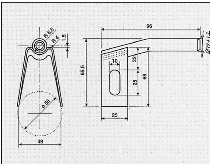
VOLKSWAGEN GOLF III 1.8 CATALIZZATA 90 HP ATTACCO centrale COD. AT 860120
