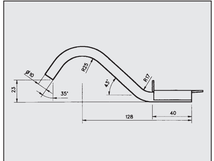
FORD FIESTA XR2 1600 ATTACCO per posteriore COD. R 260308
