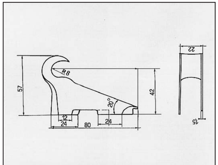
POLO 1ª SERIE ATTACCO per posteriore COD. AT 860302
