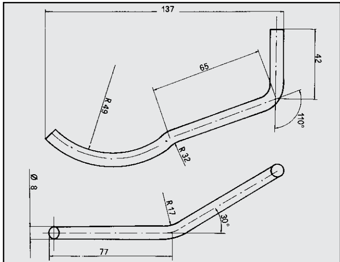
ALFA MILANO ATTACCO per posteriore COD. AT 020702
