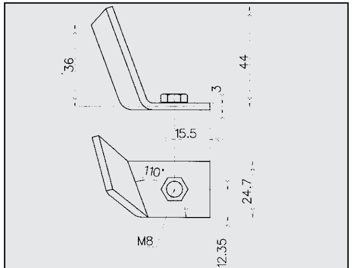
FIAT 1,3 - 1,5 '62 ATTACCO COD. AT 240502 4241982
