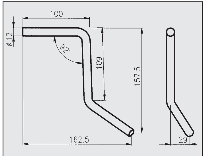
OPEL ASTRA 1.8 16V ATTACCO per posteriore COD. AT 520913
