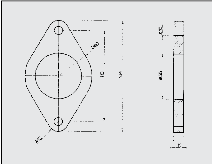
ALFA GTV 2.0 FLANGIA COD. FL 020616
