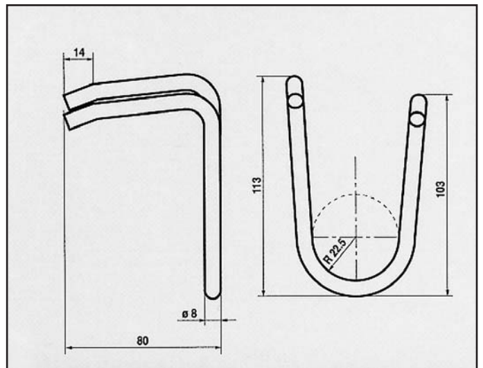
RENAULT R9-R11 / 1986-88 ATTACCO per posteriore COD. AT 600209
