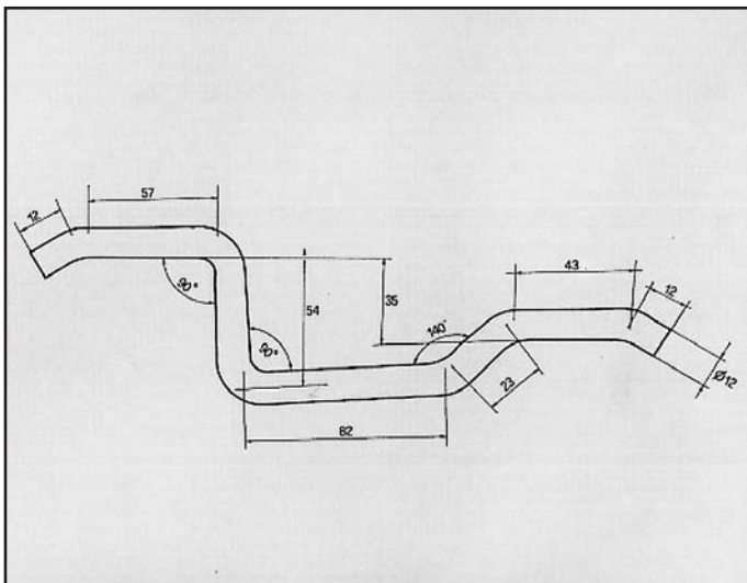
OMEGA ATTACCO per posteriore COD. AT 520604
