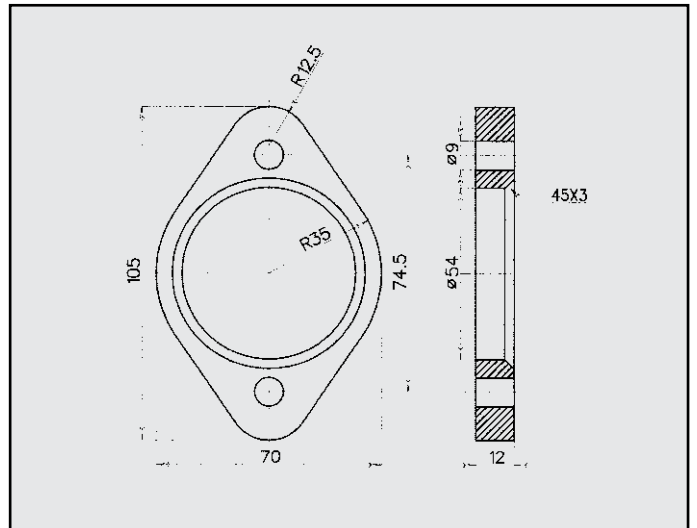
B M W / MERCEDES 190 FLANGIA COD. FL 120501
