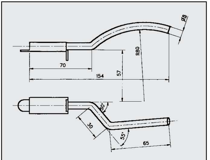
MINI METRO ATTACCO per posteriore COD. AT 060109
