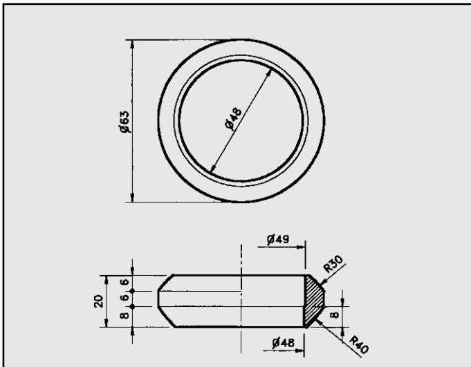
LANCIA BETA ANELLO senza collare \varnothing esterno mm 63 \varnothing interno mm 47 COD. AN 380101
