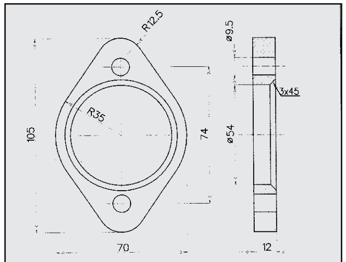
B M W 325 FLANGIA POSTERIORE COD. FL 120502
