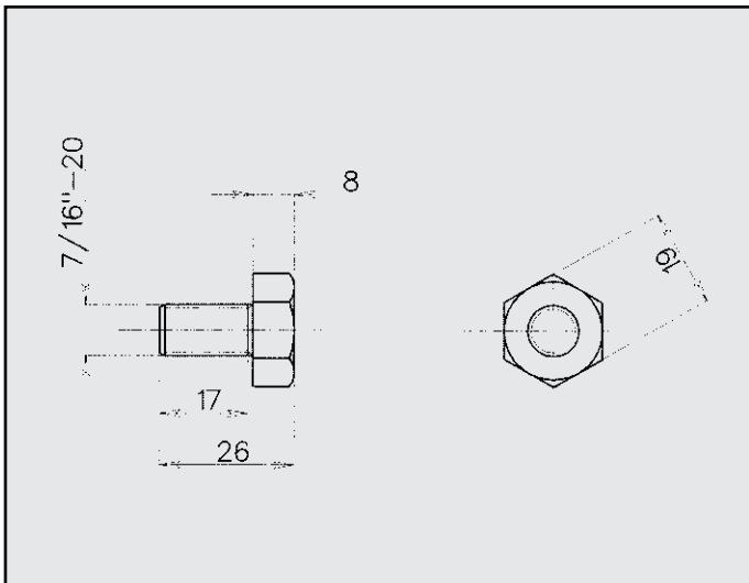
FIAT TIPO/TEMPRA - LANCIA DELTA VITE COD. VI 241727
