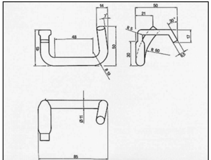
UNO TURBO DIESEL ATTACCO per posteriore COD. AT 240910
