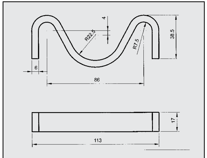
FIAT DUCATO ATTACCO COD. AT 241507
