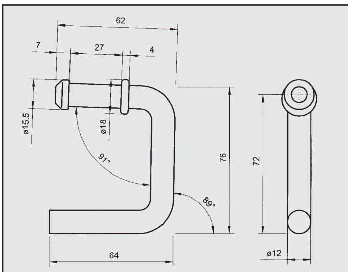
TOYOTA COROLLA 1.6 ATTACCO per posteriore COD. AT 800419
