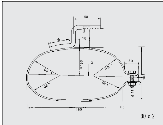
OPEL KADET GT FASCETTA per posteriore COD. F 520101 X = 100-123-127
