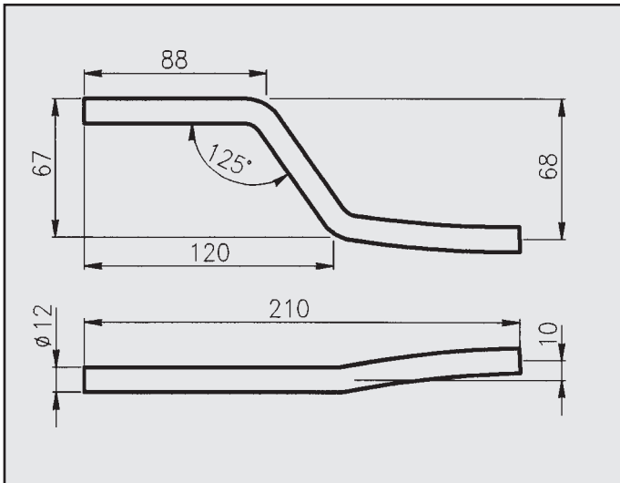
OPEL ASTRA 1.8 16V ATTACCO per posteriore COD. AT 520915
