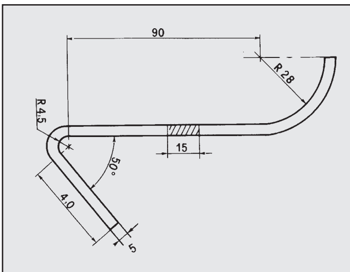
740 TURBO ATTACCO per posteriore COD. AT 880201
