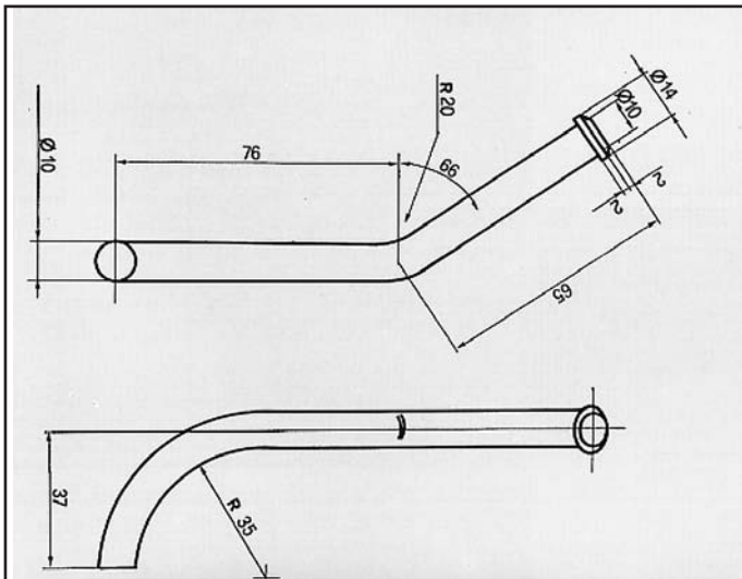
CEDRIC ATTACCO per posteriore COD. AT 500101
