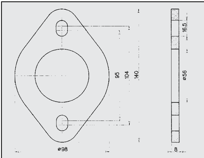
ALFA 155 2.0 FLANGIA CENTRALE COD. FL 021015
