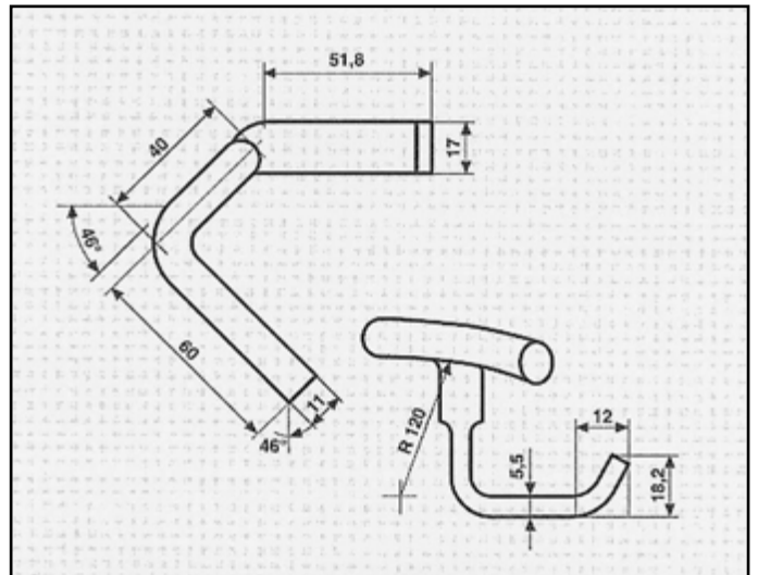
FIAT CINQUECENTO NUOVA ATTACCO anteriore per posteriore COD. AT 242102
