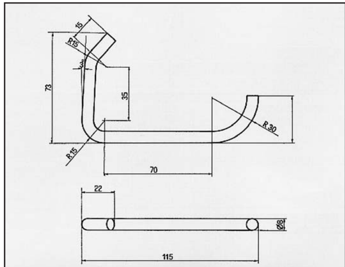
HORIZON ATTACCO per posteriore COD. AT 780202 0059114807 0059129407
