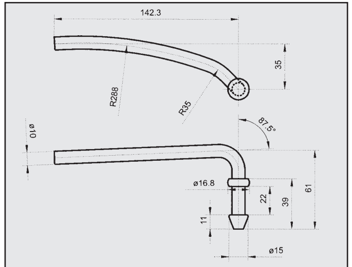
FORD FIESTA 1,2i CAT '95 ATTACCO per posteriore COD. AT 260333
