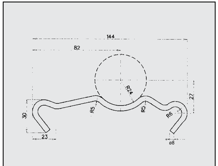
FIAT FIORINO ATTACCO CENTRALE COD. AT 241803
