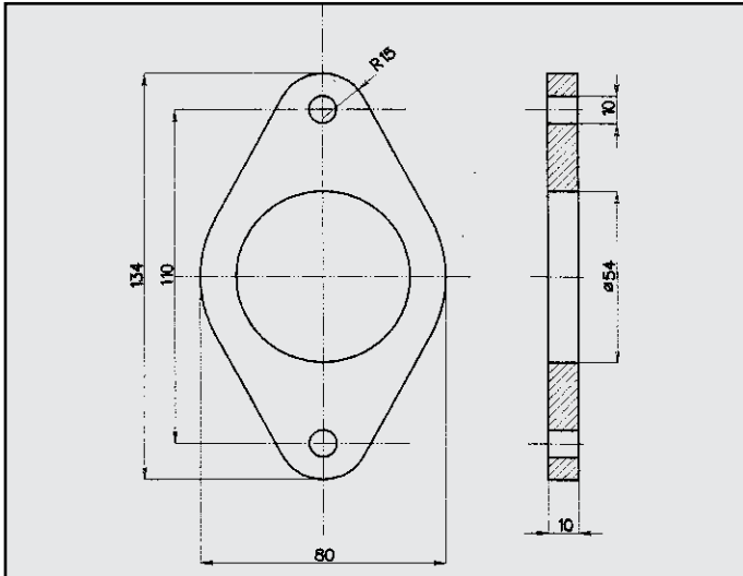
ALFA GTV FLANGIA COD. FL 020615
