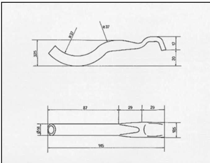
TIPO BENZINA E DIESEL ATTACCO per anteriore COD. AT 241703
