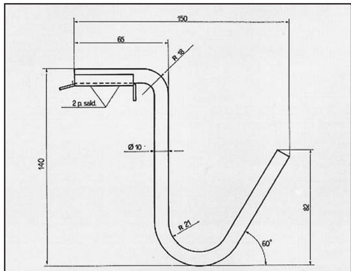
ESCORT 1100/82 ATTACCO per posteriore COD. AT 260208 6150799 6131717
