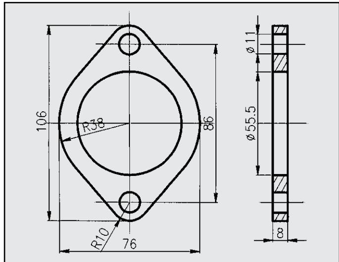
RENAULT CLIO FLANGIA COD. FL 601306
