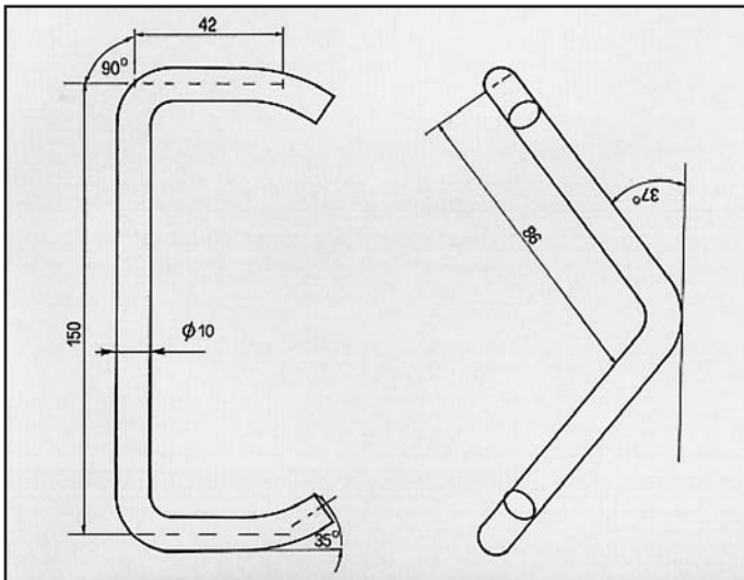
CIVIC 1500 ATTACCO per posteriore COD. AT 280408
