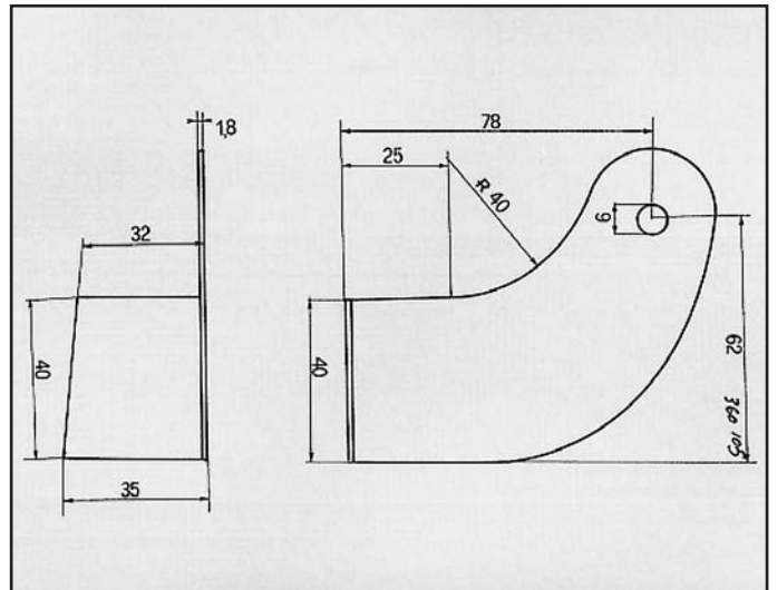
BETA/TREVI 3ª SERIE ATTACCO per centrale dx COD. AT 380105
