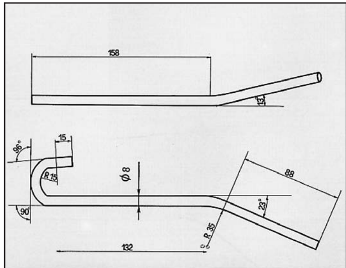
626 ATTACCO per tubo centrale COD. AT 420502
