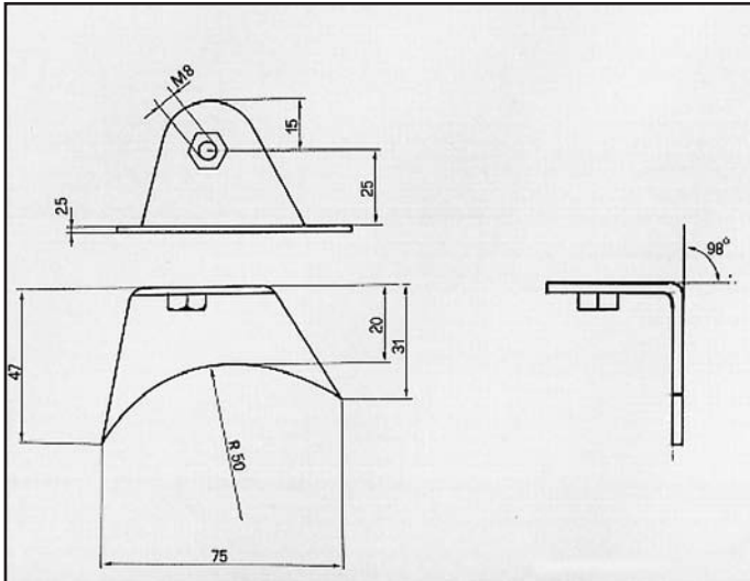
DELTA 1500 ATTACCO per centrale COD. AT 380303
