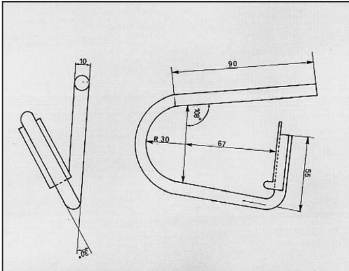
FIESTA 1400 ATTACCO per posteriore COD. AT 260311
