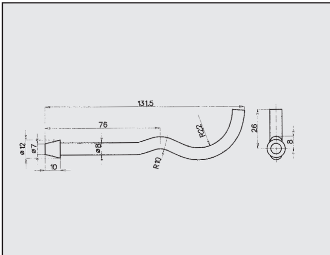
LANCIA Y 1.2i 16V ATTACCO COD. AT 381202
