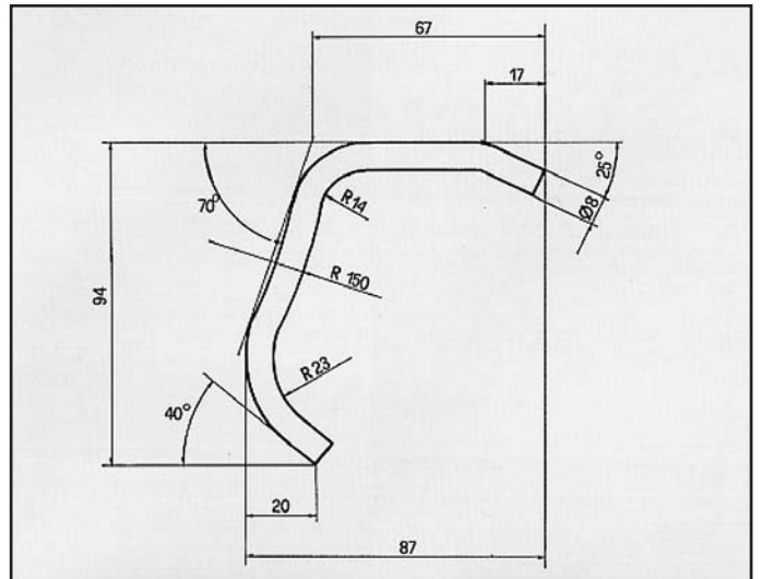
R9-R11 ATTACCO per posteriore COD. AT600206
