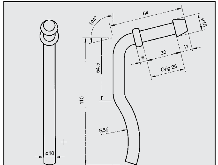
BMW 316 1.6 COMPACT ATTACCO per posteriore COD. AT 120113
