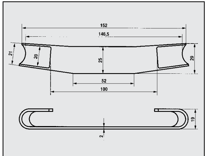
ALFA 75 INIEZIONE ATTACCO centrale COD. AT 020309
