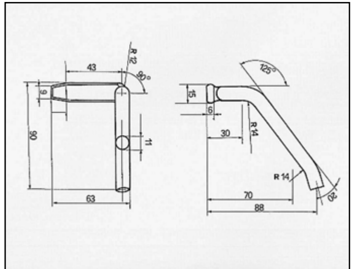
RITMO TURBO DIESEL ATTACCO per posteriore COD. AT 240807
