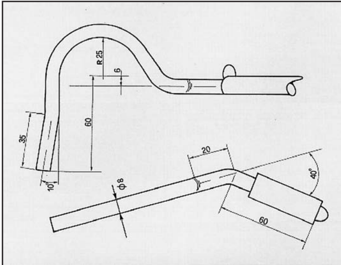
ESCORT 1100 ATTACCO per centrale COD. AT 260229
