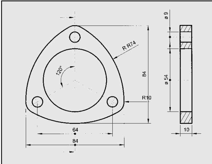
LANCIA DELTA PRISMA FLANGIA COD. FL 380343
