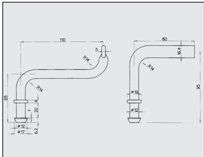
MERCEDES CLASSE A ATTACCO COD. AT 440705
