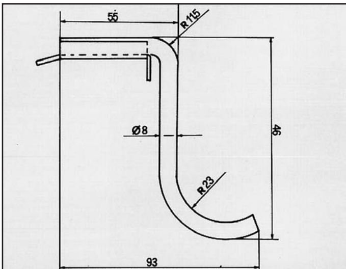
SIERRA 1300/1600 1ª SERIE ATTACCO per posteriore COD. AT 260614
