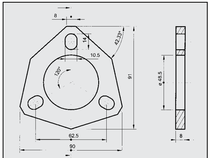
LANCIA DELTA PRISMA FLANGIA COD. FL 380340
