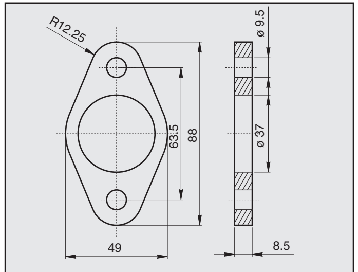
FIAT 500 BICILINDRICO FLANGIA COD. FL 242108
