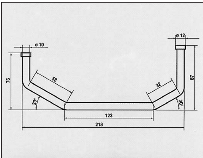
MAZDA 1.6 iniezione /1989 ATTACCO per posteriore COD. AT 420702
