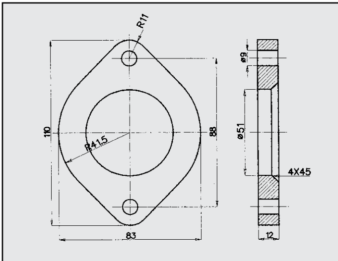
ALFA ROMEO 147 FLANGIA COD. FL 021501
