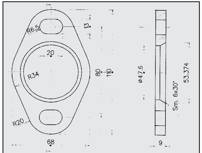
FIAT TIPO 1.4 FLANGIA COD. FL 241728
