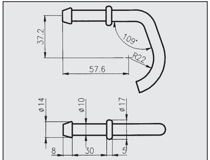
FORD KA ATTACCO per posteriore COD. AT 261401
