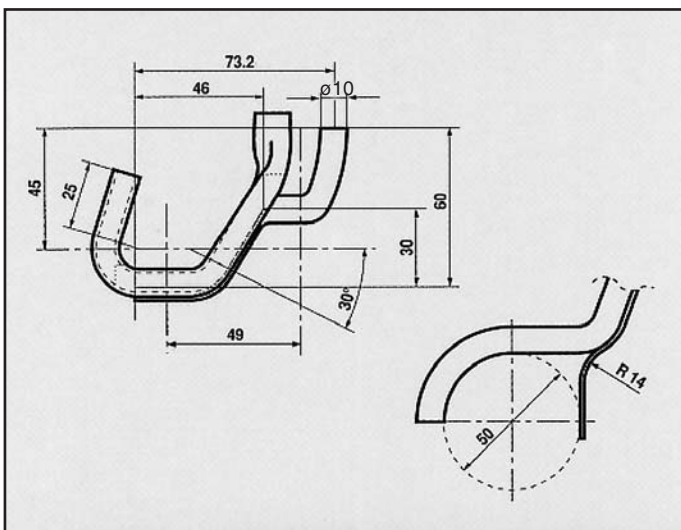
OPEL OMEGA 1991 ATTACCO per posteriore COD. AT 520606
