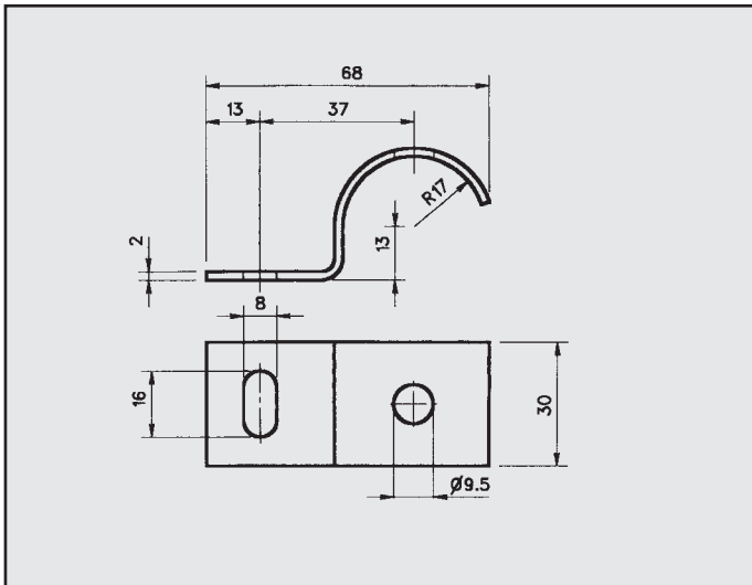
RENAULT R5 ATTACCO per tubo centrale COD. AT 600109
