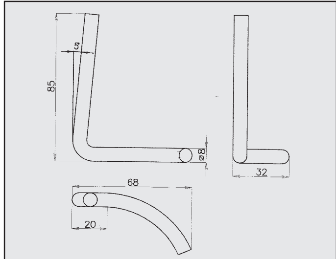
PEUGEOT 104 ZS ATTACCO POSTERIORE COD. AT 540202
