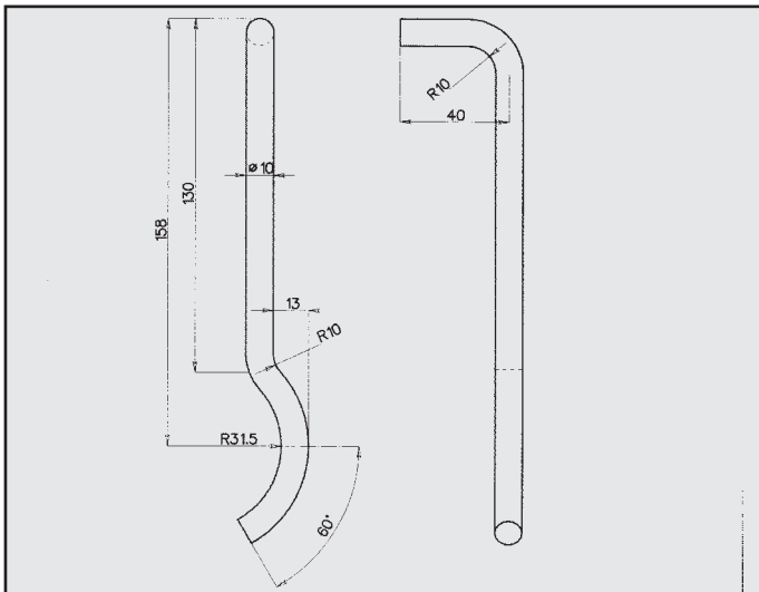
AUTO DA CORSA ATTACCO COD. AT 010002
