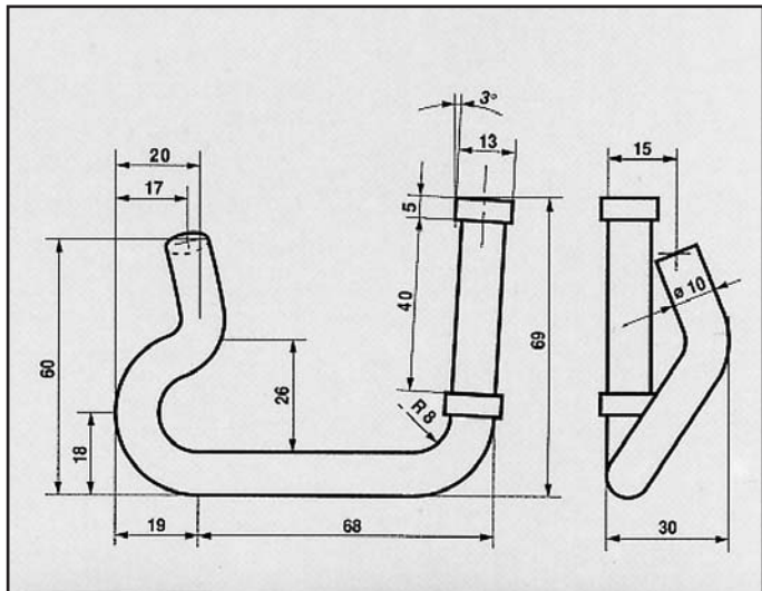
VOLVO 440/460/1.7 ATTACCO per posteriore COD. AT 880402 3414882-5
