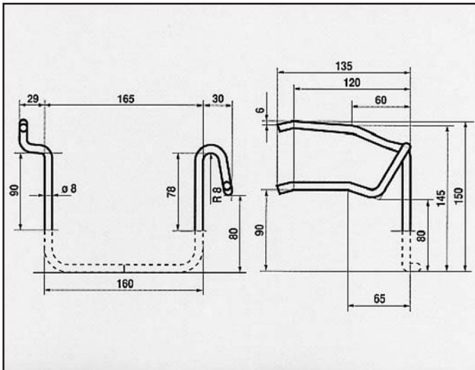
PEUGEOT 205/1988 ATTACCO per posteriore COD. AT 540312/2
