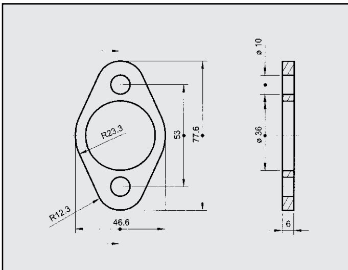
FIAT 126 FLANGIA COD. FL 240008
