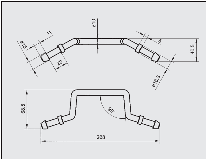
FORD ESCORT 1.8 115 CV ATTACCO centrale COD. AT 260262
