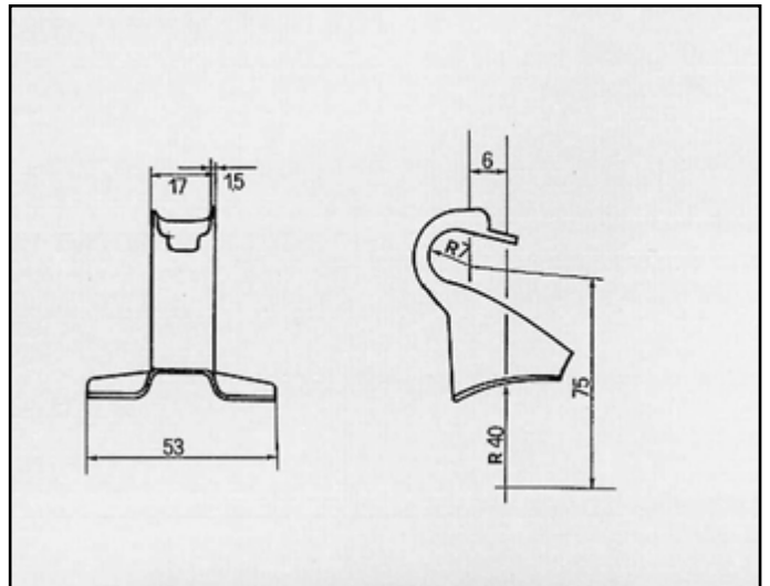
REGATA 70 ATTACCO per centrale COD. AT 241101
