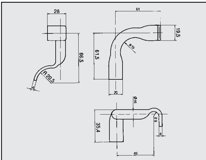
Y10 FIRE ATTACCO per posteriore COD. AT 080204
