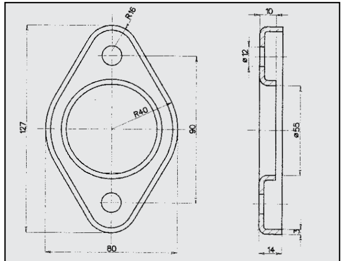
ROVER FLANGIA COD. FL 620003
