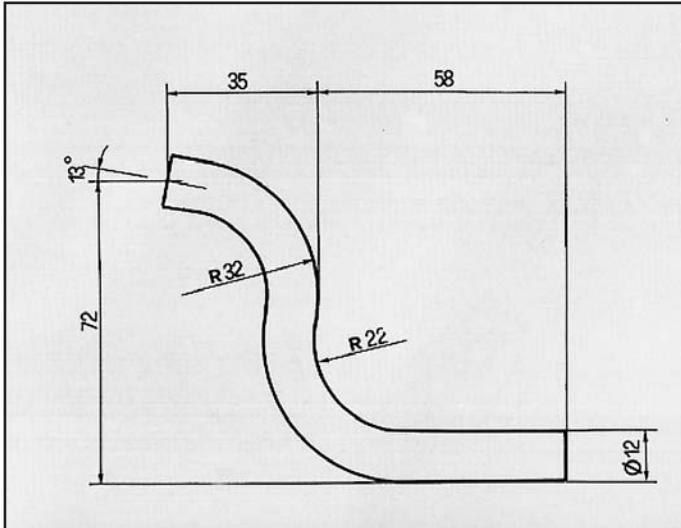
DELTA HF ATTACCO per posteriore COD. AT 380304
