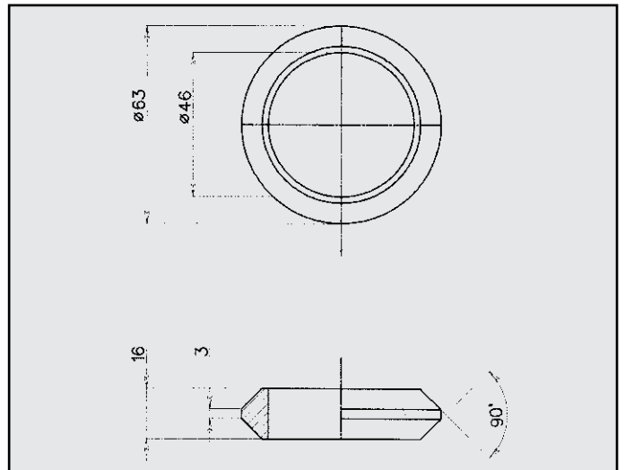
RENAULT CLIO 1.4 ANELLO COD. AN 601302
