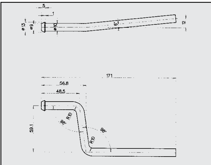
FIAT PUNTO TD ATTACCO COD. AT 242239
