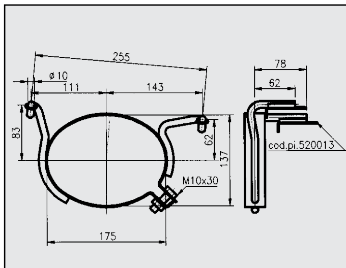
FIAT ULISSE FASCETTA per centrale COD. F 242701
