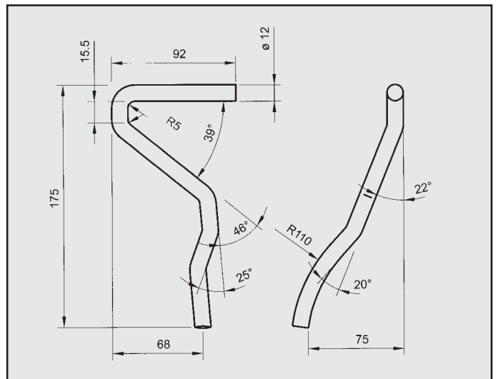
OPEL ASTRA ATTACCO per posteriore COD. AT 520908
