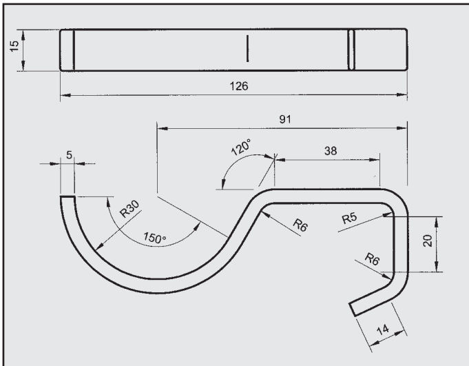
MERCEDES 300 SD TURBO DIESEL ATTACCO per posteriore COD. AT 440203
