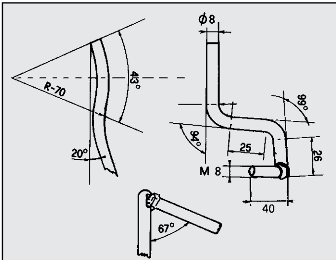
PULSAR 1600 ATTACCO per posteriore COD. AT 200101
