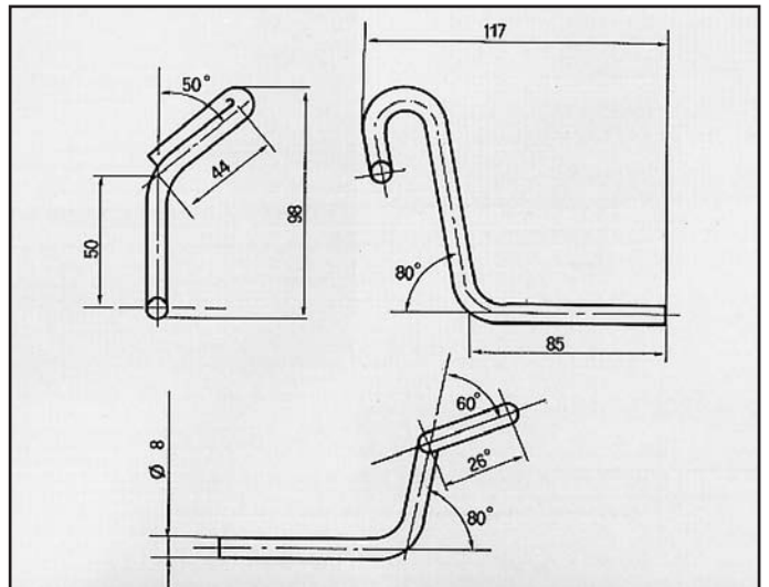
COROLLA 2ª SERIE ATTACCO per posteriore COD. AT 800404
