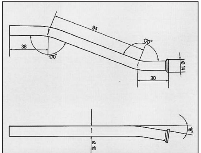
626 2000 16V ATTACCO posteriore dx per posteriore COD. AT 420515
