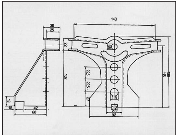
190 ATTACCO per posteriore COD. AT 440301
