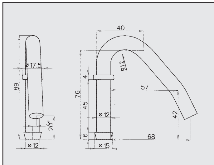
LANCIA LYBRA ATTACCO COD. AT 381103
