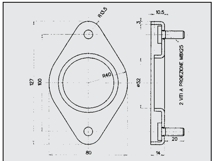
FIAT BRAVO-BRAVA 1.2 16V FLANGIA COD. FL 242325
