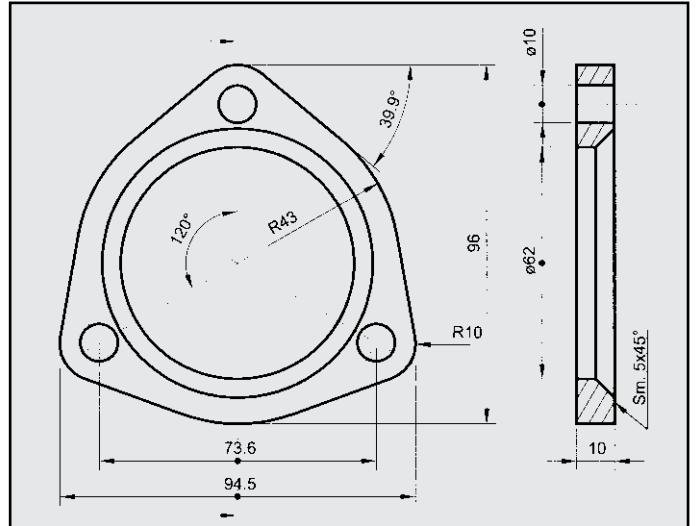
LANCIA THEMA - FIAT CROMA FLANGIA COD. FL 020905
