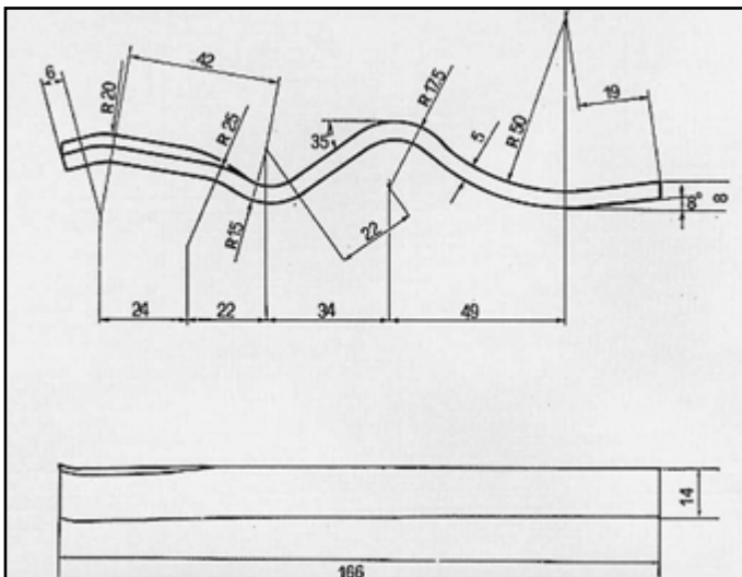
UNO DIESEL ATTACCO per posteriore COD. AT 240908
