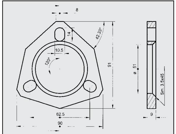
ALFA 164/87 - FIAT CROMA - LANCIA THEMA PRISMA FLANGIA COD. FL 020904
