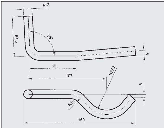
DELTA 2000 4WD ATTACCO per posteriore COD. AT 380324
