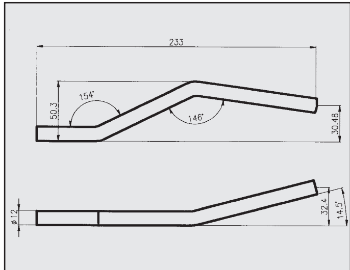
OPEL ASTRA ATTACCO per posteriore COD. AT 520925
