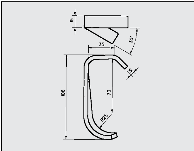
AUTOBIANCHI Y10 TURBO / Y10 GTIE ATTACCO anteriore per marmitta posteriore COD. AT 080209 7571237 7538231 7649426
