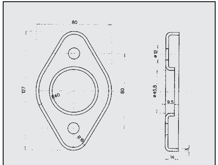
DAEWOO MATIZ 800 FLANGIA COD. FL 160104
