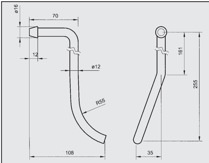
NISSAN PRIMERA 2.0 D. ATTACCO per posteriore COD. AT 500407
