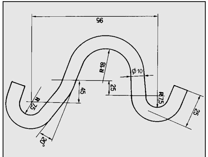
ALFA 33 1500 4x4 ATTACCO per centrale COD. AT 020110
