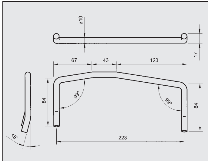
ROVER 414 ATTACCO per posteriore COD. AT 620902
