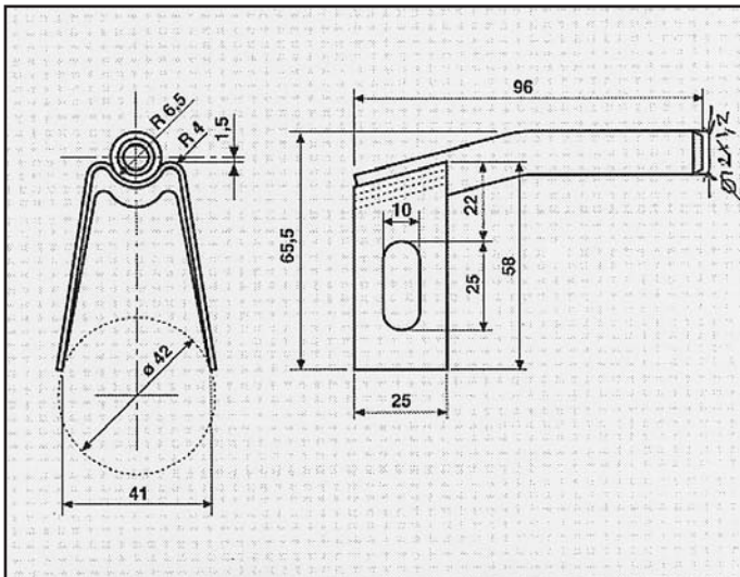
VOLKSWAGEN GOLF III 1.4/1.8 CATALIZZATA ATTACCO posteriore COD. AT 860119
