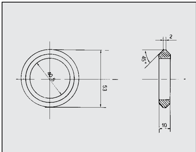
CITROEN AX 10 ANELLO \varnothing esterno mm 53 \varnothing interno mm 40,5 larghezza mm 10 COD. AN 140701
