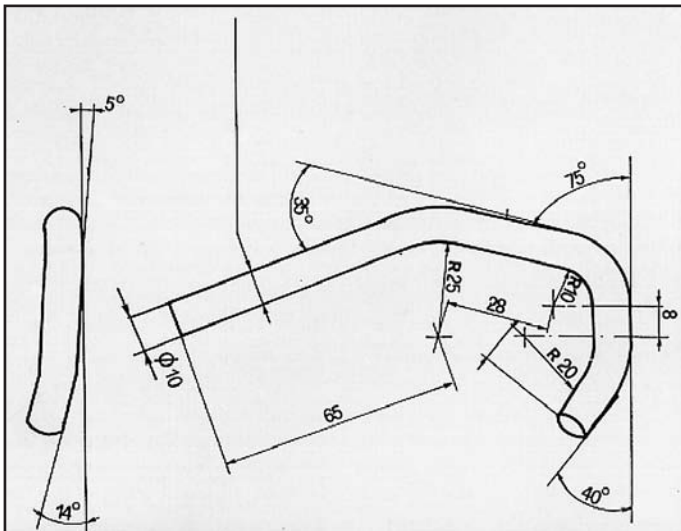
CRX ATTACCO per posteriore COD. AT 280502
