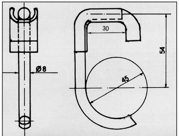
CORSA ATTACCO per centrale COD. AT 520304
