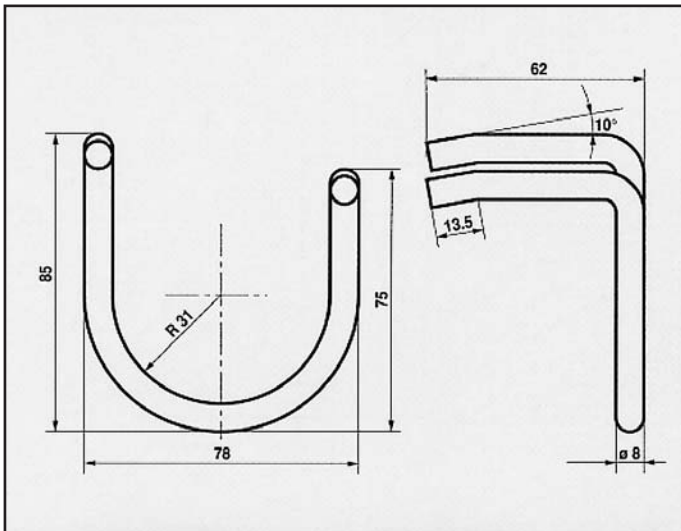
RENAULT SUPER 5 GT Turbo 1400/85-86 ATTACCO per centrale COD. AT 600116
