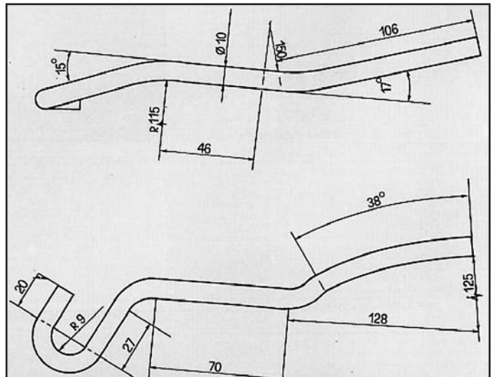
626 ATTACCO per anteriore dx COD. AT 420509
