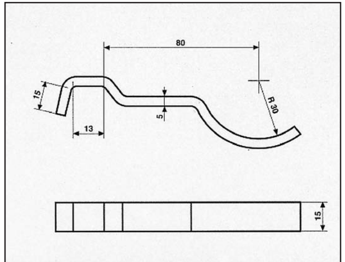
DEDRA 2000 TURBO DIESEL ATTACCO per centrale COD. AT 380802
