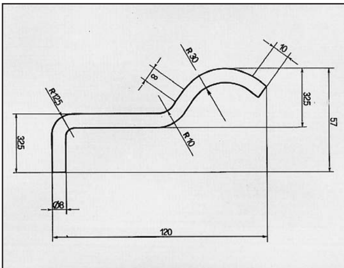
ESCORT 1100-1300/82 RINFORZO per centrale COD. R 260201 6104207 6128785
