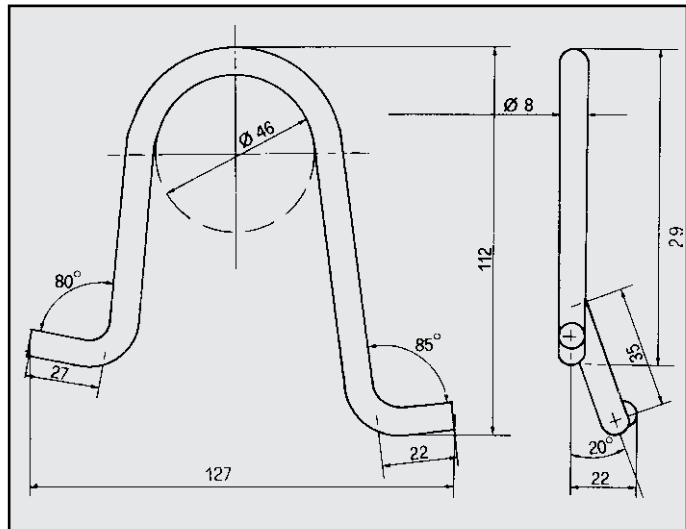
AUDI 100 RINFORZO per centrale COD. R 040101
