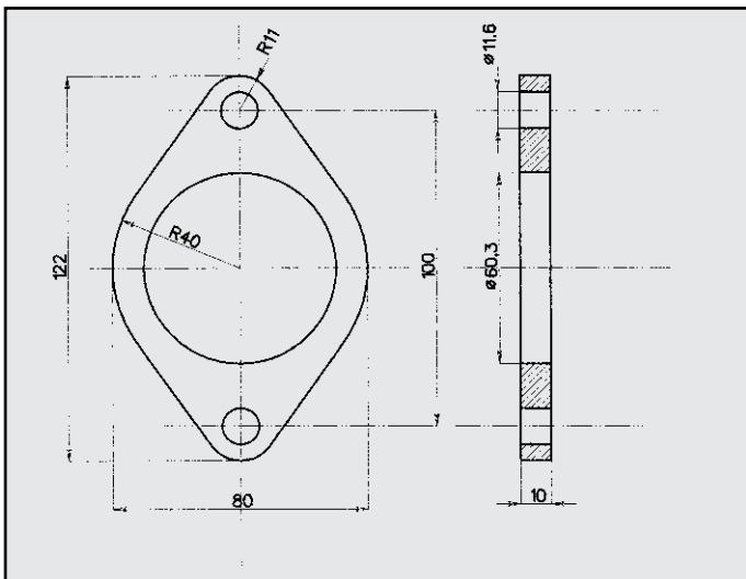
FORD FLANGIA COD. FL 260029
