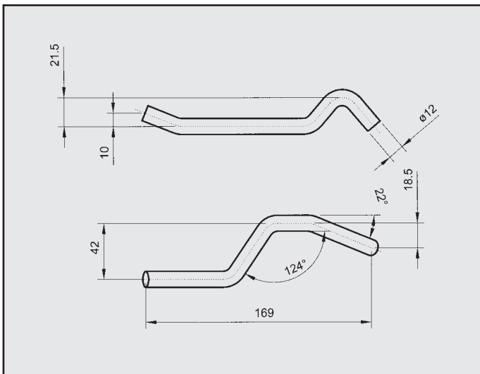
SAAB 900 2.0 16V ATTACCO per centrale COD. AT 640206
