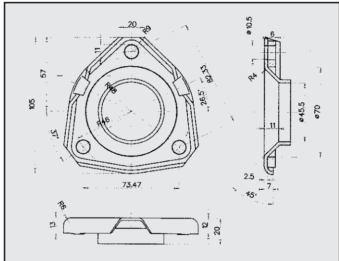
PEUGEOT 206 FLANGIA COD. FL 541212
