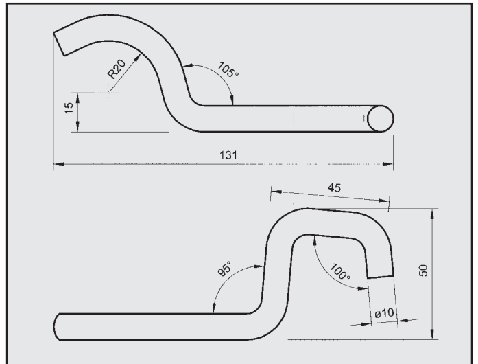
HONDA CIVIC COUPE' ATTACCO per posteriore COD. AT 280424
