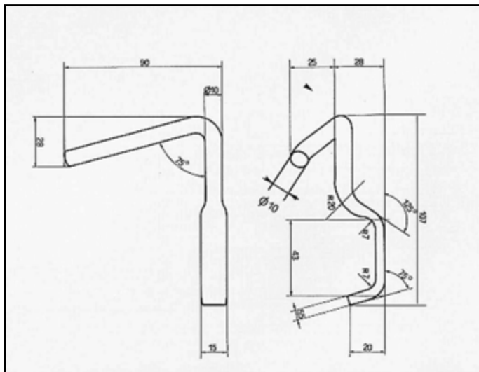
REGATA 2° ATTO 1600 BENZINA / 1900 DIESEL ATTACCO marmitta centrale COD. AT 241112
