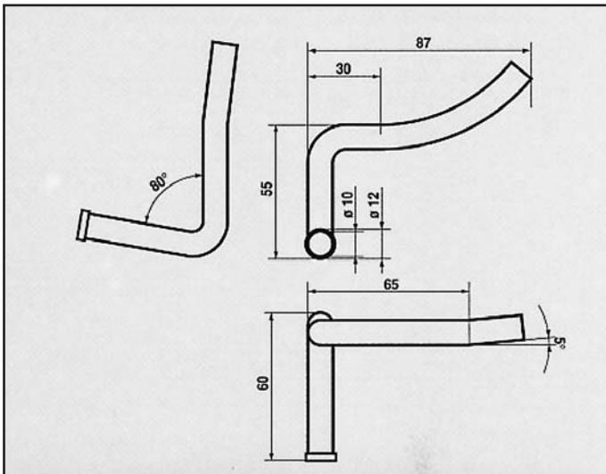
MAZDA 1.6 iniezione /1989 ATTACCO per posteriore COD. AT 420701
