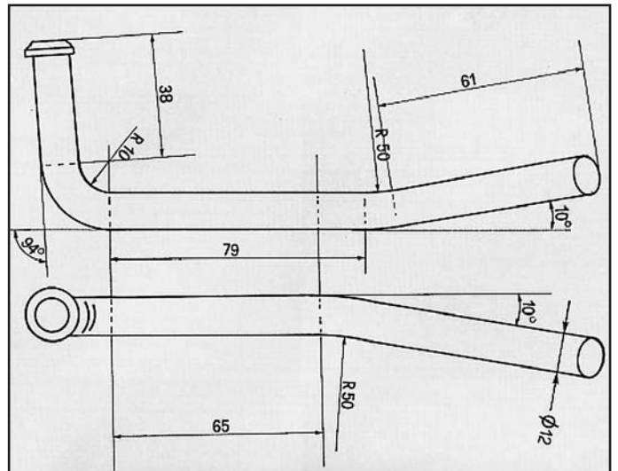
NEW CELICA ATTACCO per posteriore COD. AT 800302
