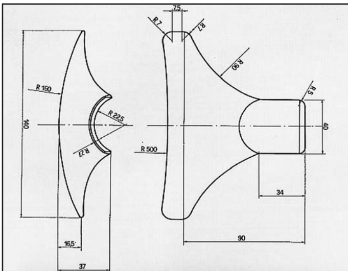
GOLF 1500-1600 BENZINA E DIESEL RINFORZO per posteriore COD. R 860103
