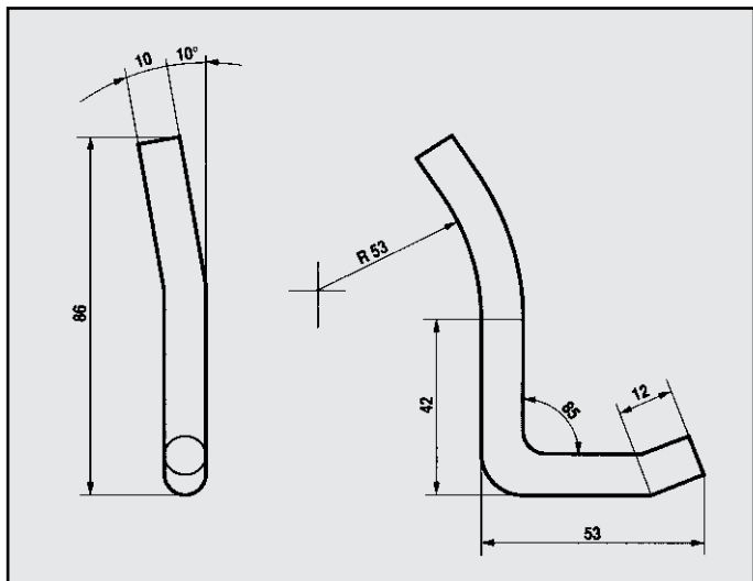
DAIHATSU CHARADE GTI-1987 ATTACCO per posteriore COD. AT 180201
