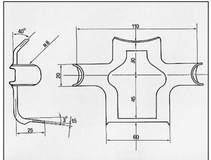
ASCONA MANTA ATTACCO per centrale COD. AT 520204
