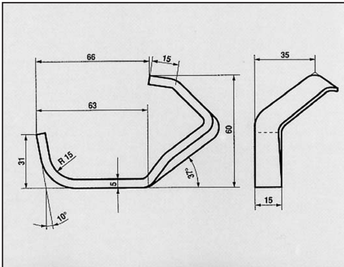
SEAT MALAGA 1500 iniezione/87 ATTACCO per posteriore COD. AT 680503
