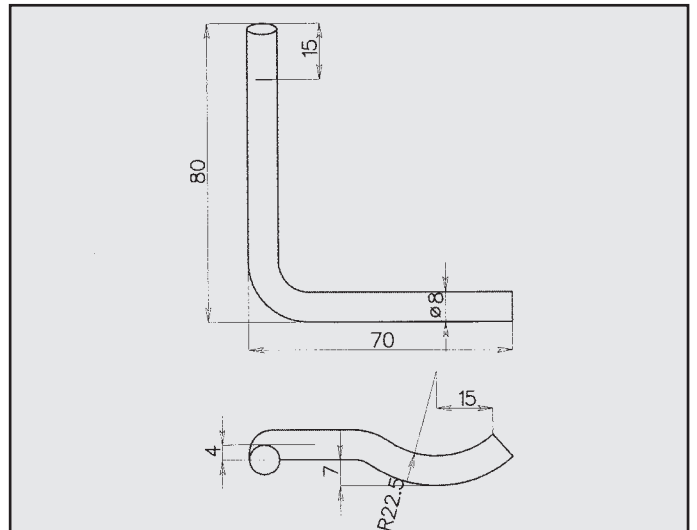
TICO ATTACCO POSTERIORE COD. AT 790004
