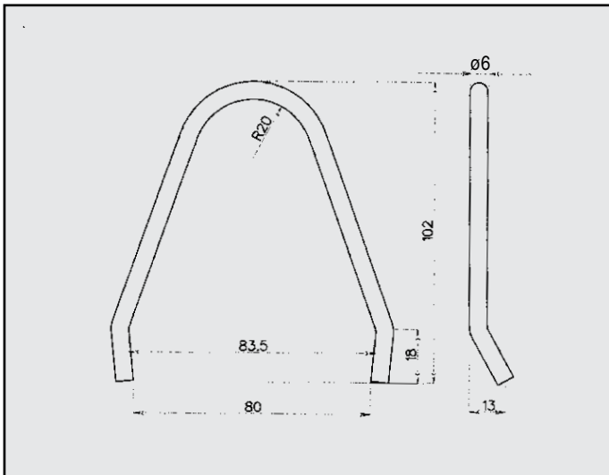
FIAT PANDA RINFORZO COD. R 240116
