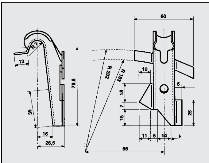
AUDI 80 mod. 91/92 ATTACCO COD. AT 040309
