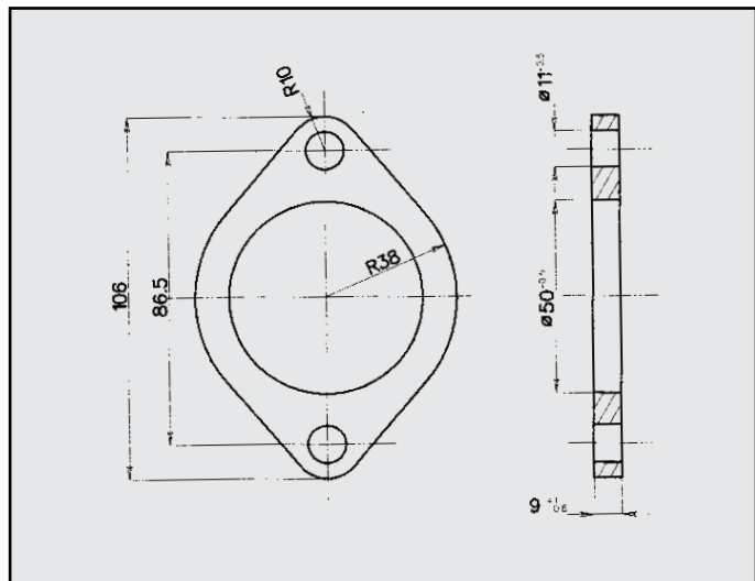
RENAULT CLIO FLANGIA COD. FL 601315
