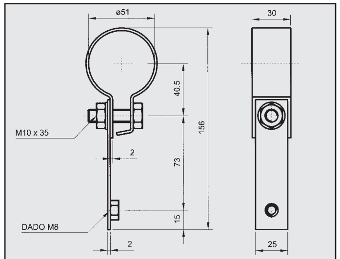
NISSAN BLUE BIRD 1.8 ATTACCO FASCETTA per posteriore COD. AT 500503
