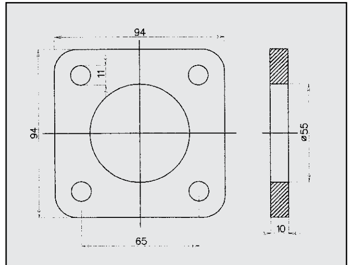
FIAT CROMA 2.0 FLANGIA COD. FL 242904
