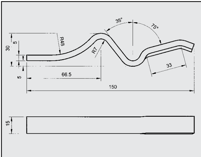
FIAT UNO D. ATTACCO COD. AT 240914
