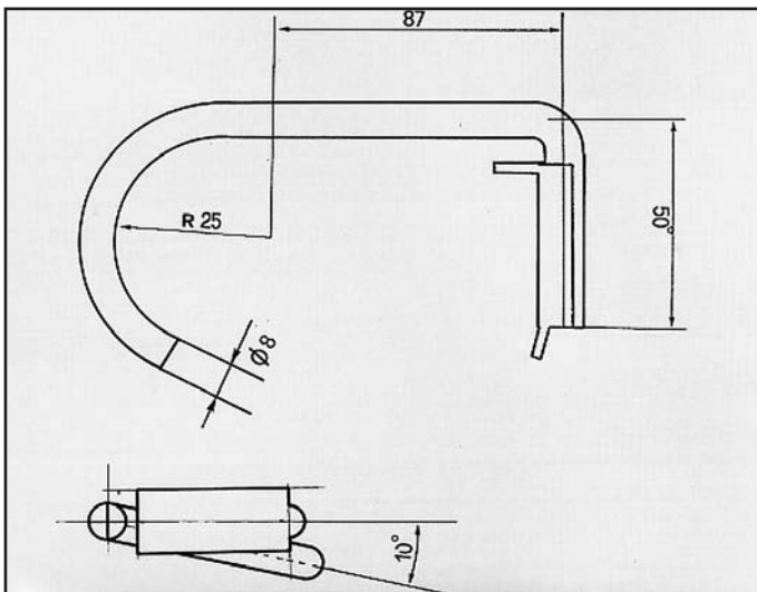
TAUNUS ATTACCO per posteriore COD. AT 260703
