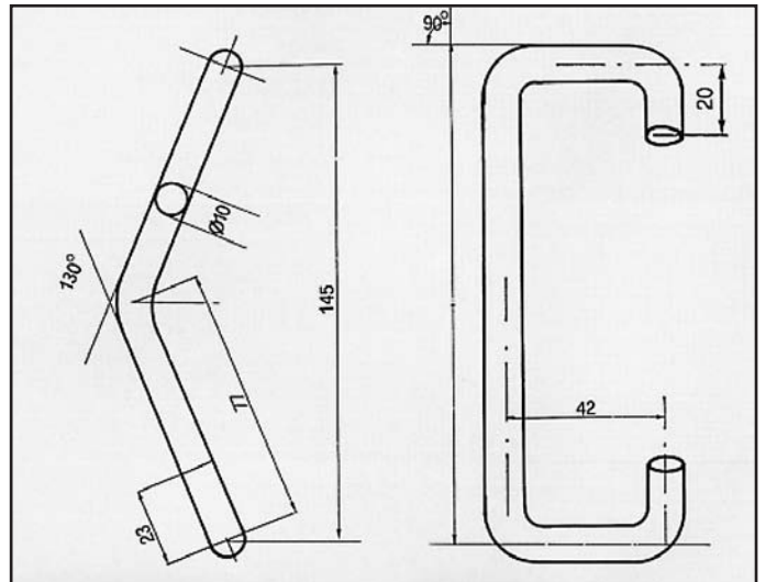
CIVIC/CRX ATTACCO per centrale COD. AT 280411
