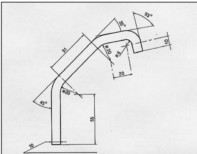
CIVIC ATTACCO per posteriore COD. AT 280403
