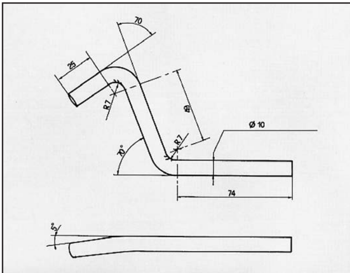
CELICA ATTACCO per posteriore COD. AT 800202
