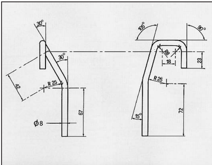
COROLLA 3KC ATTACCO per posteriore COD. AT 800407
