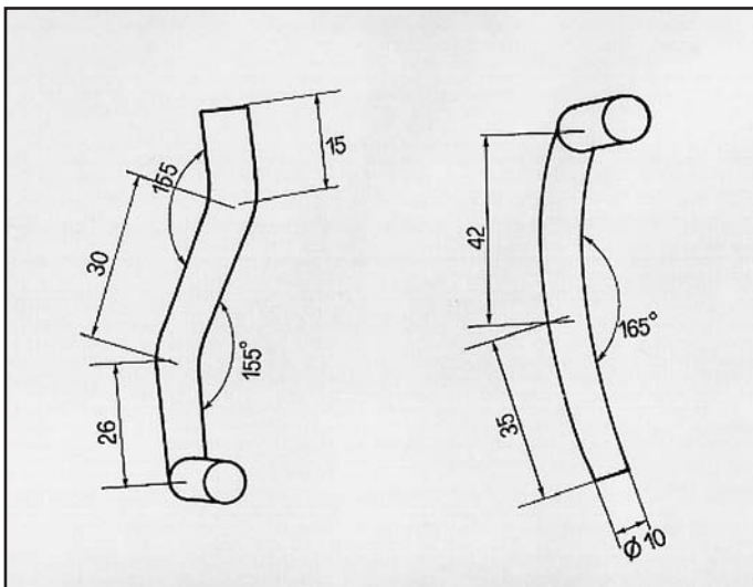
R 19 CHAMADE ATTACCO per centrale COD. AT 600905
