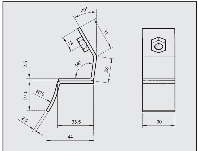
NISSAN MICRA ATTACCO per posteriore COD. AT 500208
