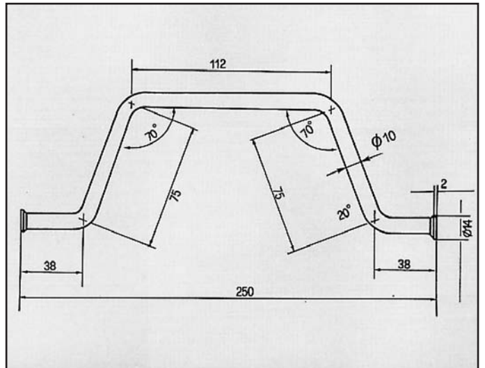
626 2000 16V ATTACCO posteriore anteriore COD. AT 420514
