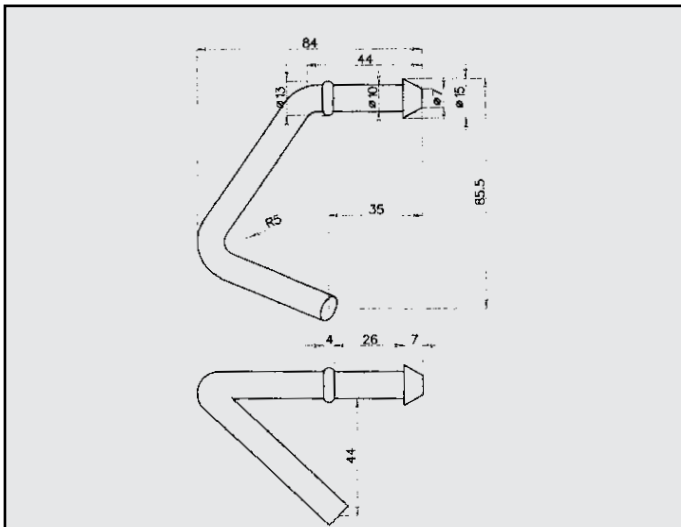
DAEWOO NUBIRA ATTACCO SUPERIORE ANTERIORE COD. AT 160302
