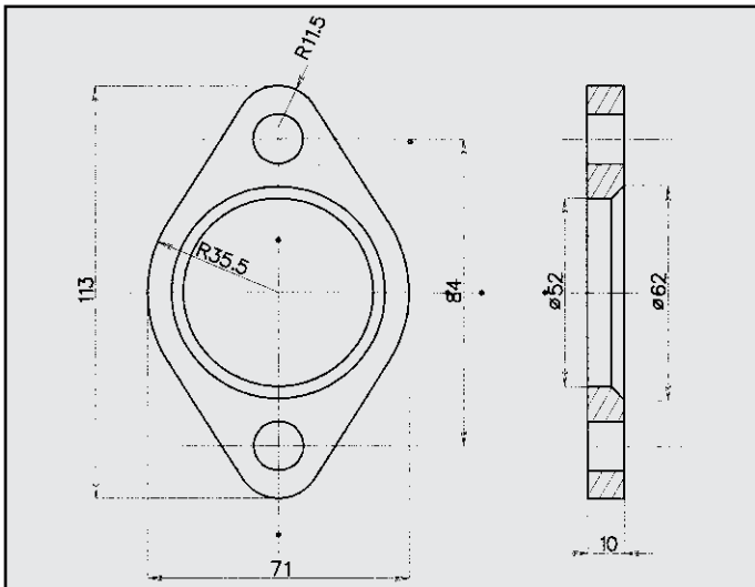
RENAULT FLANGIA COD. FL 600003
