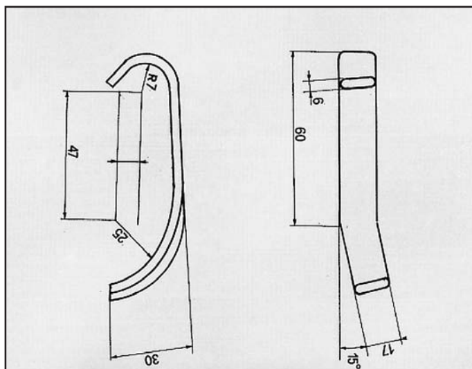
OPEL MONZA ATTACCO per posteriore COD. AT 520702
