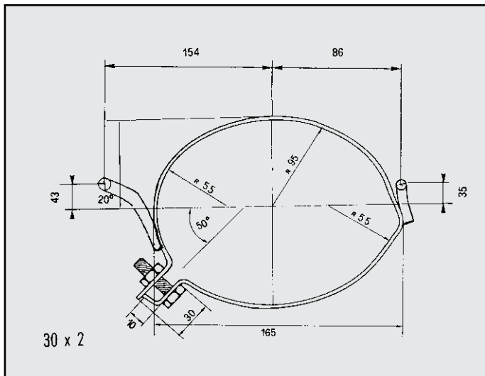
PEUGEOT 205 FASCETTA per barilotto COD. F 540302
