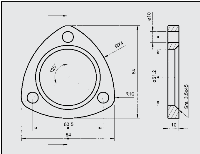
ALFA 164 2.0 TS 90 FLANGIA COD. FL 020903
