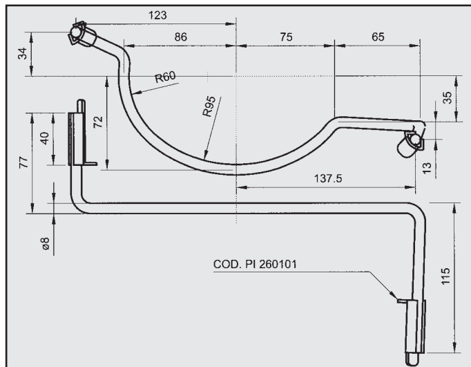
PEUGEOT 306 ATTACCO (Sostituisce COD. F 540901) COD. AT 540905
