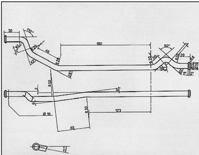
626 ATTACCO per posteriore COD. AT 420506
