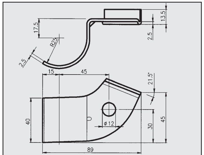
RENAULT R25 2000 DIESEL BENZINA ATTACCO per tubo centrale COD. AT 601501
