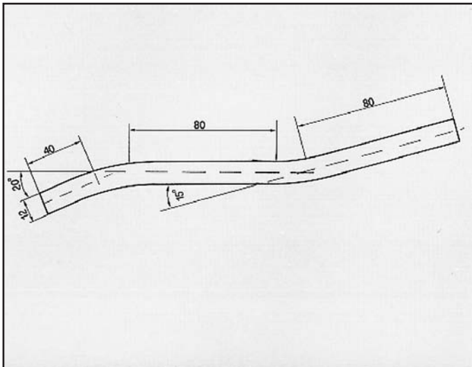
PRISMA 1600 ATTACCO per posteriore COD. AT 380309
