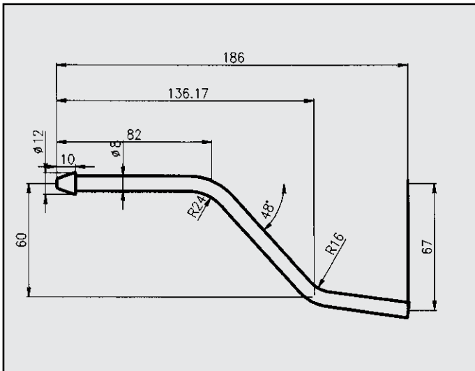
FIAT PUNTO ATTACCO COD. AT 242222
