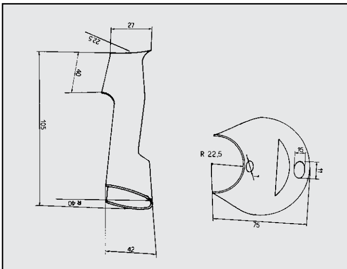
ALFETTA RINFORZO per posteriore COD. R 020202
