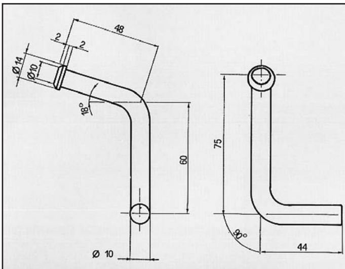
CEDRIC V30 TURBO ATTACCO per posteriore COD. AT 500102
