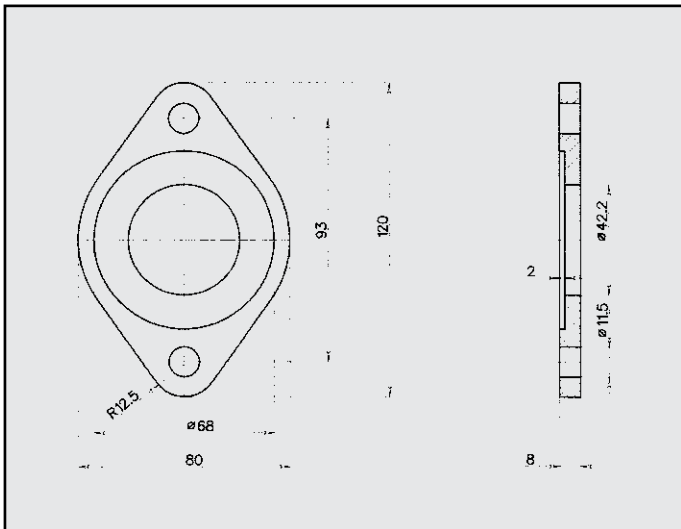
DAIHATSU FERENZA 1.6 FLANGIA COD. FL 180309
