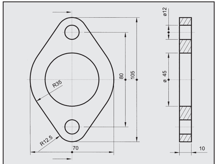
OPEL CORSA FLANGIA COD. FL 520313
