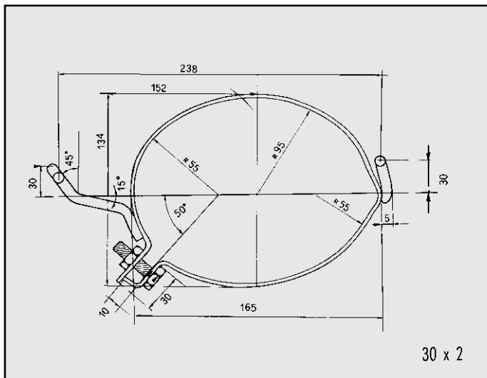
PEUGEOT 205 DIESEL 86/88 FASCETTA per barilotto COD. F 540303
