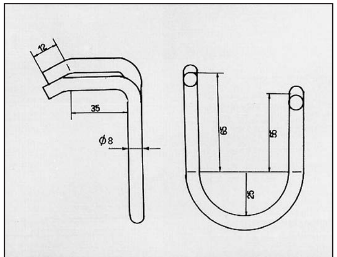
SUPER 5 - GT TURBO ATTACCO per posteriore COD. AT 600108
