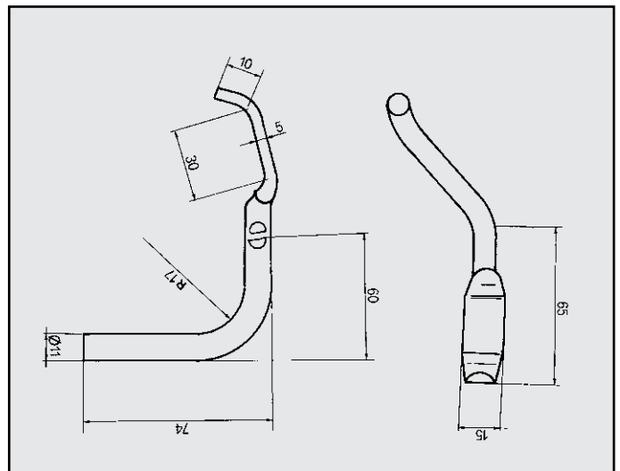
Y10 TURBO ATTACCO per posteriore COD. AT 080207
