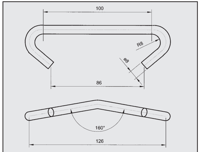
VOLVO 340 343 345 1.4 ATTACCO per centrale COD. AT 880104
