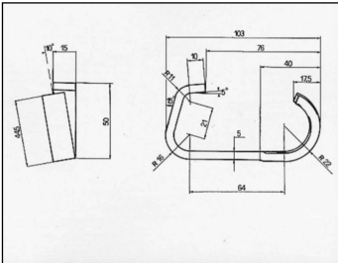
PANDA 750 YOUNG ATTACCO per posteriore COD. AT 240110
