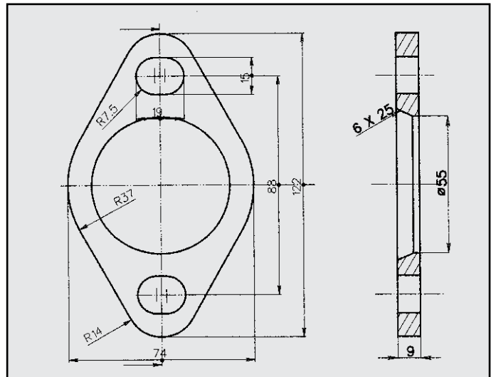
FIAT UNO FLANGIA COD. FL 240921
