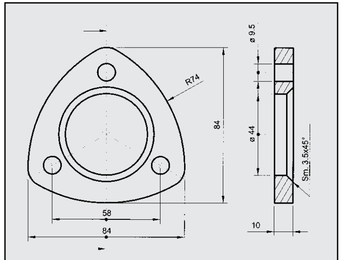
BMW 320i FLANGIA COD. FL 120109
