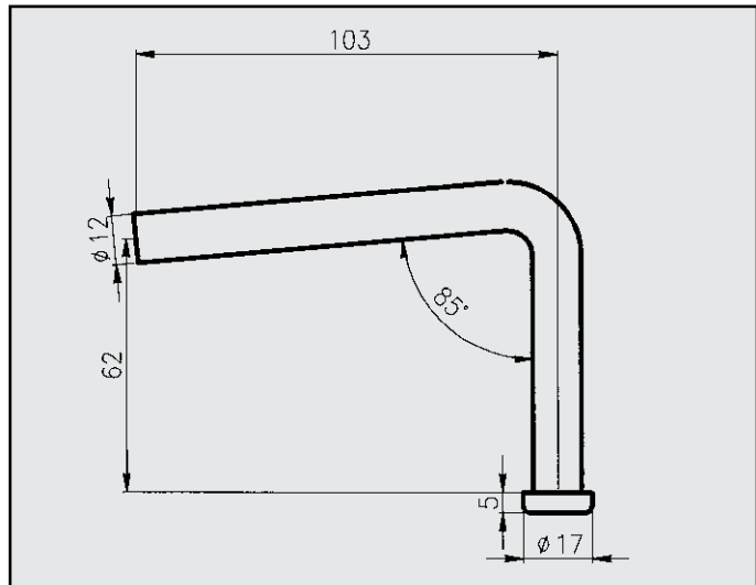
FIAT MULTIPLA ATTACCO COD. AT 242607
