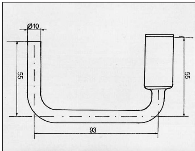
SIERRA 1800/2000 ATTACCO per centrale COD. AT 260611 6162050 1643406
