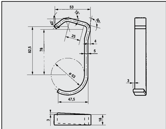
FIAT TIPO 1.9 TD ECO 94 ATTACCO posteriore COD. AT 241713 6766-7740611
