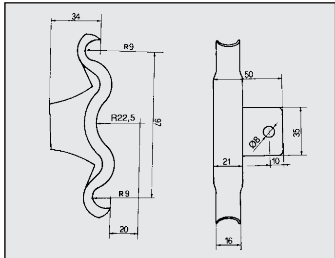
ALFASUD 3ª serie SUPPORTO per attacco COD. AT 020105
