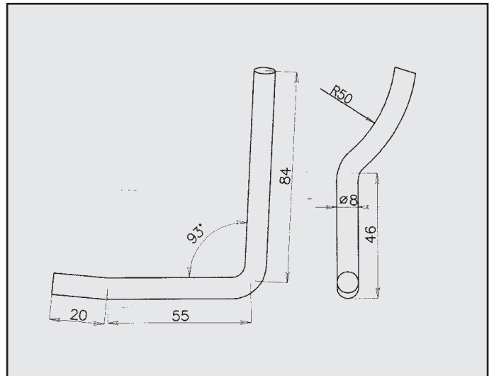
PEUGEOT 1.3 ATTACCO POSTERIORE COD. AT 540306
