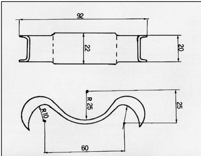
R12 ATTACCO per posteriore COD. AT 600301
