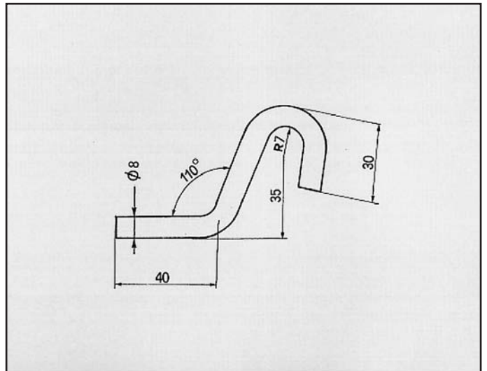
3500 V8 ATTACCO per centrale COD. AT 620102
