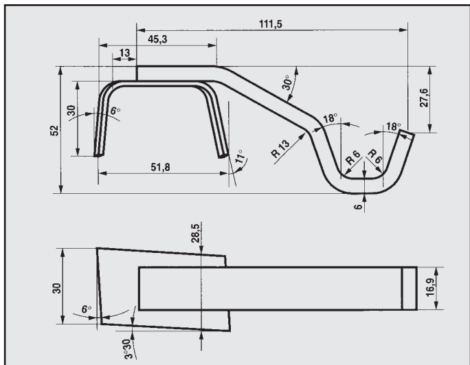
LANCIA DEDRA ATTACCO centrale COD. AT 380810
