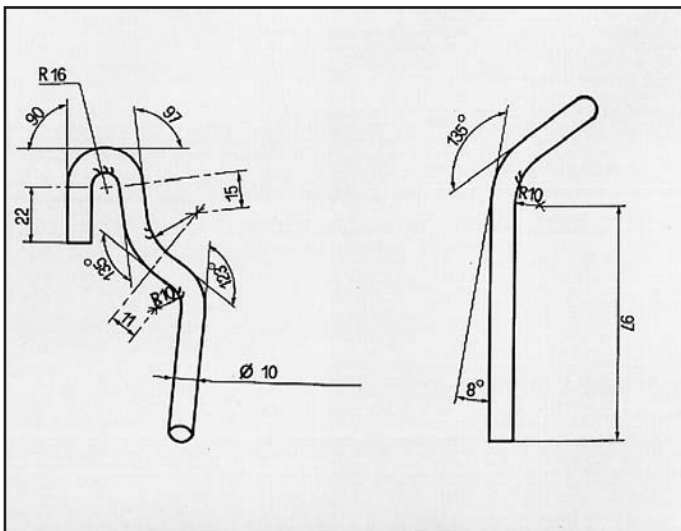
CELICA 20R ATTACCO per posteriore COD. AT 800203
