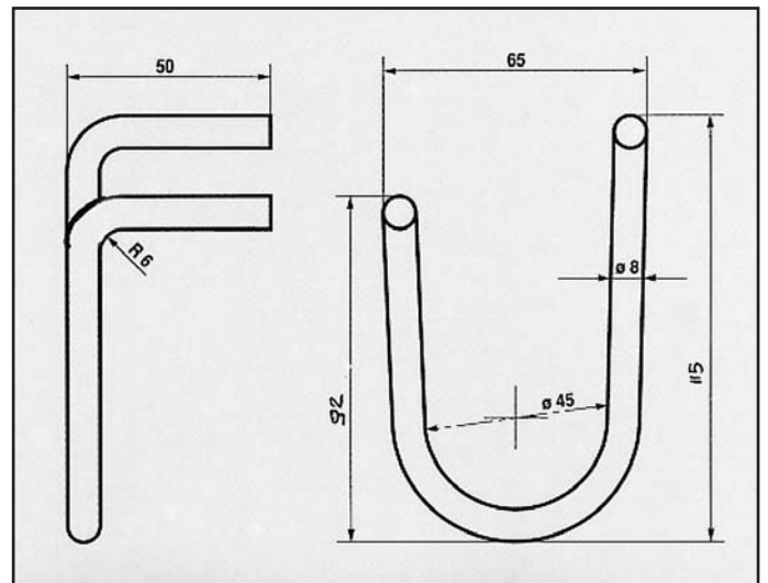
SEAT IBIZA 1400-1600 ATTACCO per posteriore COD. AT 680108
