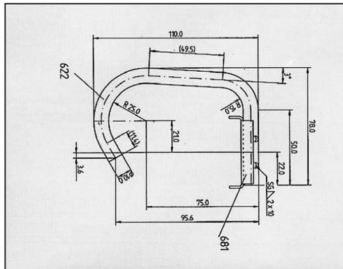
VECTRA 1400-1600 ATTACCO anteriore per posteriore COD. AT 520802
