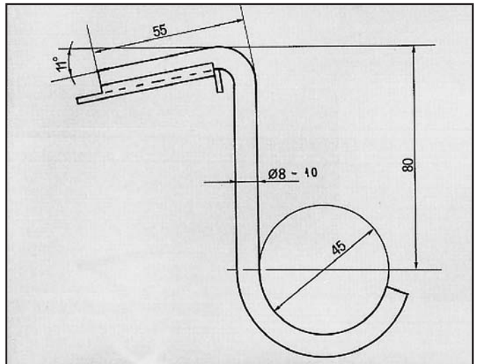
ASCONA ATTACCO per posteriore COD. AT 520201/B
