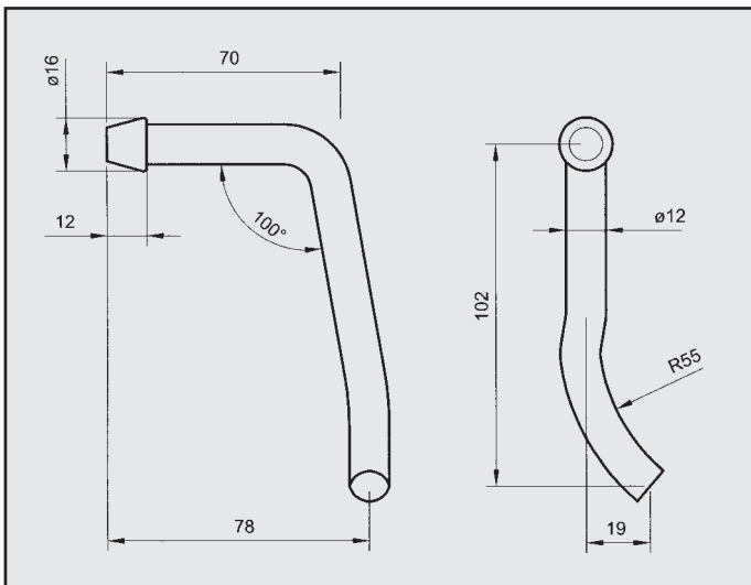
NISSAN PRIMERA 2.0 D. ATTACCO SX per posteriore COD. AT 500409
