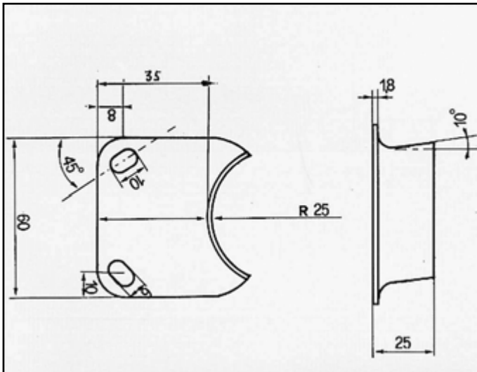
132 INIEZIONE ATTACCO per centrale COD. AT 240703
