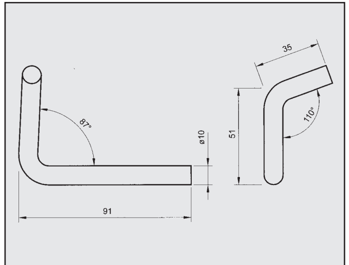
FORD MONDEO RINFORZO per posteriore COD. R 261208
