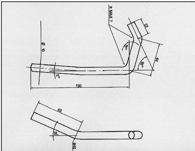
ACCORD 79-ON ATTACCO per posteriore COD. AT 280104
