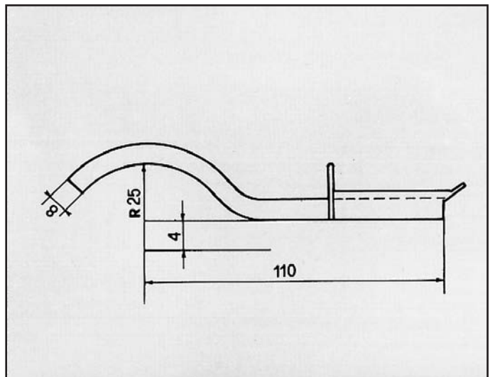
FIESTA 1100 ATTACCO per posteriore COD. AT 260302
