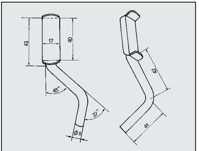
MINI METRO 1000 ATTACCO per posteriore COD. AT 060110
