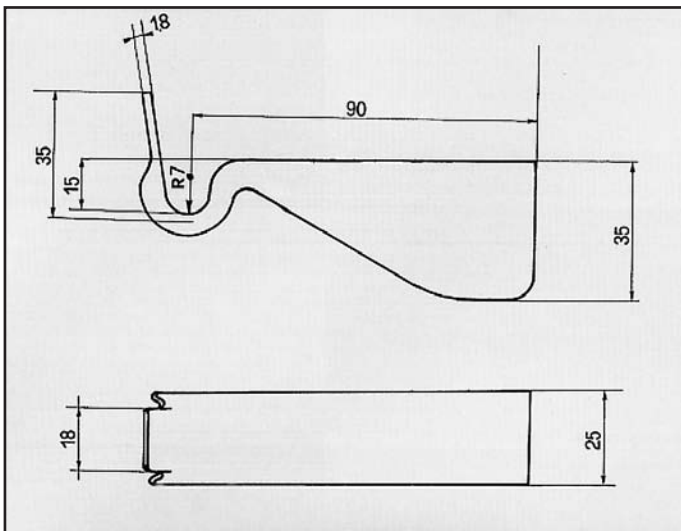
1100 SIMCA ATTACCO per posteriore COD. AT 780301
