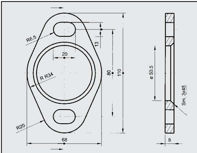
FIAT REGATA TIPO FLANGIA COD. FL 241116
