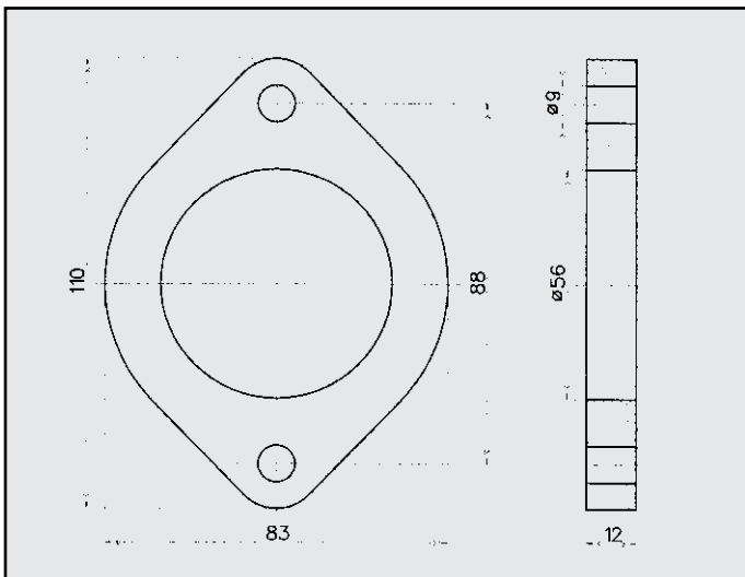
ALFA ROMEO FLANGIA COD. FL 020002
