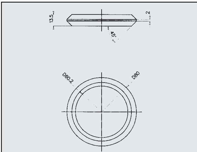
PEUGEOT 406 ANELLO COD. AN 541105
