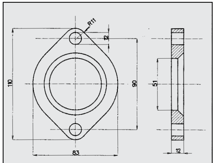
ROVER 414 FLANGIA COD. FL 620005
