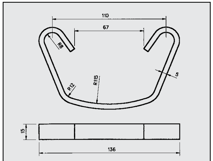
FIAT DUCATO ATTACCO per posteriore COD. AT 241502
