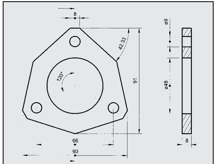
AUDI 80 DIESEL FLANGIA COD. FL 040313
