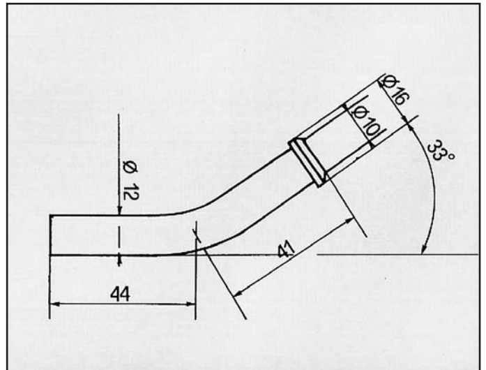
COROLLA 4ALC ATTACCO per posteriore COD. AT 800410
