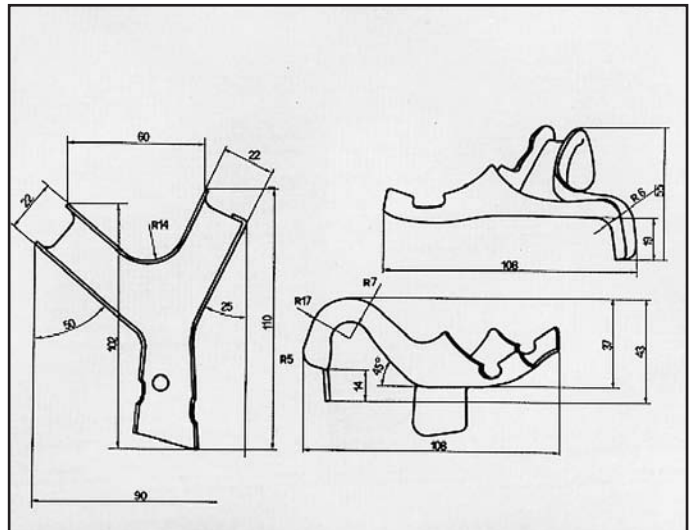
POLO 1050 ATTACCO per posteriore COD. AT 860110
