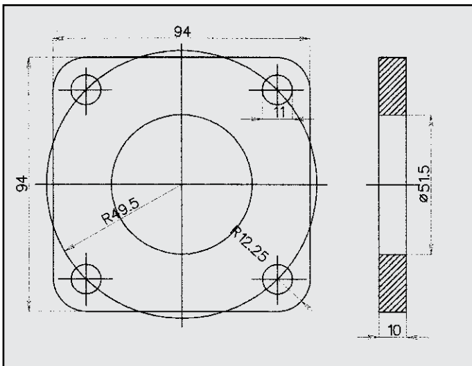
VOLKSWAGEN FLANGIA COD. FL 860028
