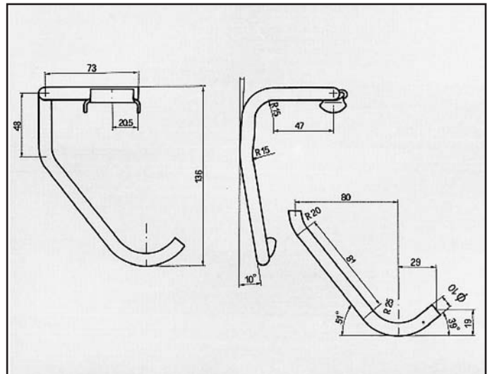
ESCORT XR3 INIEZIONE/ORION INIEZIONE ATTACCO per posteriore COD. AT 260225
