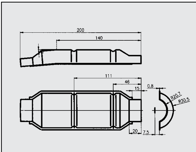
FIAT PUNTO 1.7 D PROTEZIONE CALORE COD. PC 242223
