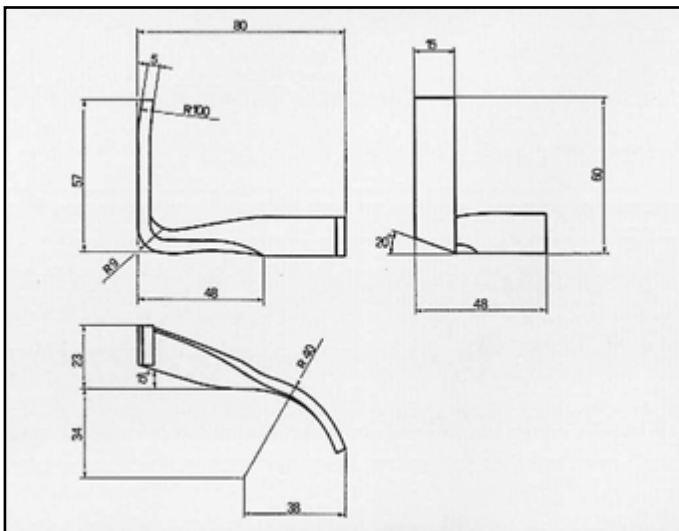
REGATA 85-100 1ª SERIE ATTACCO per posteriore COD. AT 241106
