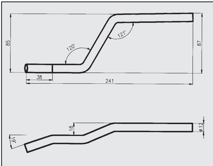
OPEL ASTRA ATTACCO per posteriore COD. AT 520923
