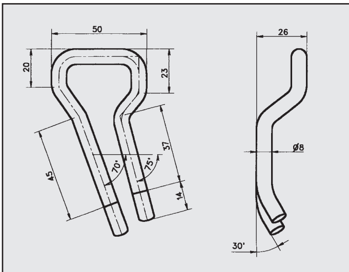
LANCIA DELTA TD 93 ATTACCO per posteriore COD. AT 380807
