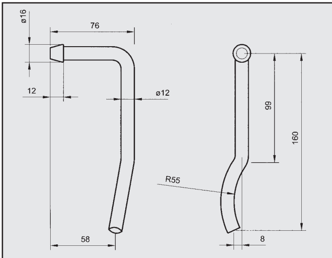
NISSAN PRIMERA 2.0 D. ATTACCO DX per posteriore COD. AT 500408
