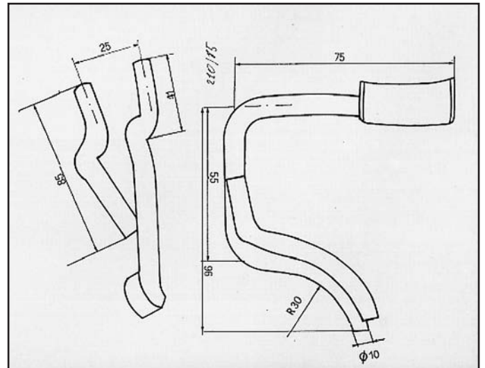
SCORPIO 2000 ATTACCO per centrale COD. AT 260801
