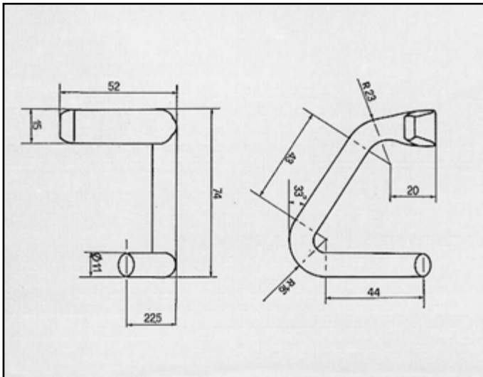
UNO TURBO IE ATTACCO per posteriore COD. AT 240906
