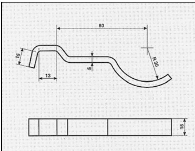
FIAT TEMPRA 1.9 TURBO DIESEL S.W. (1990) ATTACCO centrale COD. AT 241904
