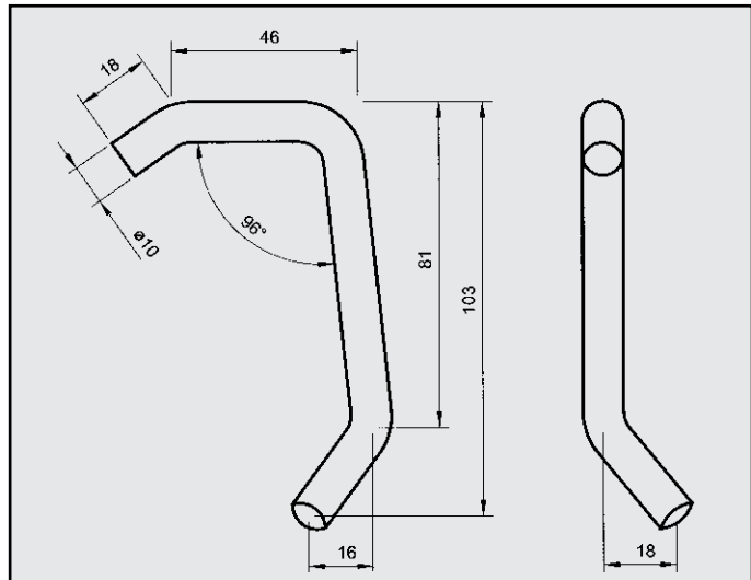
DAIHATSU FERENZA 1.6 16V 4x4 ATTACCO per posteriore COD. AT 180303 544681 544594
