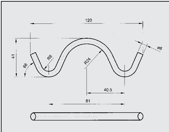
FIAT RITMO CABRIO ATTACCO centrale COD. AT 240811
