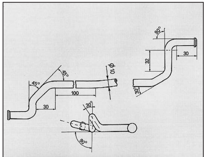
GLC 1500 ATTACCO per tubo intermedio COD. AT 420302
