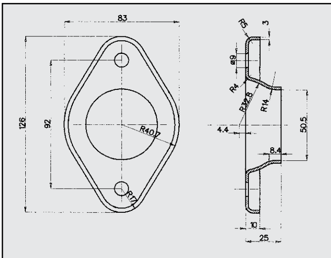
BMW FLANGIA COD. FL 120019
