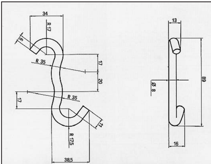
R14 ATTACCO per posteriore COD. AT 600401
