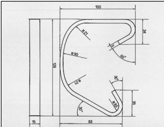
DUCATO TURBO DIESEL ATTACCO per posteriore COD. AT 241503
