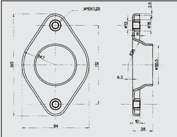
TOYOTA FLANGIA COD. FL 800005
