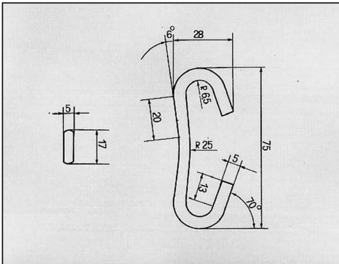
MINI 3 CILINDRI ATTACCO per centrale COD. AT 320102
