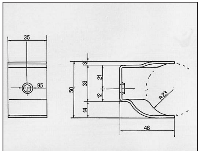
DELTA 1500 ATTACCO per centrale COD. AT 380302
