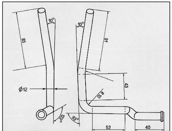
NEW CELICA ATTACCO per posteriore COD. AT 800303
