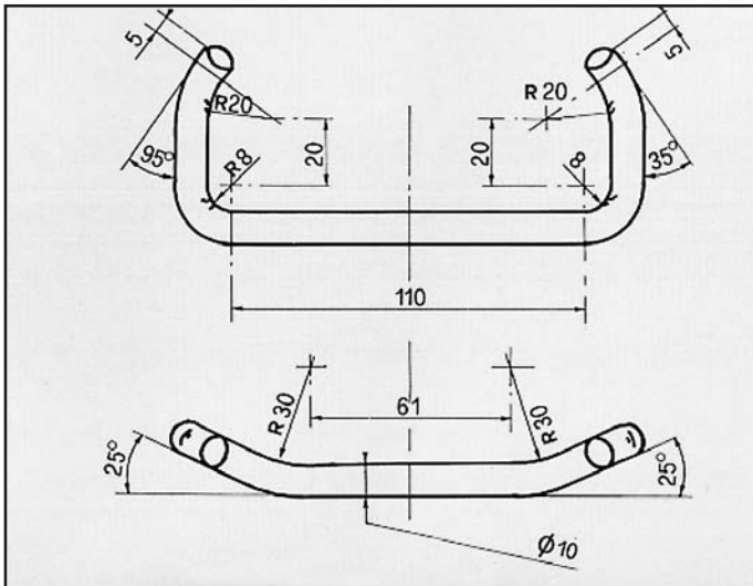
CIVIC 1500 ATTACCO per centrale COD. AT 280407
