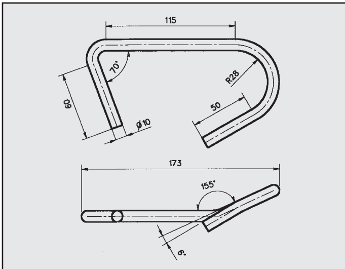
VOLKSWAGEN FOX ATTACCO per posteriore COD. AT 860501
