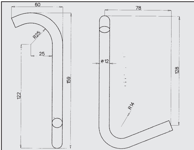
MERCEDES CLASSE C ATTACCO COD. AT 441001
