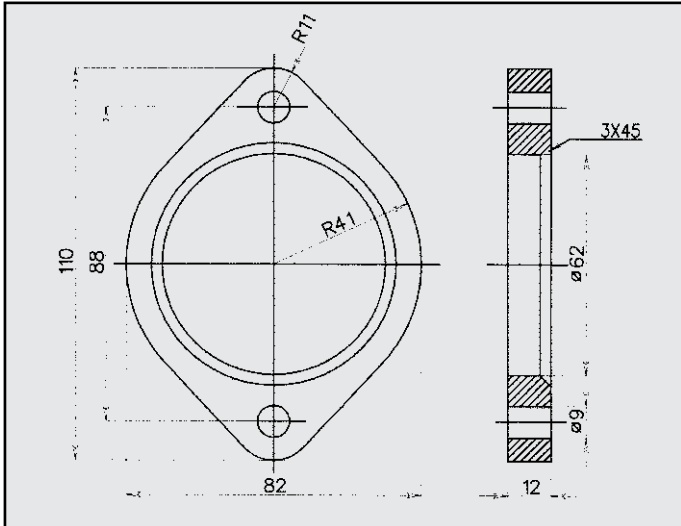
SAAB FLANGIA COD. FL 640002
