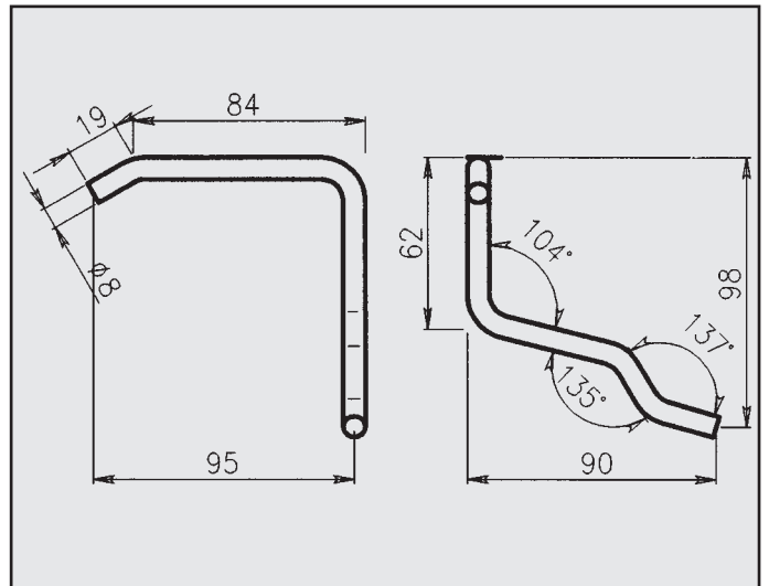
RENAULT ESPACE 2.2 ATTACCO per centrale COD. AT 601103
