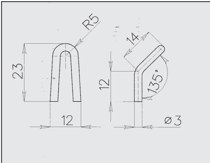
ATTACCO PER MOLLA COD. AT 010001
