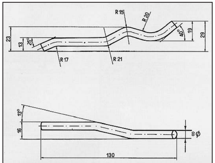
R18 ATTACCO per centrale COD. AT 600501
