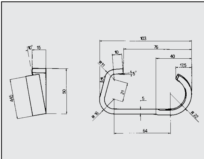
Y10 FIRE ATTACCO per posteriore COD. AT 080203
