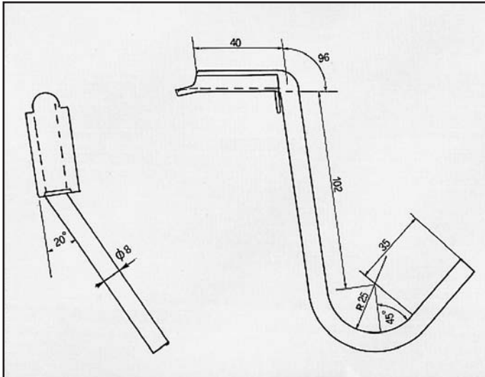
ESCORT 1100/83 ATTACCO per posteriore COD. AT 260228
