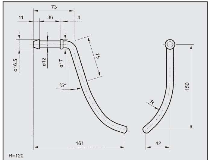
LANCIA ATTACCO COD. AT 380901
