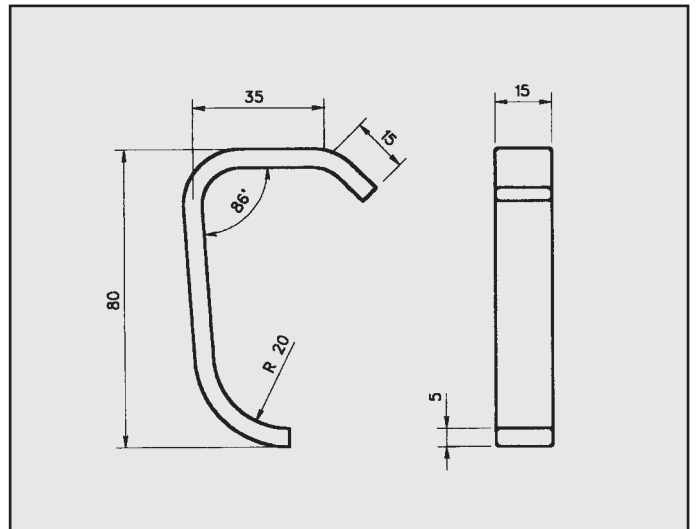
SEAT RONDA ATTACCO per posteriore COD. AT 680201
