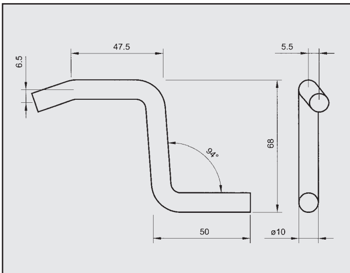
ROVER 414 ATTACCO per posteriore COD. AT 620901
