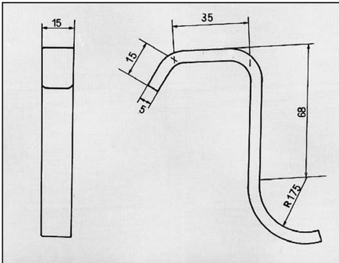
TERRA ATTACCO per tubo uscita posteriore COD. AT 680401
