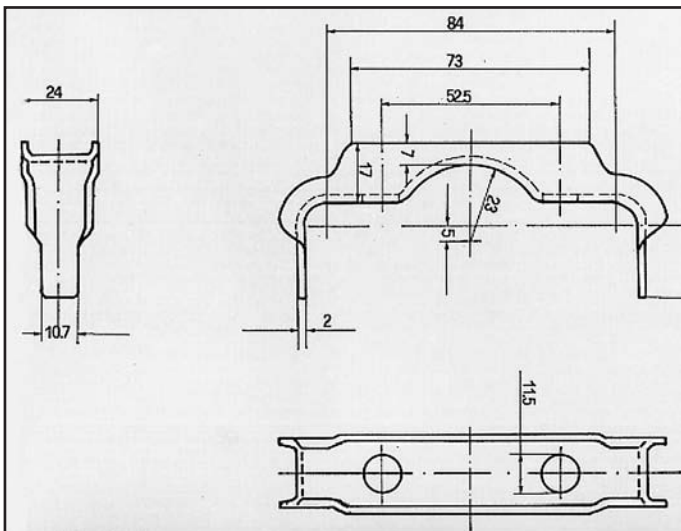
GOLF 1500-1600 BENZINA/DIESEL ATTACCO per posteriore COD. AT 860104
