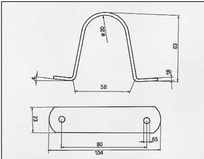
R5 ATTACCO per posteriore COD. AT 600102
