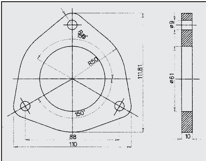
FIAT MAREA 1.9D 55KW FLANGIA COD. FL 242816
