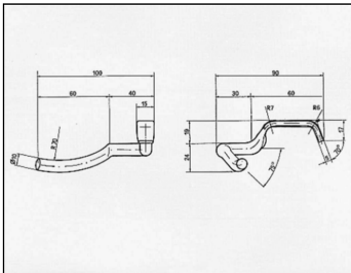
REGATA 2° ATTO 1600 TURBO DIESEL ATTACCO marmitta centrale COD. AT 241111
