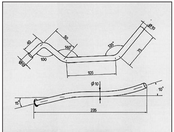
323 ATTACCO centrale COD. AT 420601
