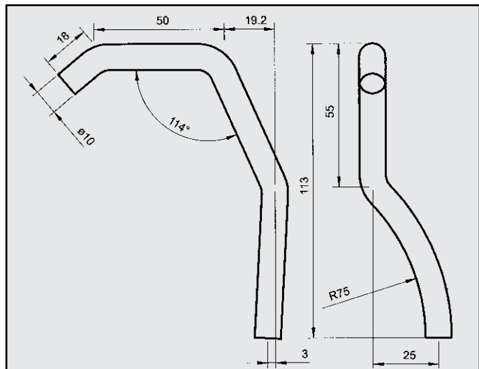
DAIHATSU FERENZA ATTACCO per posteriore COD. AT 180305
