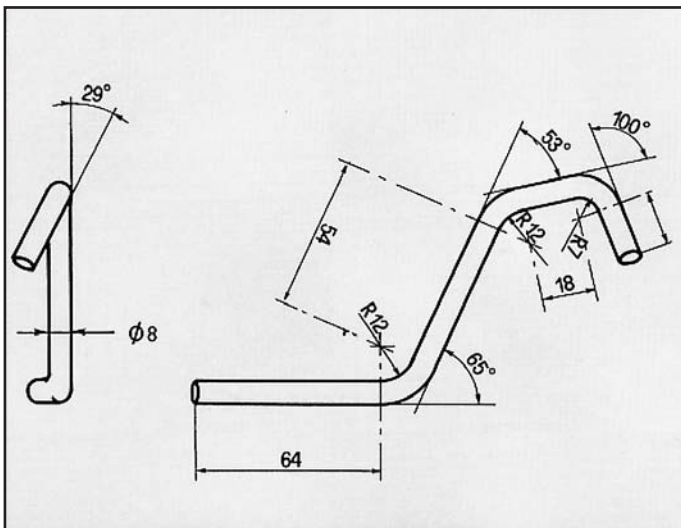
COROLLA 3KC ATTACCO per posteriore COD. AT 800408
