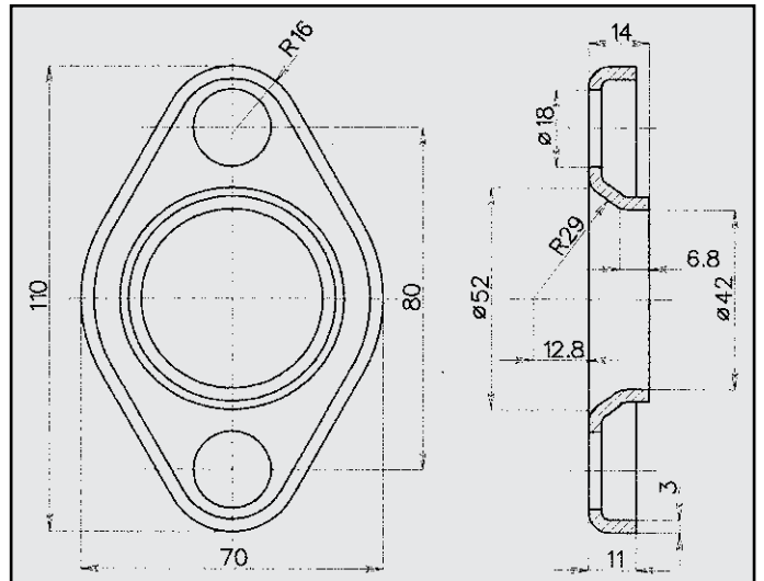
TICO FLANGIA COD. FL 790004
