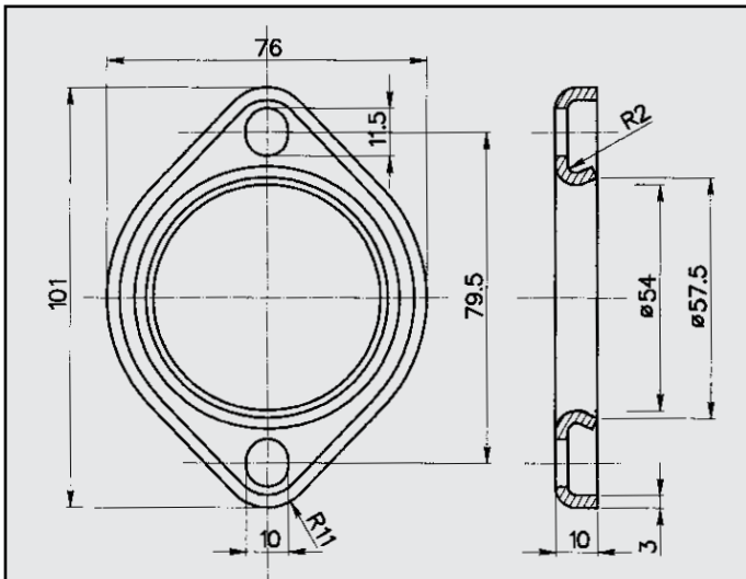
MERCEDES 200D FLANGIA COD. FL 440012
