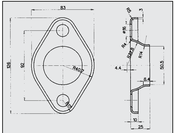
BMW FLANGIA COD. FL 120020
