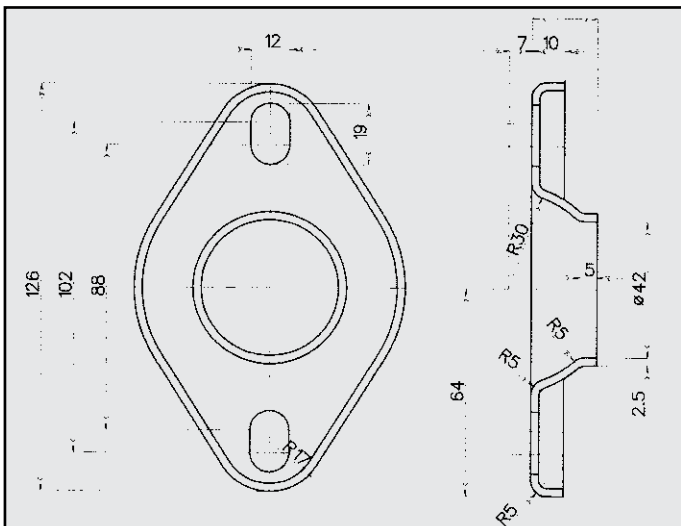
CITROEN C2 FLANGIA COD. FL 141504
