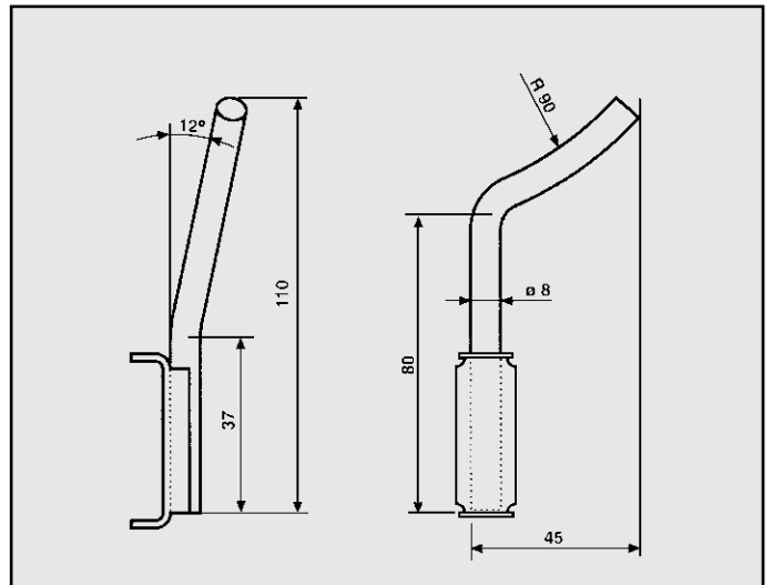
AUSTIN MONTEGO 1300 ATTACCO CENTRALE COD. AT 060401
