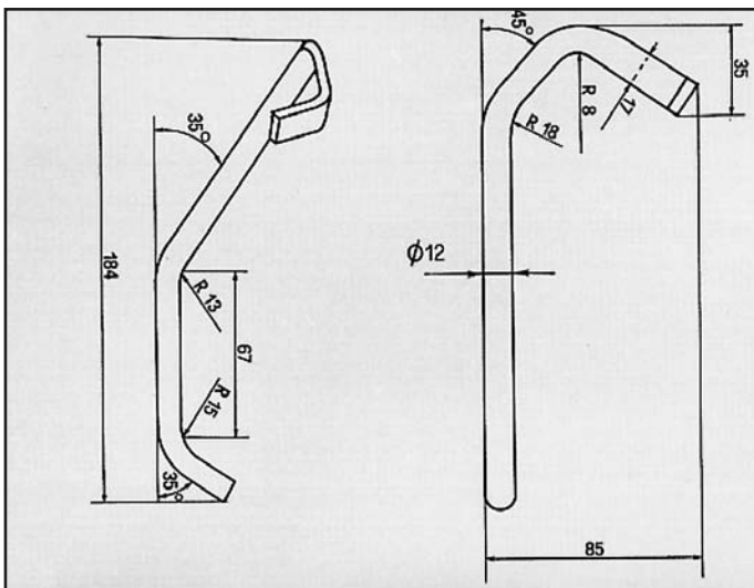
280 S-SE ATTACCO COD. AT 440402
