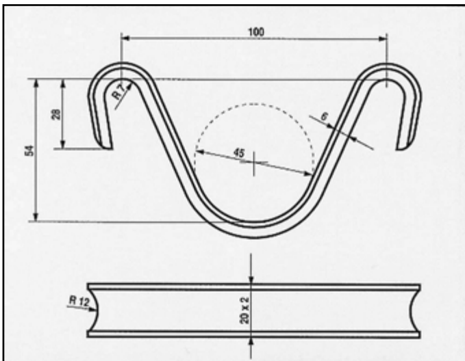
FIAT TALENTO DIESEL 1988 RINFORZO per posteriore COD. AT 242002
