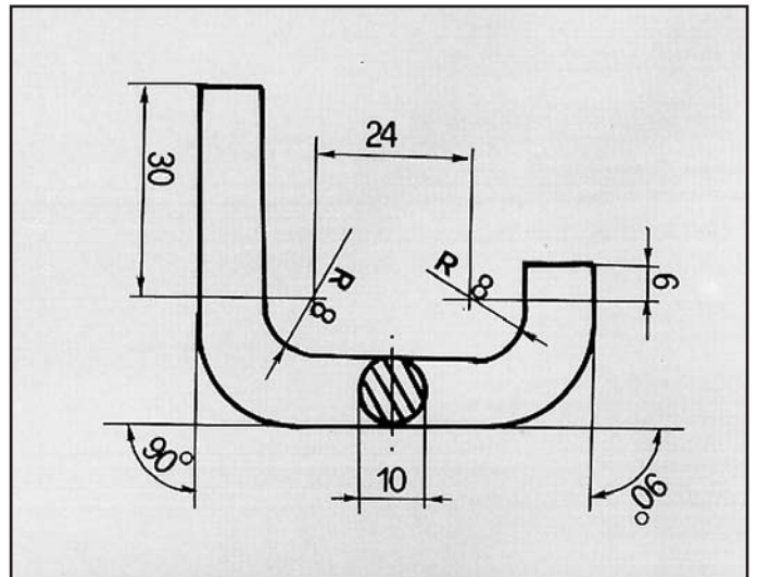
ACCORD 1800 ATTACCO per posteriore COD. AT 280101
