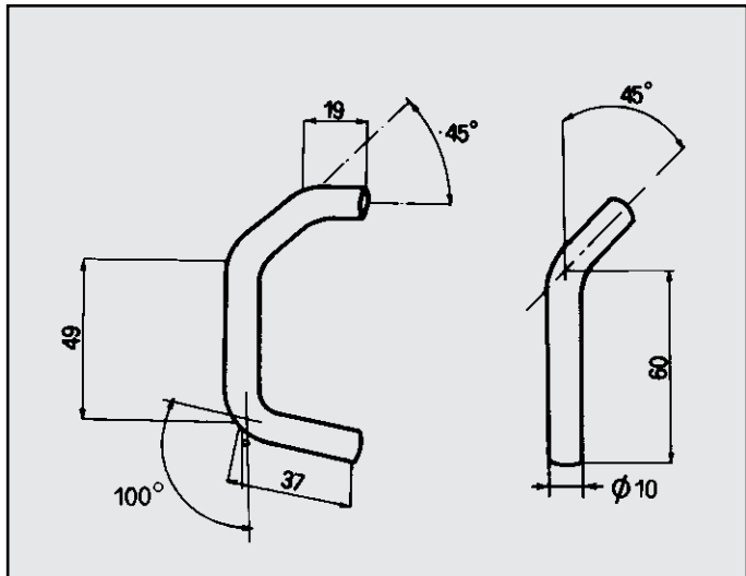
MIRA TURBO ATTACCO per posteriore COD. AT 180101
