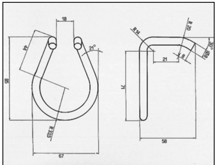
REGATA 70 ATTACCO per posteriore COD. AT 241103
