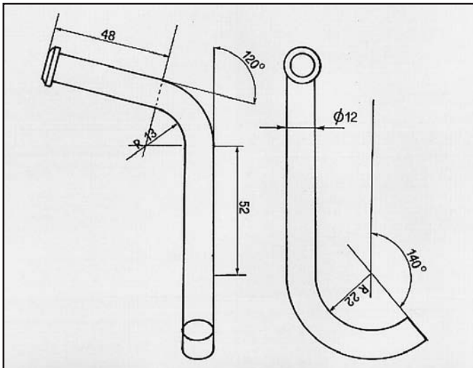
CAMRY 2 ATTACCO per centrale COD. AT 800104
