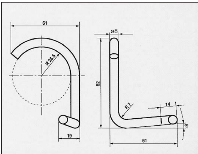
RENAULT SUPER 5 GT Turbo 1400/87 ATTACCO per posteriore COD. AT 600117
