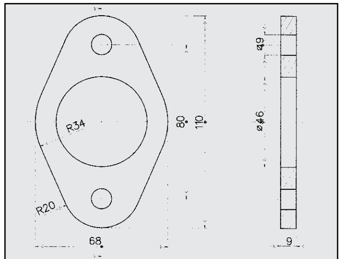
FIAT UNO FLANGIA COD. FL 240922
