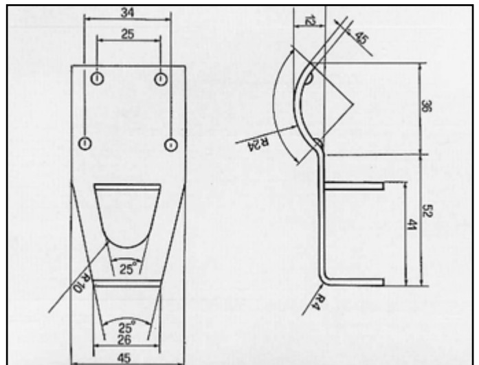
124 ATTACCO per posteriore COD. AT 241601
