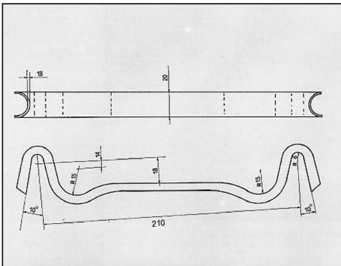
THEMA ATTACCO per tubo collettore COD. AT 380706 82412755
