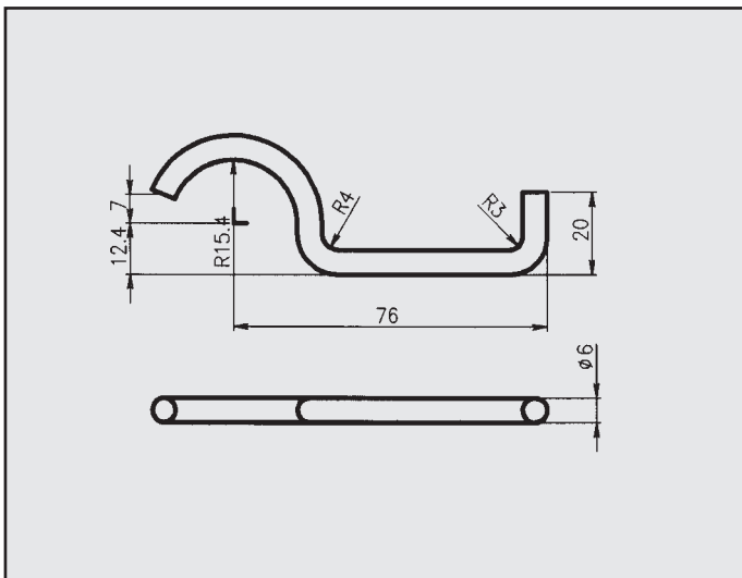
LIGIER ATTACCO posteriore COD. AT 390003
