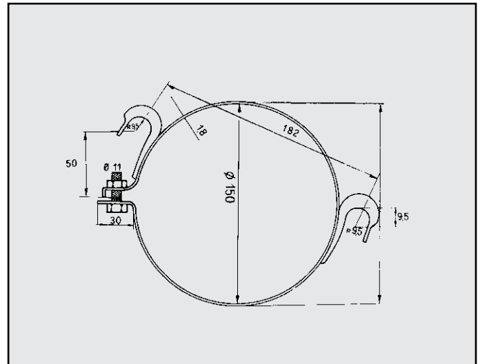
BMW 320/323 FASCETTA per posteriore COD. F 120102
