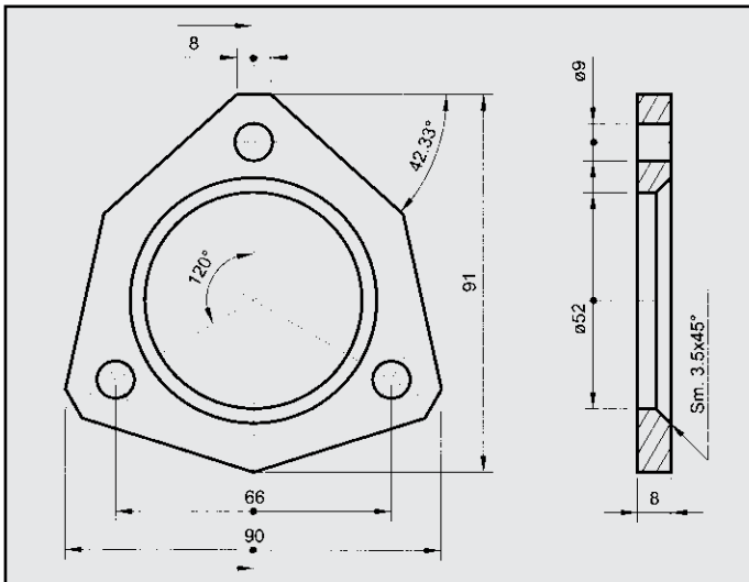
ALFA ROMEO FLANGIA COD. FL 020001
