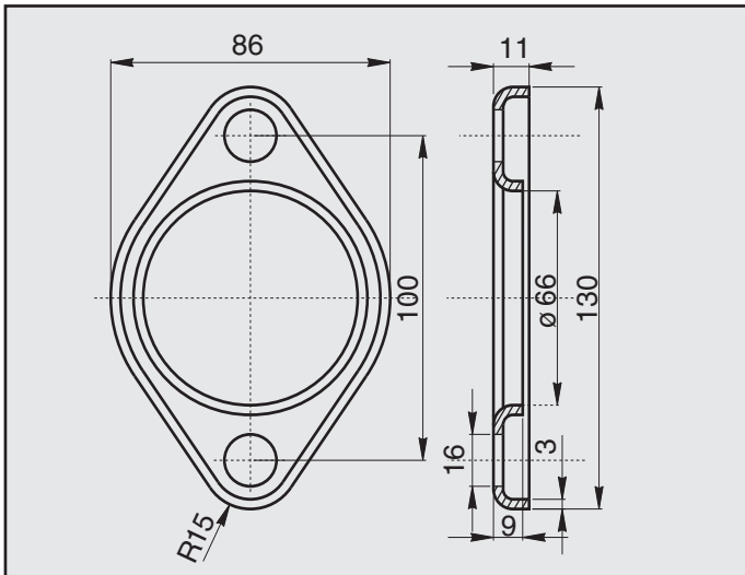
FORD ESCORT / ORION 1.6i FLANGIA COD. FL 260274
