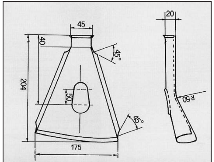
POLO 1300 DIESEL RINFORZO posteriore COD. AT 860307
