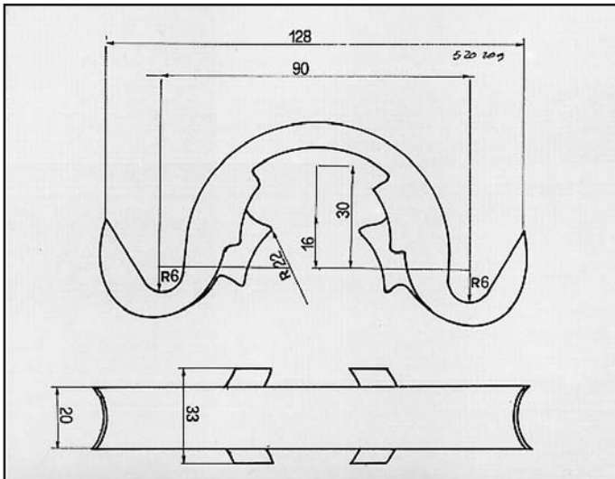
ASCONA ATTACCO per centrale COD. AT 520209
