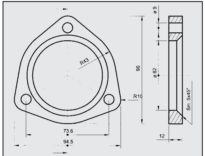
FIAT FLANGIA COD. FL 240002
