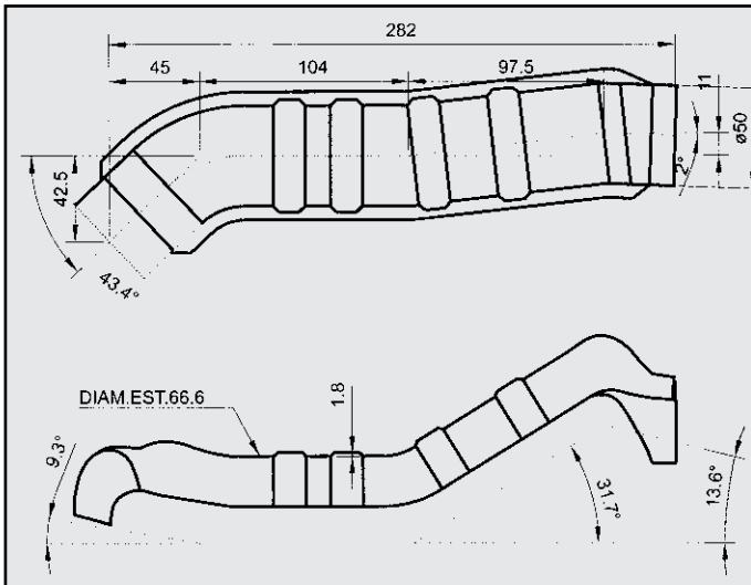
FIAT BRAVO BRAVA 1.4 '95 RINFORZO per centrale COD. PC 242302
