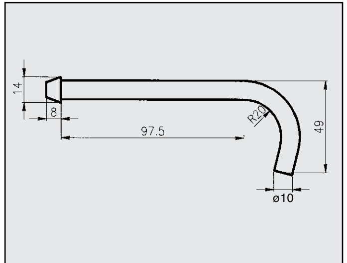
FIAT PALIO ATTACCO per centrale COD. AT 243003
