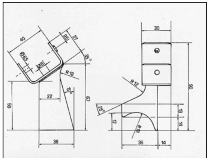
127 SPORT ATTACCO per posteriore COD. AT 240209
