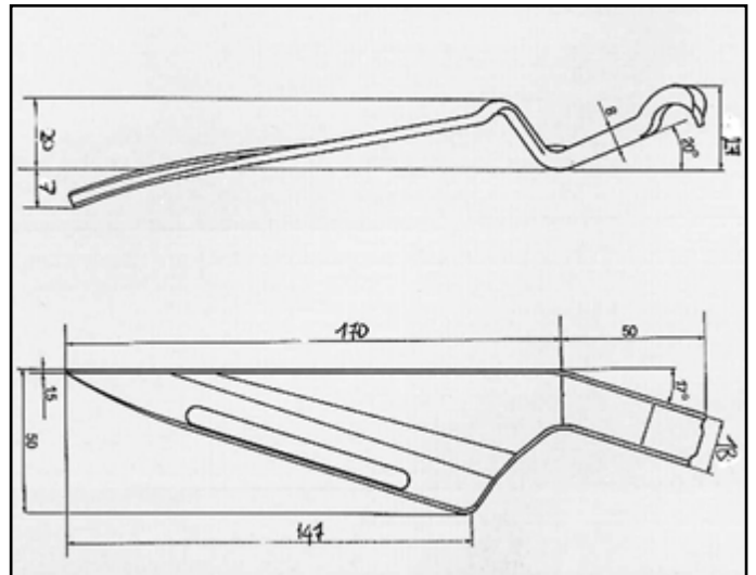
FIAT TURBO DIESEL ATTACCO per centrale COD. AT 241704
