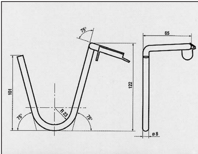
FORD ESCORT / ORION 1300 L - GL - GHIA (9/86-88) FORD ESCORT 1100 (8/86-8/88) ATTACCO per posteriore COD. AT 260234 6160811
