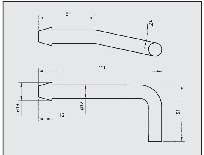
NISSAN PRIMERA 2.0 ATTACCO per posteriore COD. AT 500410
