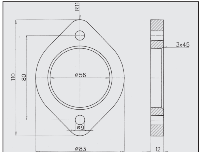
OPEL ASTRA 1.8 16V FLANGIA COD. FL 520935
