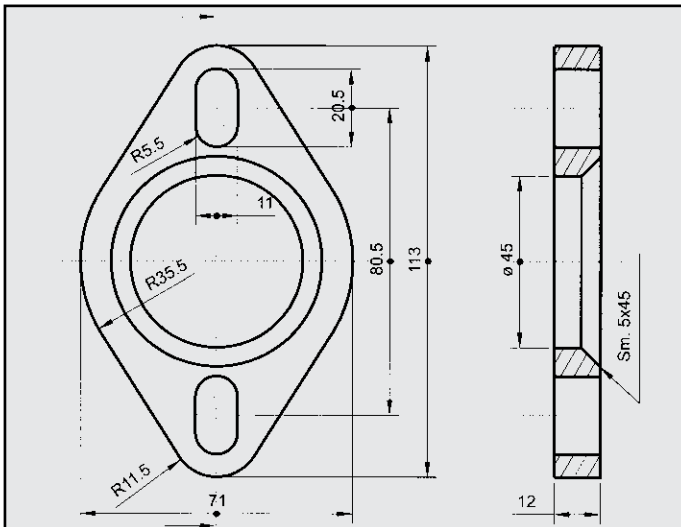
FORD FIESTA FLANGIA COD. FL 260342
