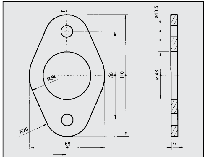
SUZUKI VITARA FLANGIA COD. FL 720109
