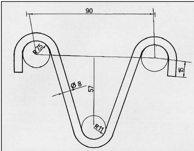
343/345 1400 ATTACCO per posteriore COD. AT 880101
