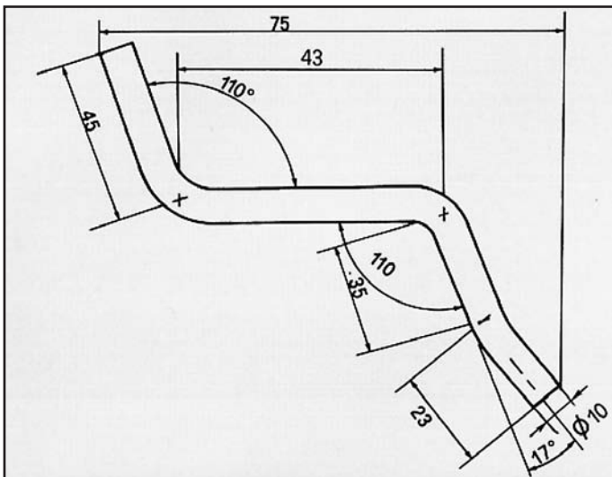
CIVIC/CRX ATTACCO per centrale COD. AT 280410
