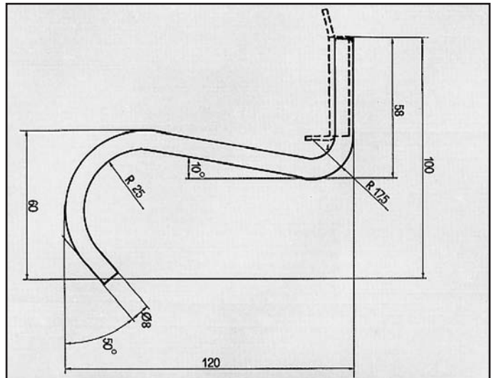
ASCONA ATTACCO posteriore COD. AT 520201/A
