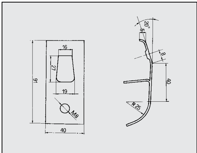
ALFETTA ATTACCO per posteriore COD. AT 02028
