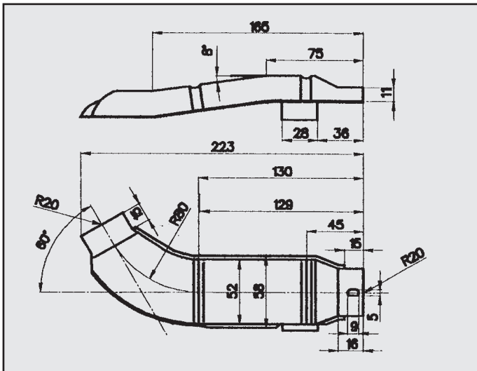
LANCIA Y 10 PROTEZIONE CALORE COD. PC 381002
