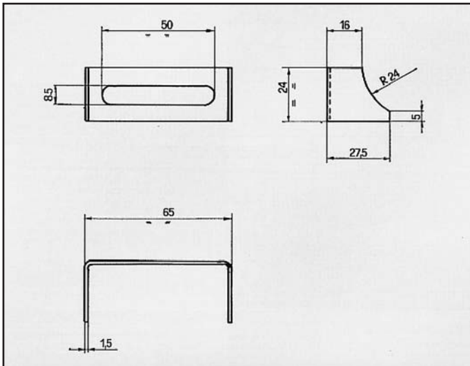
HORIZON ATTACCO per posteriore COD. AT 780205
