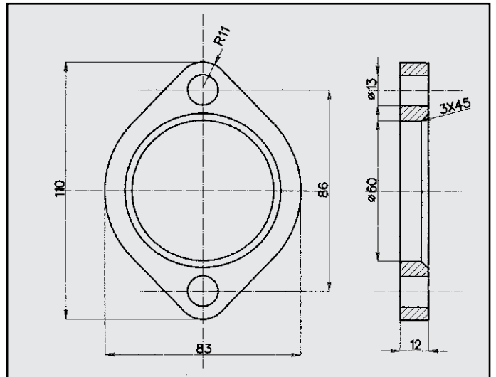
BMW 318 TDS FLANGIA COD. FL 120605
