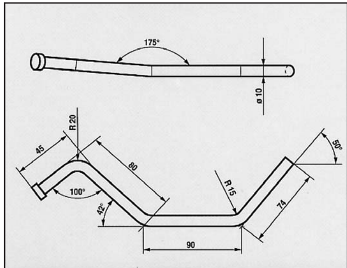
MAZDA 323 / 1986-87 ATTACCO per posteriore COD. AT 420606 E 52540100 B/C/F
