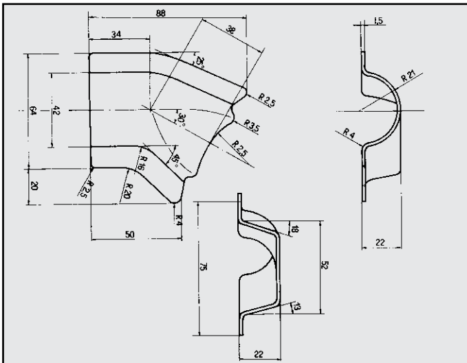
ALFASUD 3ª serie SUPPORTO per attacco COD. AT 020102
