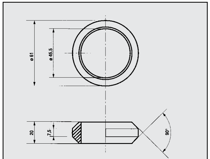
RENAULT R 19 CHAMADE ANELLO per silenziatore centrale COD. AN 600906
