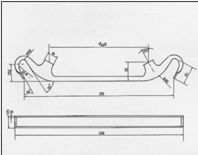
TIPO BENZINA E DIESEL ATTACCO centrale COD. AT 241701
