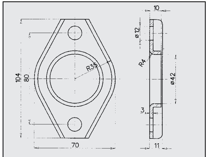
DAEWOO MATIZ - TICO FLANGIA CENTRALE COD. FL 160106
