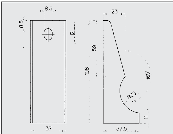
242 BENZINA - 242 DIESEL ATTACCO per centrale COD. AT 241401
