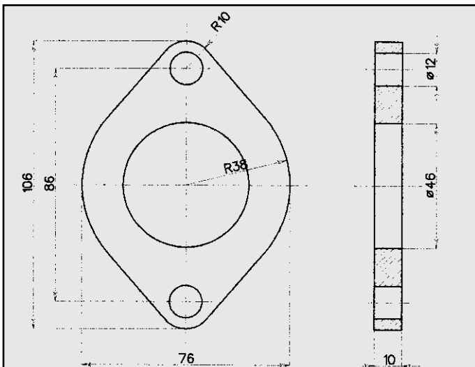
DAEWOO LANOS FLANGIA COD. FL 160204
