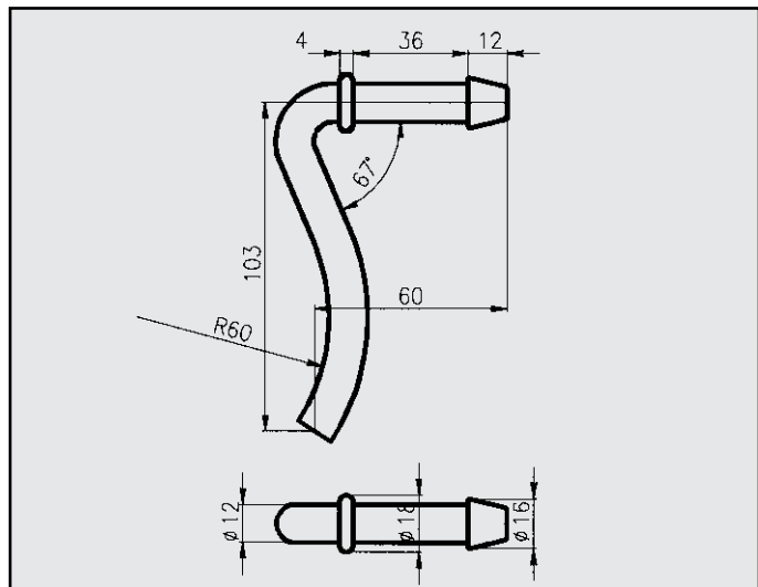
FIAT MULTIPLA ATTACCO COD. AT 242608
