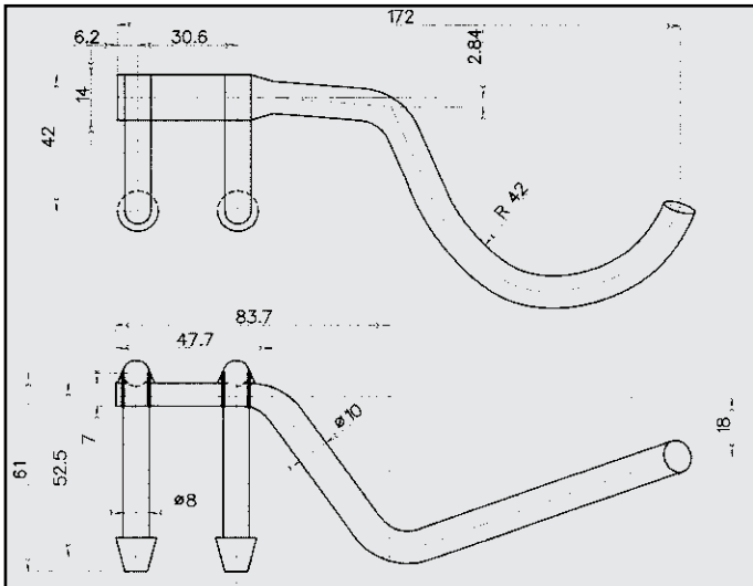
FIAT PUNTO 55/95 ATTACCO COD. AT 242215
