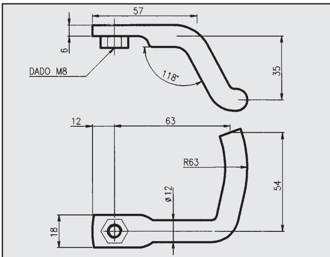
MITSUBISHI PAJERO '90 ATTACCO per posteriore COD. AT 460208
