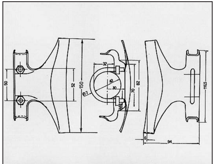
GOLF 1500-1600 BENZINA/DIESEL ATTACCO-RINFORZO per posteriore COD. AT 860116
