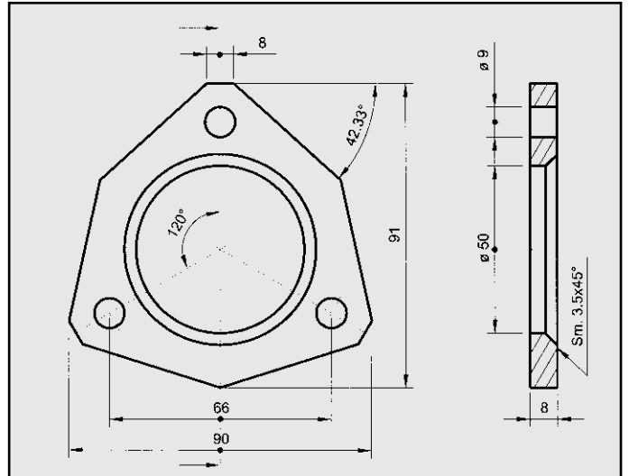
LANCIA THEMA FIAT CROMA FLANGIA COD. FL 380711
