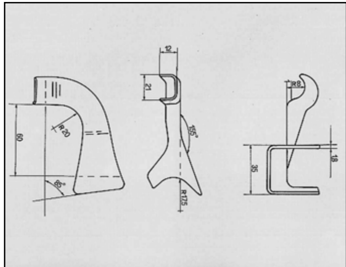
PANDA 45 ATTACCO per posteriore COD. AT 240106 4449004 5888166
