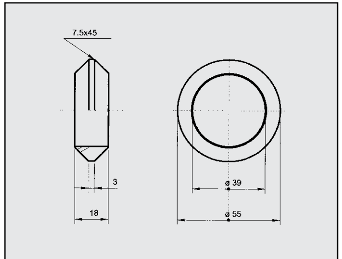
RENAULT R5 ANELLO COD. AN 600120
