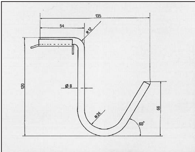
ESCORT 1100/82 ATTACCO per posteriore COD. AT 260209
