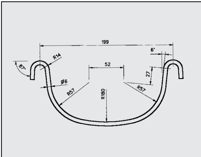
FIAT 132 INIEZIONE ATTACCO per posteriore COD. AT 240704
