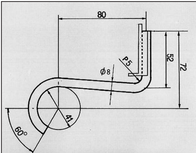
ASCONA ATTACCO per posteriore COD. AT 520201/D
