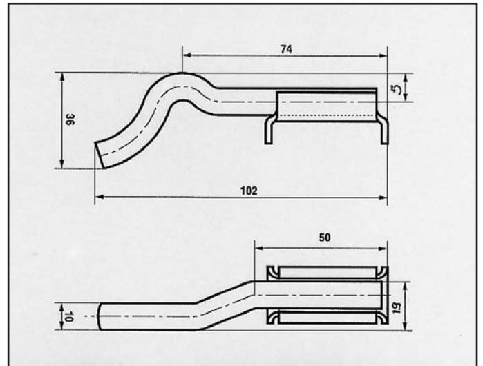
FORD ESCORT 1.4 E ATTACCO COD. AT 260243
