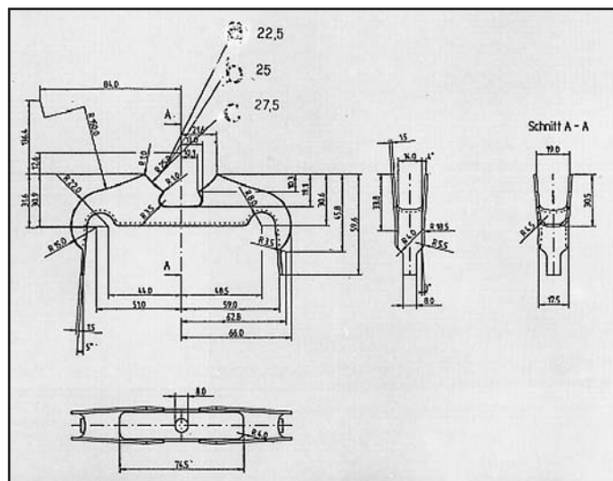
VECTRA 1400-1600-1800 ATTACCO per centrale COD. AT 520803
