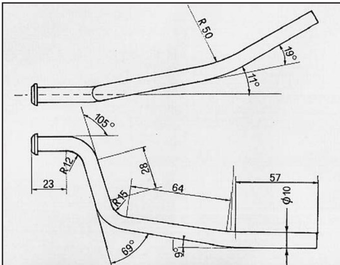
COROLLA ATTACCO per posteriore COD. AT 800401
