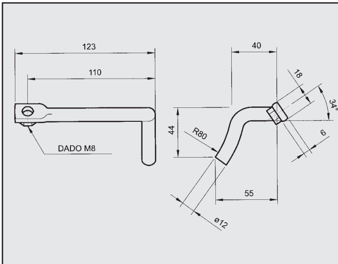
MITSUBISHI SPACE WAGON 2.0 ATTACCO per posteriore COD. AT 460303
