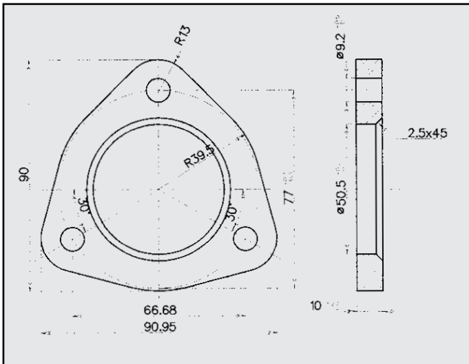
VOLKSWAGEN FLANGIA COD. FL 860027
