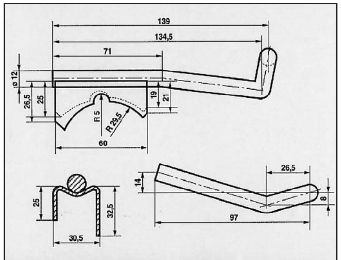
LANCIA DELTA HF ATTACCO posteriore COD. AT 380329
