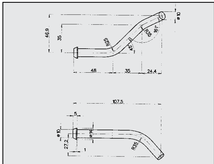
DAEWOO NUBIRA 1.6 ATTACCO POSTERIORE COD. AT 160306
