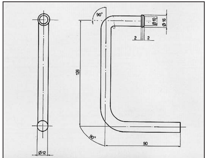
SOARER ATTACCO anteriore per posteriore COD. AT 800701
