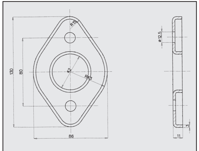
NISSAN FLANGIA COD. FL 500002
