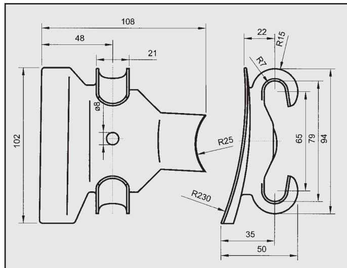
VW GOLF 1.1 1.3 1.6 1.8 ATTACCO RINFORZO per posteriore COD. AT 860106/1
