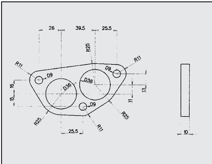
LANCIA / FIAT PUNTO FLANGIA COD. FL 381004
