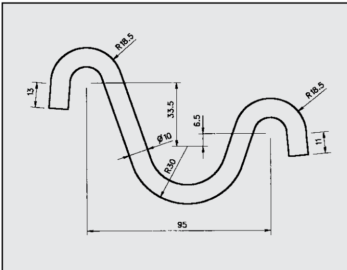
ALFA 33 ATTACCO per posteriore COD. AT 020108
