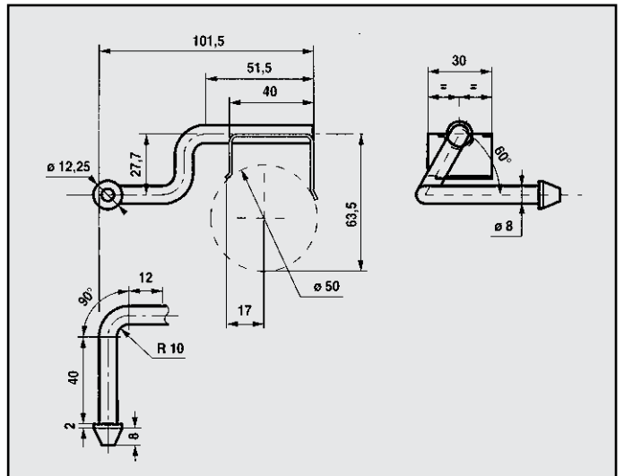
FIAT PUNTO 1.7 TURBO DIESEL ATTACCO COD. AT 242212
