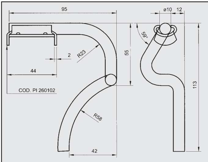
FORD FIESTA 1.8 D KAT. ATTACCO posteriore COD. AT 260330
