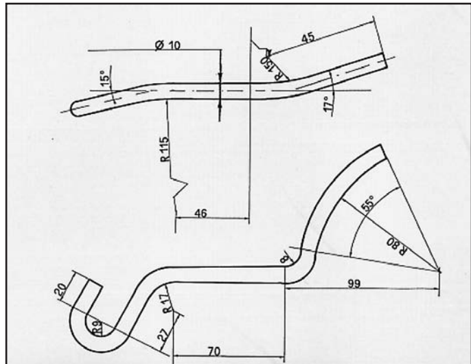
626 ATTACCO per anteriore COD. AT 420501
