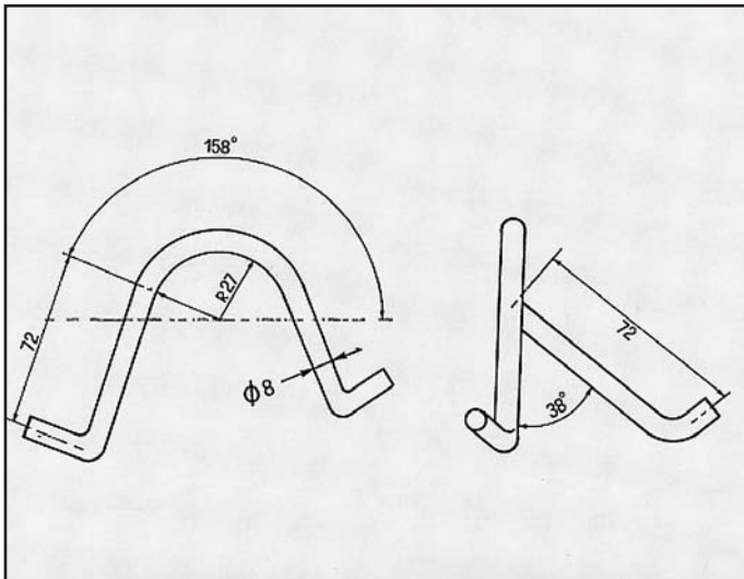
GOLF 16V RINFORZO per centrale COD. R 860113
