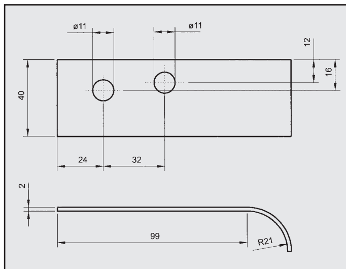
PEUGEOT 305 ATTACCO per tubo COD. AT 541002
