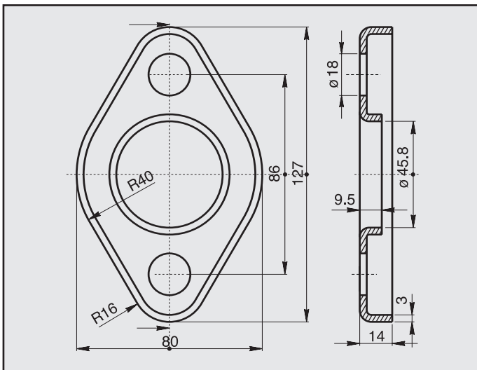
OPEL CORSA FLANGIA COD. FL 520317
