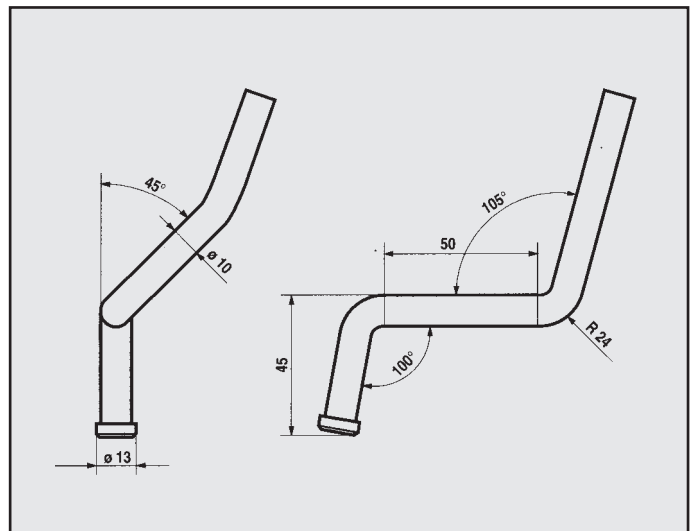
FORD FESTIVA 1987/89 ATTACCO per posteriore COD. AT 260901
