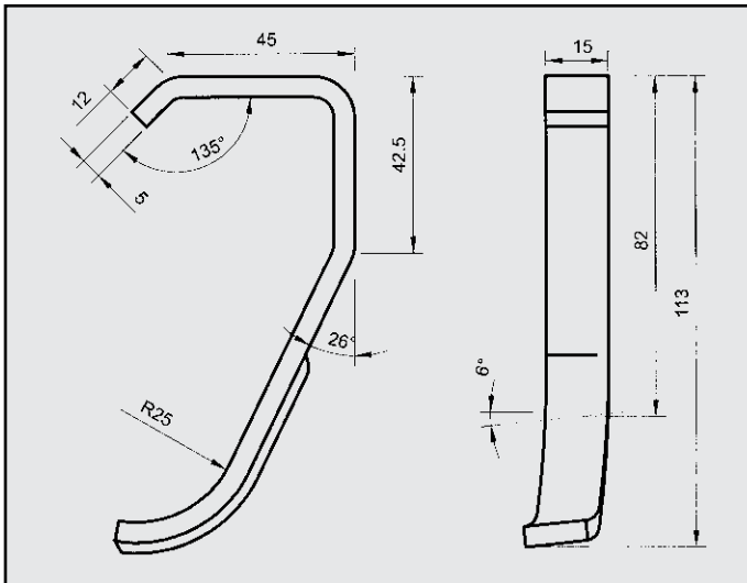
FIAT TEMPRA TD SW CAT. ATTACCO per posteriore COD. AT 241908
