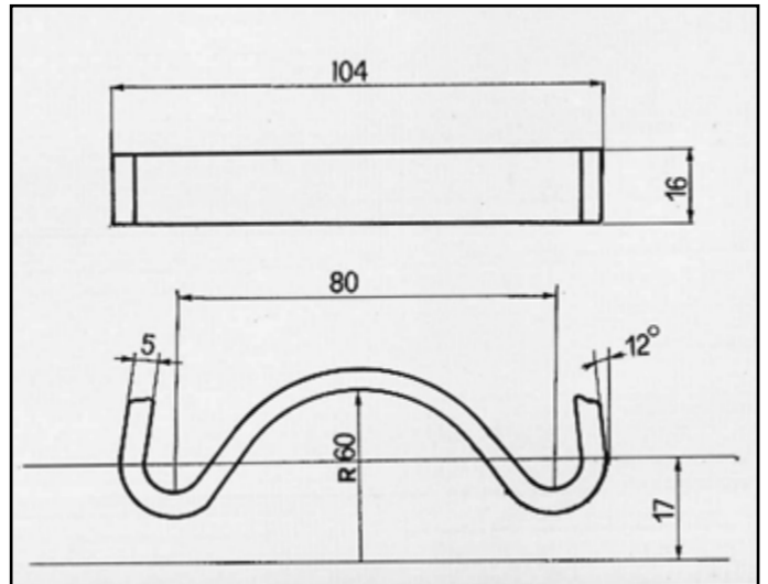
RITMO 1ª SERIE ATTACCO per centrale COD. AT 240801
