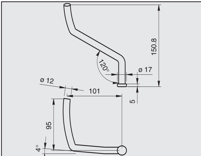
AUDI A6 ATTACCO COD. AT 040801 544681 544594
