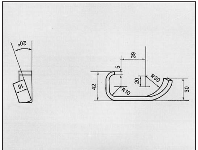
CORSA 1000 2 VOL. ATTACCO per centrale COD. AT 520303
