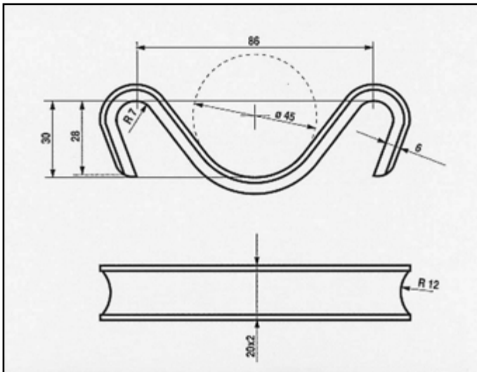
FIAT TALENTO DIESEL 1988 ATTACCO anteriore per posteriore COD. AT 242001
