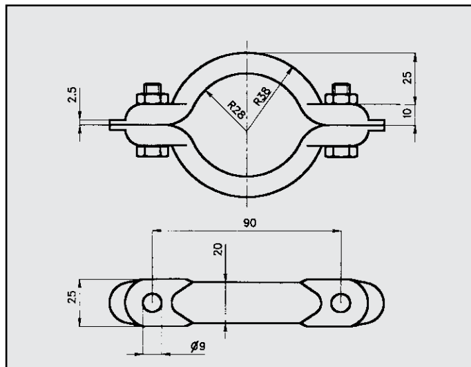
PEUGEOT 205 FASCETTA COD. F 540306
