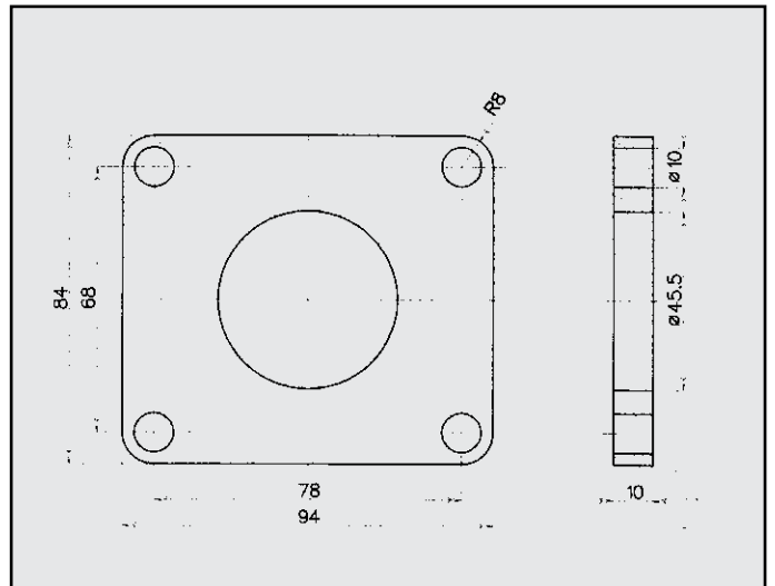
DAEWOO CIELO FLANGIA COD. FL 160401
