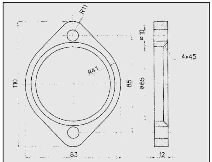
BMW 320 FLANGIA COD. FL 120405
