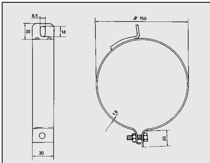
BMW 316 FASCETTA per posteriore COD. F 120101
