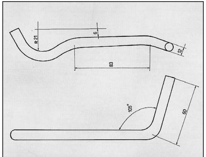
PRISMA 4WD ATTACCO per posteriore COD. AT 380327
