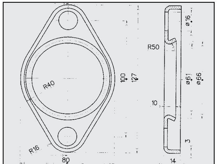
FORD ESCORT ORION FLANGIA COD. FL 260268
