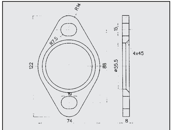
ROVER 214 -414 FLANGIA COD. FL 620611
