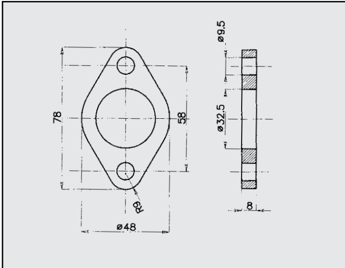
VOLKSWAGEN FLANGIA COD. FL 860034
