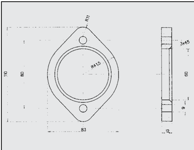
CENTRALE OPEL OMEGA 2.0 FLANGIA COD. FL 520617
