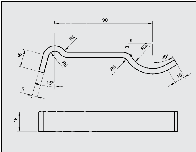
FIAT TIPO 1.6 S SX '91-'92 ATTACCO COD. AT 241716
