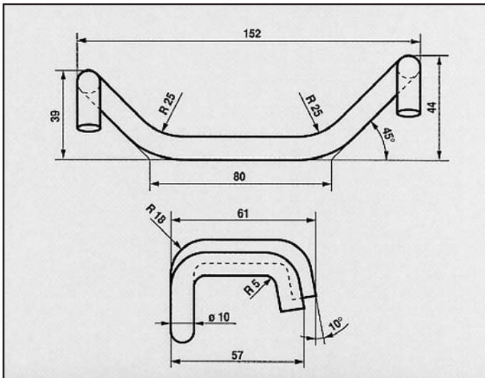
HONDA INTEGRA 1986/88 ATTACCO per posteriore COD. AT 281001
