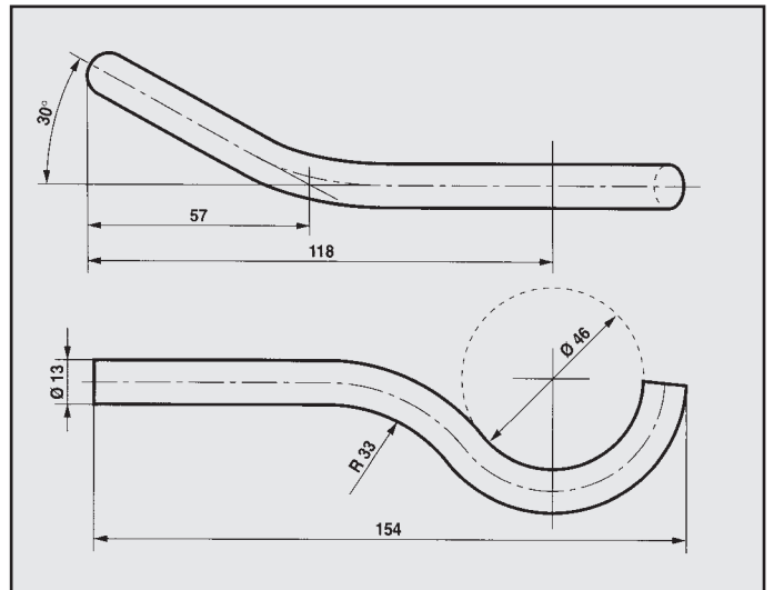
OPEL CORSA ATTACCO COD. AT 520309
