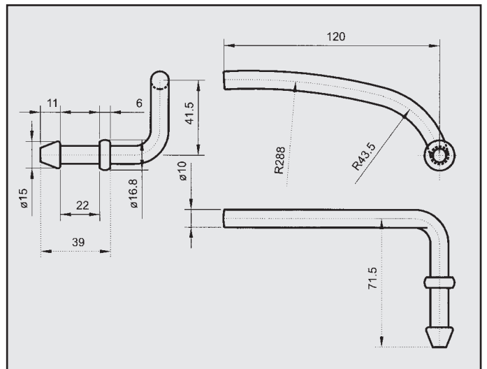
FORD FIESTA 1,2i CAT '95 ATTACCO per posteriore COD. AT 260335
