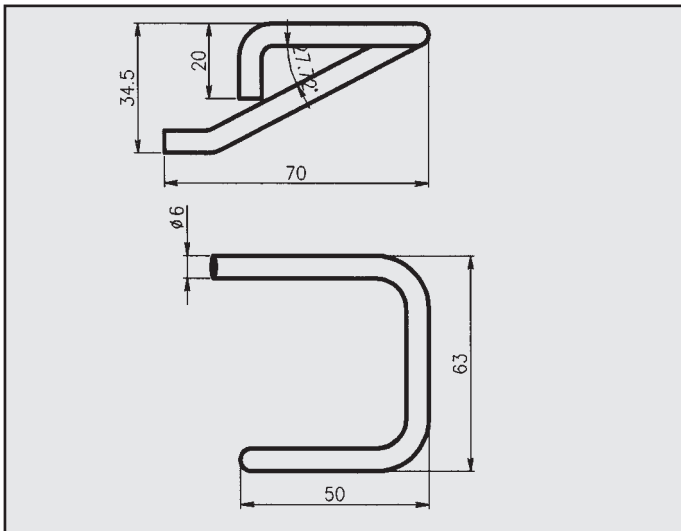
LIGIER ATTACCO COD. AT 390002
