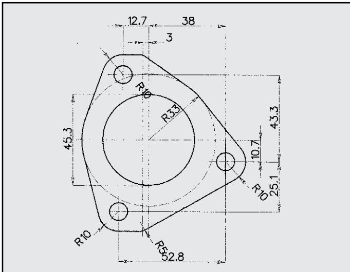
FIAT BRAVO / BRAVA FLANGIA COD. FL 242327
