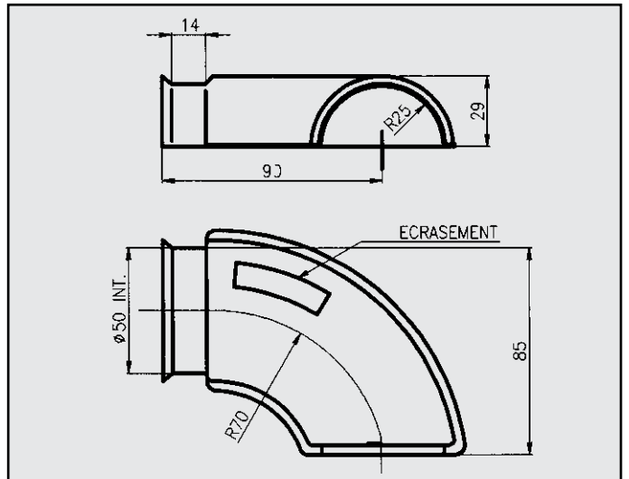
FIAT BRAVO PROTEZIONE CALORE COD. PC 242316
