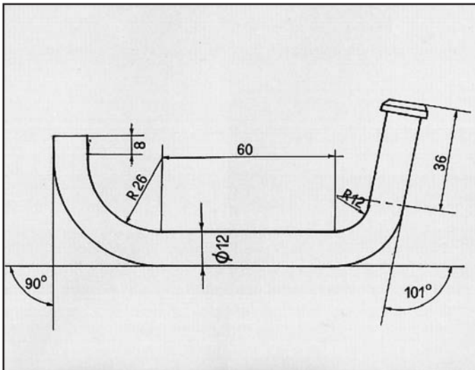
STARLET ATTACCO per posteriore COD. AT 800803
