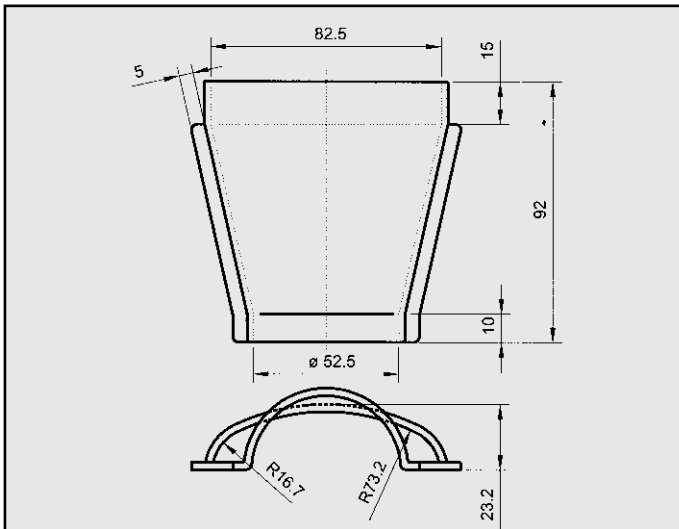
BMW 520i KAT MANICOTTO COD. M 120211
