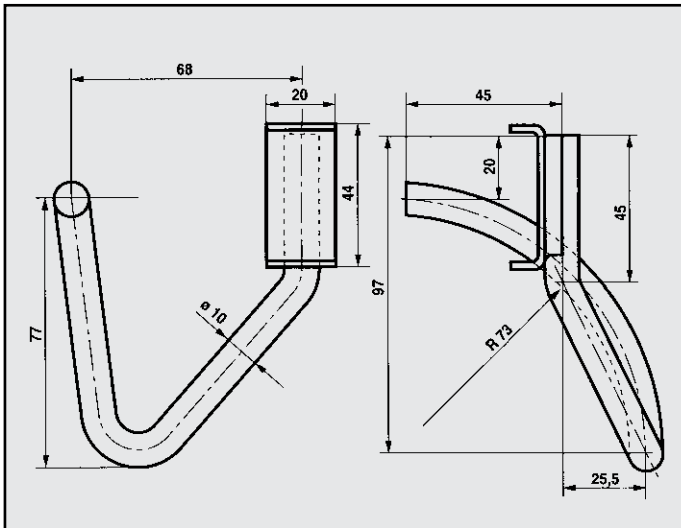
CITROEN XANTIA 1.6 CAT. ATTACCO posteriore COD. AT 141001 96164115
