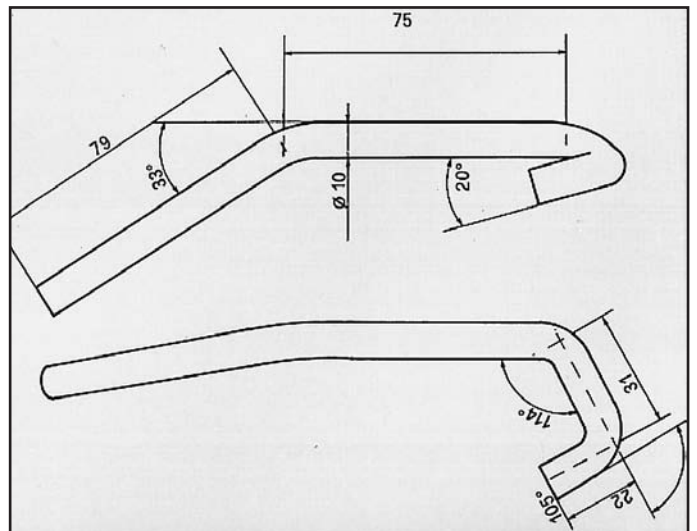
ACTY ATTACCO per posteriore COD. AT 280205
